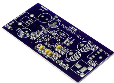
半完成基板 (80x36x1.6mm) (x1)
