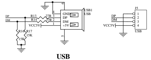
USB
