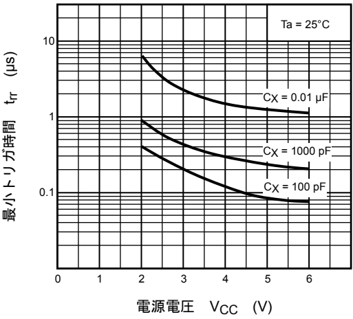
最小トリガ時間 - 電源電圧特性 (標準)
