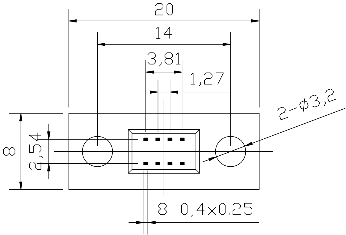
底视图
