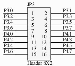
I/O口扩展电路
