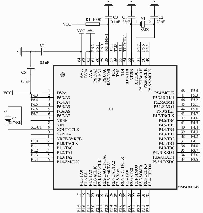
MSP430F149最小系统电路
