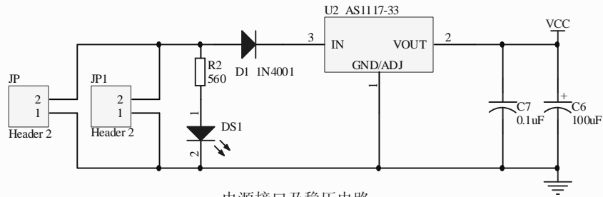
电源接口及稳压电路
