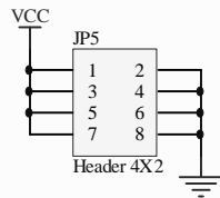
3.3V输出，外部设备电源供给
