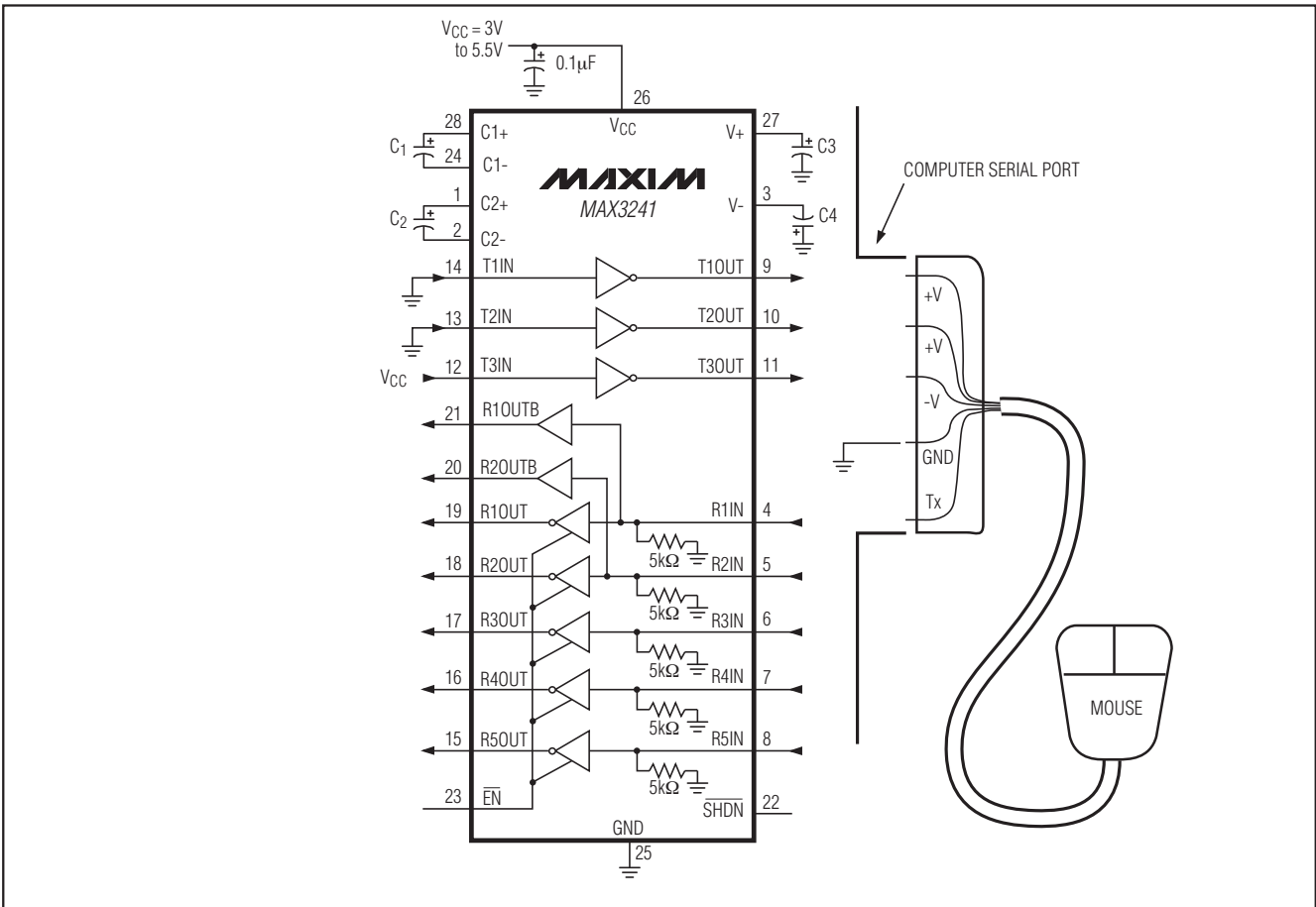
図4b. マウスの試験回路
