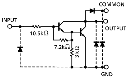
TD62004P/AP/F/AF
