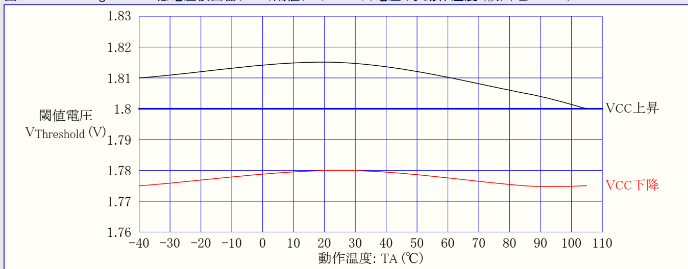
図31-267. ATmega168PA: 低電圧検出器(BOD)閾値(スレッショルト)電圧 対 動作温度 (検出電圧1.8V)
