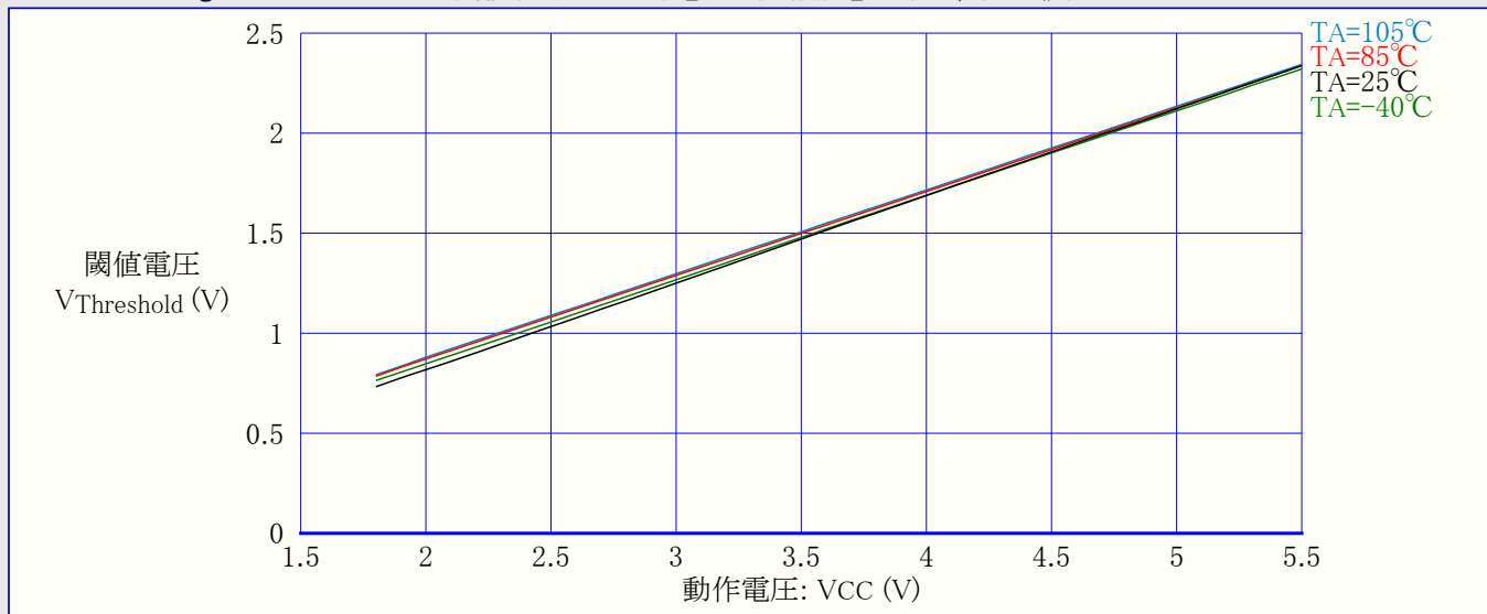
図32-74. ATmega88PA: RESET入力閾値(スレッショルド)電圧 対 動作電圧 (VIL,0読み値)
