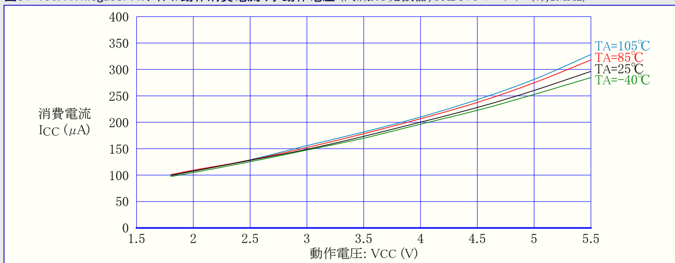
図31-150. ATmega88PA: アイドル動作消費電流 対 動作電圧 (内蔵RC発振器, CKDIV8=プログラム(0), 1MHz)
