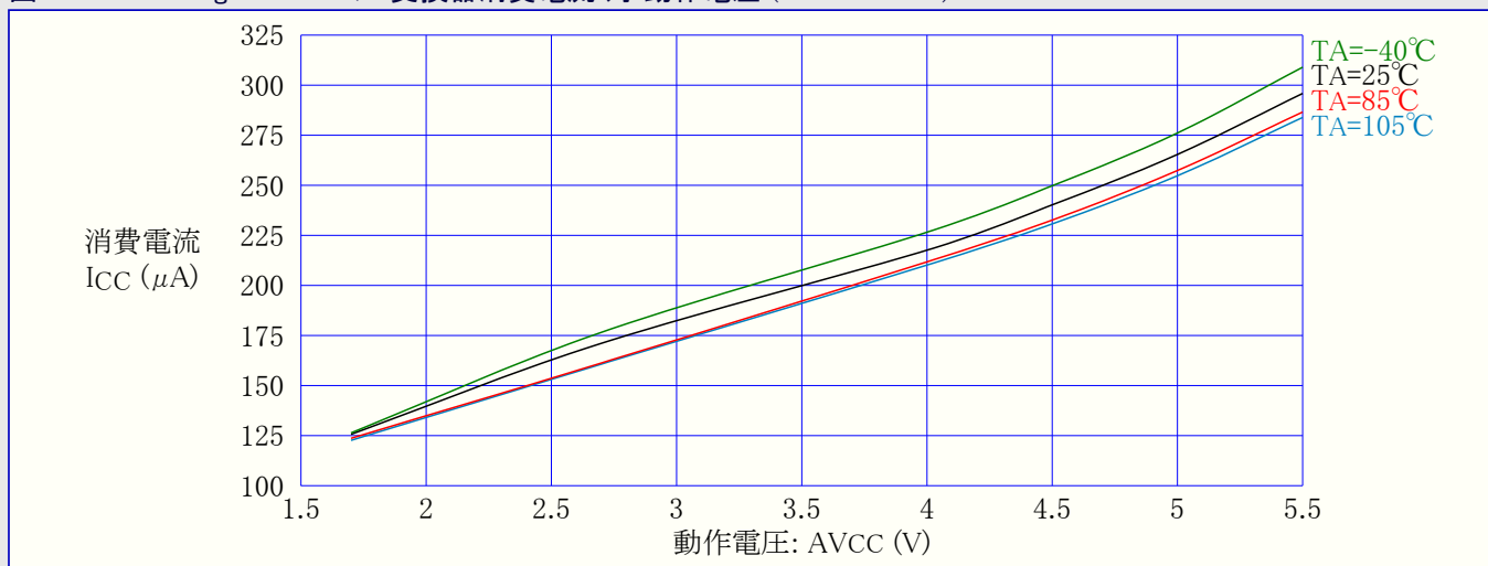
図31-371. ATmega328PA: A/D変換器消費電流 対 動作電圧 (AREF=AVCC)
