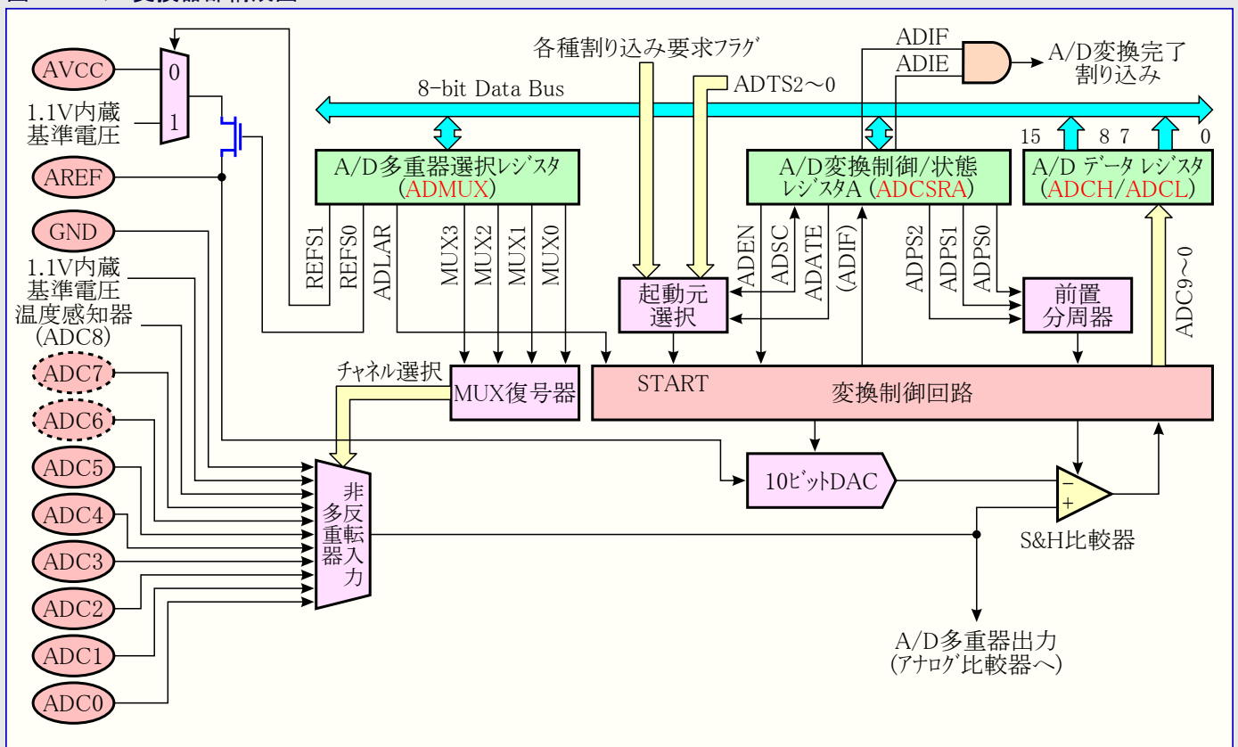
図24-1. A/D変換器部構成図
