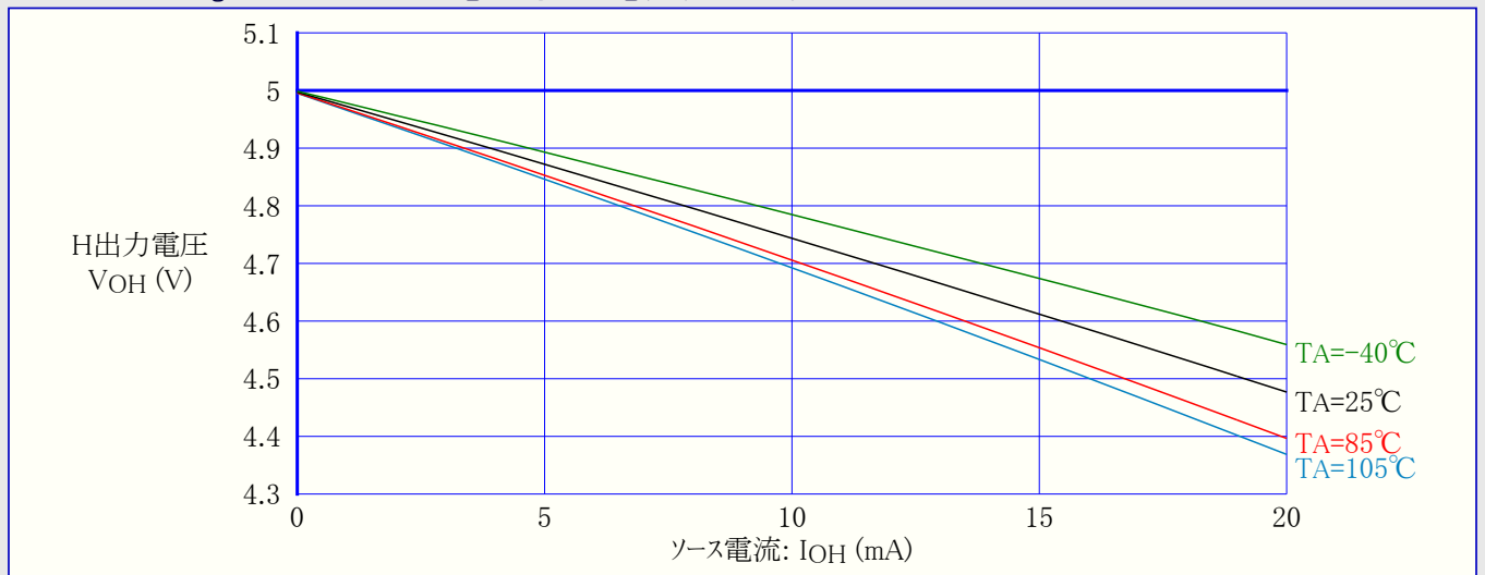
図31-355. ATmega328P:I/Oピン出力電圧 対 ソース電流 (VCC=5V)
