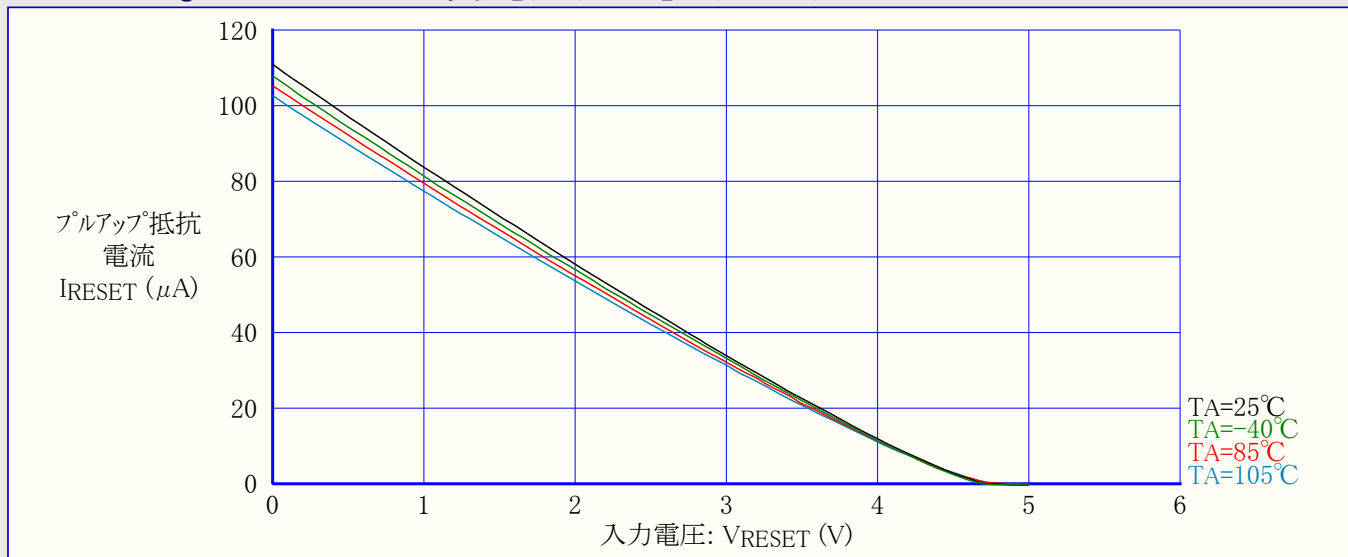
図32-65. ATmega88PA: RESETプルアップ抵抗電流 対 入力電圧 (VCC=5V)
