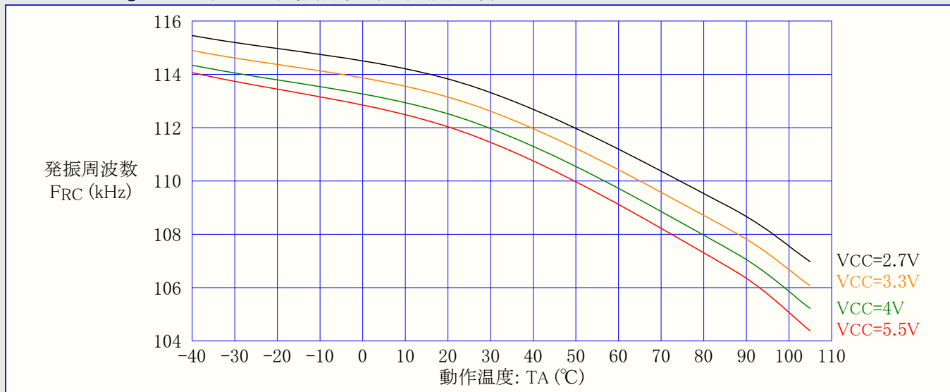
図31-82. ATmega48PA: ウォッチドッグ発振器周波数 対 動作温度
