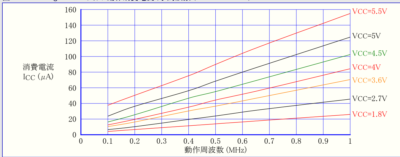
図32-97. ATmega168PA: アイドル動作消費電流 対 周波数 (100kHz~1MHz)
