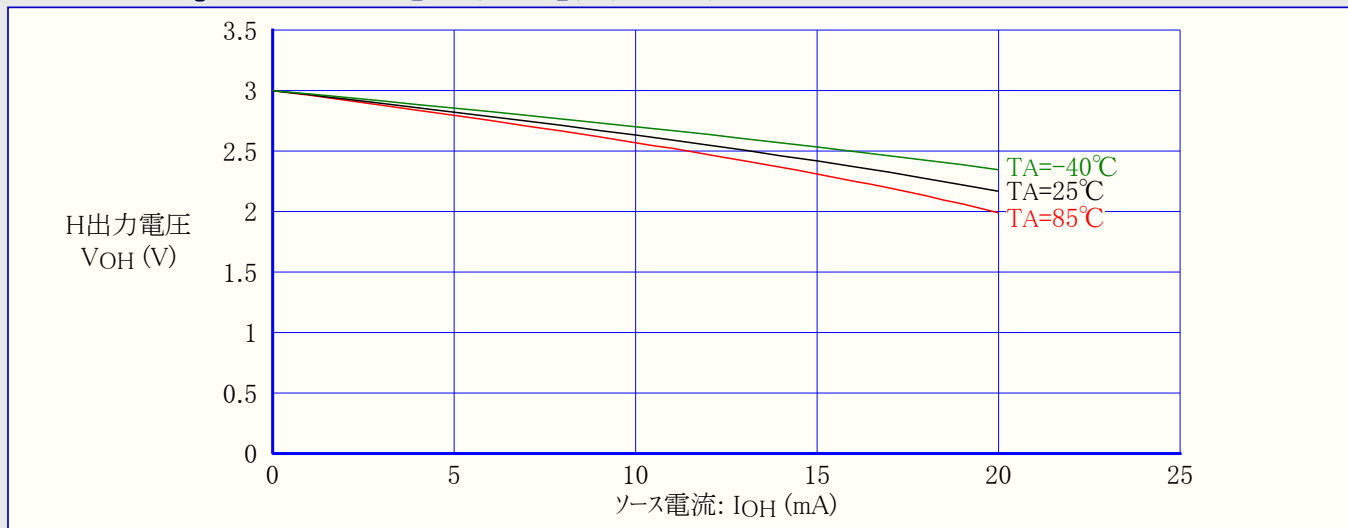
図31-307. ATmega328:I/Oピン出力電圧 対 ソース電流 (VCC=3V)
