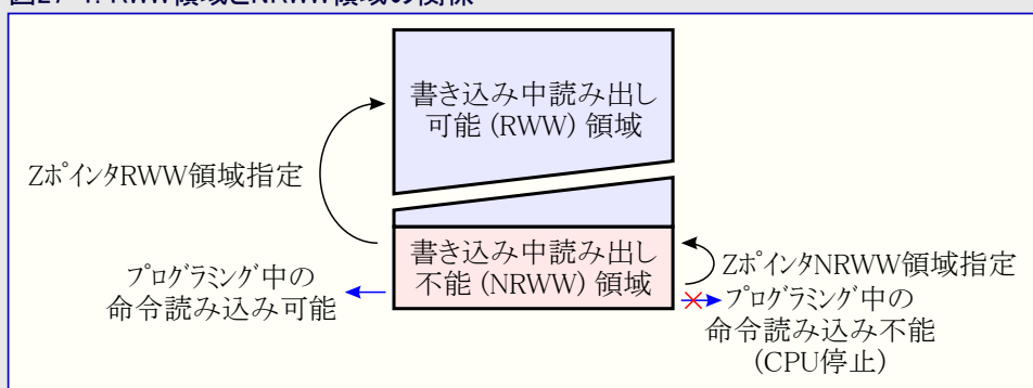
図27-1. RWW領域とNRWW領域の関係
