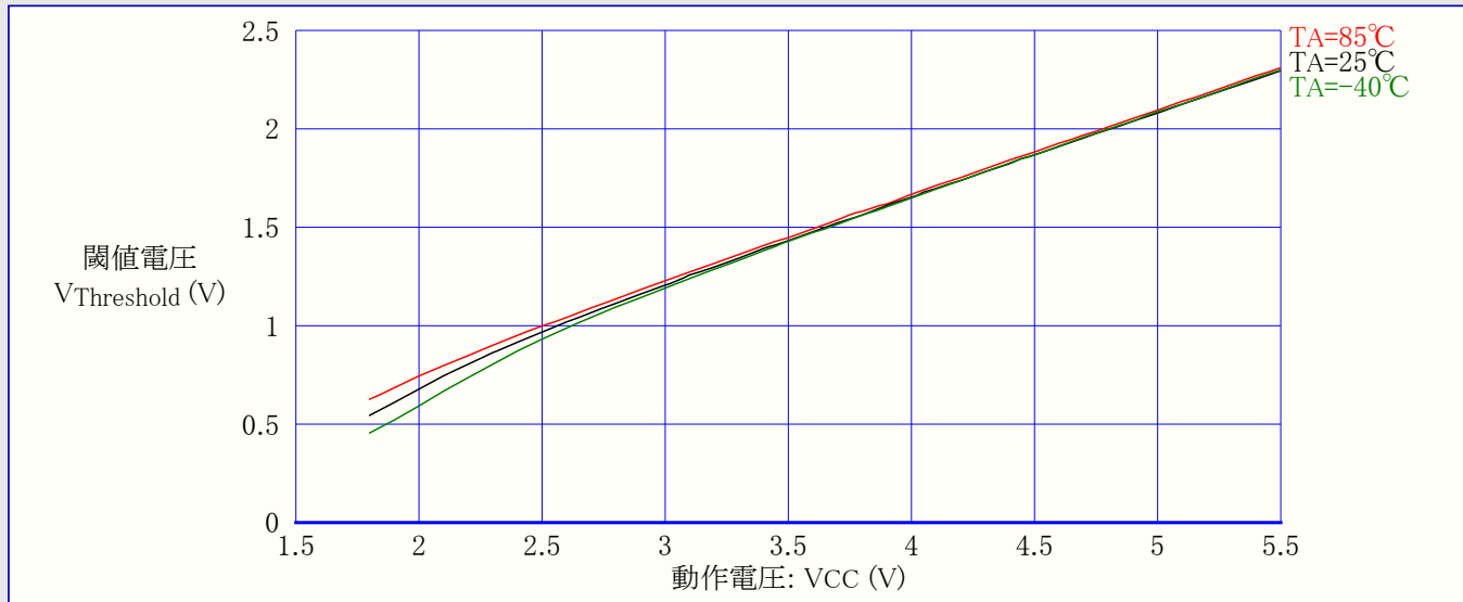
図31-310. ATmega328:I/Oピン入力閾値(スレッショルド)電圧 対 動作電圧 (VIL,0読み値)
