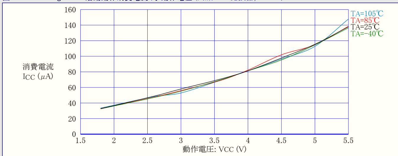
図31-334. ATmega328P: 活動動作消費電流 対 動作電圧 (内蔵WDT発振器, 128kHz)
