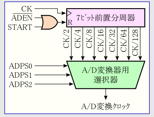
図24-3. A/D変換前置分周器部構成
