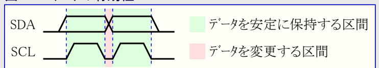
図22-2. データの有効性
