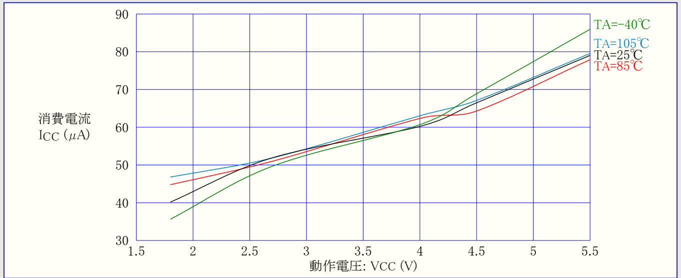
図32-135. ATmega168PA: 低電圧検出器(BOD)消費電流 対 動作電圧
