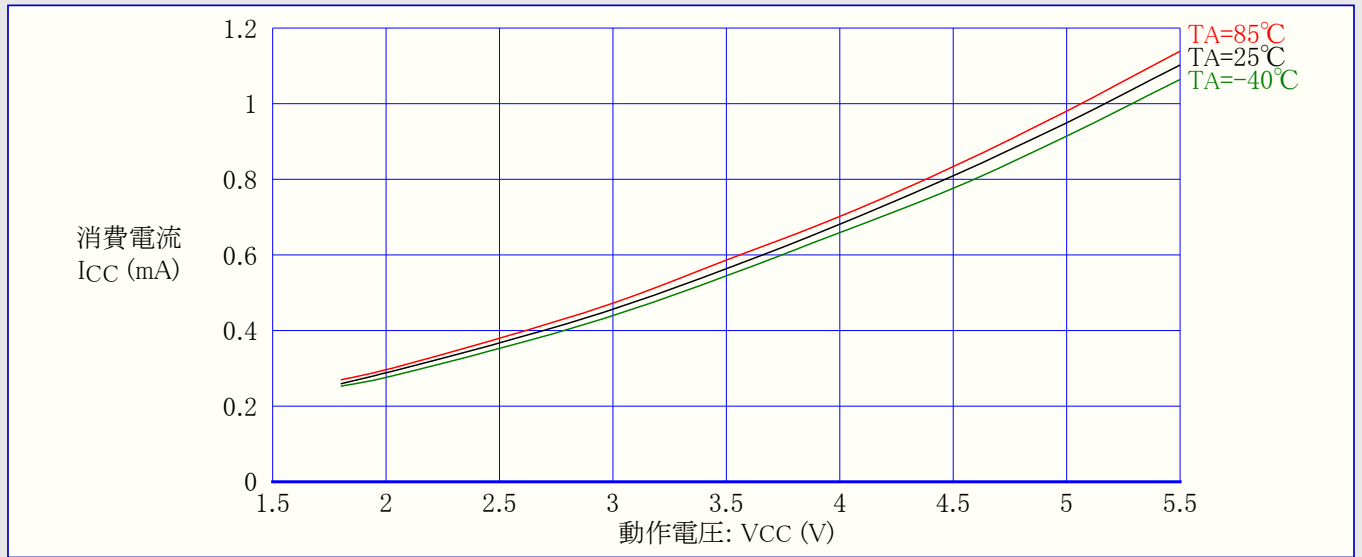
図31-98. ATmega88A: 活動動作消費電流 対 動作電圧 (内蔵RC発振器,CKDIV8=プログラム(0),1MHz)
