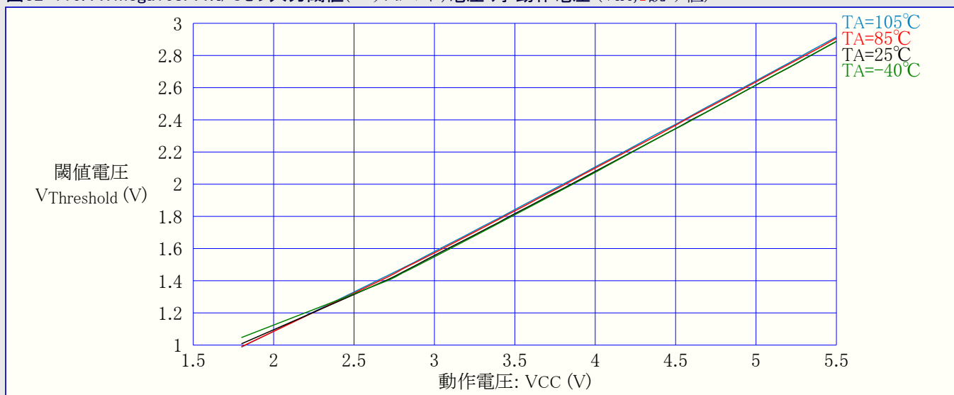
図32-116. ATmega168PA:I/Oピン入力閾値(スレッショルド)電圧 対 動作電圧 ( V_{IH,1} 読み値)
