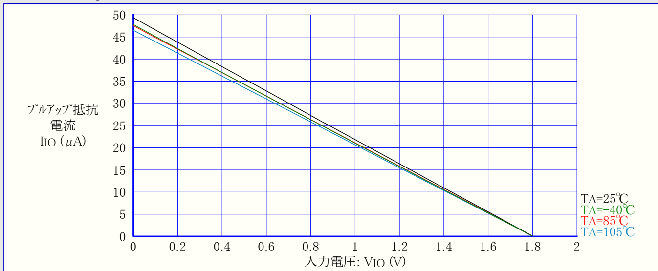
図31-346. ATmega328P:I/Oピンプルアップ抵抗電流 対 入力電圧 ( V_{CC}=1.8V )
