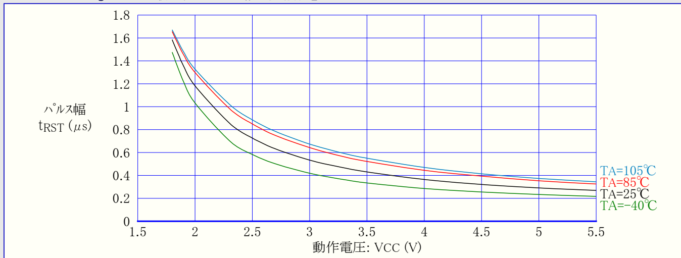
図32-139. ATmega168PA:最小リセットパルス幅 対 動作電圧
