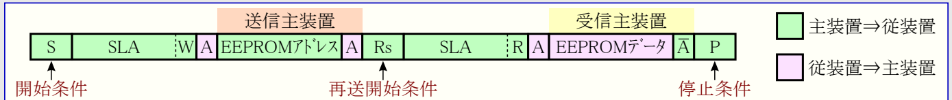
図22-19. 直列EEPROMアクセスでの各種TWI動作種別の組み合わせ
