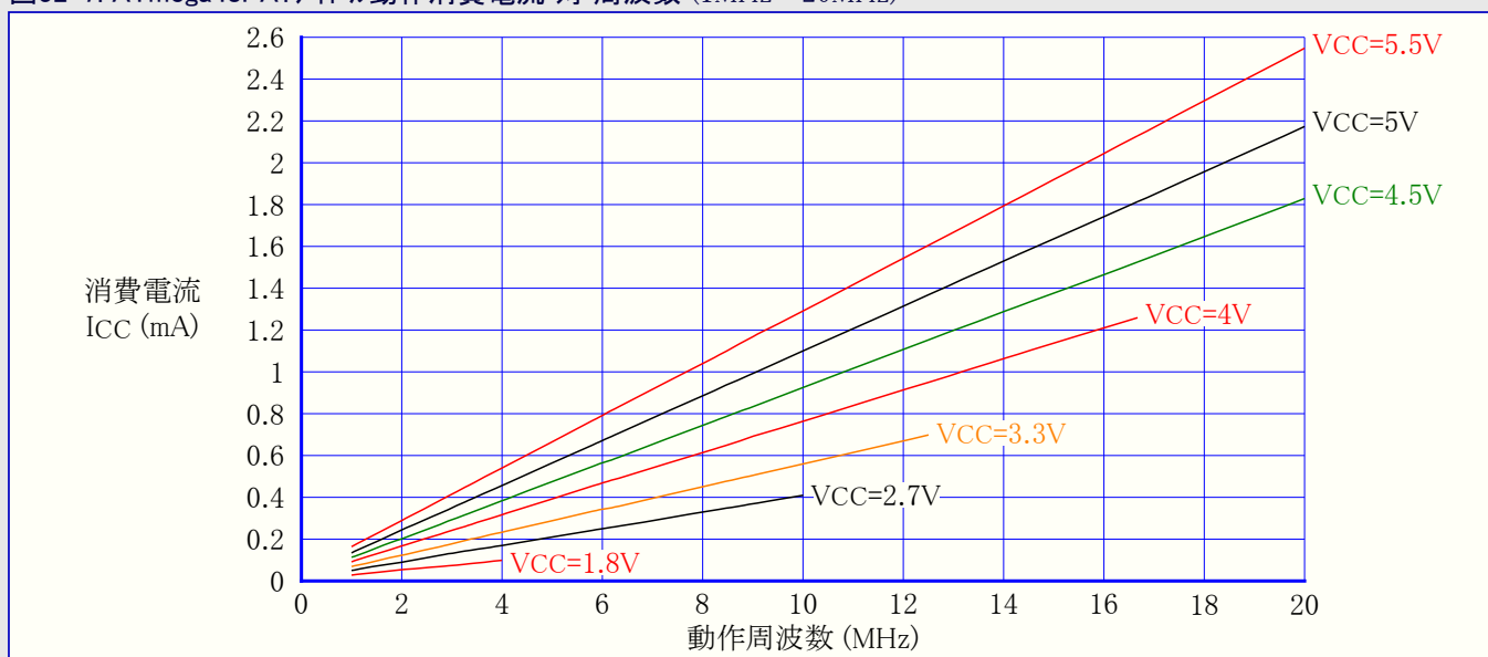
図32-7. ATmega48PA: アイドル動作消費電流 対 周波数 (1MHz~20MHz)
