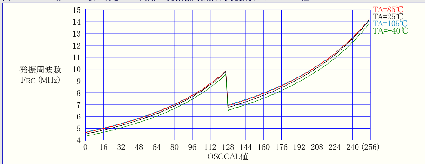
図32-38. ATmega48PA: 校正付き8MHz内蔵RC発振器周波数 対 発振校正(OSCCAL)値
