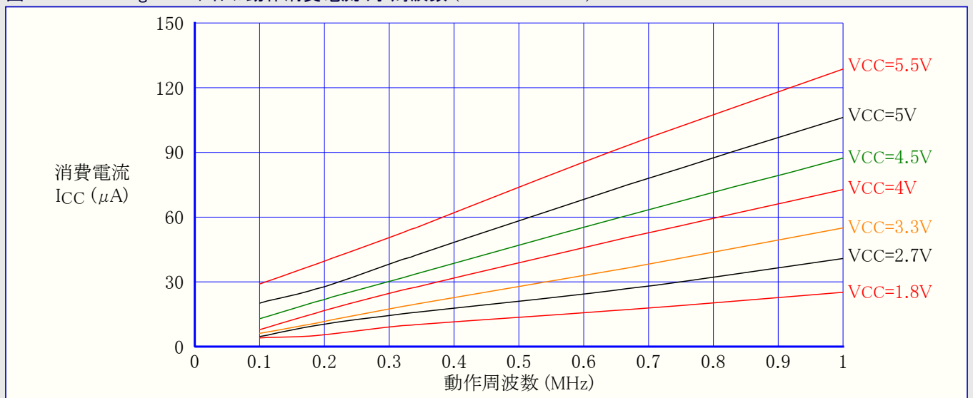
図31-100. ATmega88A: アイドル動作消費電流 対 周波数 (100kHz~1MHz)
