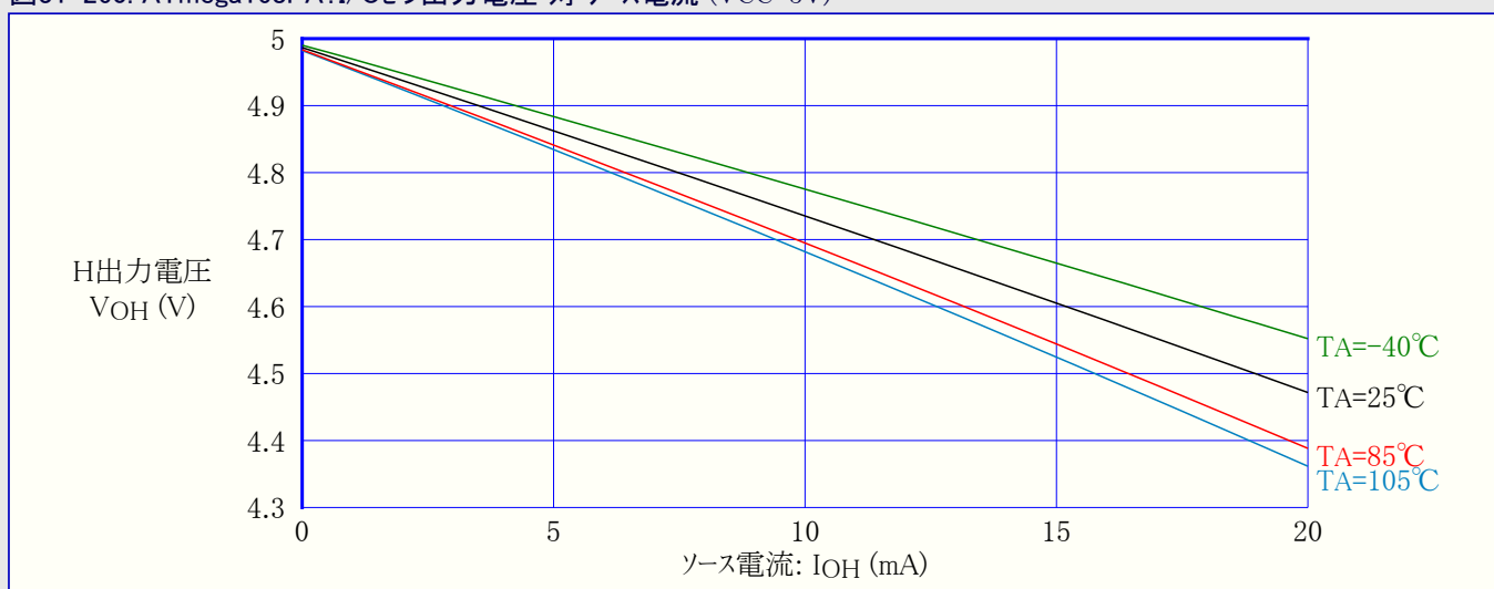
図31-260. ATmega168PA:I/Oピン出力電圧 対 ソース電流 (VCC=5V)
