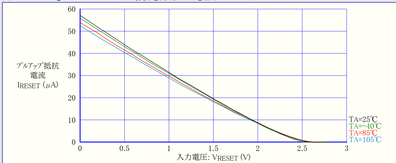
図31-160. ATmega88PA:RESETプルアップ抵抗電流 対 入力電圧 (VCC=2.7V)
