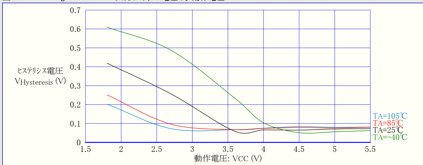
図31-361. ATmega328P: RESET入力ヒステリシス電圧 対 動作電圧
