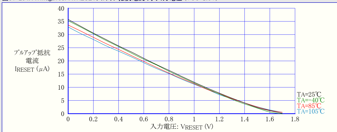
図31-254. ATmega168PA:RESETプルアップ抵抗電流 対 入力電圧 (VCC=1.8V)
