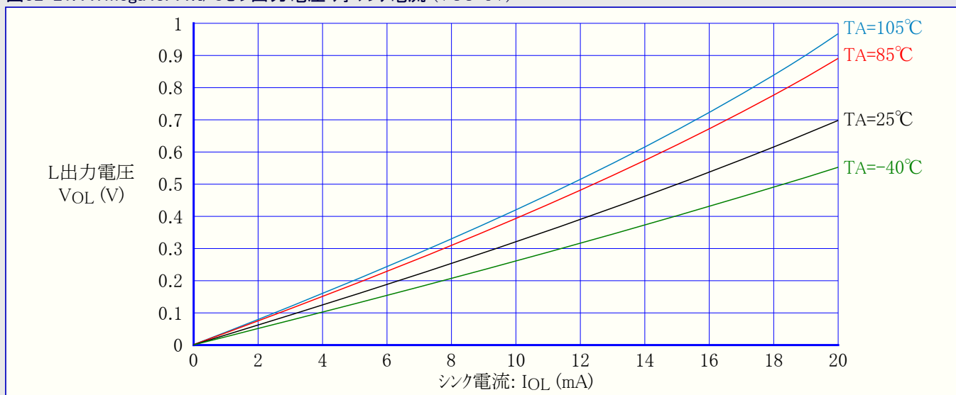
図32-21. ATmega48PA: I/Oピン出力電圧 対 シンク電流 (VCC=3V)
