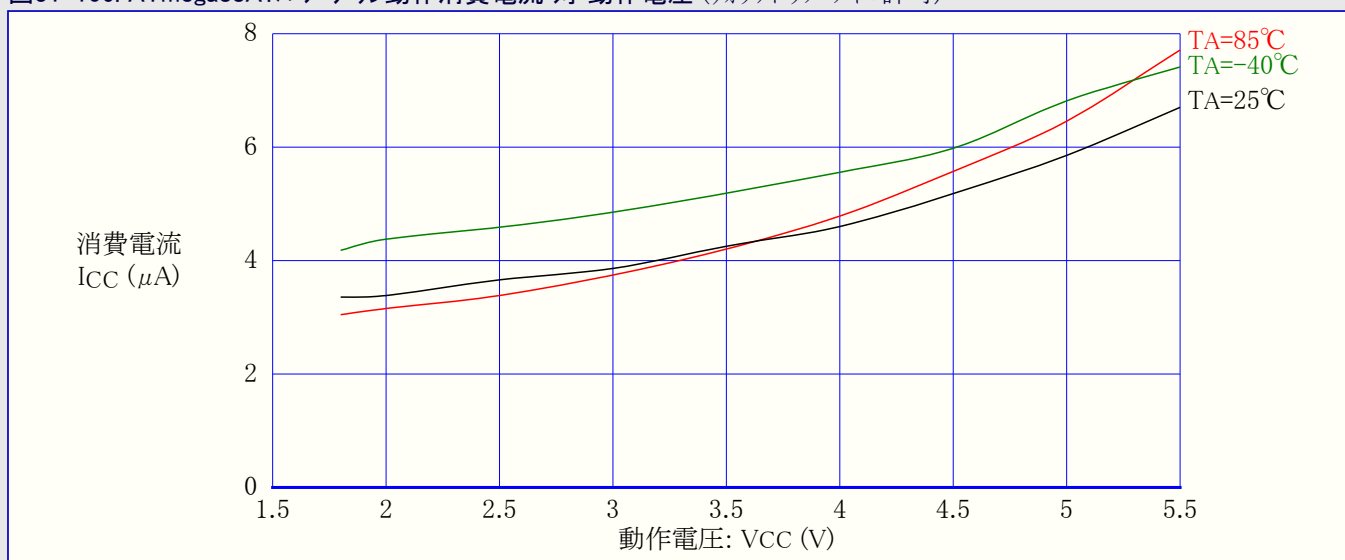
図31-106. ATmega88A: パワーダウン動作消費電流 対 動作電圧 (ウォッチドッグ タイマ許可)
