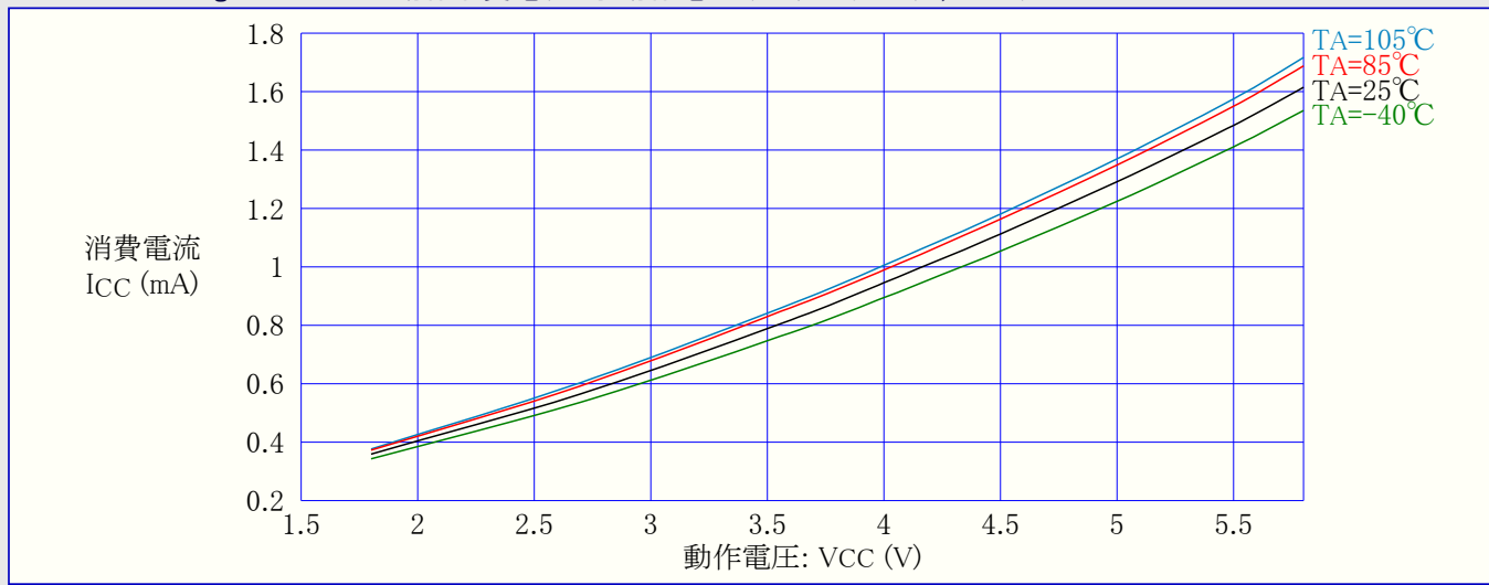
図32-149. ATmega328P:アトル動作消費電流 対 動作電圧 (内蔵RC発振器,8MHz)
