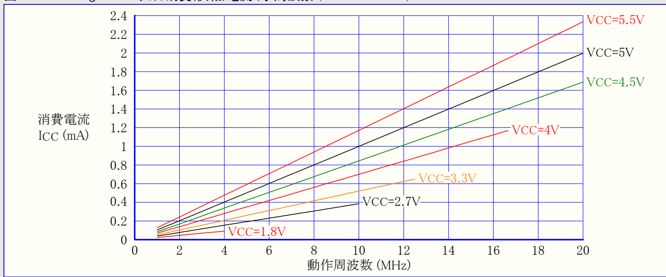
図31-93. ATmega48PA:リセット消費(供給)電流 対 周波数 (1MHz~20MHz)
