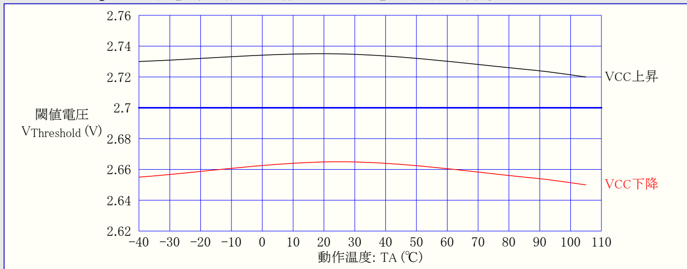
図31-268. ATmega168PA: 低電圧検出器(BOD)閾値(スレッシュホールド)電圧 対 動作温度 (検出電圧2.7V)
