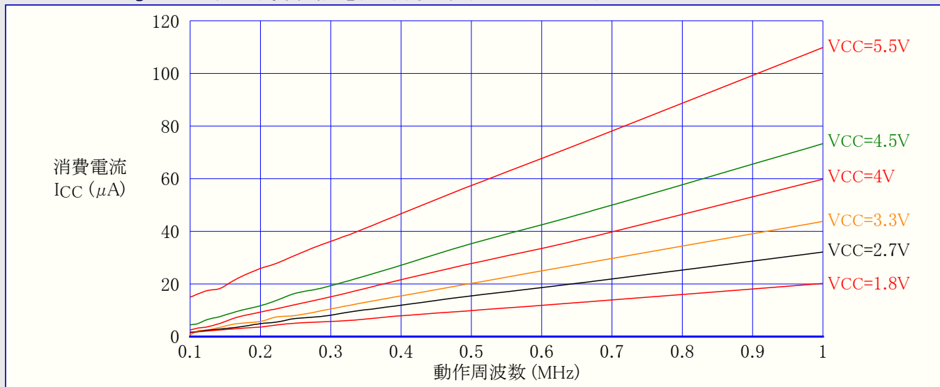
図32-137. ATmega168PA:リセット消費(供給)電流 対 周波数 (100kHz~1MHz)
