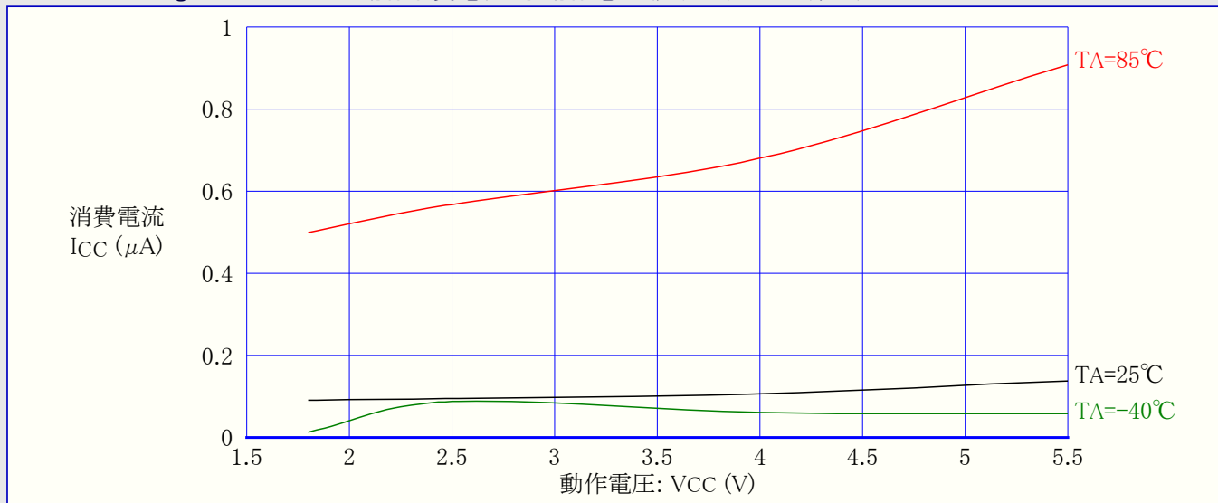
図31-200. ATmega168A: パワーダウン動作消費電流 対 動作電圧 (ウォッチドッグ タイマ禁止)
