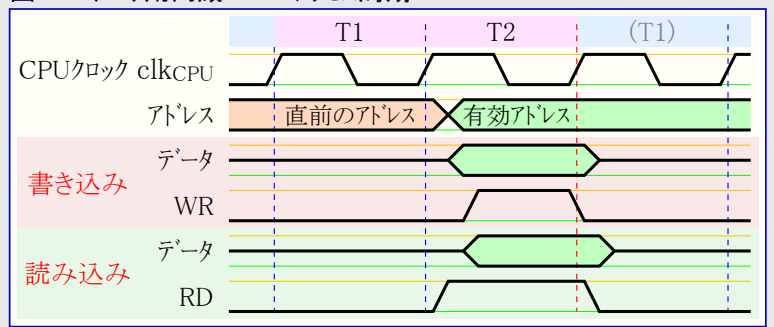
図8-4. データ用内蔵SRAMアクセス周期
