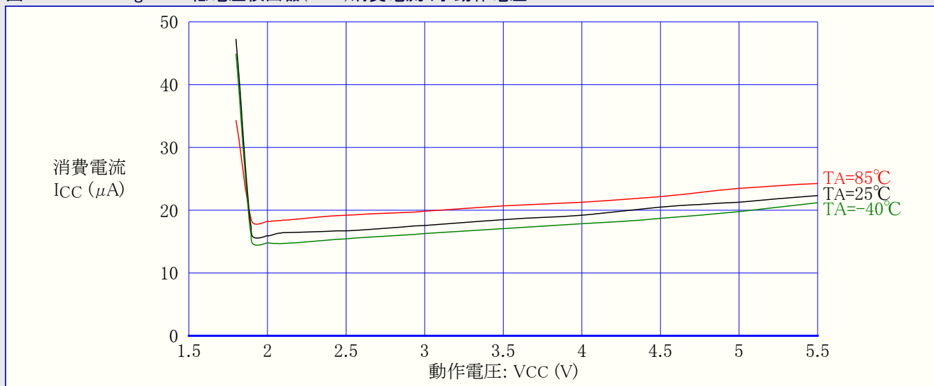
図31-137. ATmega88A: 低電圧検出器(BOD)消費電流 対 動作電圧
