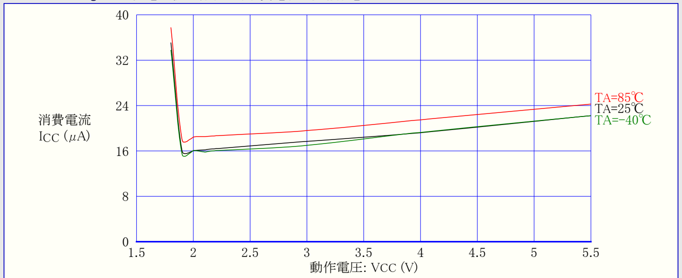
図31-43. ATmega48A: 低電圧検出器(BOD)消費電流 対 動作電圧
