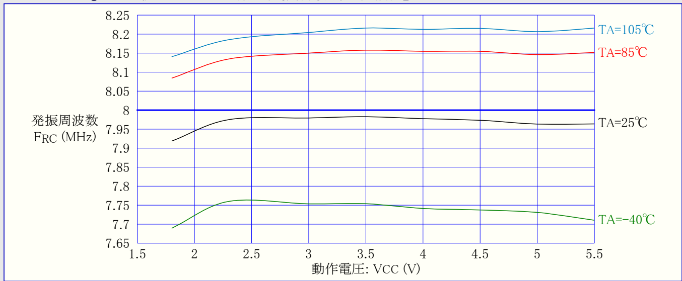
図32-36. ATmega48PA: 校正付き8MHz内蔵RC発振器周波数 対 動作電圧
