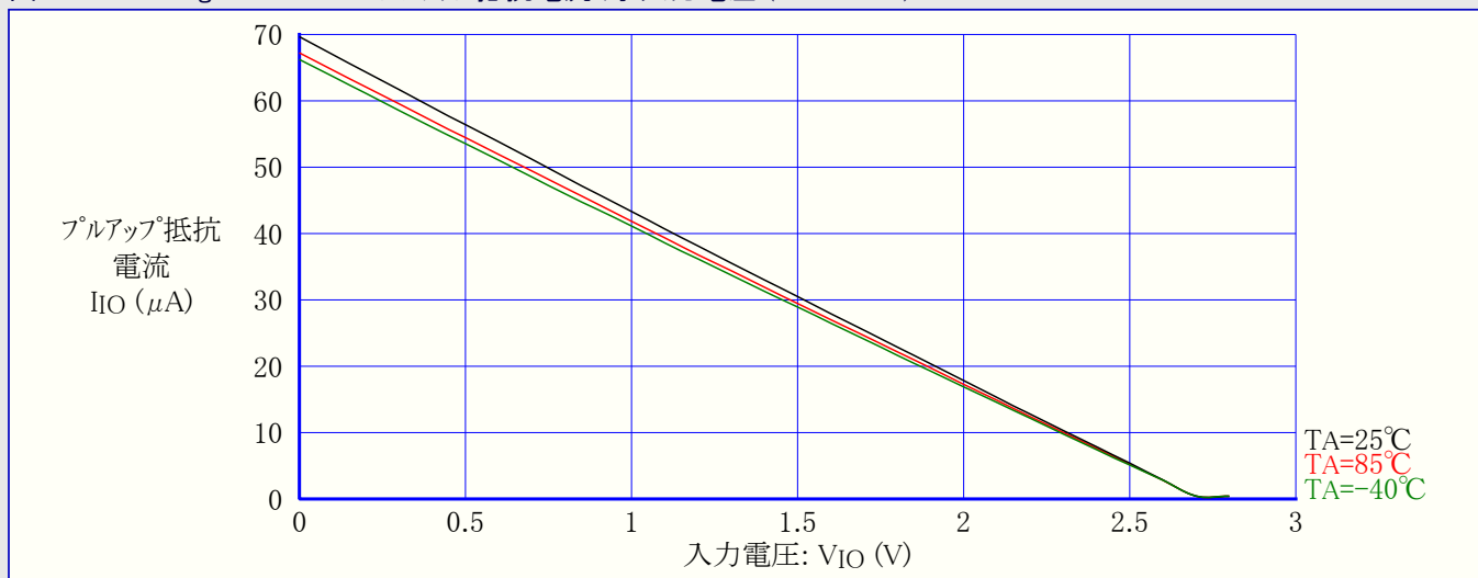
図31-16. ATmega48A:I/Oピンプルアップ抵抗電流 対 入力電圧 ( V_{CC}=2.7V )
