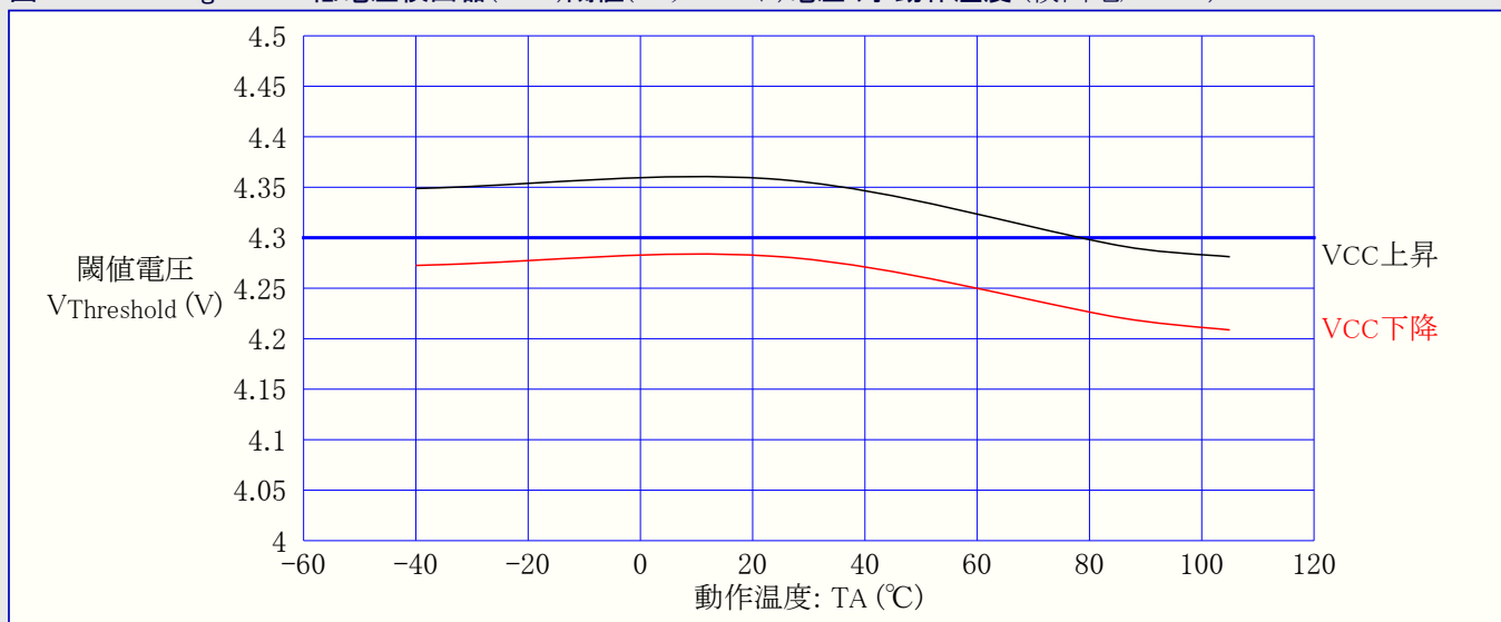
図32-78. ATmega88PA: 低電圧検出器(BOD)閾値(スレッショルド)電圧 対 動作温度 (検出電圧4.3V)
