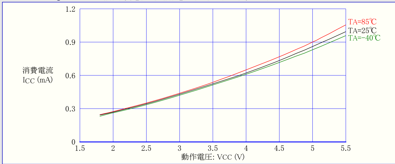
図31-104. ATmega88A: アイドル動作消費電流 対 動作電圧 (内蔵RC発振器, 8MHz)
