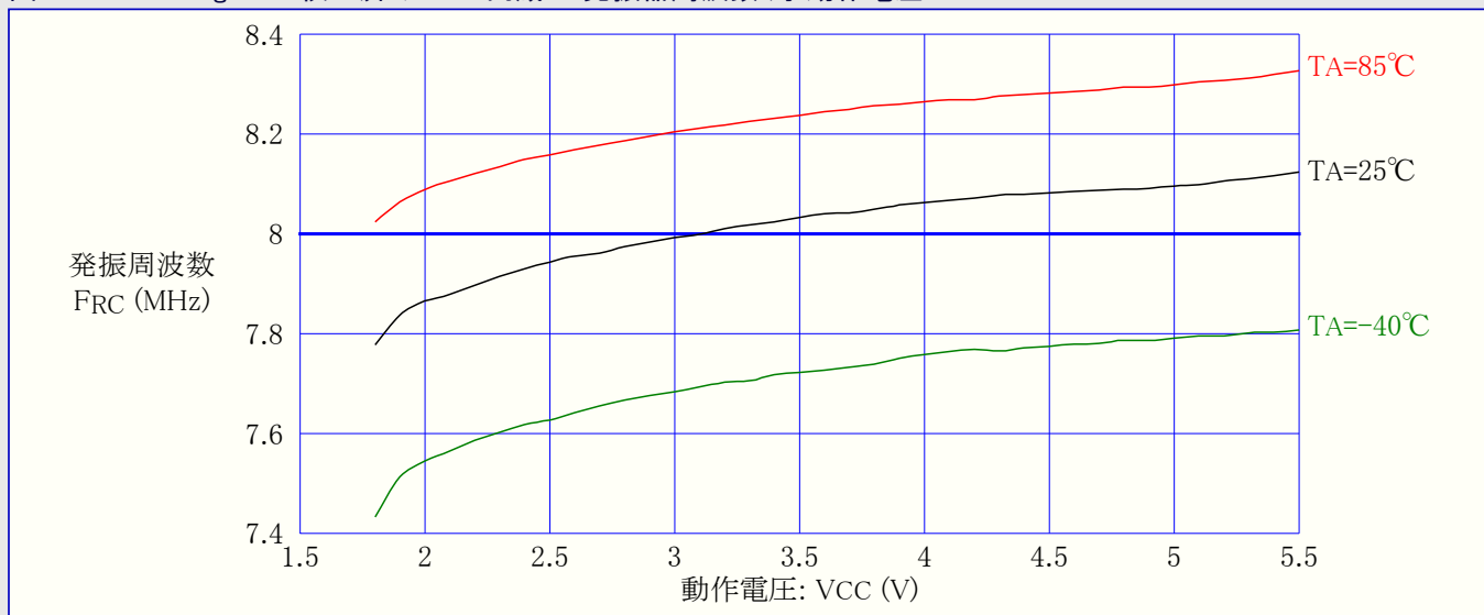
図31-321. ATmega328: 校正済み8MHz内蔵RC発振器周波数 対 動作電圧
