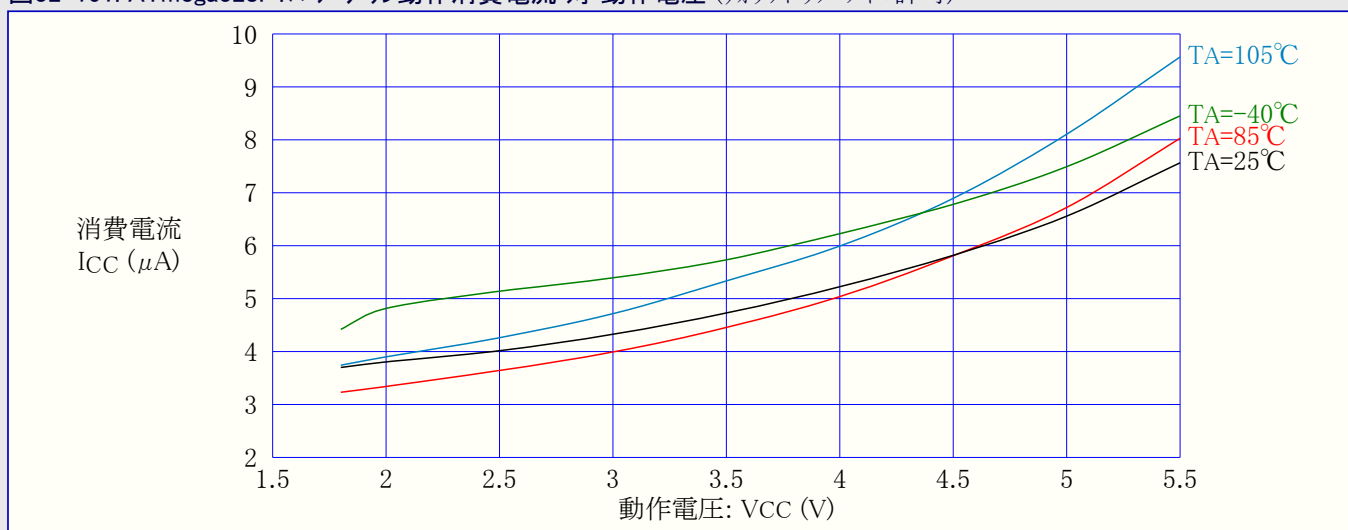
図32-151. ATmega328P:パワーダウン動作消費電流 対 動作電圧 (ウォッチドッグ タイマ許可)
