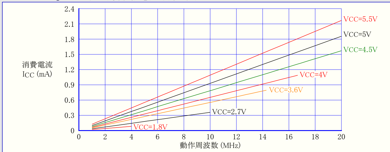
図31-283. ATmega168PA:リセット消費(供給)電流 対 周波数 (1MHz~20MHz)
