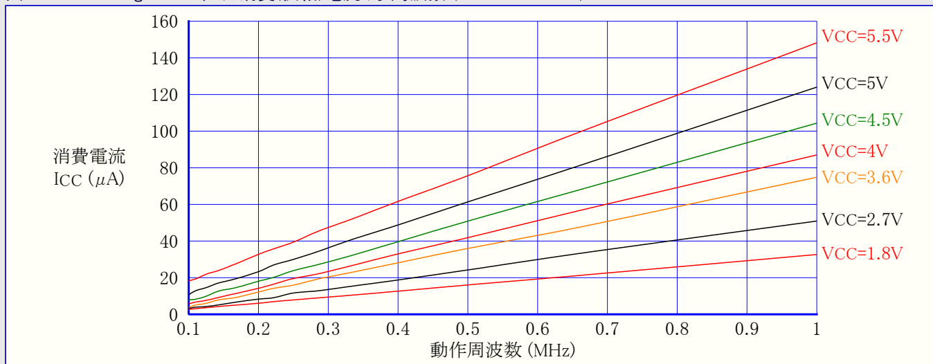
図31-376. ATmega328P:リセット消費(供給)電流 対 周波数 (100kHz~1MHz)
