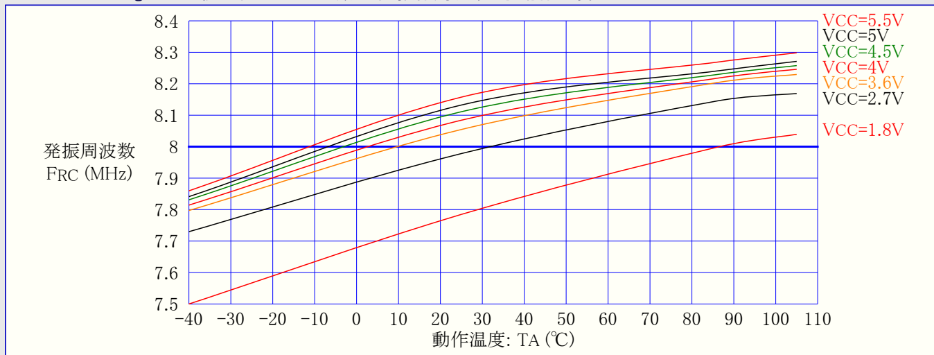
図31-369. ATmega328P: 校正済み8MHz内蔵RC発振器周波数 対 動作温度
