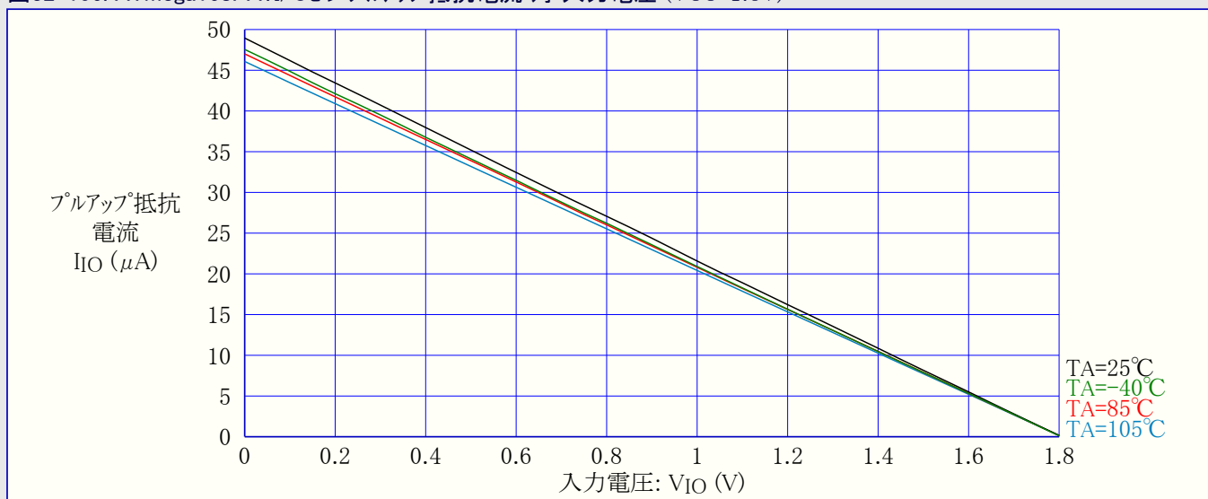
図32-106. ATmega168PA:I/Oピンプルアップ抵抗電流 対 入力電圧 (VCC=1.8V)
