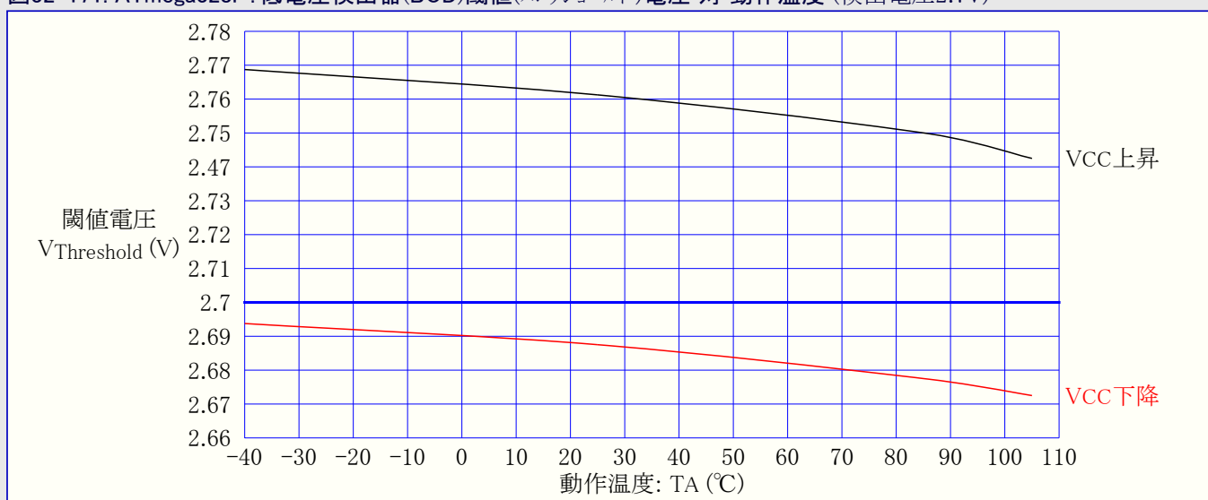
図32-171. ATmega328P: 低電圧検出器(BOD)閾値(スレッシュホールド)電圧 対 動作温度 (検出電圧2.7V)
