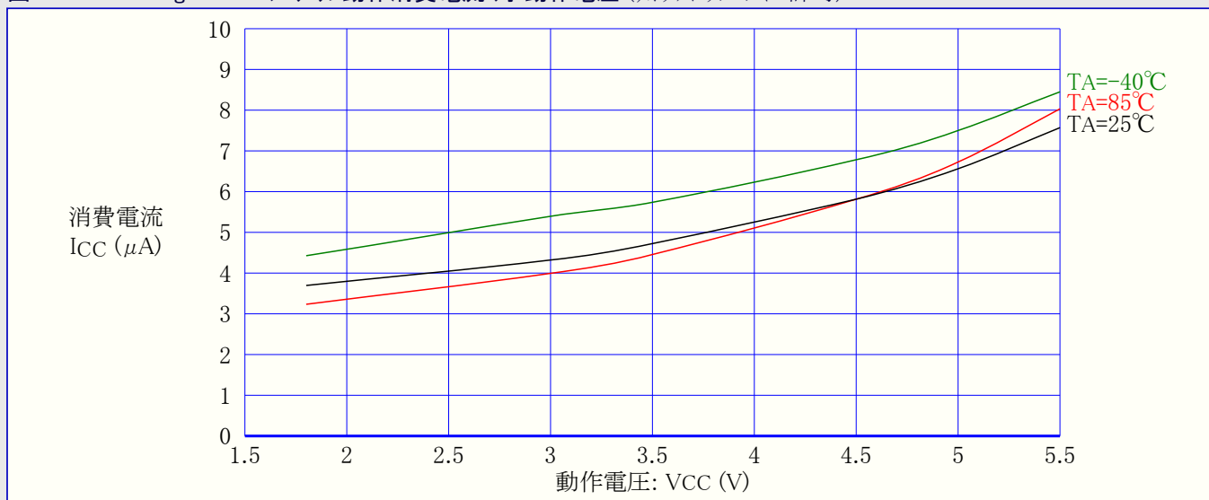
図31-296. ATmega328: パワーダウン動作消費電流 対 動作電圧 (ウォッチドッグ タイマ許可)
