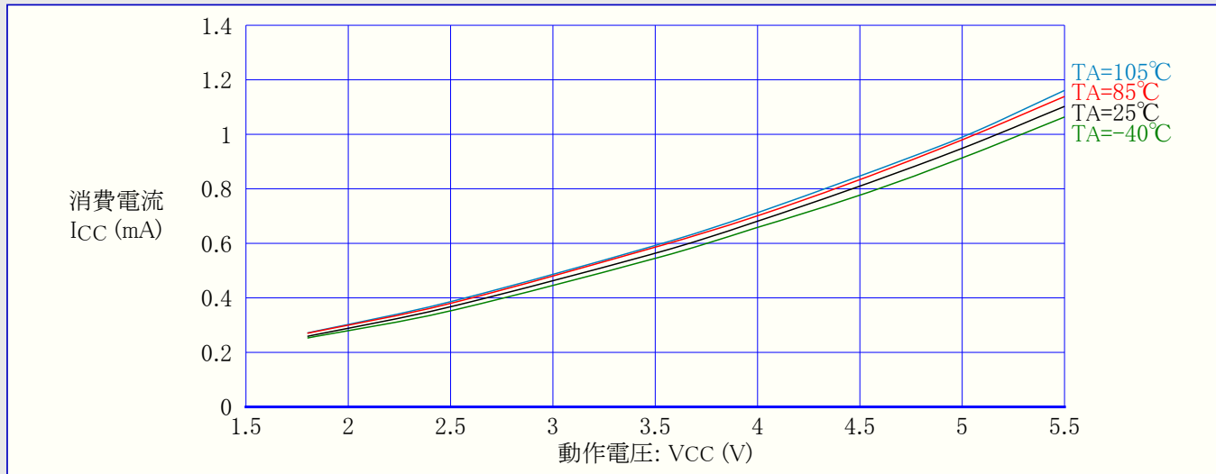
図32-50. ATmega88PA: 活動動作消費電流 対 動作電圧 (内蔵RC発振器, CKDIV8=プログラム(0), 1MHz)
