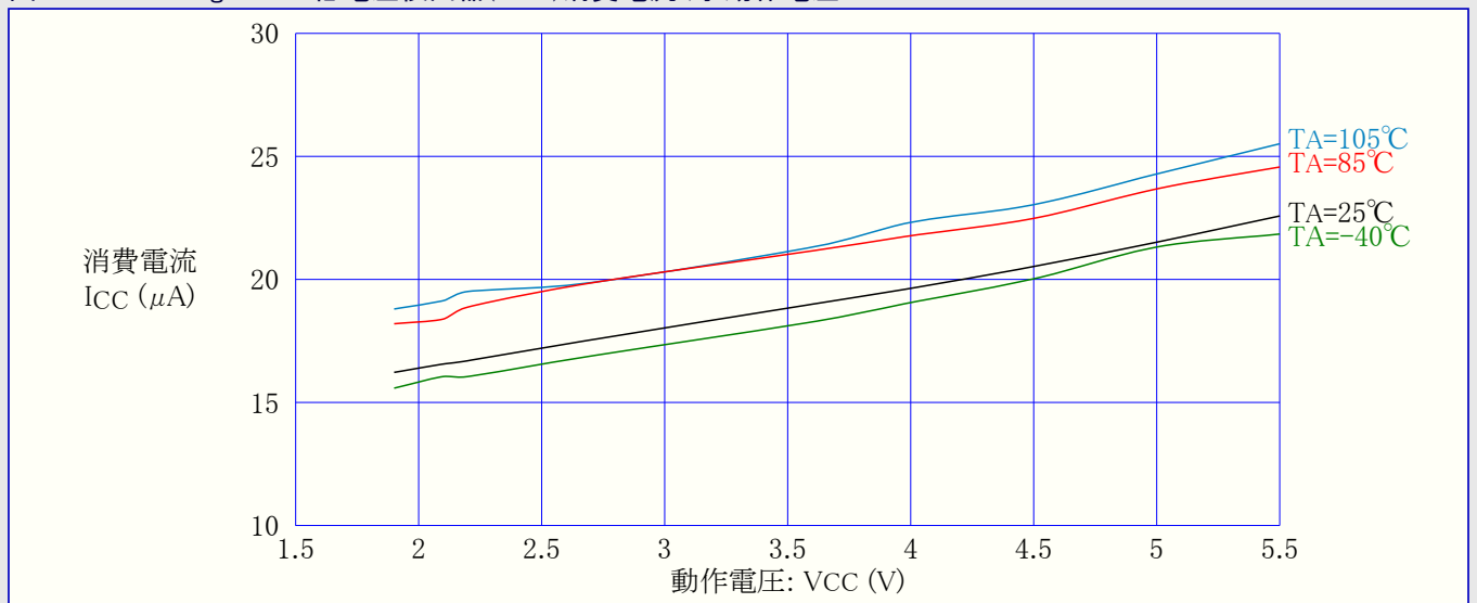
図31-374. ATmega328P: 低電圧検出器(BOD)消費電流 対 動作電圧
