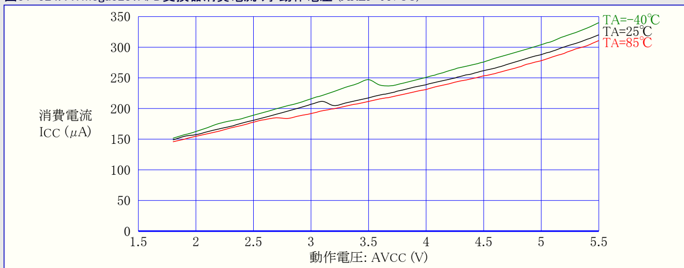
図31-324. ATmega328: A/D変換器消費電流 対 動作電圧 (AREF=AVCC)
