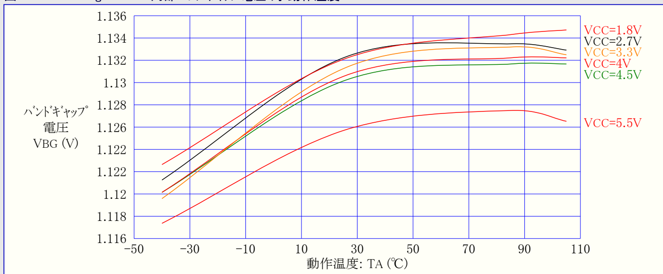
図31-270. ATmega168PA: 内部バンドギャップ電圧 対 動作温度
