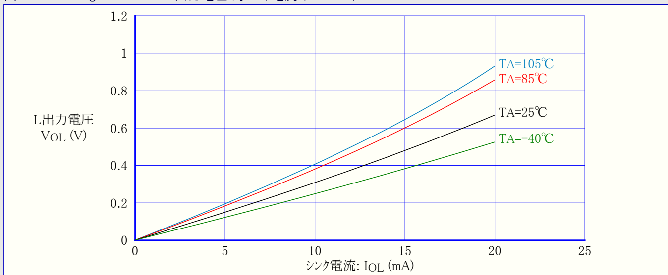
図32-66. ATmega88PA: I/Oピン出力電圧 対 シンク電流 (VCC=3V)
