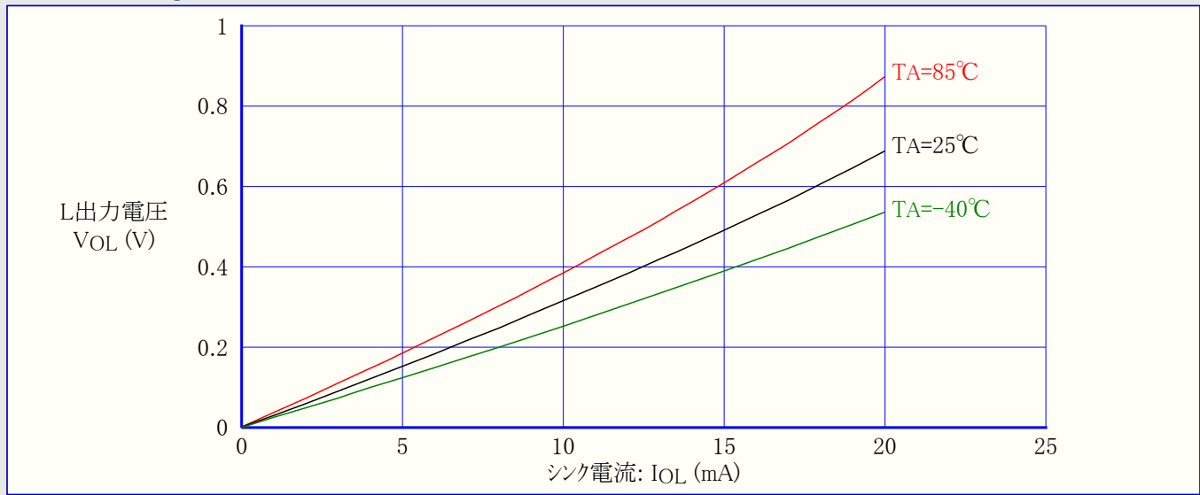
図31-305. ATmega328: I/Oピン出力電圧 対 シンク電流 (VCC=3V)
