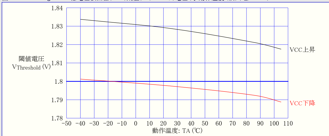
図31-362. ATmega328P: 低電圧検出器(BOD)閾値(スレッシュホールド)電圧 対 動作温度 (検出電圧1.8V)
