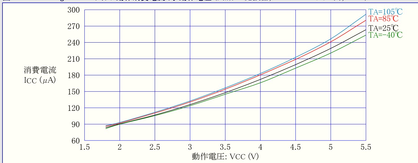
図31-245. ATmega168PA: アイドル動作消費電流 対 動作電圧 (内蔵RC発振器, CKDIV8=プログラム(0), 1MHz)
