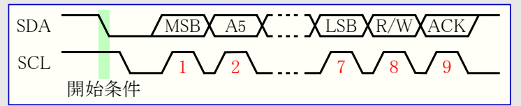
図22-4. アドレス パケット形式
