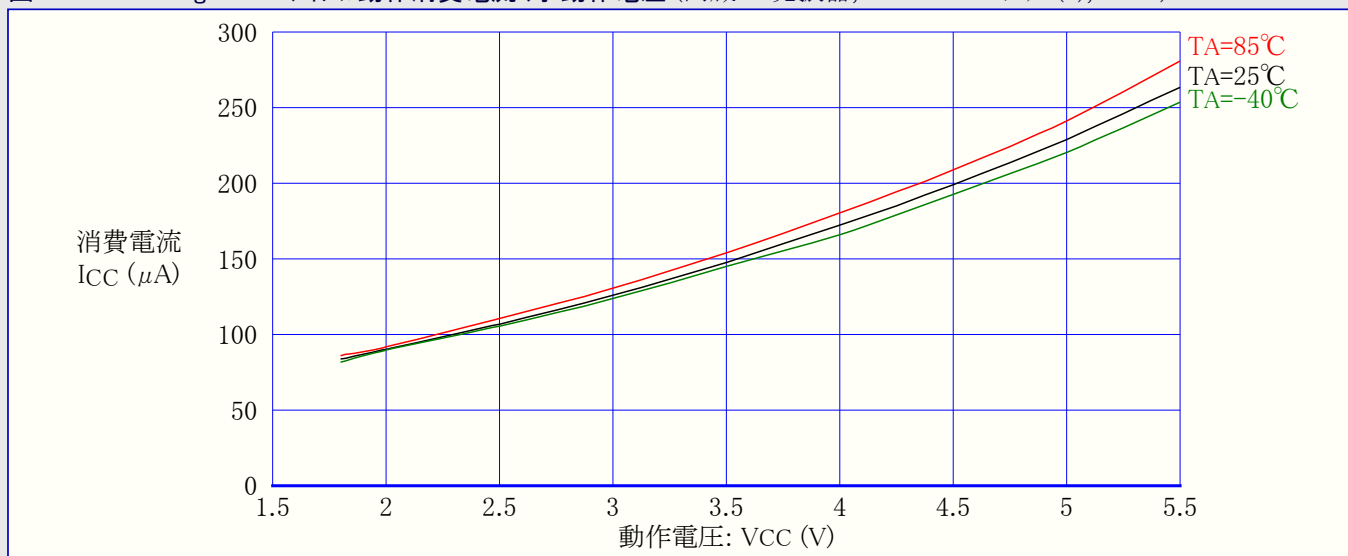
図31-198. ATmega168A: アイドル動作消費電流 対 動作電圧 (内蔵RC発振器, CKDIV8=プログラム(0), 1MHz)
