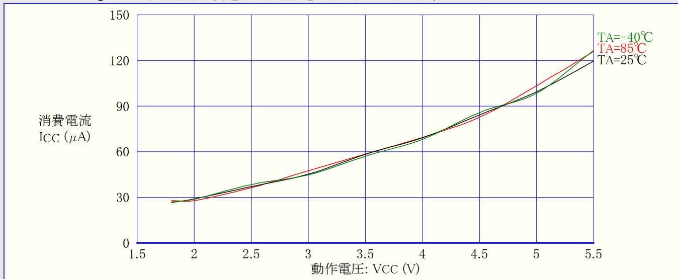
図31-192. ATmega168A: 活動動作消費電流 対 動作電圧 (内蔵WDT発振器, 128kHz)
