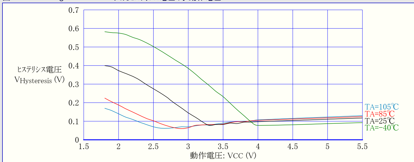
図31-171. ATmega88PA: RESET入力ヒステリシス電圧 対 動作電圧
