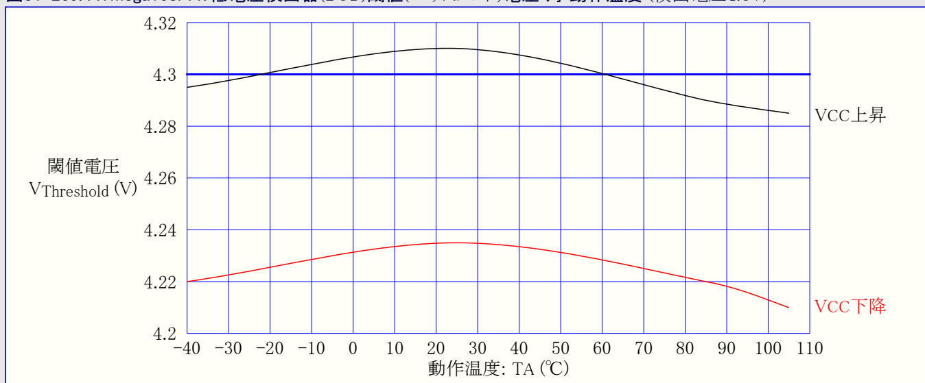
図31-269. ATmega168PA: 低電圧検出器(BOD)閾値(スレッシュホールド)電圧 対 動作温度 (検出電圧4.3V)
