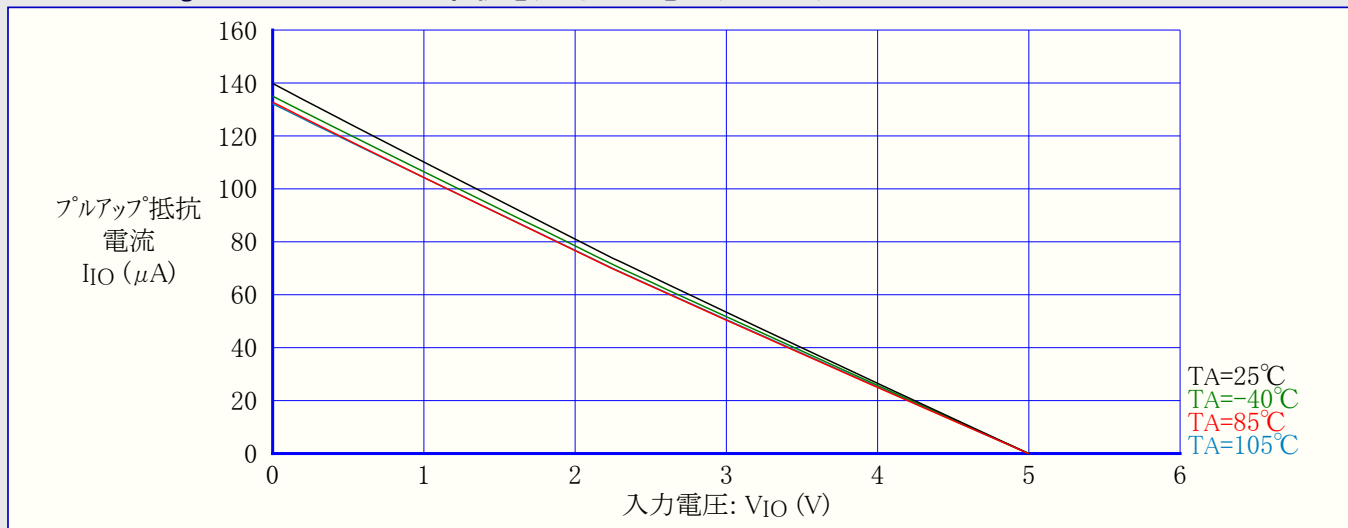
図32-62. ATmega88PA: I/Oピンプルアップ抵抗電流 対 入力電圧 (VCC=5V)
