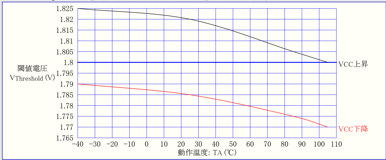
図31-78. ATmega48PA: 低電圧検出器(BOD)閾値(スレッシュホールド)電圧 対 動作温度 (検出電圧1.8V)
