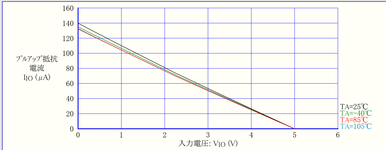
図31-158. ATmega88PA:I/Oピンプルアップ抵抗電流 対 入力電圧 (VCC=5V)
