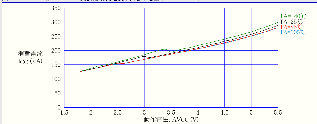
図31-182. ATmega88PA: A/D変換器消費電流 対 動作電圧 (AREF=AVCC)
