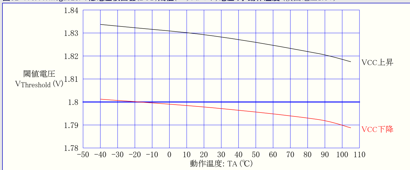
図32-170. ATmega328P: 低電圧検出器(BOD)閾値(スレッシュホールド)電圧 対 動作温度 (検出電圧1.8V)
