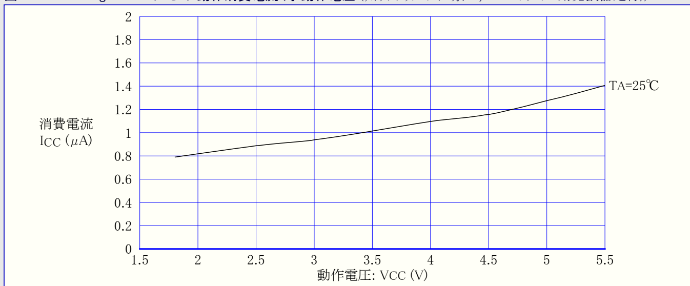
図31-297. ATmega328: パワーセーブ動作消費電流 対 動作電圧 (ウォッチドッグ タイマ禁止, 32kHz クリスタル用発振器走行)
