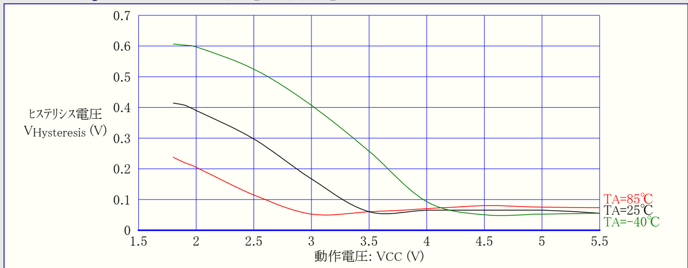
図31-30. ATmega48A: RESET入力ヒステリシス電圧 対 動作電圧
