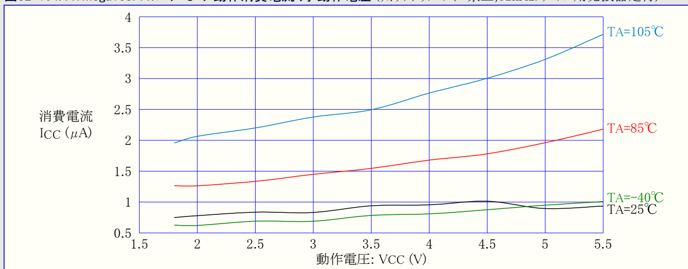
図32-104. ATmega168PA:パワーセーブ動作消費電流 対 動作電圧 (ウォッチドッグ タイマ禁止, 32kHzクリスタル用発振器走行)
