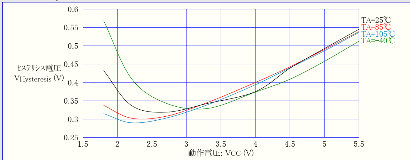
図32-27. ATmega48PA:I/Oピン入力ヒステリシス電圧 対 動作電圧
