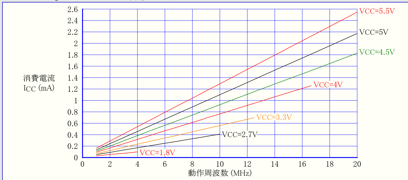
図31-54. ATmega48PA: アイドル動作消費電流 対 周波数 (1MHz~20MHz)
