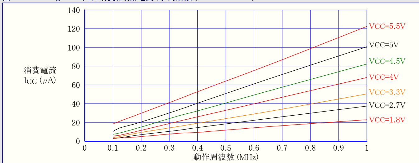
図31-45. ATmega48A:リセット消費(供給)電流 対 周波数 (100kHz~1MHz)
