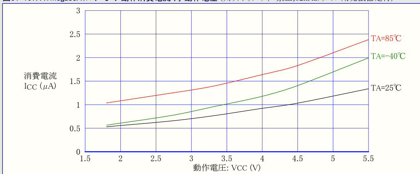
図31-107. ATmega88A: パワーセーブ動作消費電流 対 動作電圧 (ウォッチドッグ タイマ禁止, 32kHzクリスタル用発振器走行)
