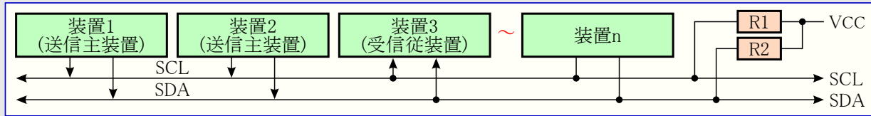
図22-20. バスの競合調停例
