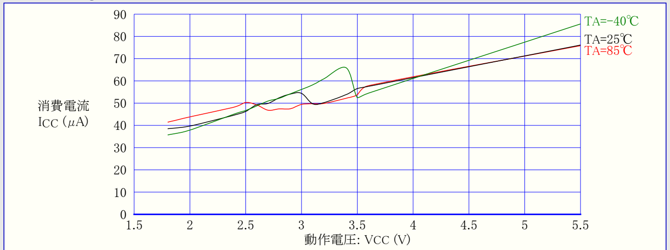
図31-42. ATmega48A: アナログ比較器消費電流 対 動作電圧
