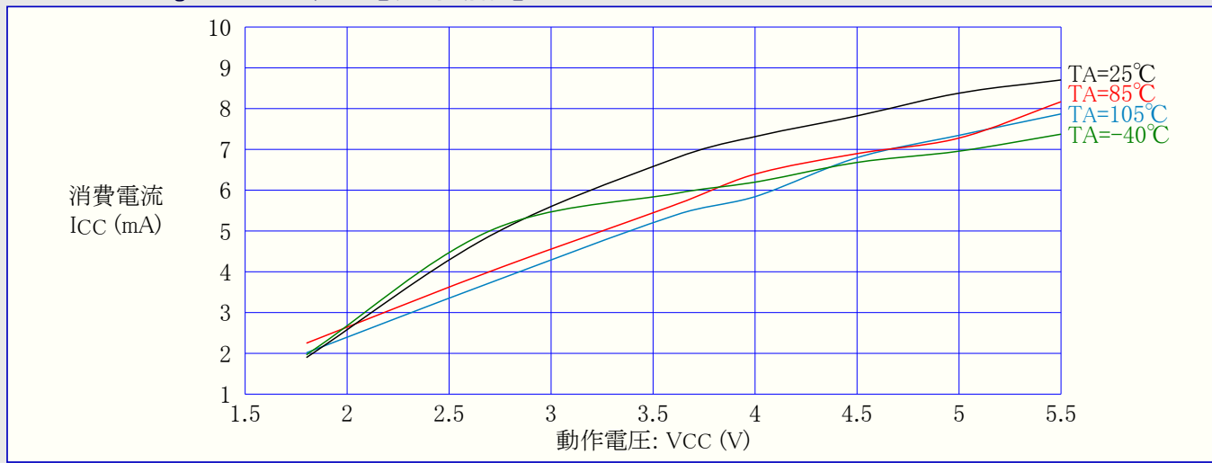
図31-375. ATmega328P:プログラミング電流 対 動作電圧
