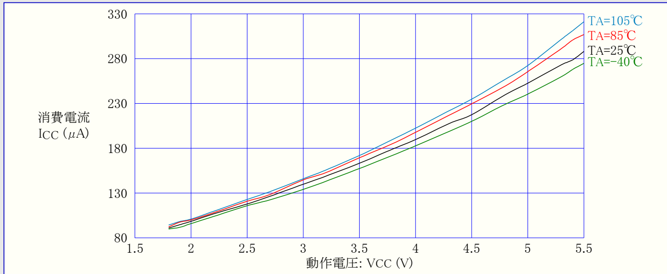
図32-9. ATmega48PA:アイドル動作消費電流 対 動作電圧 (内蔵RC発振器,CKDIV8=プログラム(0),1MHz)
