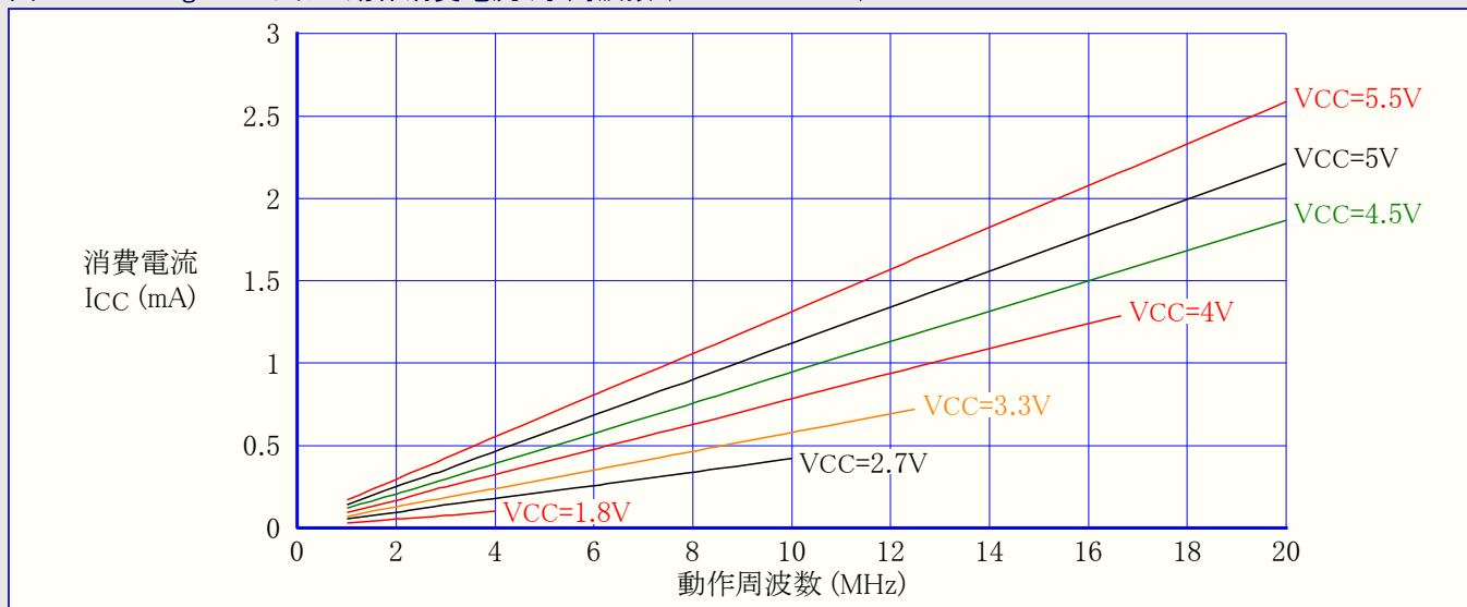
図31-7. ATmega48A: アイドル動作消費電流 対 周波数 (1MHz~20MHz)
