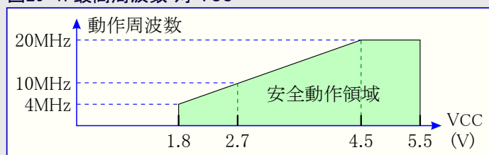
図29-1. 最高周波数 対 VCC
