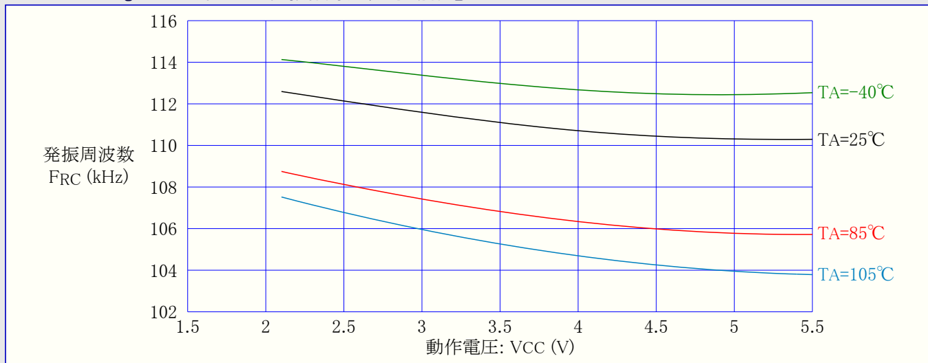
図32-80. ATmega88PA: ウォッチドッグ発振器周波数 対 動作電圧
