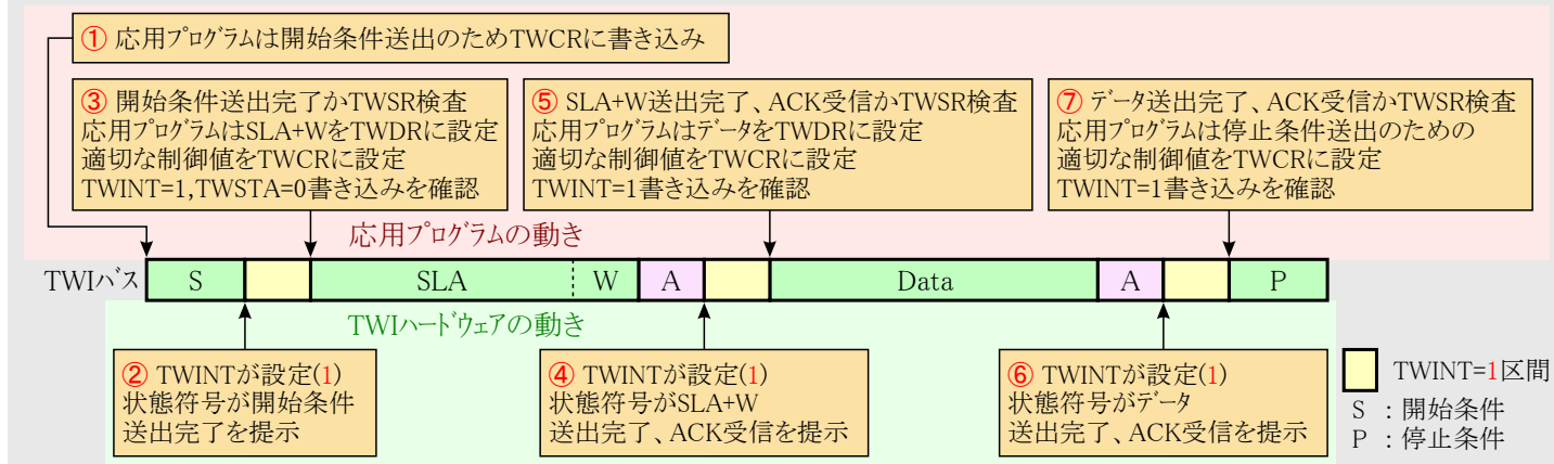
図22-10. 代表的な送信でのアプリケーションプログラムとTWIのインターフェース
