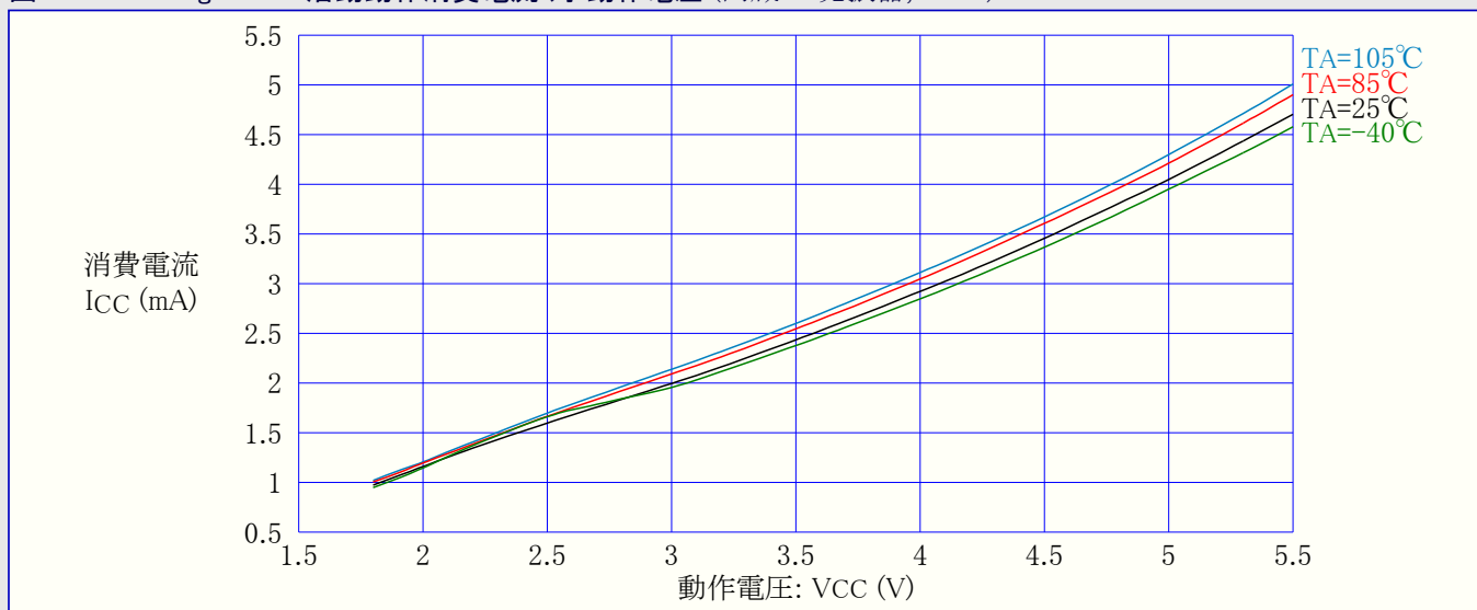
図31-52. ATmega48PA: 活動動作消費電流 対 動作電圧 (内蔵RC発振器, 8MHz)
