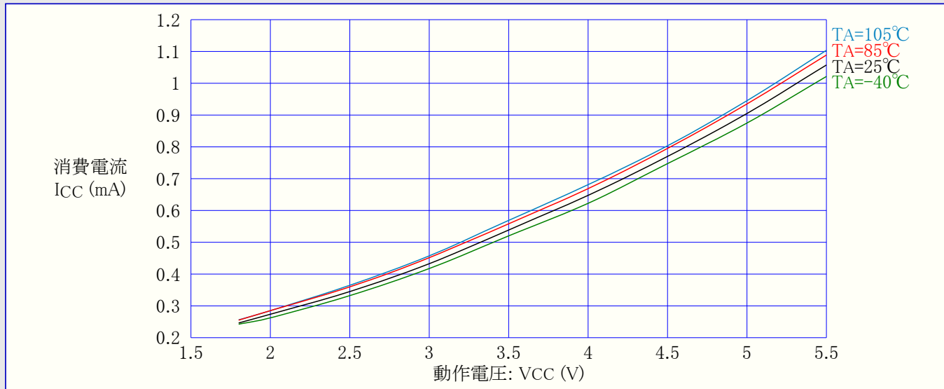
図32-95. ATmega168PA: 活動動作消費電流 対 動作電圧 (内蔵RC発振器, CKDIV8=プログラム(0), 1MHz)
