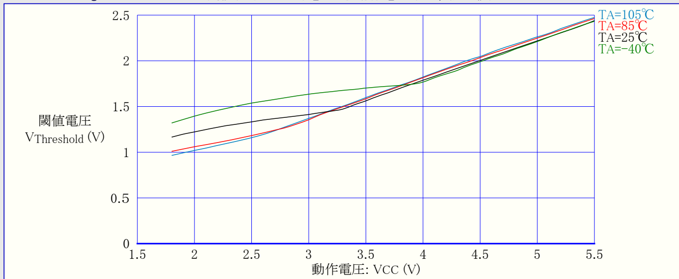
図32-73. ATmega88PA:RESET入力閾値(スレッショルド)電圧 対 動作電圧 (VIH,1読み値)
