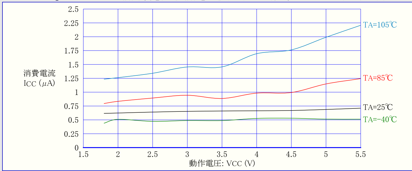
図32-13. ATmega48PA:パワーセーブ動作消費電流 対 動作電圧 (ウォッチドッグ タイマ禁止, 32kHzクリスタル用発振器走行)
