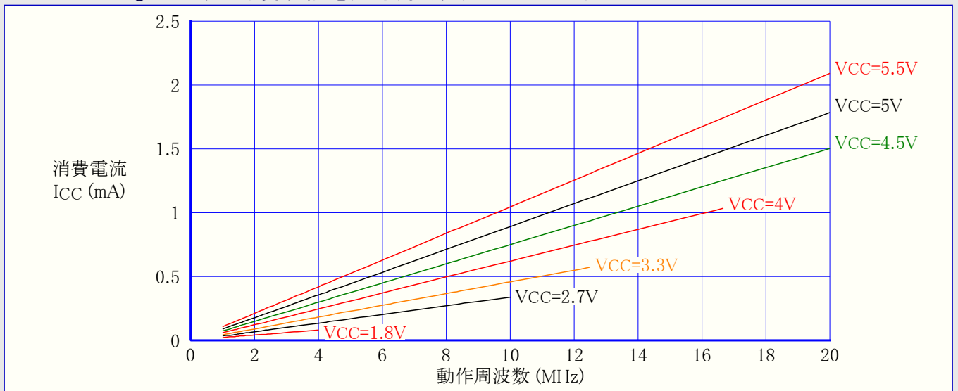
図31-235. ATmega168A:リセット消費(供給)電流 対 周波数 (1MHz~20MHz)
