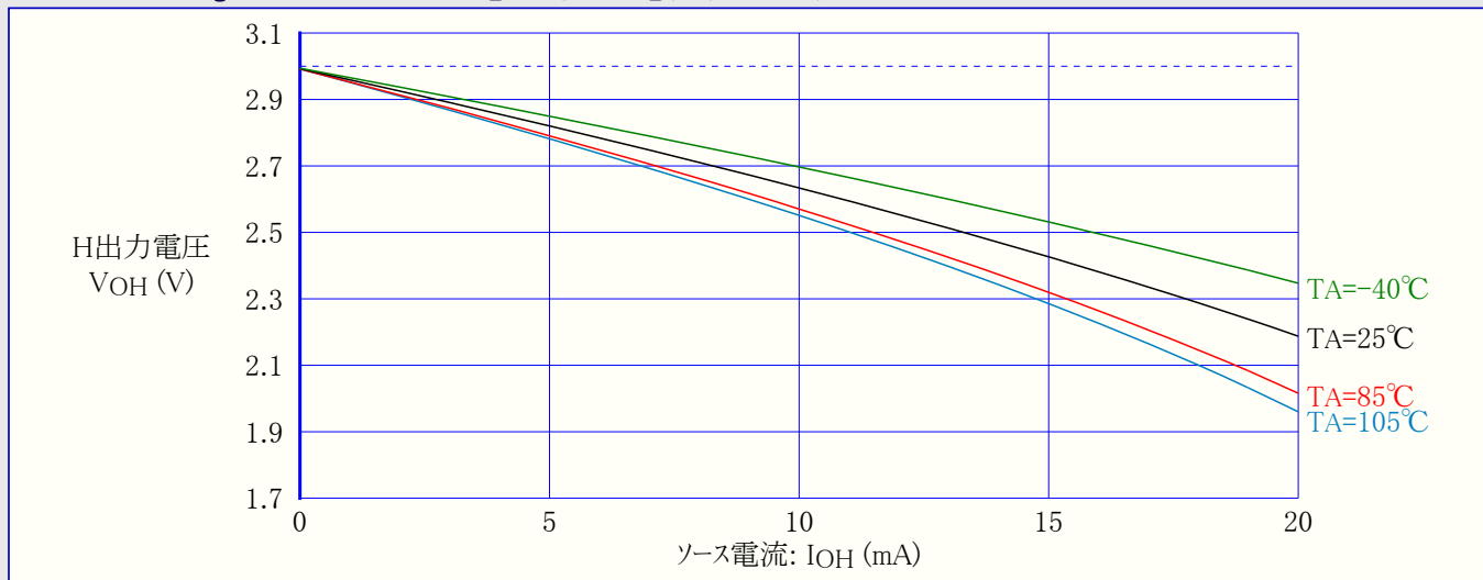
図31-259. ATmega168PA:I/Oピン出力電圧 対 ソース電流 (VCC=3V)
