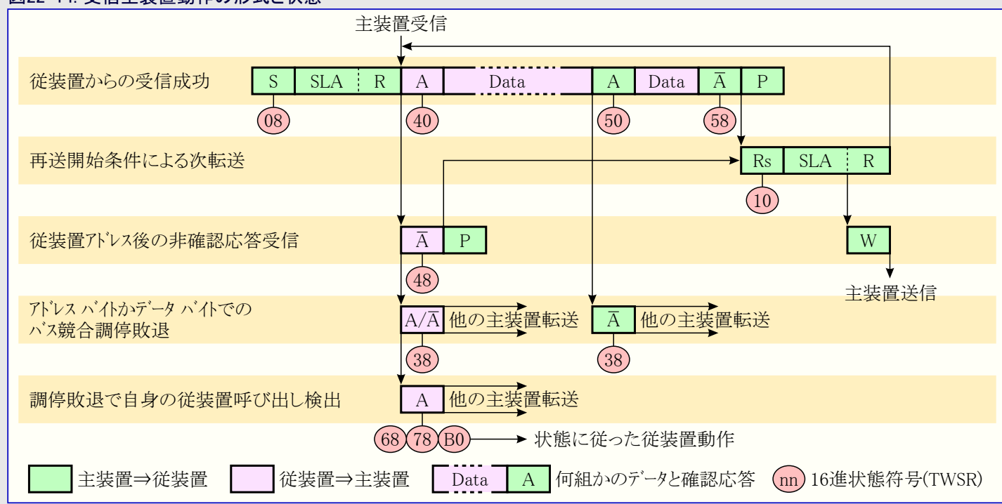
図22-14. 受信主装置動作の形式と状態
