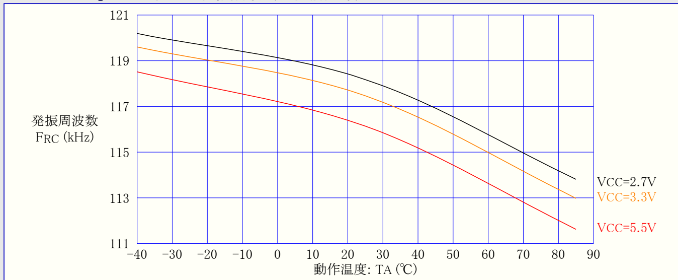
図31-224. ATmega168A: ウォッチドッグ発振器周波数 対 動作温度
