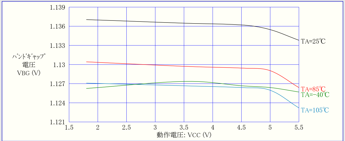
図32-173. ATmega328P: 内部バンドギャップ電圧 対 動作電圧
