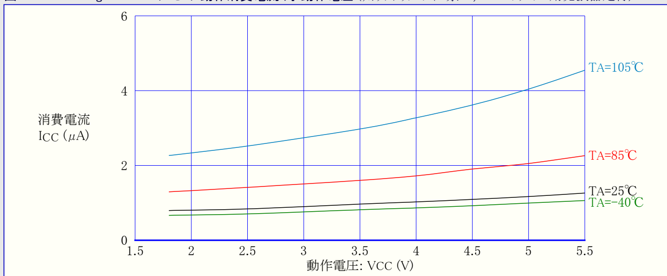
図31-154. ATmega88PA: パワーセーブ動作消費電流 対 動作電圧 (ウォッチドッグ タイマ禁止, 32kHzクリスタル用発振器走行)
