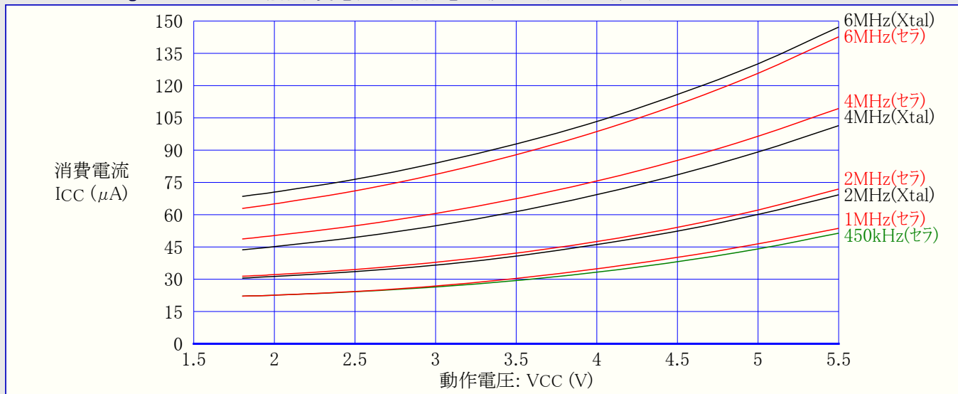
図32-14. ATmega48PA:スタンバイ動作消費電流 対 動作電圧 (ウォッチドッグ タイマ禁止)
