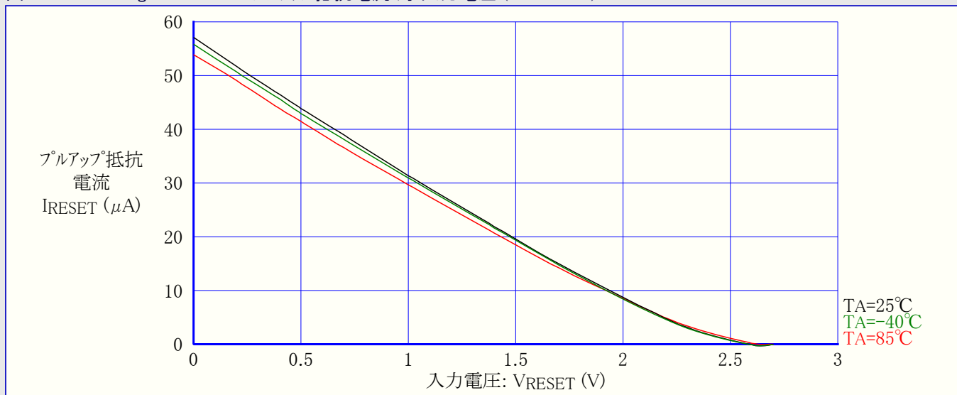
図31-113. ATmega88A:RESETプルアップ抵抗電流 対 入力電圧 (VCC=2.7V)
