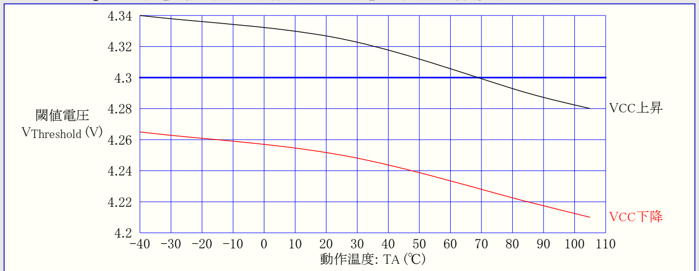
図31-80. ATmega48PA: 低電圧検出器(BOD)閾値(スレッショルド)電圧 対 動作温度 (検出電圧4.3V)
