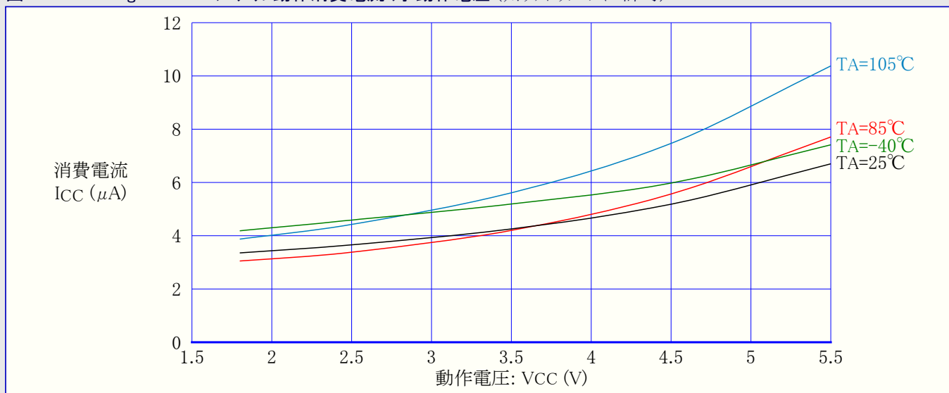
図32-58. ATmega88PA:パワーダウン動作消費電流 対 動作電圧 (ウォッチドッグ タイマ許可)
