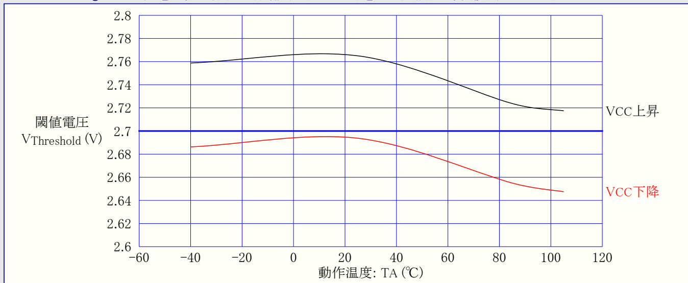
図32-77. ATmega88PA: 低電圧検出器(BOD)閾値(スレッショルド)電圧 対 動作温度 (検出電圧2.7V)
