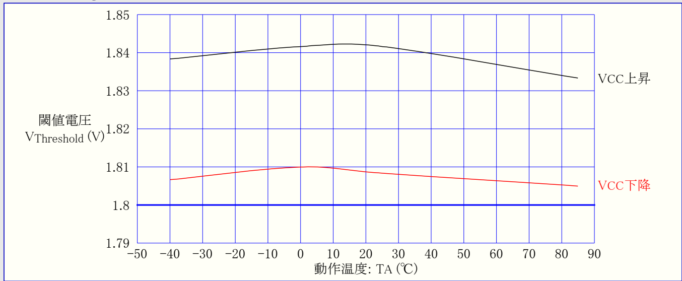
図31-31. ATmega48A: 低電圧検出器(BOD)閾値(スレッショルド)電圧 対 動作温度 (検出電圧1.8V)
