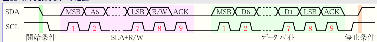
図22-6. 代表的なデータ転送
