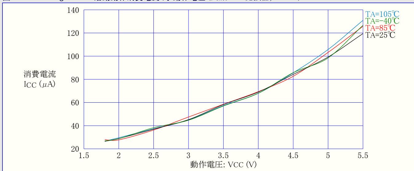
図31-239. ATmega168PA: 活動動作消費電流 対 動作電圧 (内蔵WDT発振器, 128kHz)
