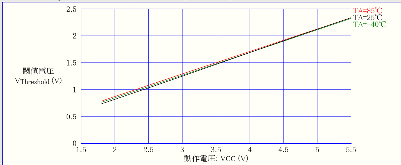
図31-123. ATmega88A: RESET入力閾値(スレッショルド)電圧 対 動作電圧 (VIL,0読み値)
