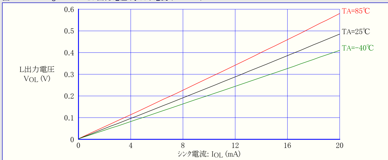
図31-22. ATmega48A: I/Oピン出力電圧 対 シンク電流 (VCC=5V)
