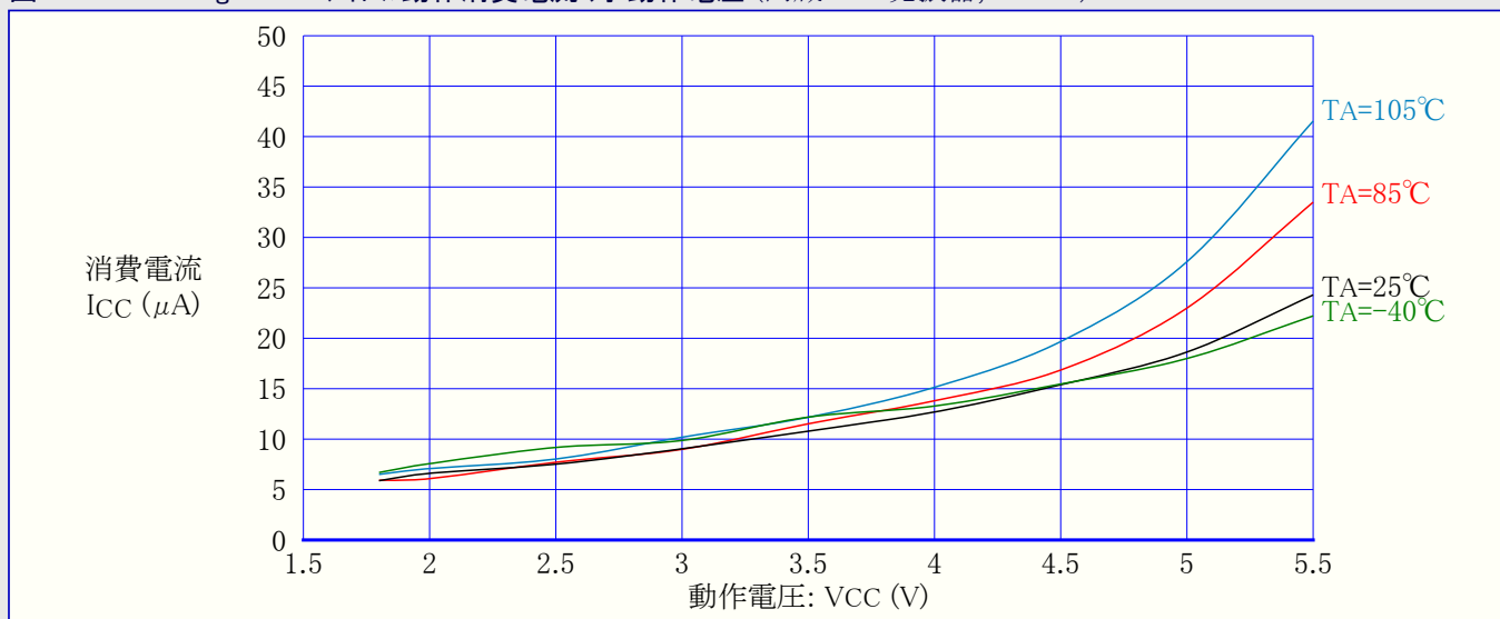
図31-149. ATmega88PA: アイドル動作消費電流 対 動作電圧 (内蔵WDT発振器, 128kHz)
