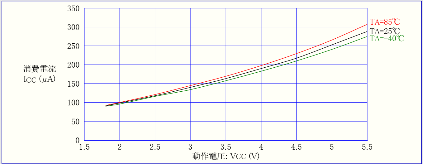
図31-9. ATmega48A: アイドル動作消費電流 対 動作電圧 (内蔵RC発振器, CKDIV8=プログラム(0), 1MHz)
