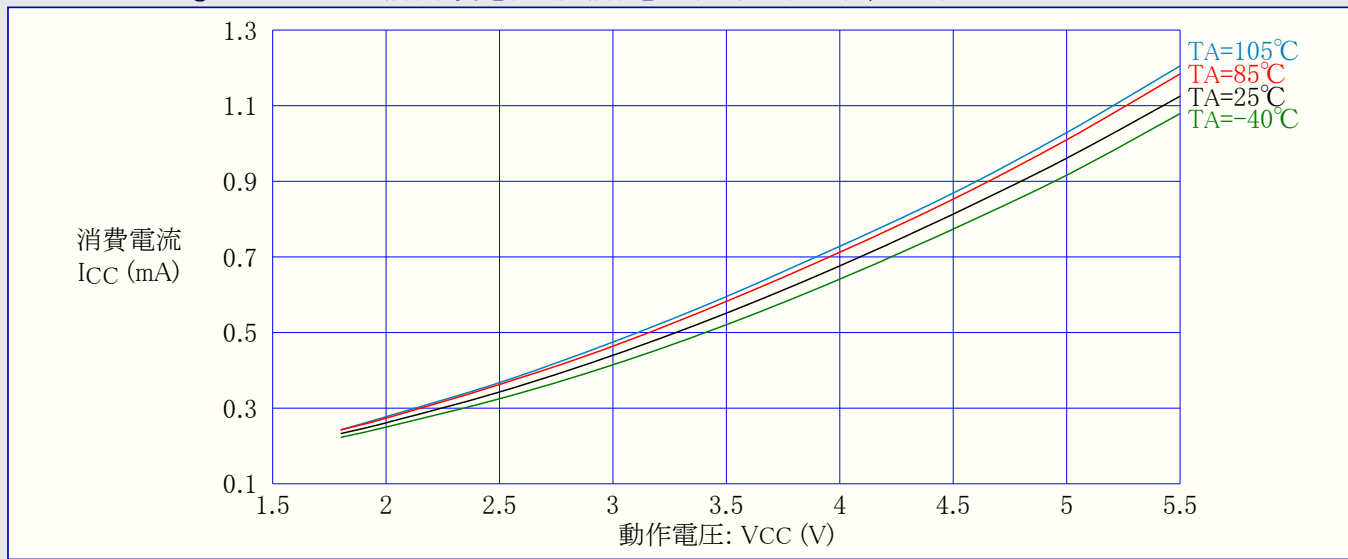
図31-246. ATmega168PA: アイドル動作消費電流 対 動作電圧 (内蔵RC発振器, 8MHz)
