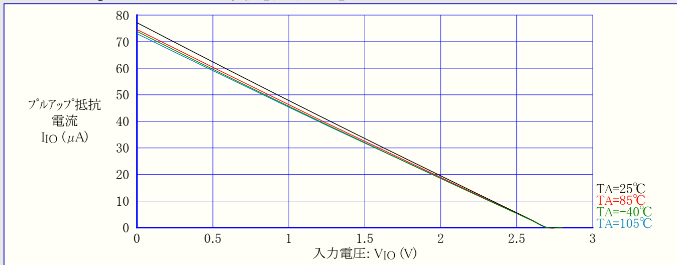
図32-155. ATmega328P:I/Oピンプルアップ抵抗電流 対 入力電圧 (VCC=2.7V)
