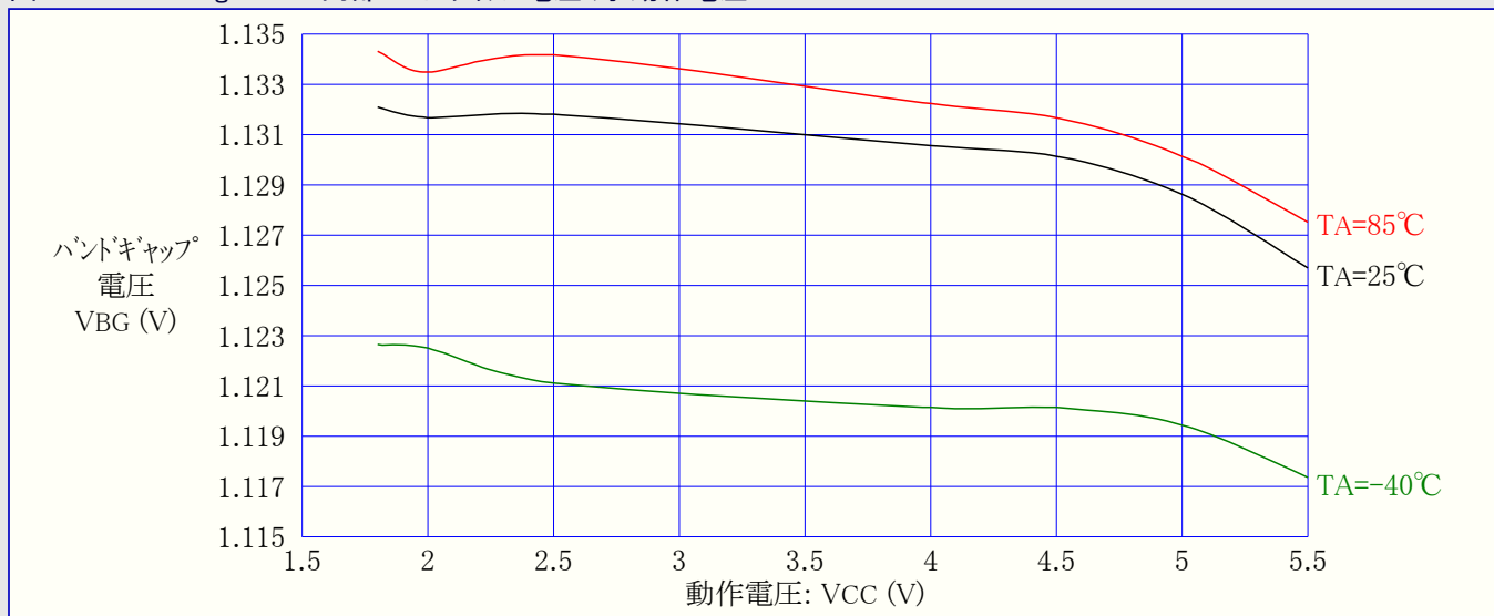
図31-223. ATmega168A: 内部バンドギャップ電圧 対 動作電圧
