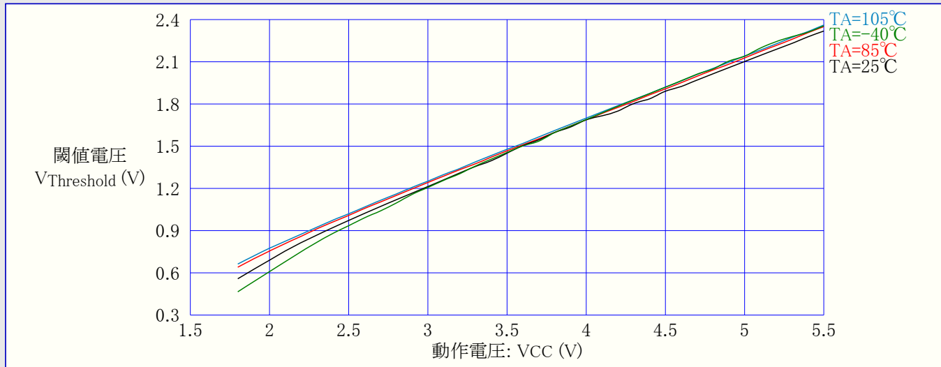
図31-73. ATmega48PA:I/Oピン入力閾値(スレッショルド)電圧 対 動作電圧 (VIL,0読み値)
