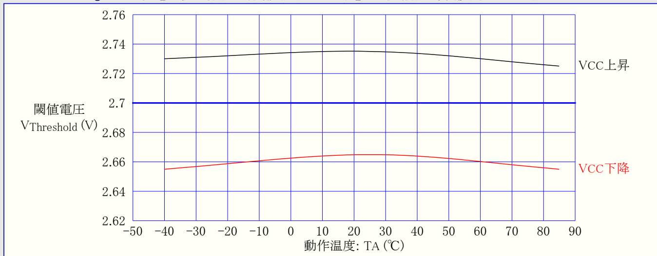
図31-221. ATmega168A: 低電圧検出器(BOD)閾値(スレッシュホールド)電圧 対 動作温度 (検出電圧2.7V)
