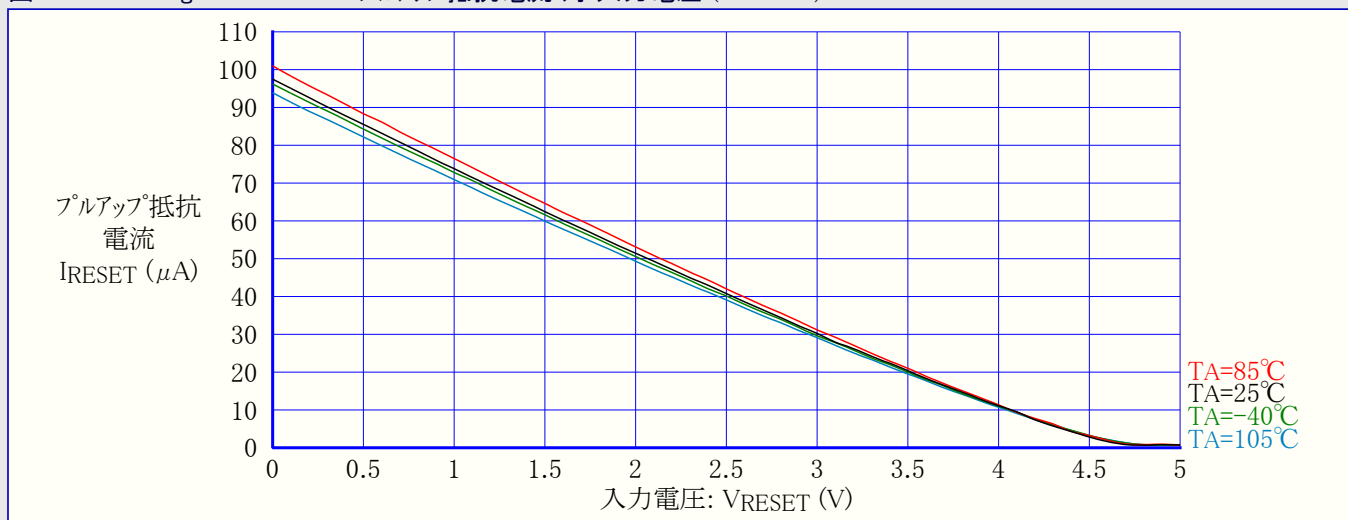
図32-20. ATmega48PA: RESETプルアップ抵抗電流 対 入力電圧 (VCC=5V)
