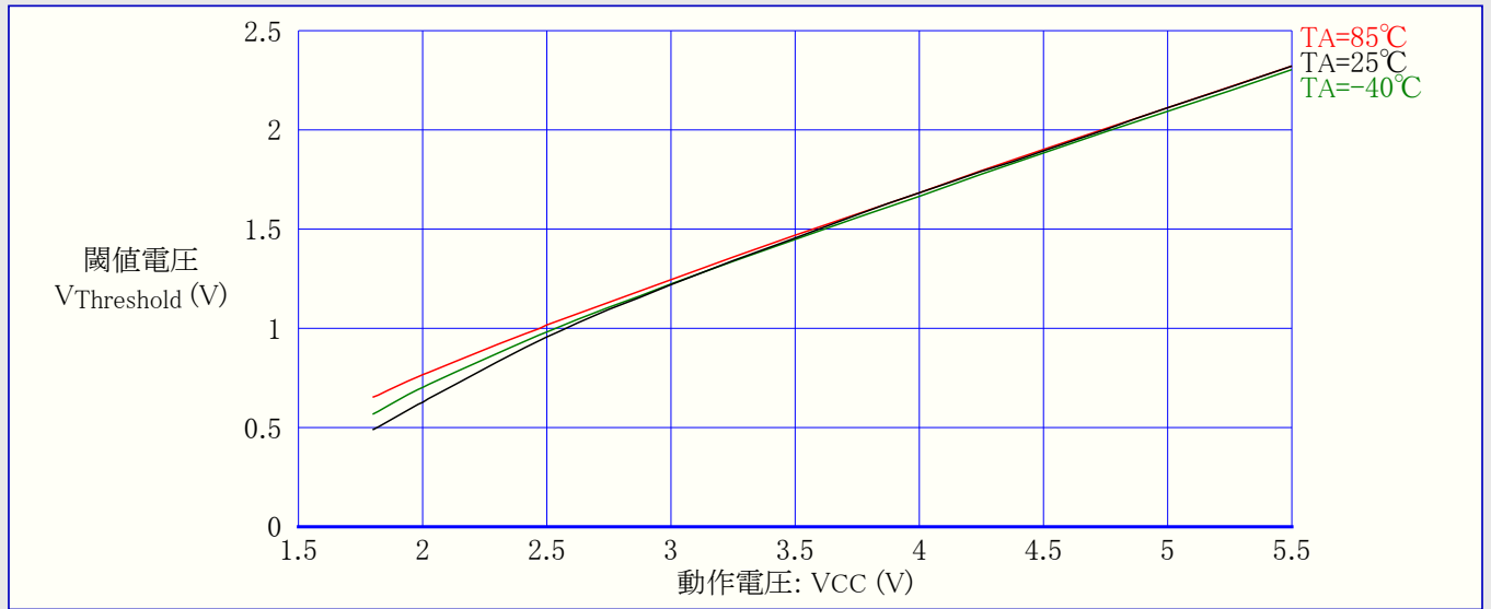
図31-215. ATmega168A:I/Oピン入力閾値(スレッショルド)電圧 対 動作電圧 (VIL,0読み値)
