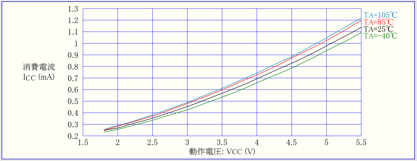
図31-57. ATmega48PA:アイドル動作消費電流 対 動作電圧 (内蔵RC発振器,8MHz)
