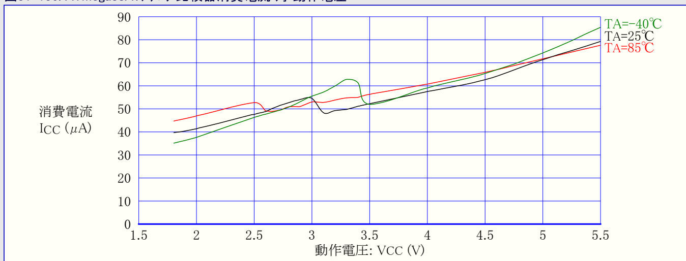
図31-136. ATmega88A: アナログ比較器消費電流 対 動作電圧
