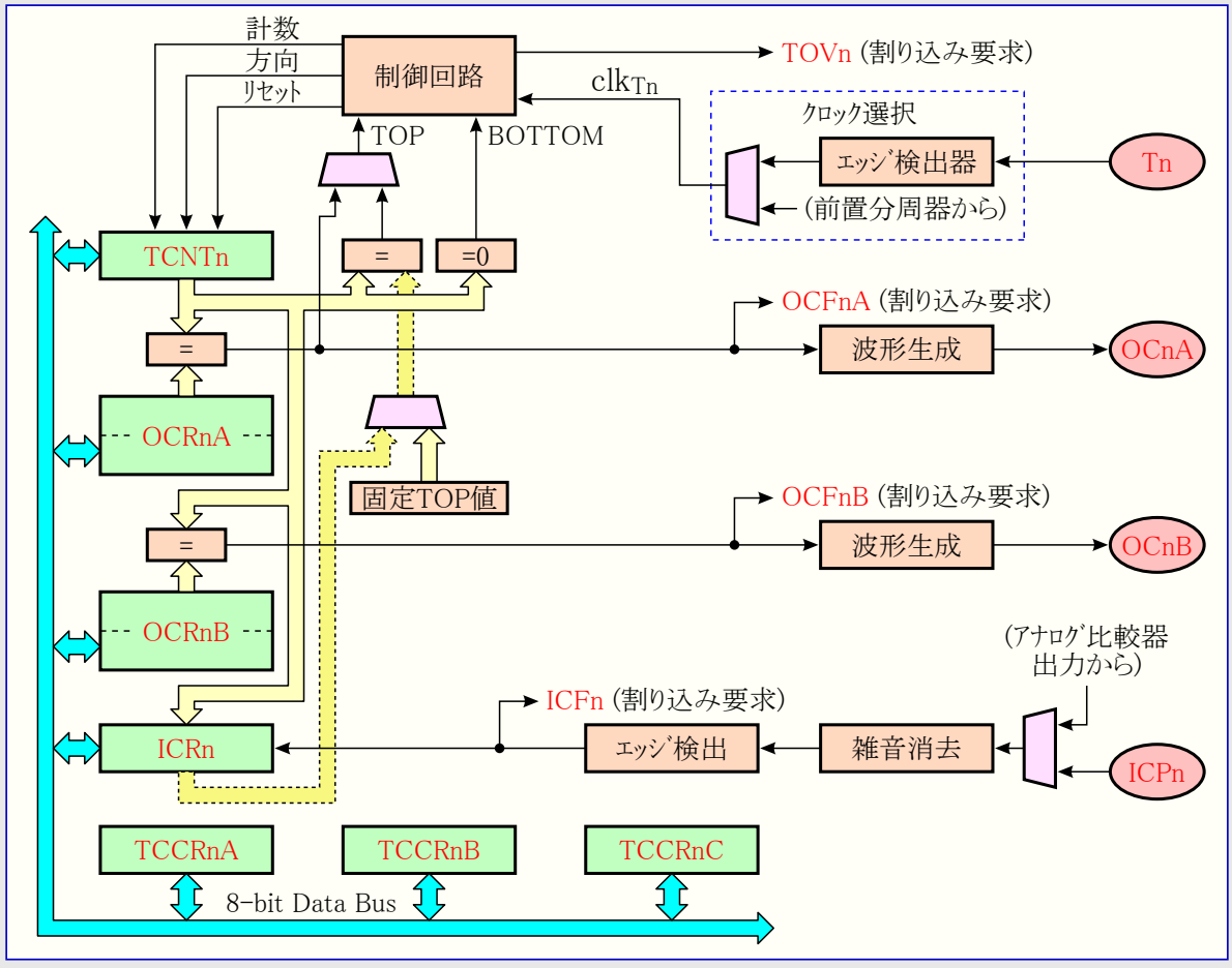
図16-1. 16ビット タイマ/カウンタ構成図
