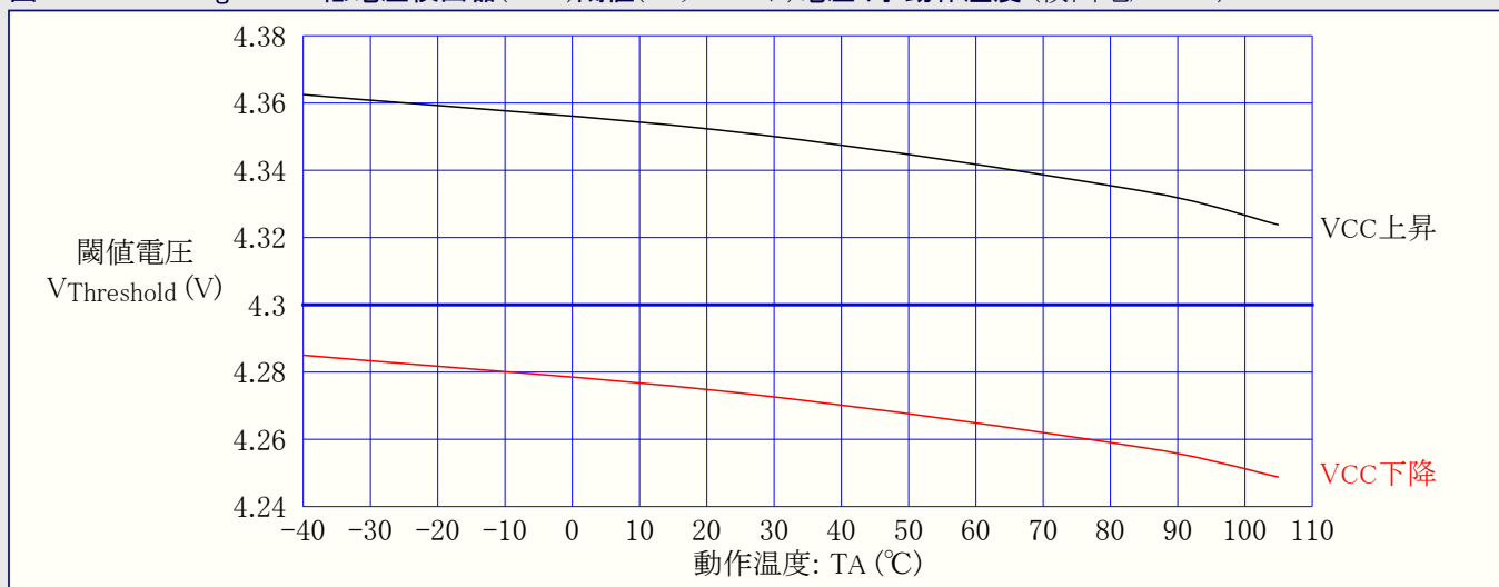
図31-364. ATmega328P: 低電圧検出器(BOD)閾値(スレッシュホールド)電圧 対 動作温度 (検出電圧4.3V)
