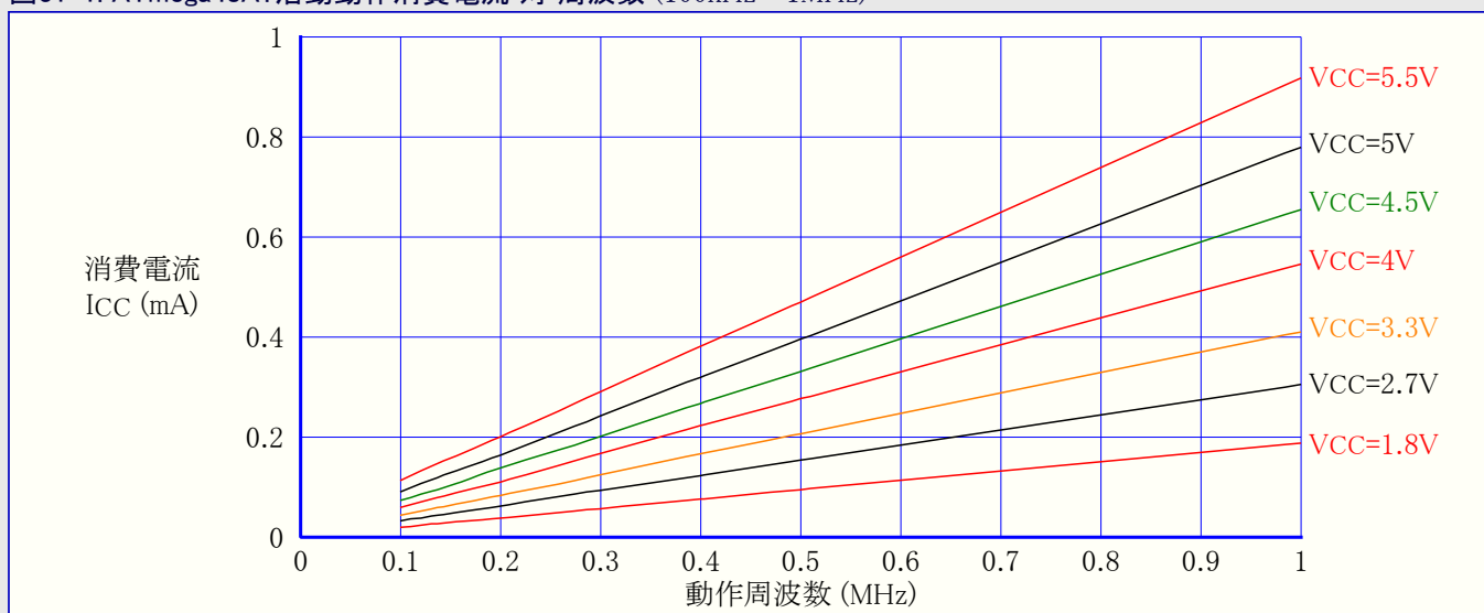
図31-1. ATmega48A: 活動動作消費電流 対 周波数 (100kHz~1MHz)
