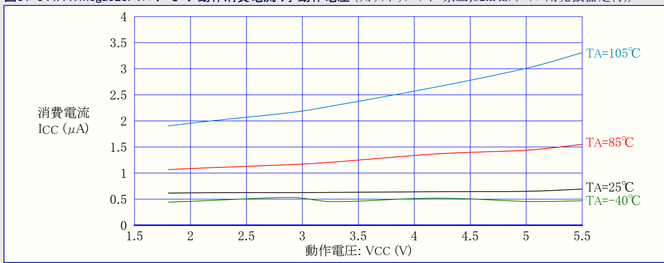
図31-344. ATmega328P: パワーセーブ動作消費電流 対 動作電圧 (ウォッチドッグ タイマ禁止, 32kHzクリスタル用発振器走行))
