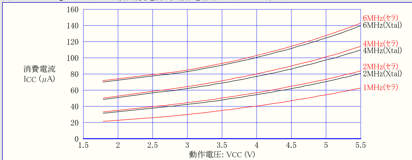
図32-153. ATmega328P: スタンバイ動作消費電流 対 動作電圧 (ウォッチドッグ タイマ禁止)
