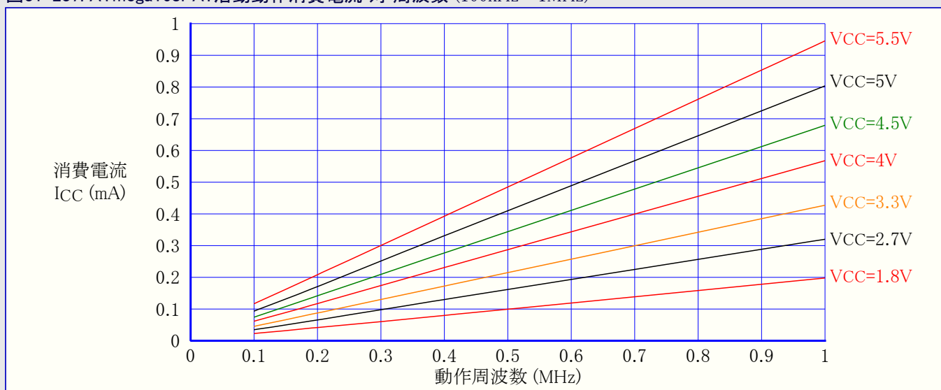
図31-237. ATmega168PA: 活動動作消費電流 対 周波数 (100kHz~1MHz)
