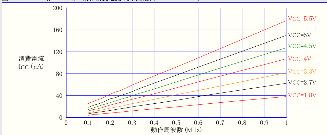
図31-290. ATmega328: アイドル動作消費電流 対 周波数 (100kHz~1MHz)
