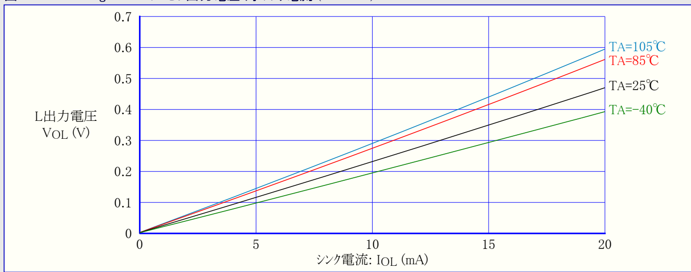
図31-353. ATmega328P: I/Oピン出力電圧 対 シンク電流 (VCC=5V)
