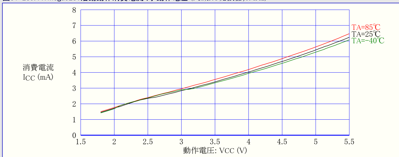
図31-289. ATmega328: 活動動作消費電流 対 動作電圧 (内蔵RC発振器, 8MHz)
