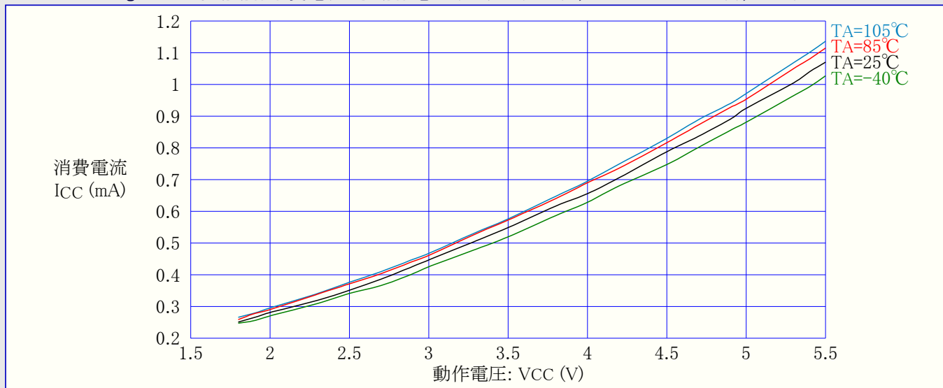
図31-51. ATmega48PA: 活動動作消費電流 対 動作電圧 (内蔵RC発振器, CKDIV8=プログラム(0), 1MHz)
