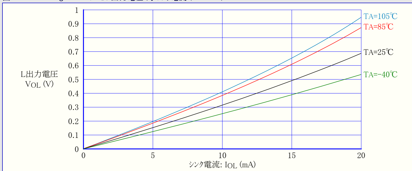
図32-160. ATmega328P: I/Oピン出力電圧 対 シンク電流 (VCC=3V)
