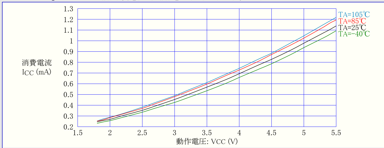
図32-10. ATmega48PA:アイドル動作消費電流 対 動作電圧 (内蔵RC発振器,8MHz)
