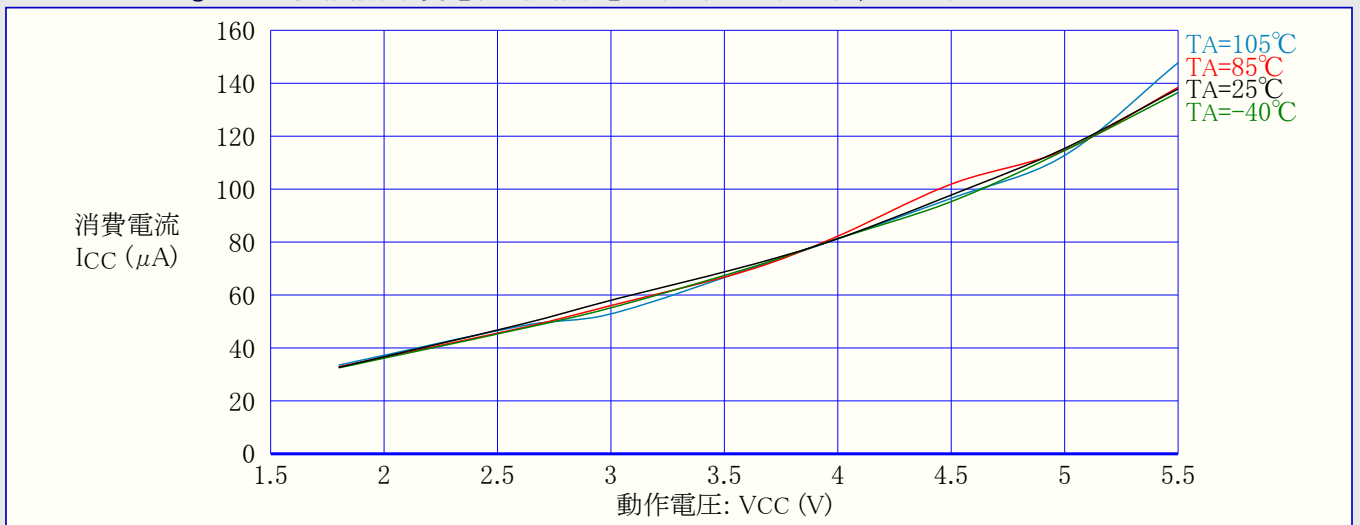
図32-142. ATmega328P: 活動動作消費電流 対 動作電圧 (内蔵WDT発振器, 128kHz)
