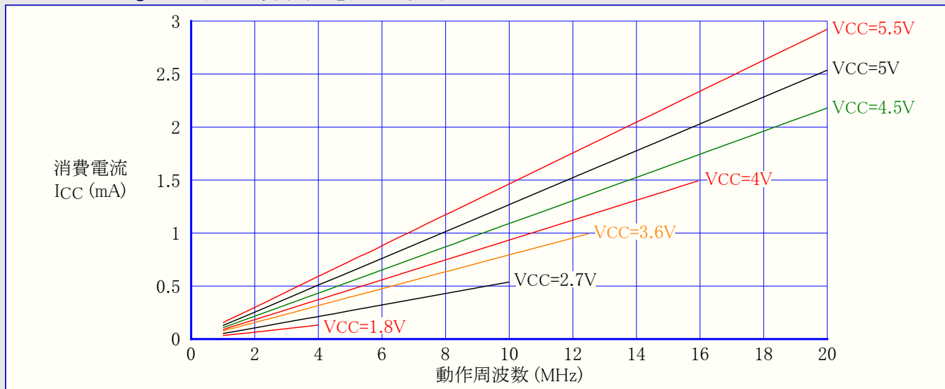
図32-185. ATmega328P:リセット消費(供給)電流 対 周波数 (1MHz~20MHz)
