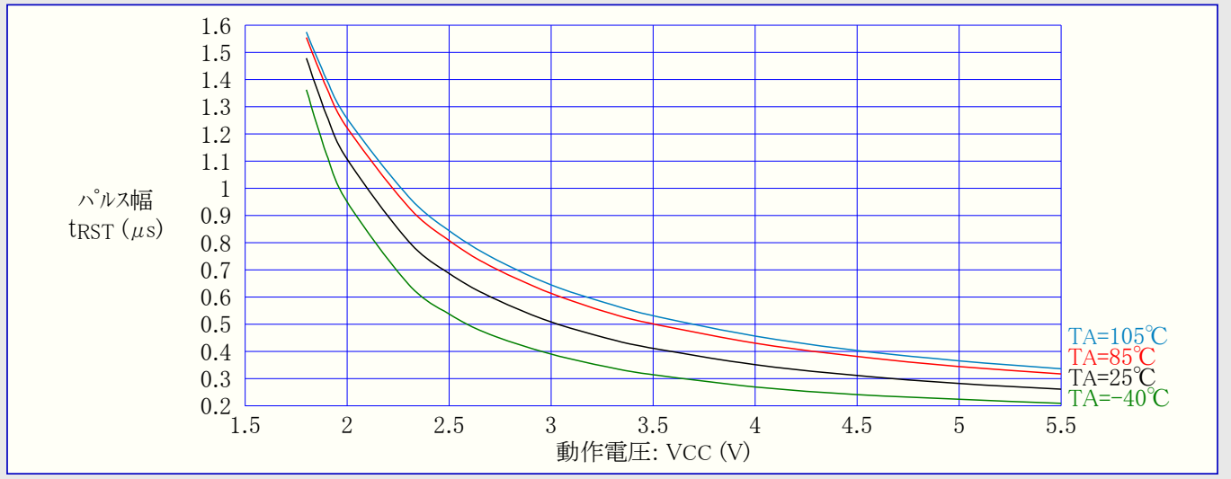
図31-94. ATmega48PA: 最小リセットパルス幅 対 動作電圧
