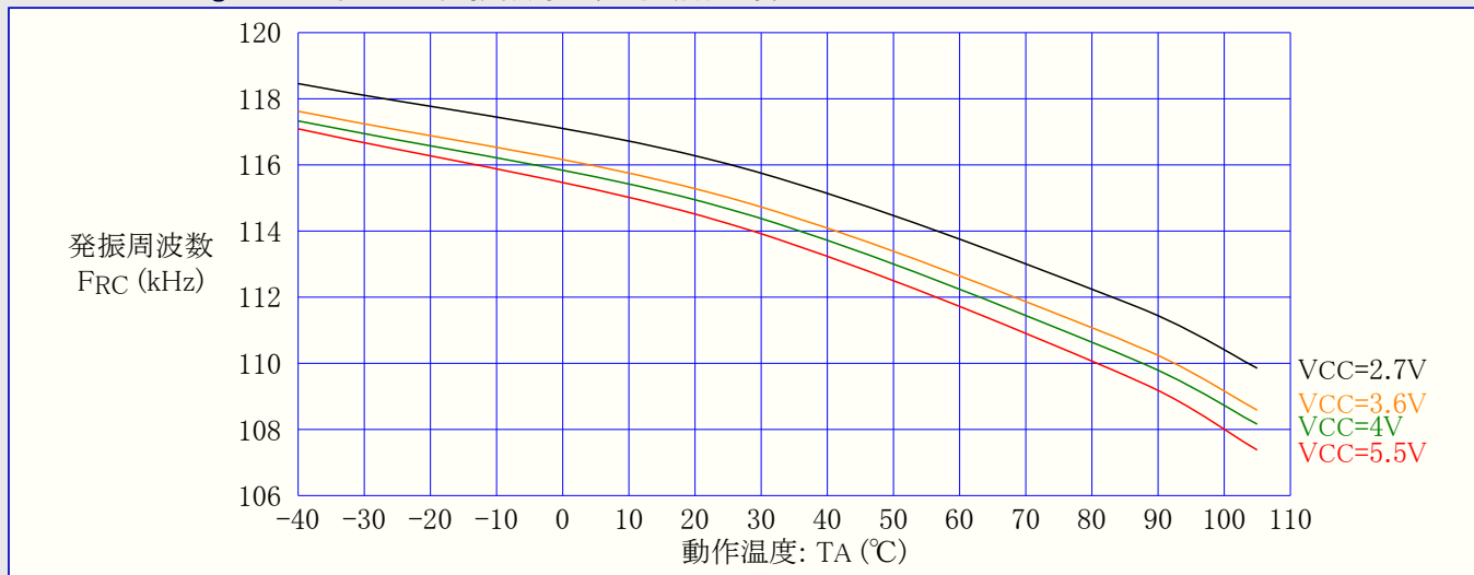
図31-366. ATmega328P: ウォッチドッグ発振器周波数 対 動作温度
