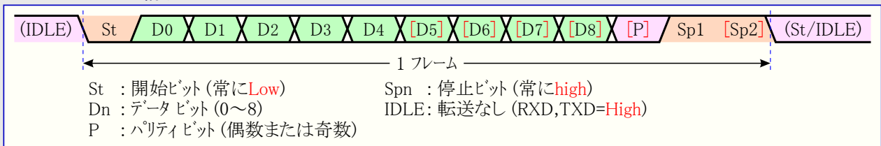
図20-4. 17フレームの構成
