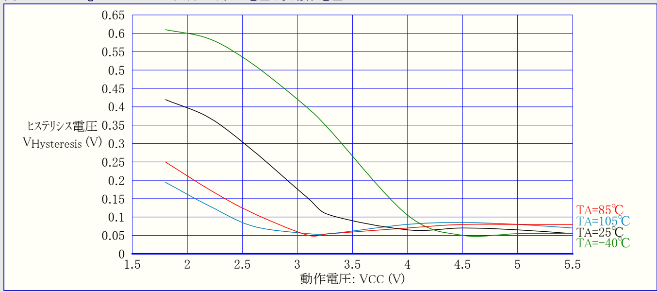
図31-77. ATmega48PA: RESET入力ヒステリシス電圧 対 動作電圧
