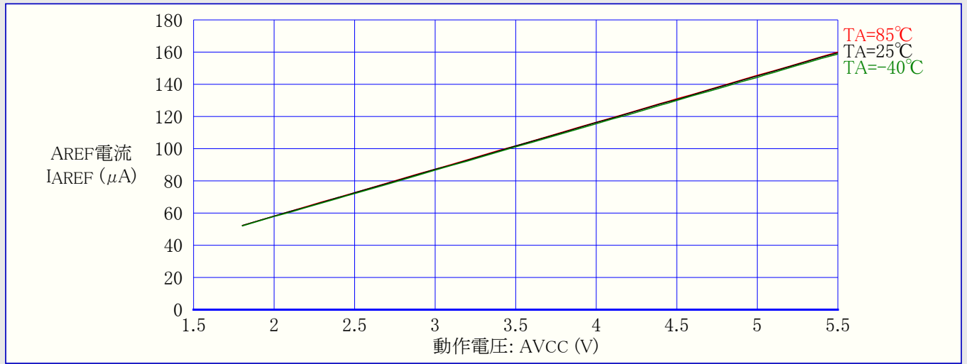
図31-326. ATmega328: アナログ比較器消費電流 対 動作電圧
