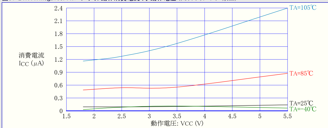
図31-247. ATmega168PA: パワーダウン動作消費電流 対 動作電圧 (ウォッチドッグ タイマ禁止)
