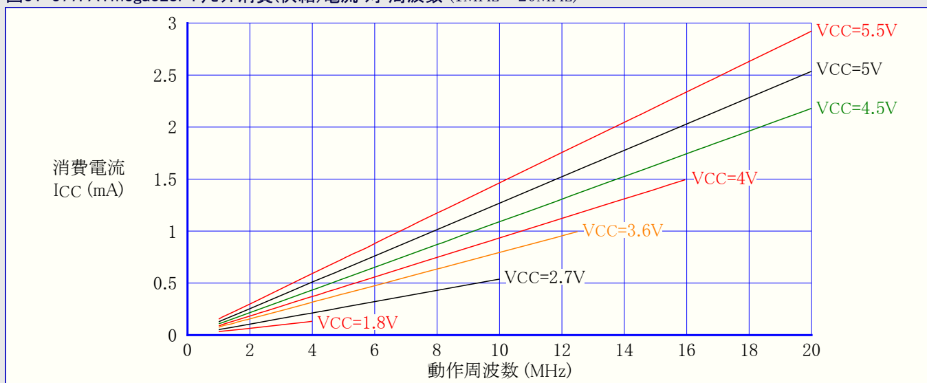
図31-377. ATmega328P:リセット消費(供給)電流 対 周波数 (1MHz~20MHz)
