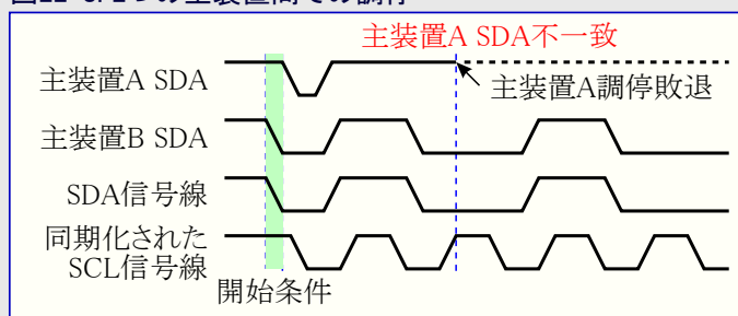
図22-8. 2つの主装置間での調停
