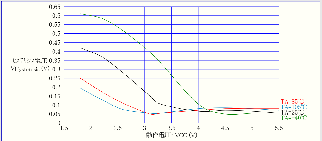
図32-30. ATmega48PA: RESET入力ヒステリシス電圧 対 動作電圧
