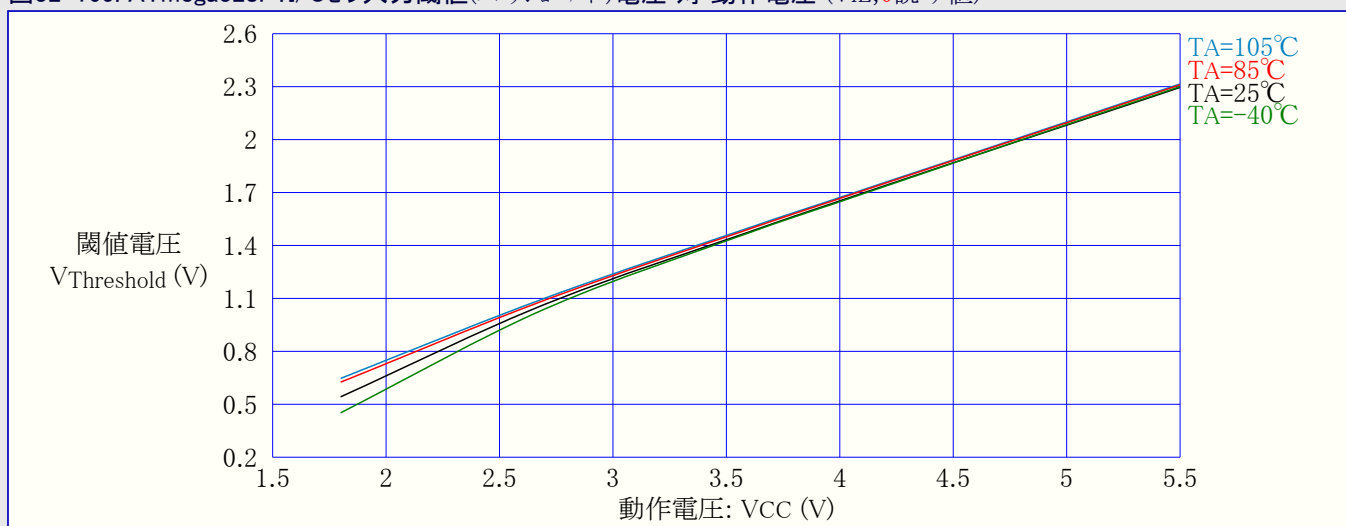
図32-165. ATmega328P:I/Oピン入力閾値(スレッショルド)電圧 対 動作電圧 ( V_{IL} , 0読み値)
