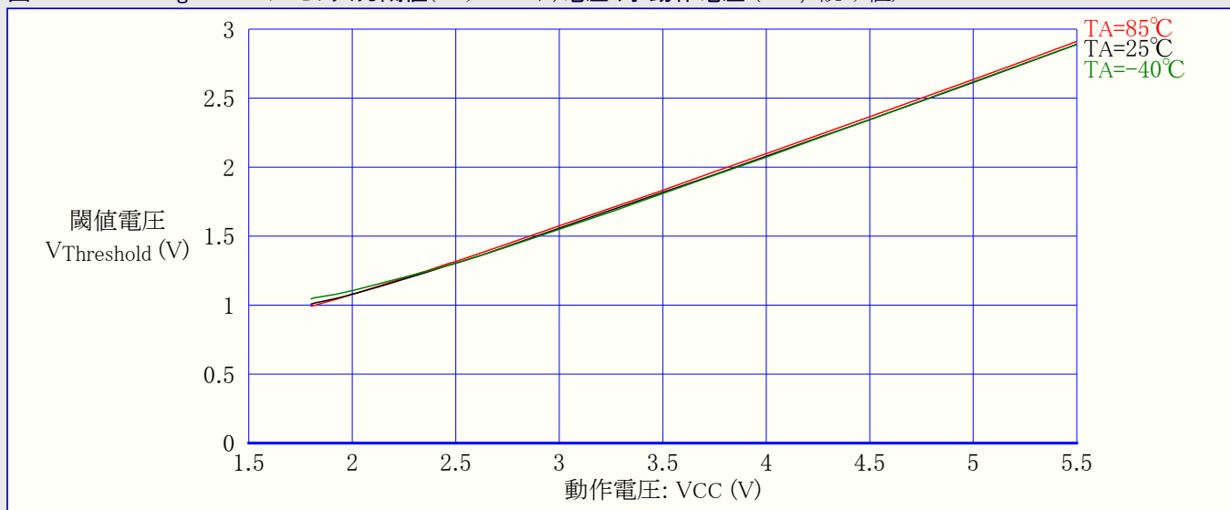
図31-214. ATmega168A:I/Oピン入力閾値(スレッシュホールド)電圧 対 動作電圧 (VIH, 1読み値)
