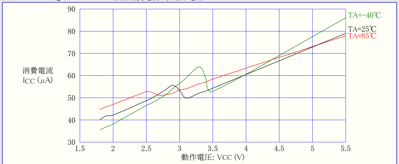
図31-232. ATmega168A: 低電圧検出器(BOD)消費電流 対 動作電圧
