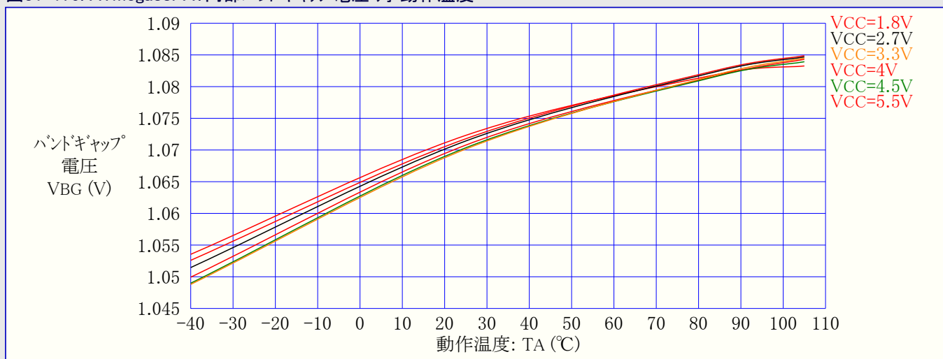
図31-175. ATmega88PA: 内部バンドギャップ電圧 対 動作温度
