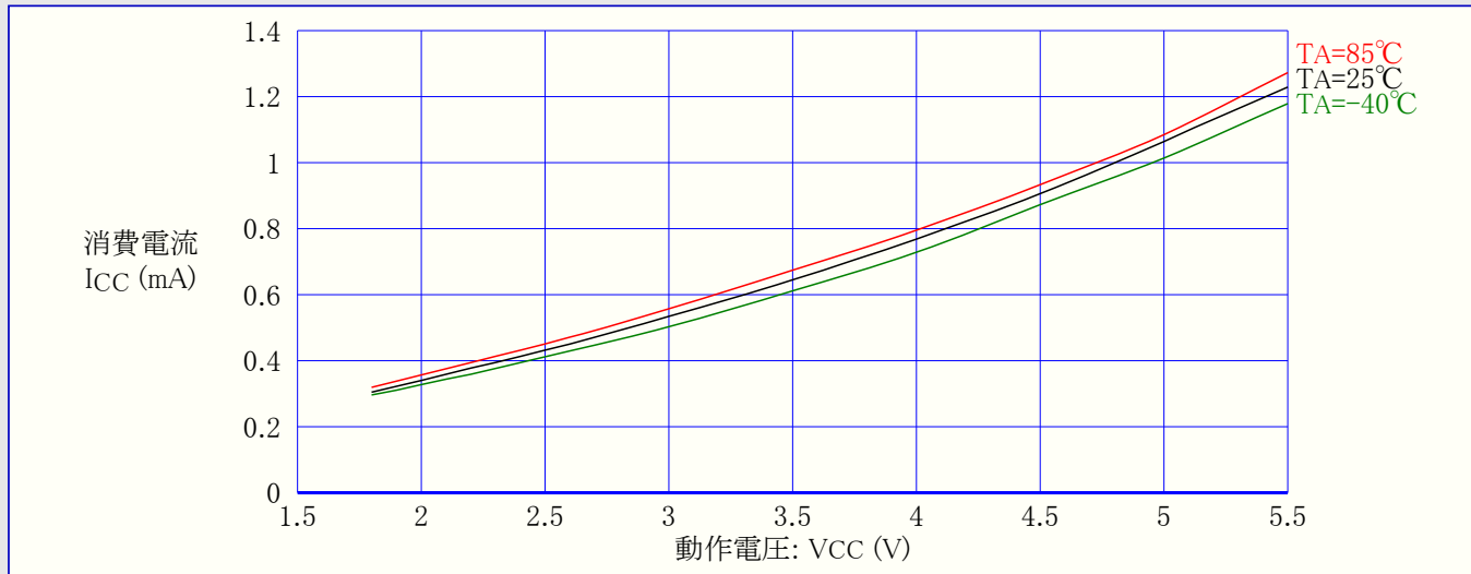
図31-288. ATmega328: 活動動作消費電流 対 動作電圧 (内蔵RC発振器, CKDIV8=プログラム(0), 1MHz)
