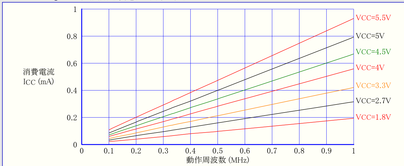
図31-95. ATmega88A: 活動動作消費電流 対 周波数 (100kHz~1MHz)
