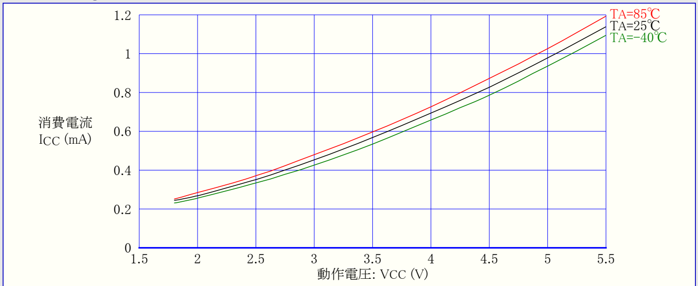
図31-10. ATmega48A: アイドル動作消費電流 対 動作電圧 (内蔵RC発振器, 8MHz)
