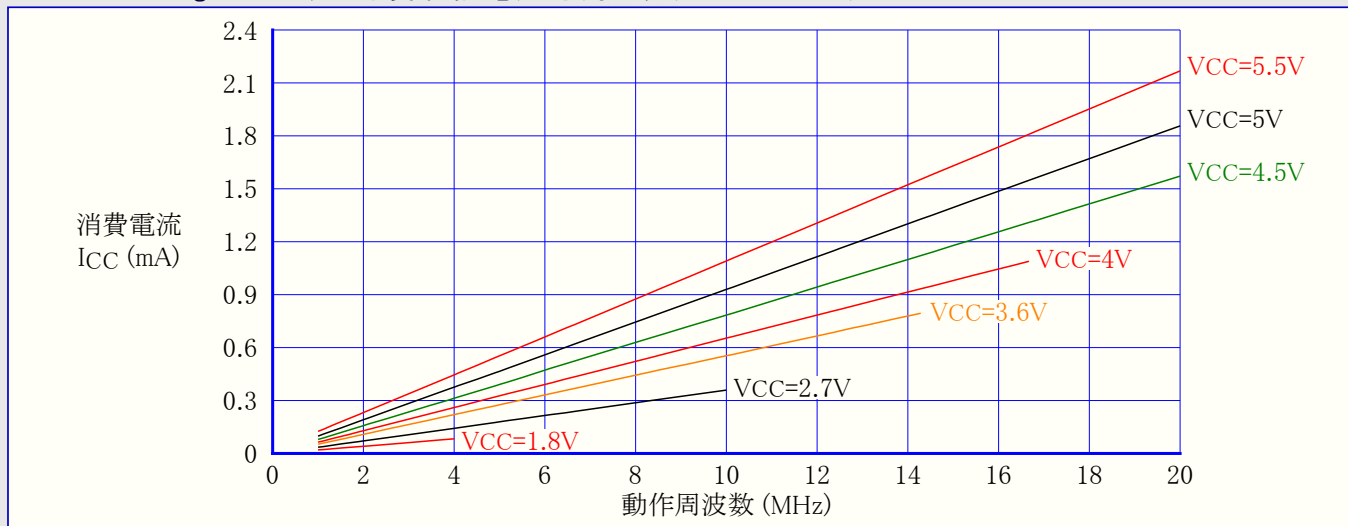
図32-138. ATmega168PA:リセット消費(供給)電流 対 周波数 (1MHz~20MHz)
