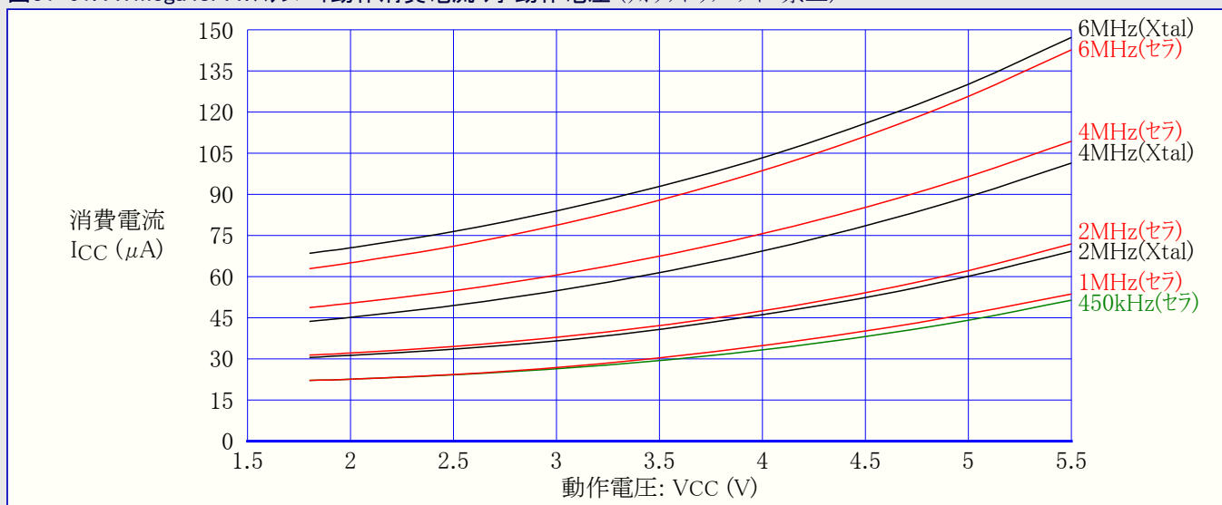
図31-61. ATmega48PA:スタンバイ動作消費電流 対 動作電圧 (ウォッチドッグ タイマ禁止)
