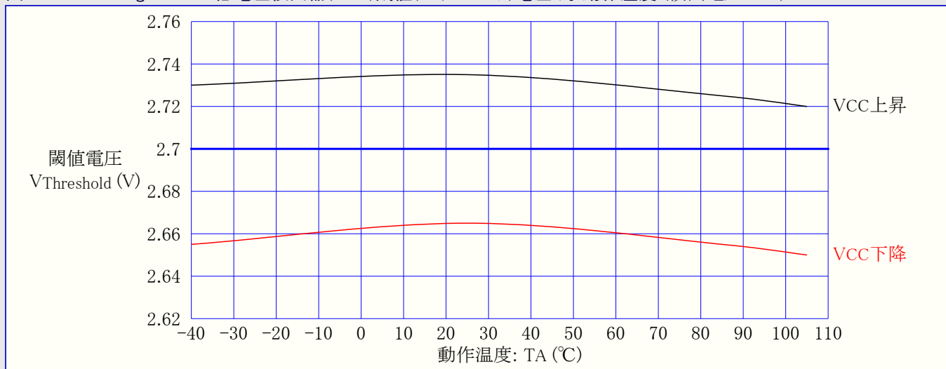
図32-123. ATmega168PA: 低電圧検出器(BOD)閾値(スレッシュホールド)電圧 対 動作温度 (検出電圧2.7V)
