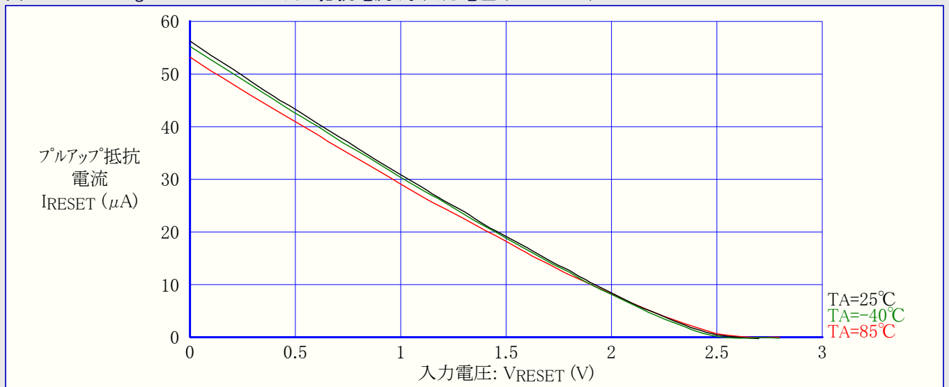
図31-208. ATmega168A: RESETプルアップ抵抗電流 対 入力電圧 (VCC=2.7V)
