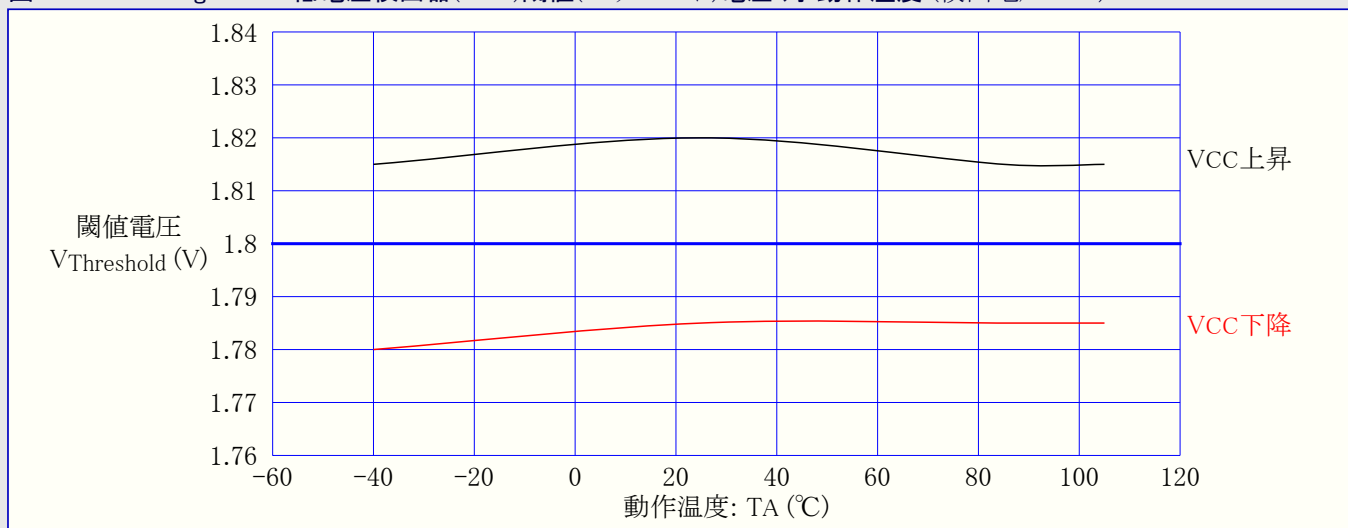
図31-172. ATmega88PA: 低電圧検出器(BOD)閾値(スレッショルド)電圧 対 動作温度 (検出電圧1.8V)
