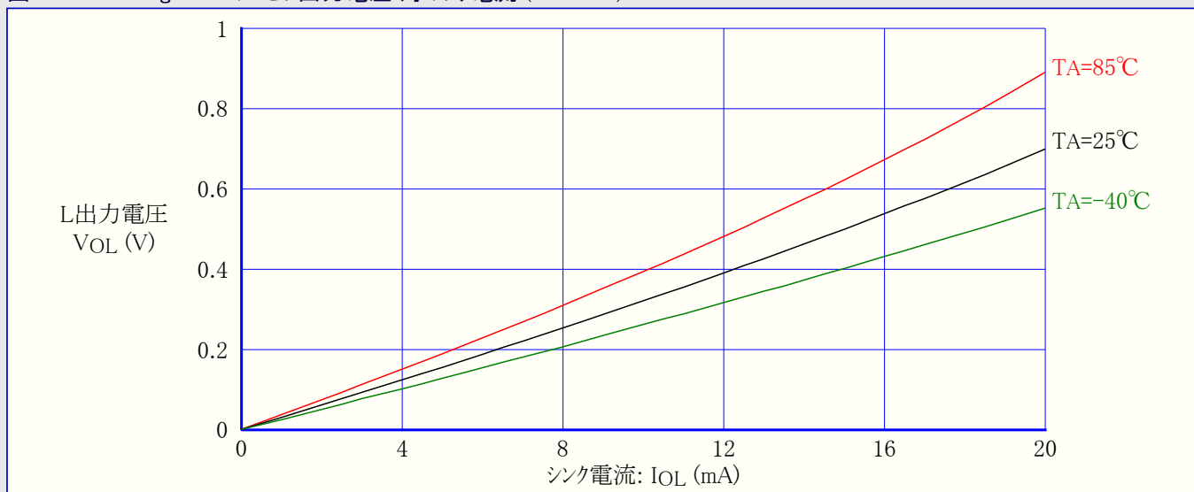
図31-21. ATmega48A: I/Oピン出力電圧 対 シンク電流 (VCC=3V)
