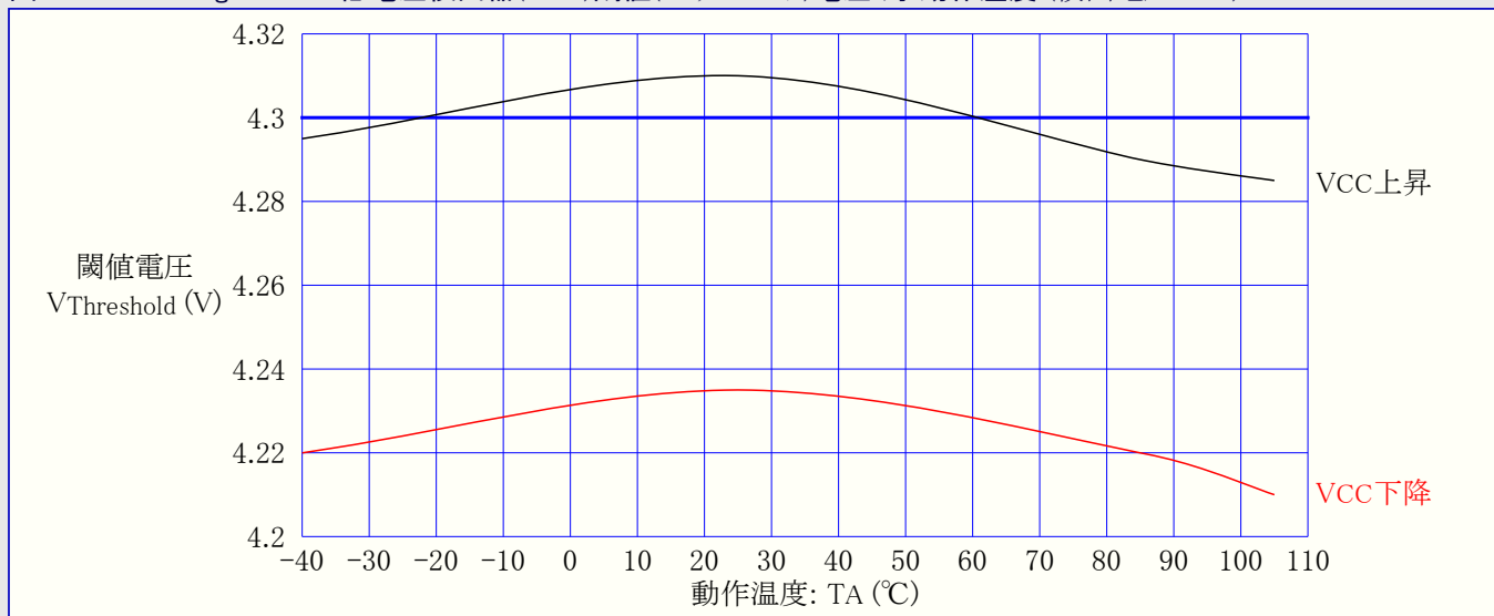
図32-124. ATmega168PA: 低電圧検出器(BOD)閾値(スレッシュホールド)電圧 対 動作温度 (検出電圧4.3V)
