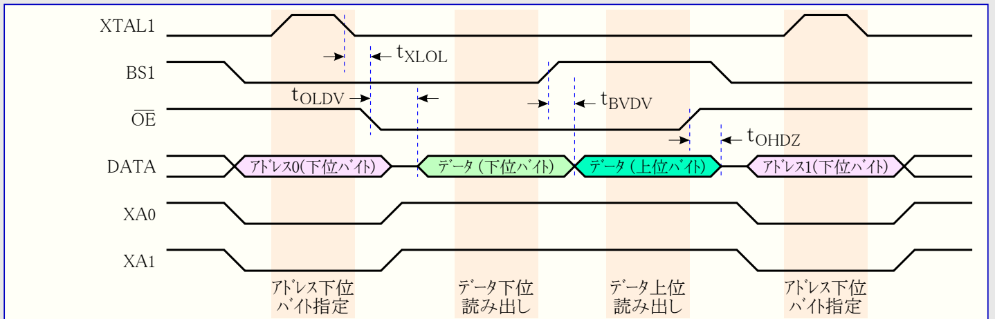
図29-8. 並列プログラミング タイミング (同一ページ読み出しでの必要条件)
