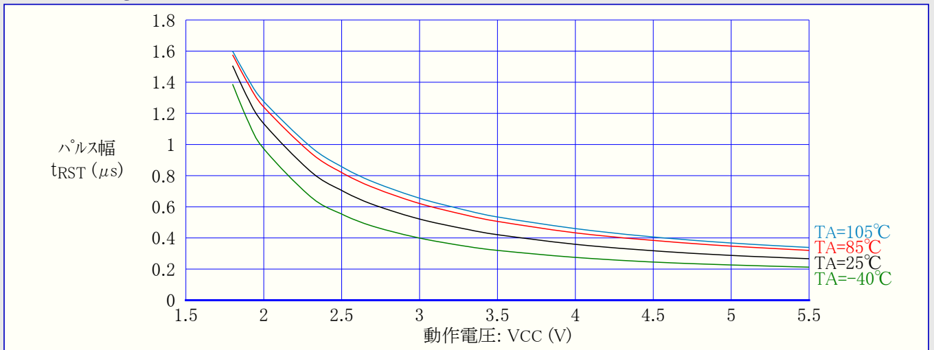
図32-91. ATmega88PA: 最小リセットパルス幅 対 動作電圧
