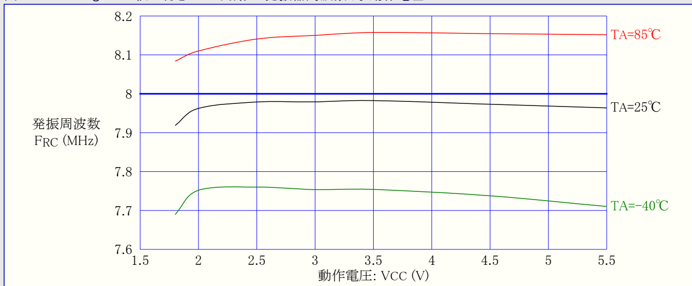
図31-37. ATmega48A: 校正付き8MHz内蔵RC発振器周波数 対 動作電圧
