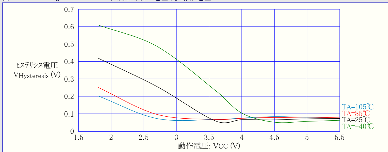
図31-266. ATmega168PA: RESET入力ヒステリシス電圧 対 動作電圧
