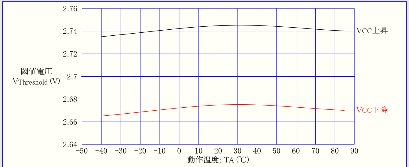
図31-127. ATmega88A: 低電圧検出器(BOD)閾値(スレッショルド)電圧 対 動作温度 (検出電圧4.3V)
