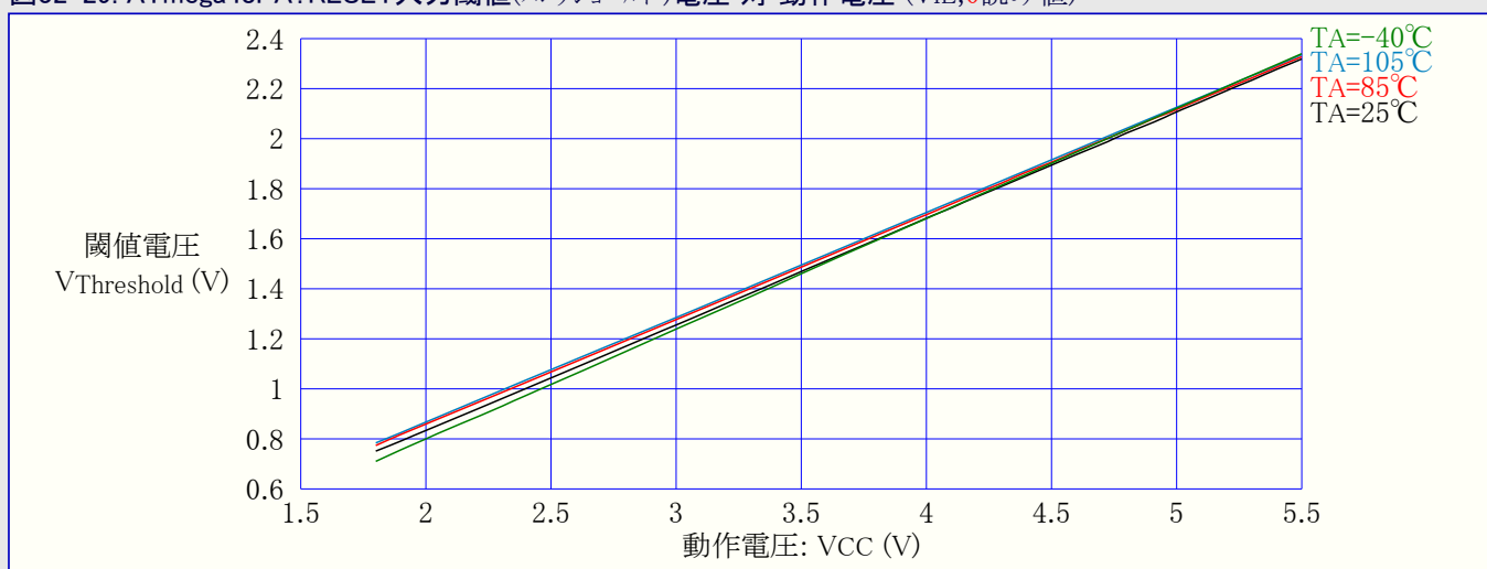
図32-29. ATmega48PA:RESET入力閾値(スレッショルド)電圧 対 動作電圧 (VIL,0読み値)
