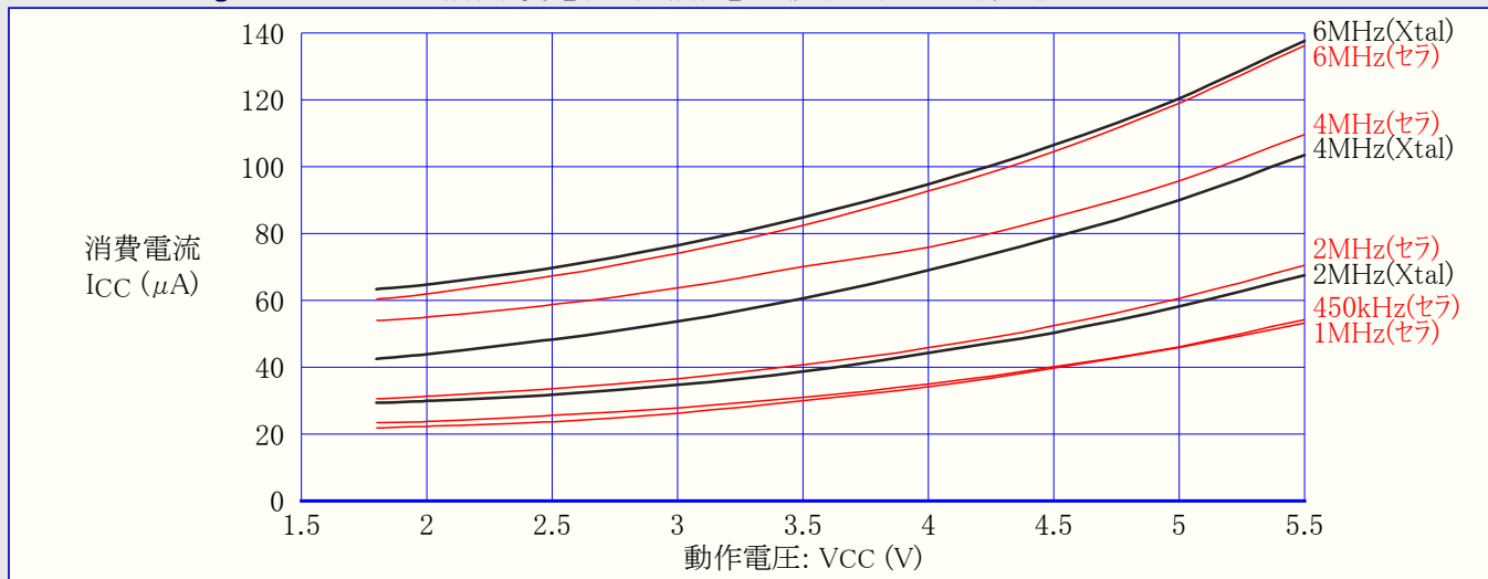
図31-250. ATmega168PA:スタンバイ動作消費電流 対 動作電圧 (ウォッチドッグ タイマ禁止)
