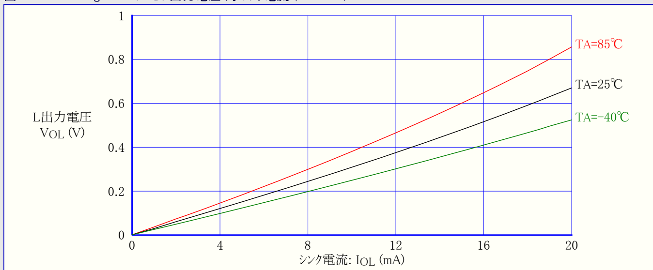
図31-115. ATmega88A: I/Oピン出力電圧 対 シンク電流 (VCC=3V)
