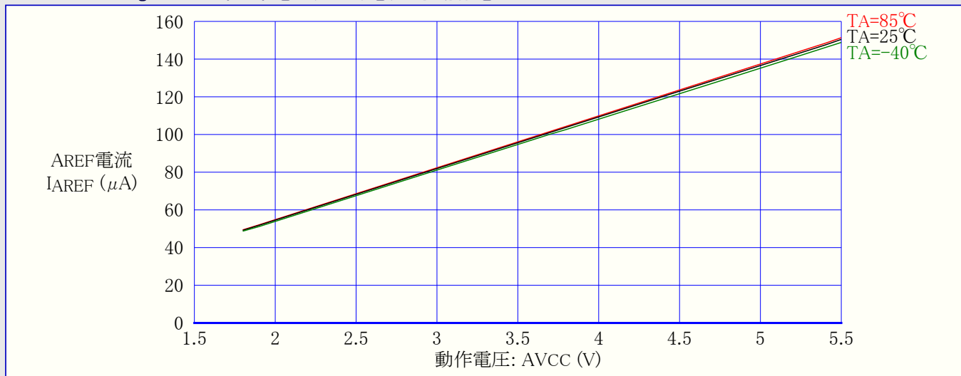
図31-135. ATmega88A: 外部基準電圧(AREF)電流 対 動作電圧
