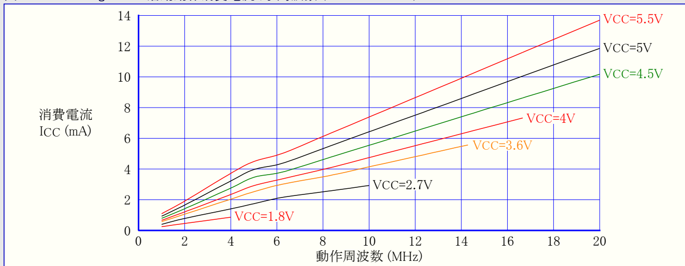
図31-333. ATmega328P: 活動動作消費電流 対 周波数 (1MHz~20MHz)
