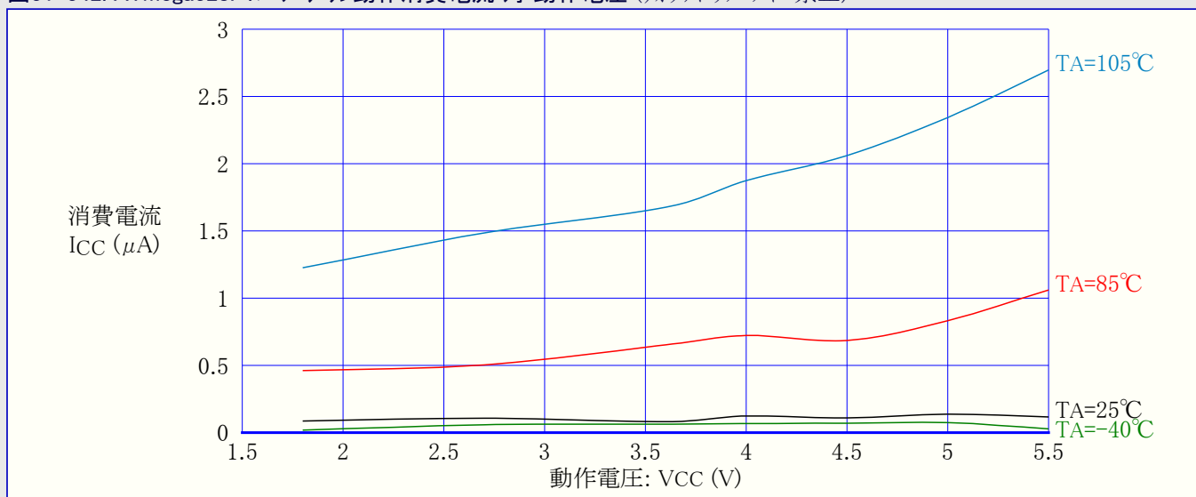
図31-342. ATmega328P: パワーダウン動作消費電流 対 動作電圧 (ウォッチドッグ タイマ禁止)
