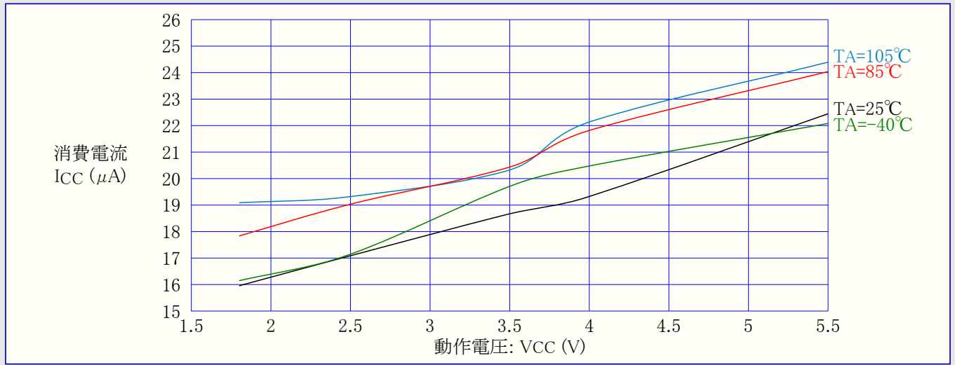
図32-42. ATmega48PA: 低電圧検出器(BOD)消費電流 対 動作電圧
