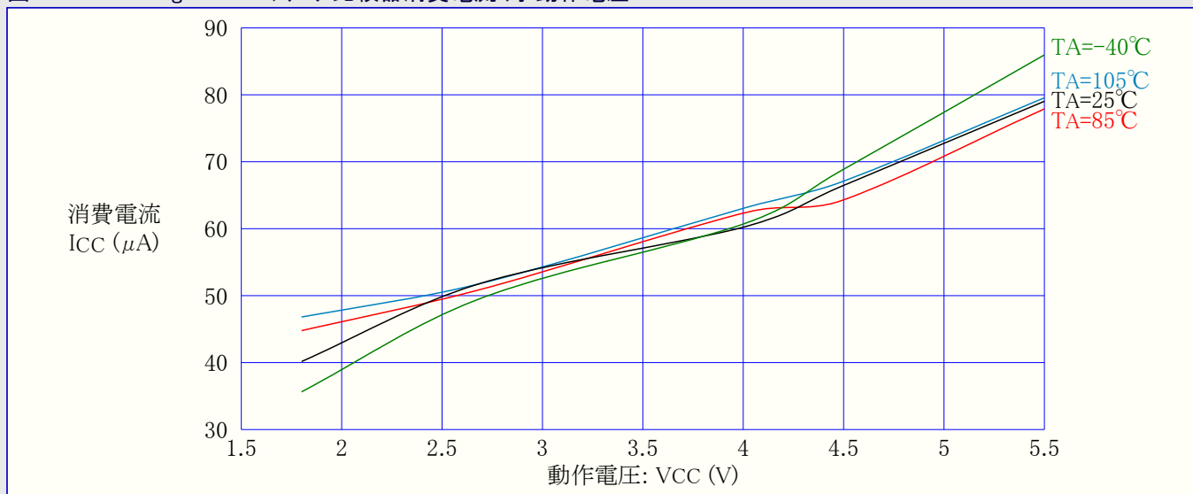
図31-279. ATmega168PA: アナログ比較器消費電流 対 動作電圧
