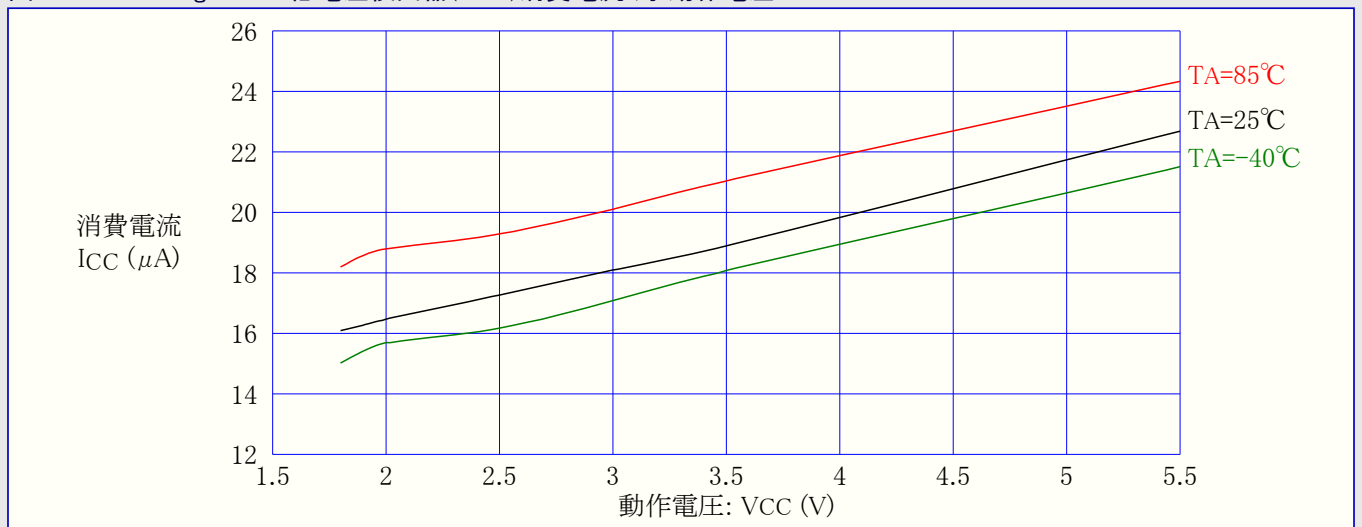
図31-232. ATmega168A: 低電圧検出器(BOD)消費電流 対 動作電圧
