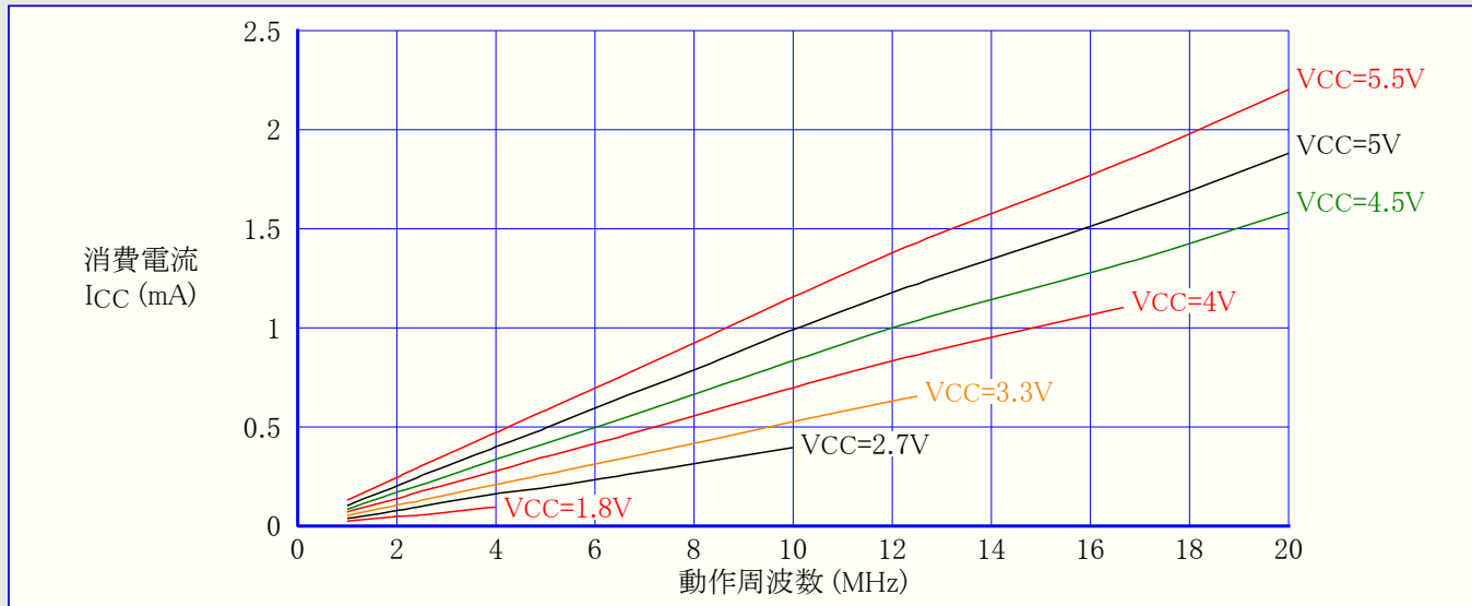
図32-53. ATmega88PA:アイドル動作消費電流 対 周波数 (1MHz~20MHz)
