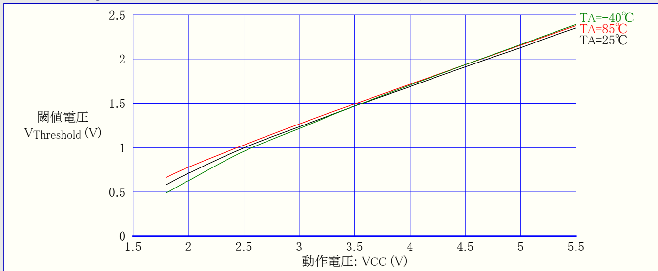
図31-120. ATmega88A:I/Oピン入力閾値(スレッショルド)電圧 対 動作電圧 (VIL,0読み値)
