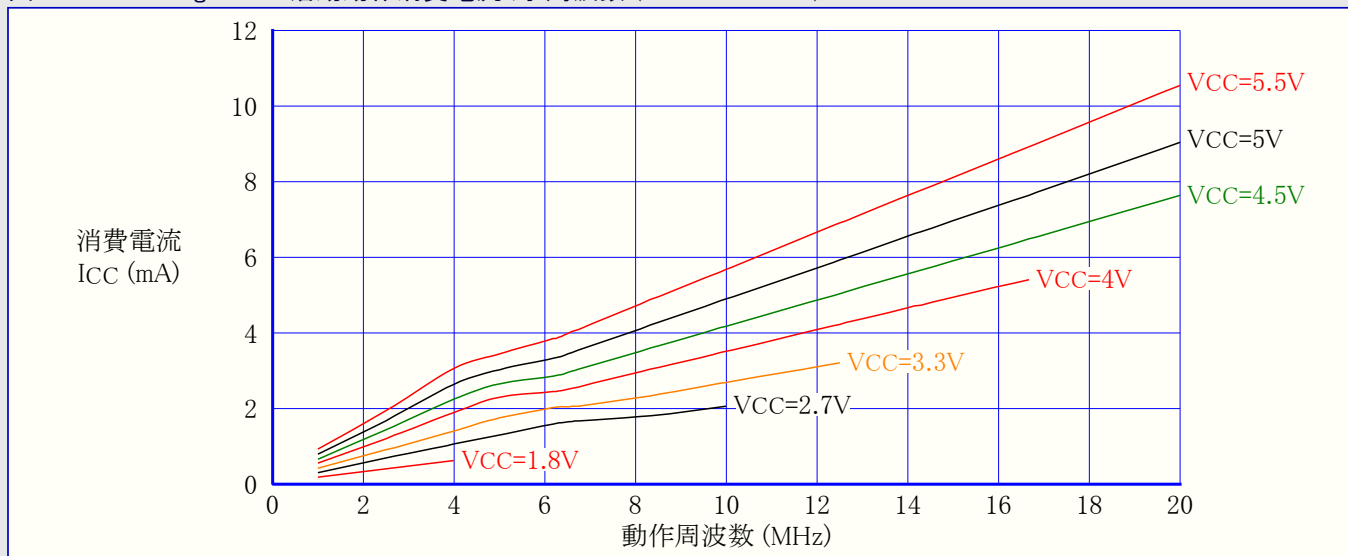
図31-191. ATmega168A: 活動動作消費電流 対 周波数 (1MHz~20MHz)
