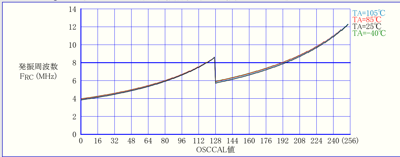
図32-83. ATmega88PA: 校正付き8MHz内蔵RC発振器周波数 対 発振校正(OSCCAL)値
