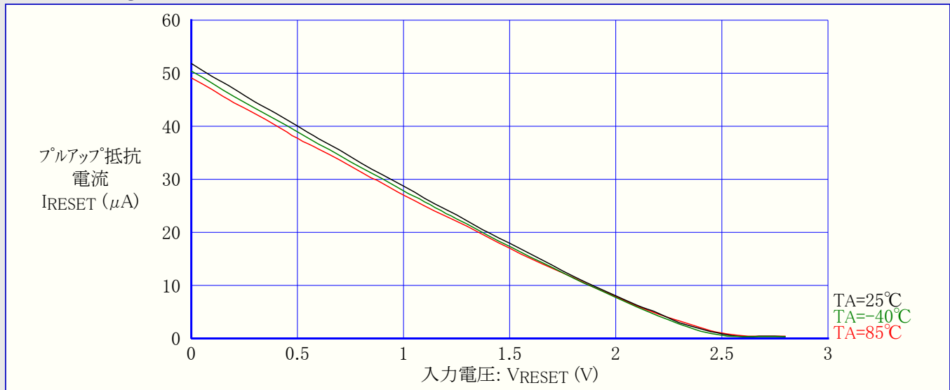
図31-19. ATmega48A: RESETプルアップ抵抗電流 対 入力電圧 (VCC=2.7V)
