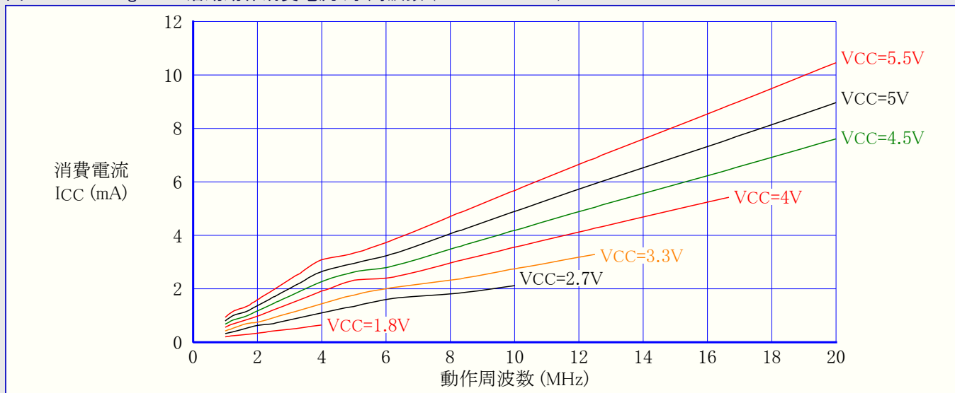
図31-96. ATmega88A: 活動動作消費電流 対 周波数 (1MHz~20MHz)
