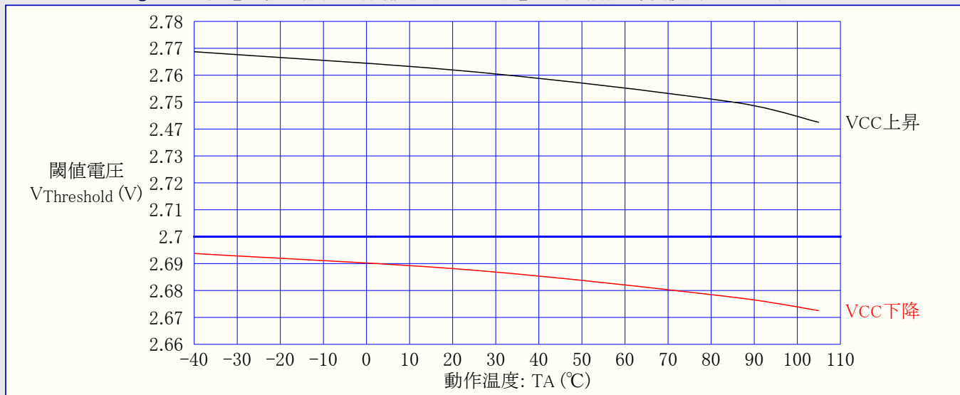
図31-363. ATmega328P: 低電圧検出器(BOD)閾値(スレッシュホールド)電圧 対 動作温度 (検出電圧2.7V)
