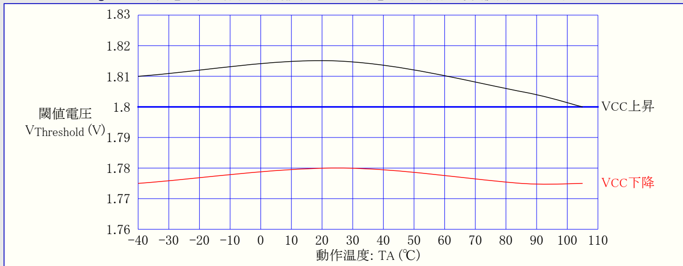
図32-122. ATmega168PA: 低電圧検出器(BOD)閾値(スレッシュホールド)電圧 対 動作温度 (検出電圧1.8V)
