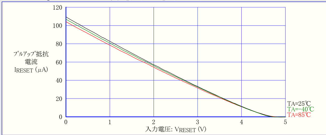
図31-209. ATmega168A: RESETフルアップ抵抗電流 対 入力電圧 (VCC=5V)
