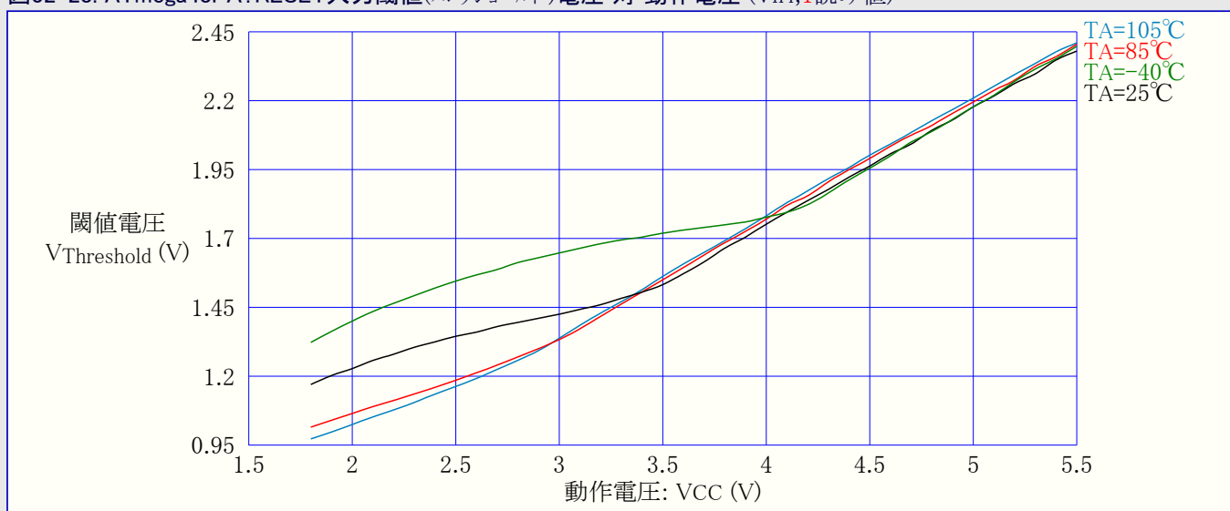
図32-29. ATmega48PA:RESET入力閾値(スレッショルド)電圧 対 動作電圧 (VIL,0読み値)
