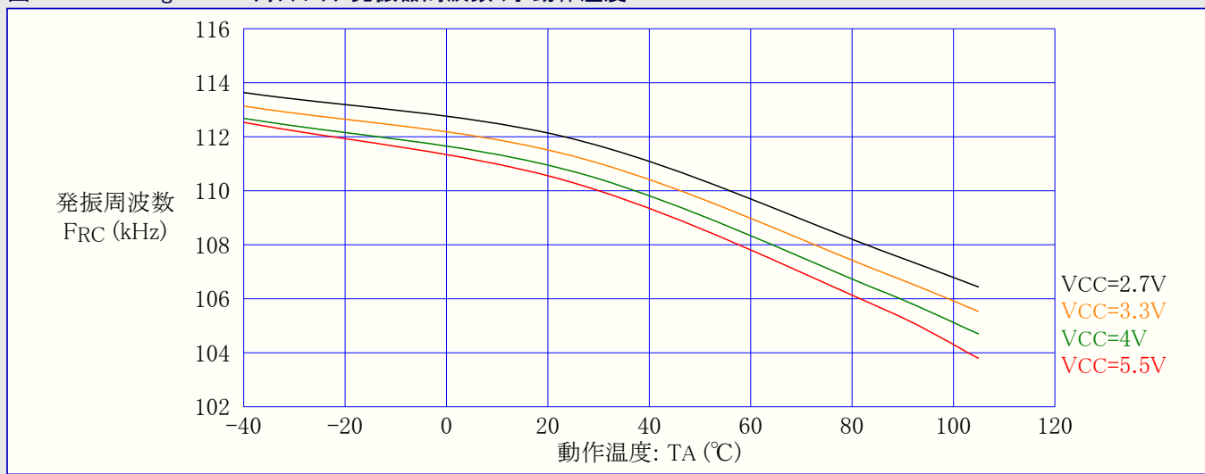
図32-79. ATmega88PA: ウォッチドッグ発振器周波数 対 動作温度
