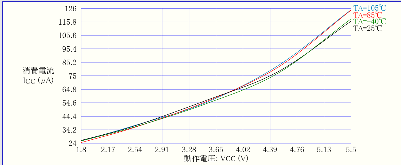
図32-3. ATmega48PA: 活動動作消費電流 対 動作電圧 (内蔵WDT発振器, 128kHz)
