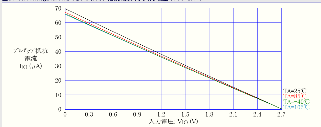
図31-63. ATmega48PA:I/Oピンプルアップ抵抗電流 対 入力電圧 ( V_{CC}=2.7V )
