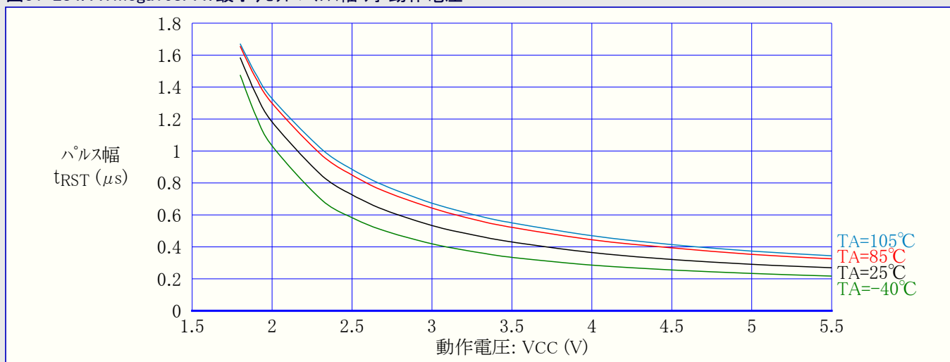
図31-284. ATmega168PA:最小リセットパルス幅 対 動作電圧
