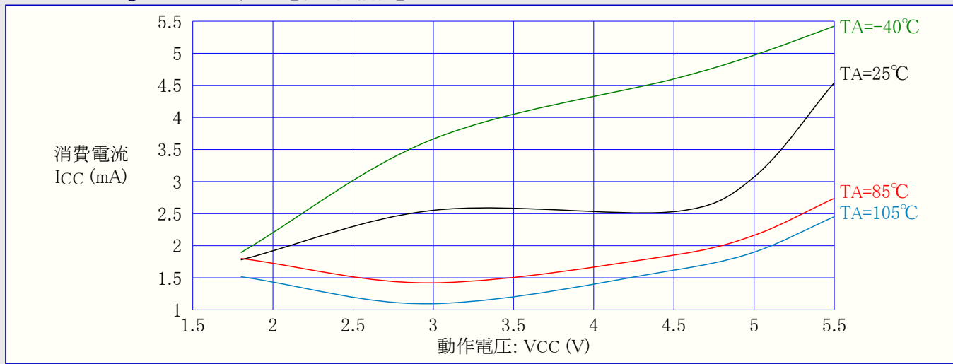
図31-91. ATmega48PA:プログラミング電流 対 動作電圧
