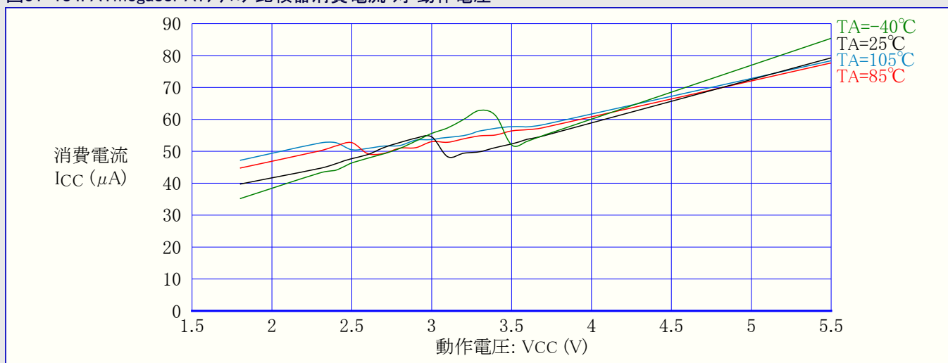
図31-184. ATmega88PA: アナログ比較器消費電流 対 動作電圧
