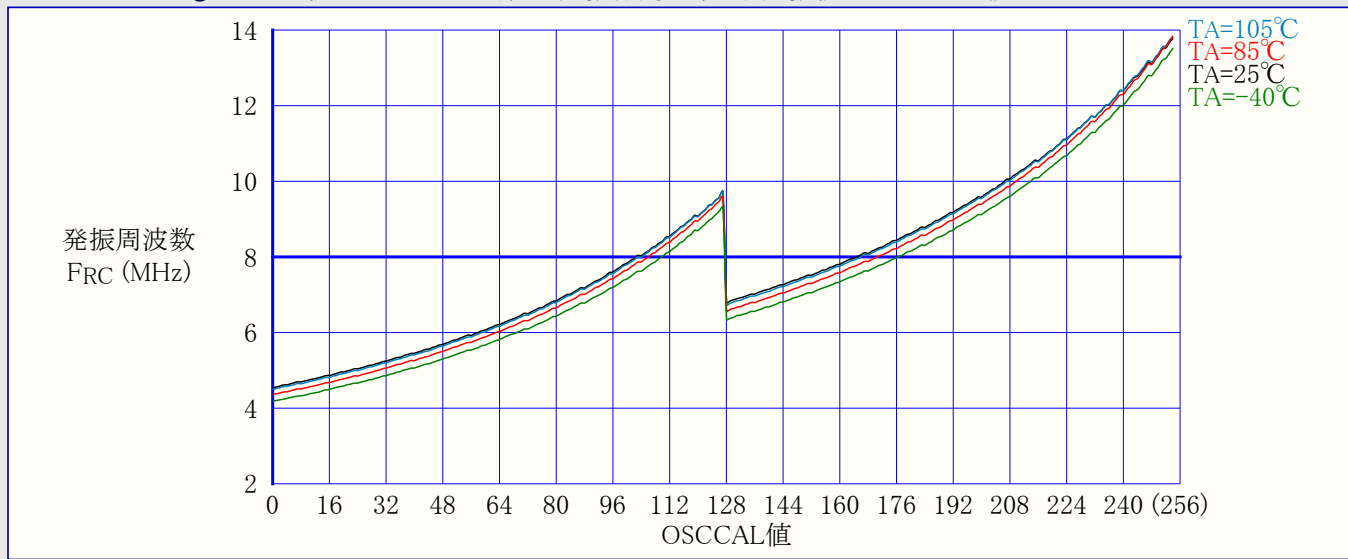
図32-131. ATmega168PA: 校正付き8MHz内蔵RC発振器周波数 対 発振校正(OSCCAL)値
