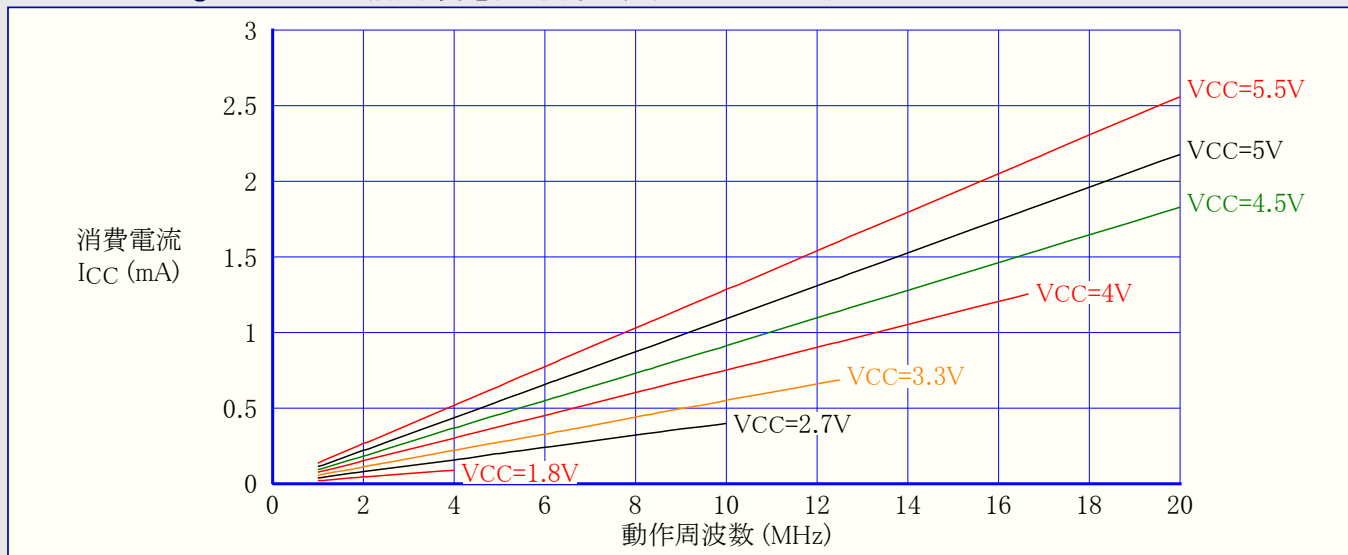
図31-196. ATmega168A: アイドル動作消費電流 対 周波数 (1MHz~20MHz)
