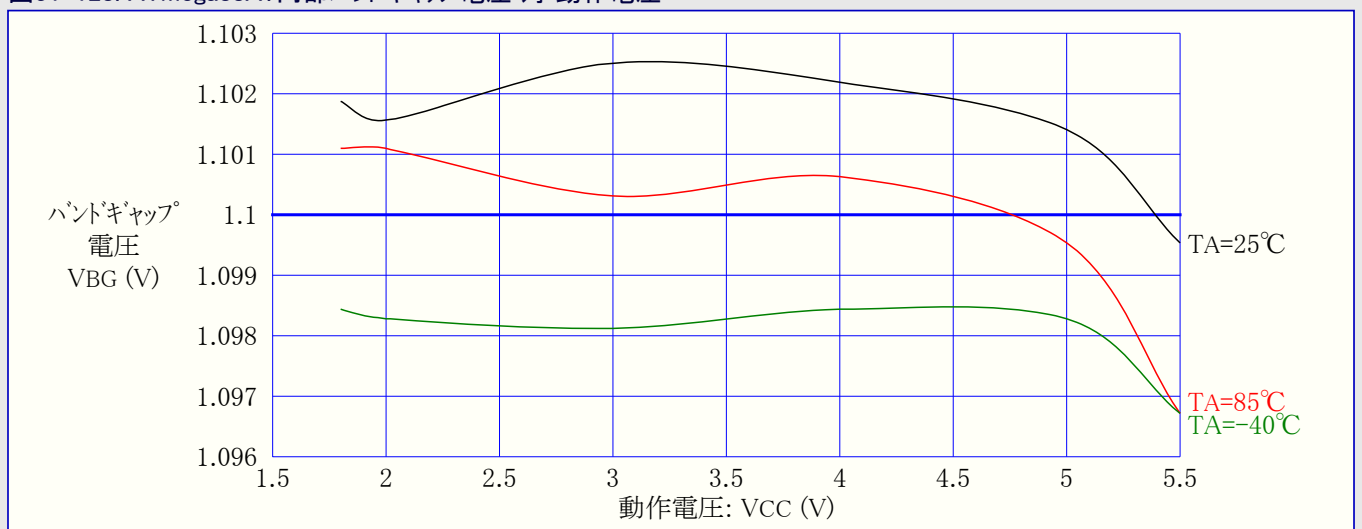
図31-128. ATmega88A: 内部バンドギャップ電圧 対 動作電圧
