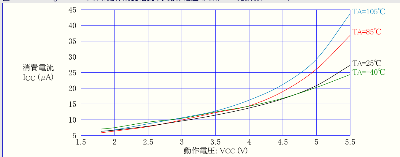
図32-99. ATmega168PA: アイドル動作消費電流 対 動作電圧 (内蔵WDT発振器, 128kHz)
