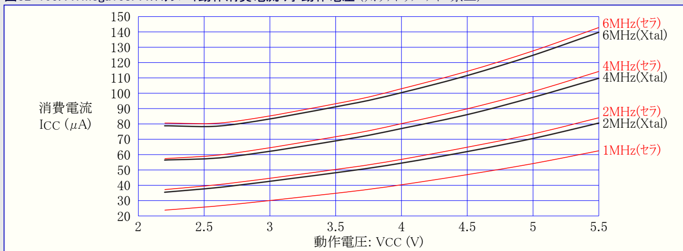
図32-105. ATmega168PA:スタンバイ動作消費電流 対 動作電圧 (ウォッチドッグ タイマ禁止)
