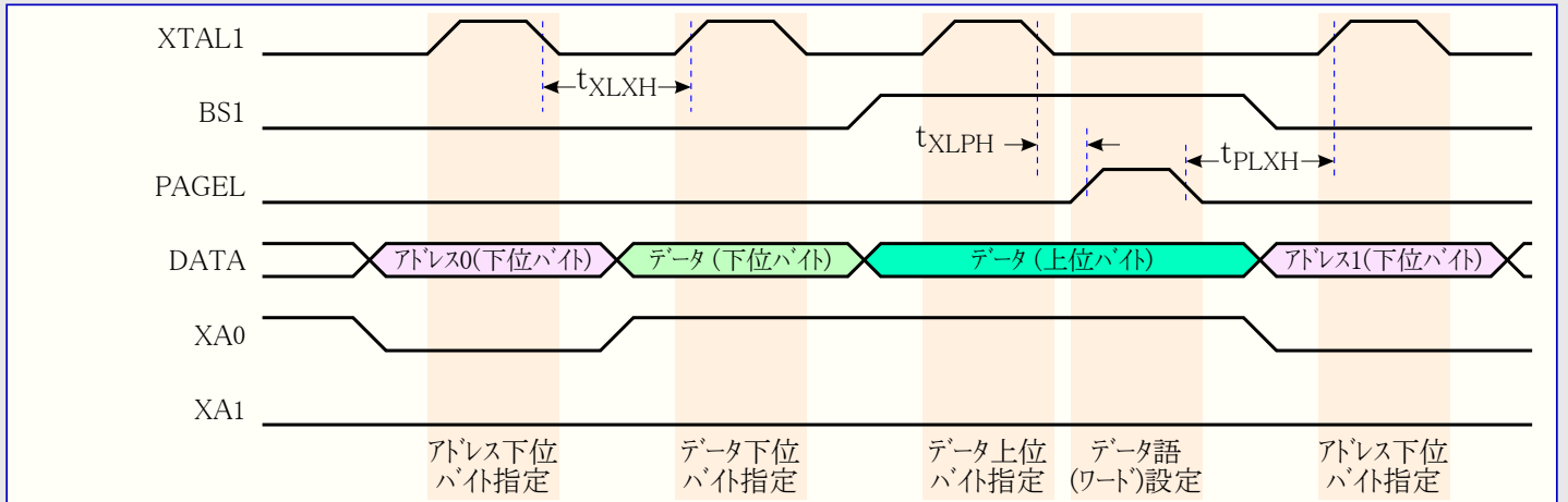
図29-7. 並列プログラミング タイミング (ページ設定での必要条件)
