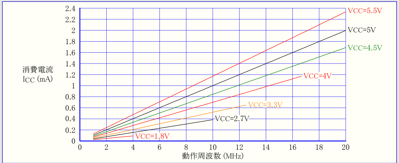
図32-45. ATmega48PA:リセット消費(供給)電流 対 周波数 (1MHz~20MHz)
