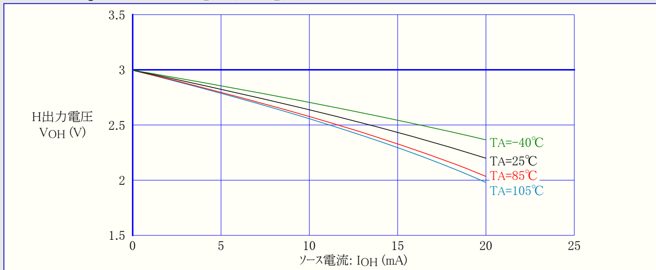
図32-68. ATmega88PA:I/Oピン出力電圧 対 ソース電流 (VCC=3V)
