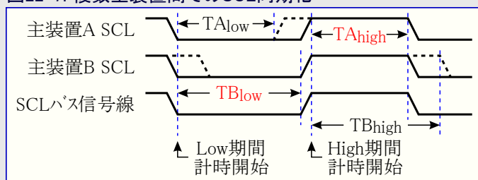
図22-7. 複数主装置間でのSCL同期化
