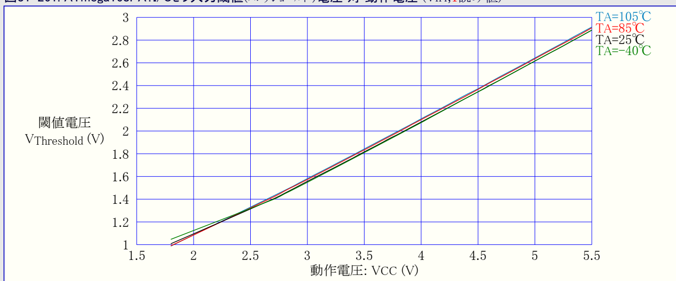
図31-261. ATmega168PA:I/Oピン入力閾値(スレッショルド)電圧 対 動作電圧 (VIH,1読み値)
