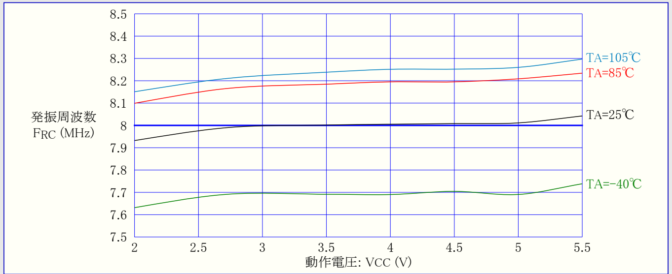
図31-274. ATmega168PA: 校正済み8MHz内蔵RC発振器周波数 対 動作電圧
