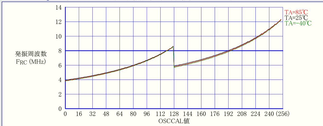
図31-133. ATmega88A: 校正付き8MHz内蔵RC発振器周波数 対 発振校正(OSCCAL)値
