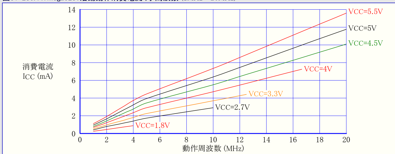
図31-286. ATmega328: 活動動作消費電流 対 周波数 (1MHz~20MHz)
