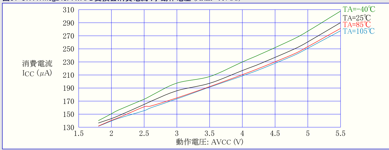
図31-87. ATmega48PA: A/D変換器消費電流 対 動作電圧 (AREF=AVCC)
