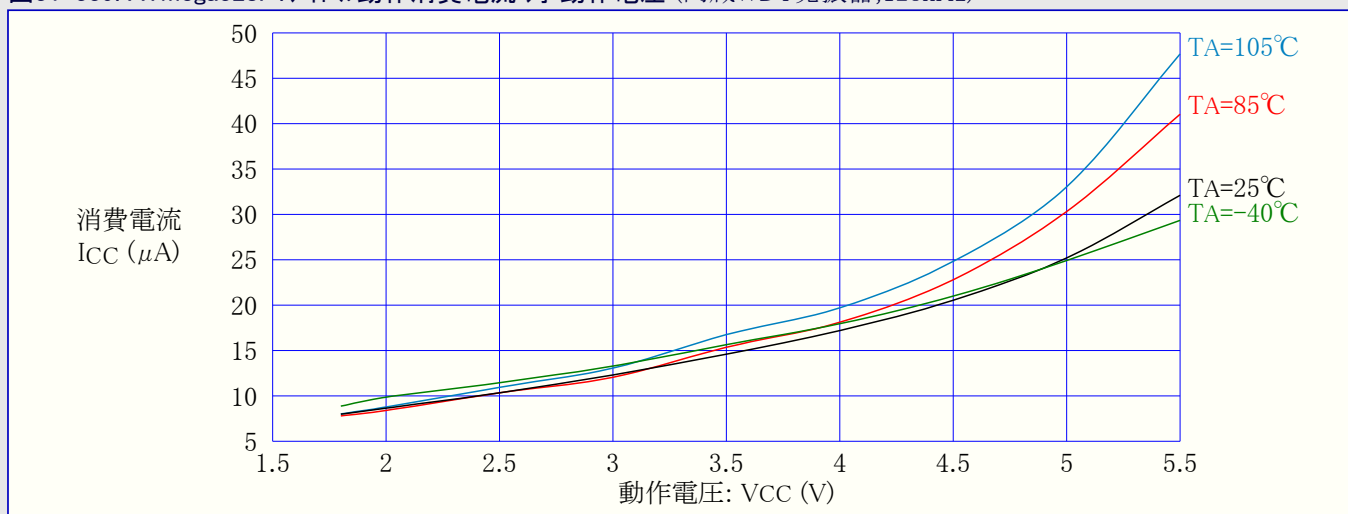
図31-339. ATmega328P: アイドル動作消費電流 対 動作電圧 (内蔵WDT発振器, 128kHz)
