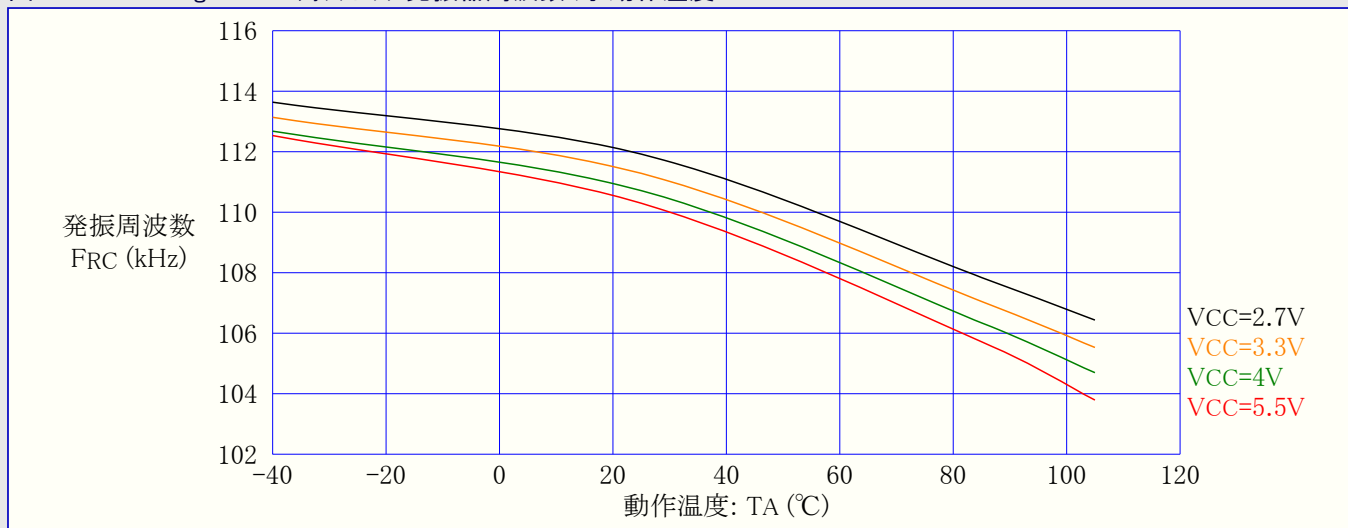
図31-177. ATmega88PA: ウォッチドッグ発振器周波数 対 動作温度
