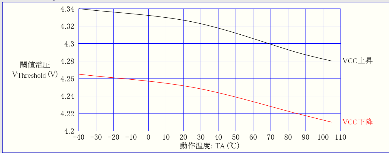
図32-33. ATmega48PA: 低電圧検出器(BOD)閾値(スレッシュホールド)電圧 対 動作温度 (検出電圧4.3V)
