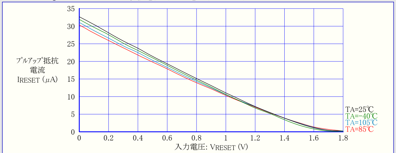
図31-65. ATmega48PA: RESETプルアップ抵抗電流 対 入力電圧 (VCC=1.8V)
