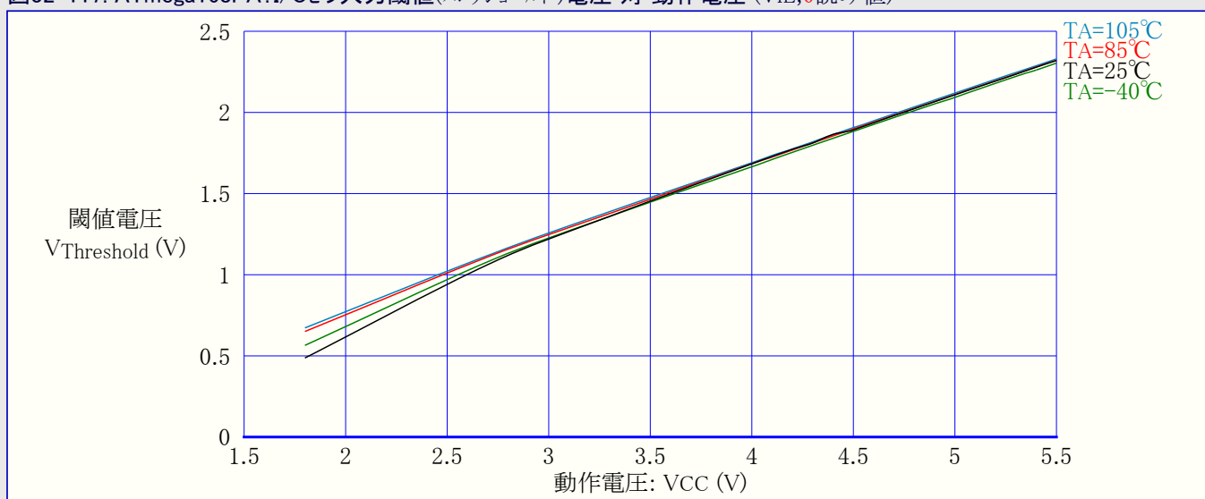
図32-117. ATmega168PA:I/Oピン入力閾値(スレッショルド)電圧 対 動作電圧 ( V_{IL,0} 読み値)
