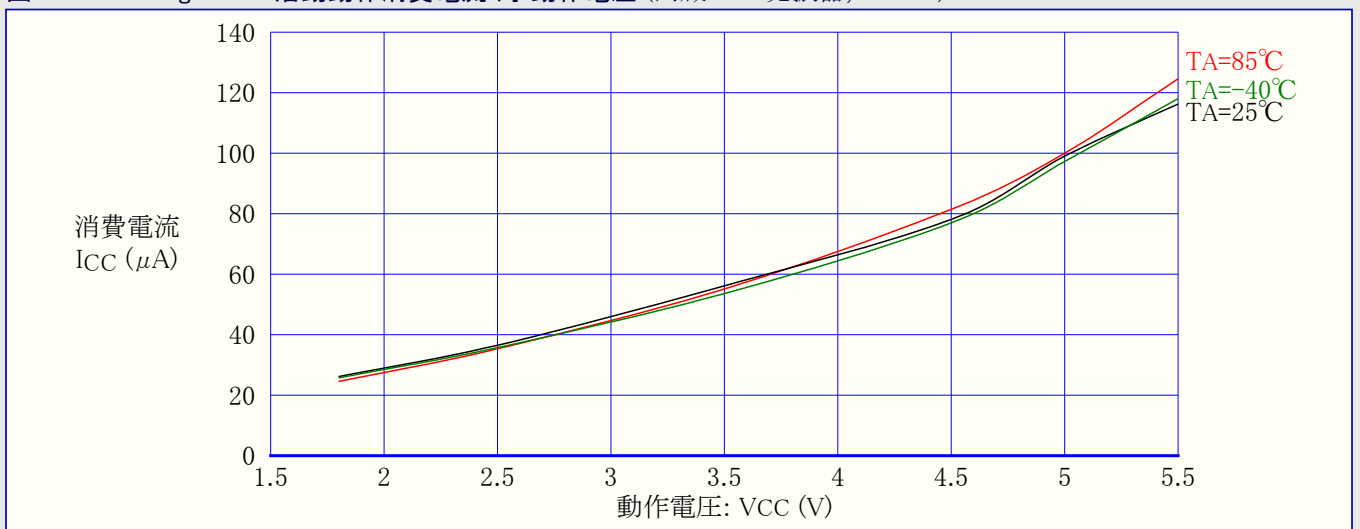
図31-50. ATmega48PA: 活動動作消費電流 対 動作電圧 (内蔵WDT発振器, 128kHz)
