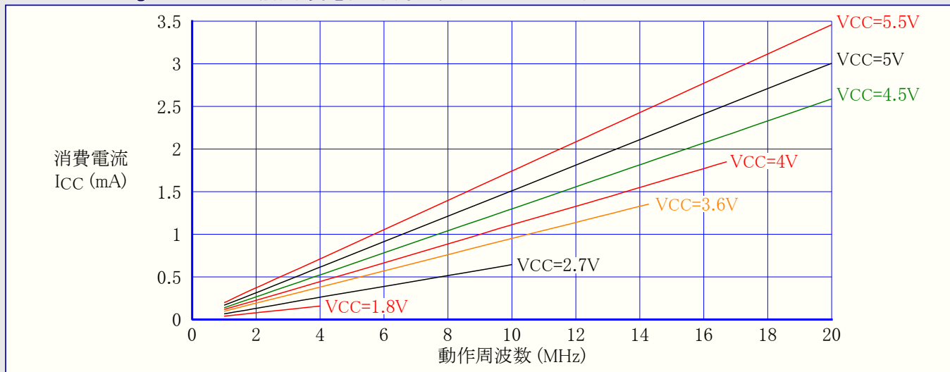
図31-338. ATmega328P: アイドル動作消費電流 対 周波数 (1MHz~20MHz)
