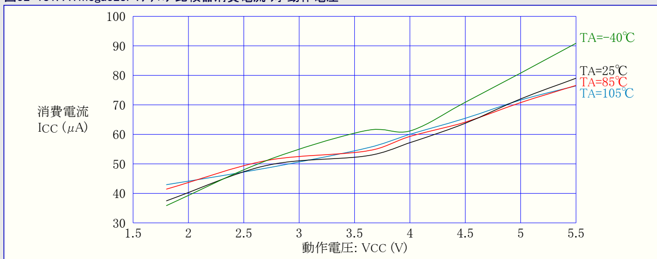
図32-181. ATmega328P: アナログ比較器消費電流 対 動作電圧
