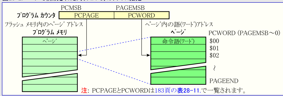
図28-2. ページで構成されたフラッシュメモリのアドレス指定
