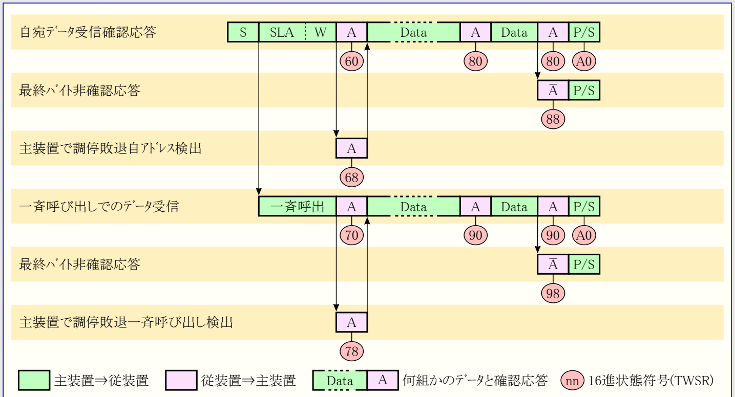
図22-16. 受信従装置動作の形式と状態
