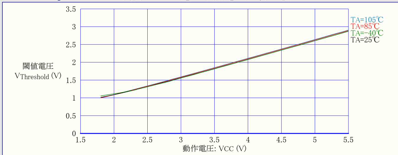
図31-166. ATmega88PA:I/Oピン入力閾値(スレッショルド)電圧 対 動作電圧 (VIH, I読み値)
