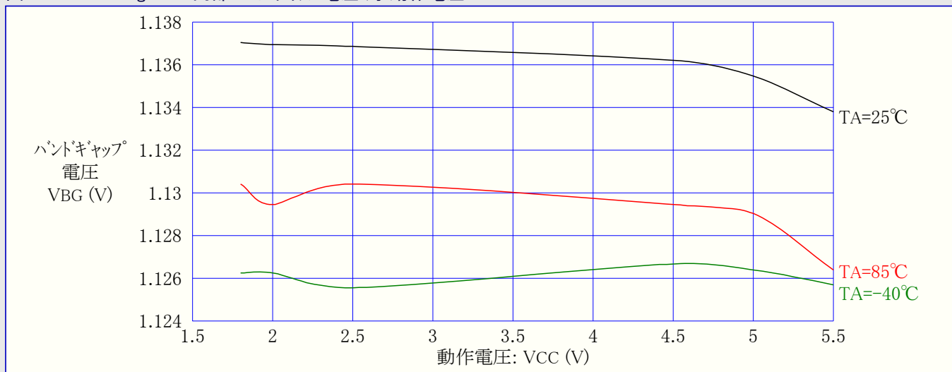
図31-318. ATmega328: 内部バンドギャップ電圧 対 動作電圧
