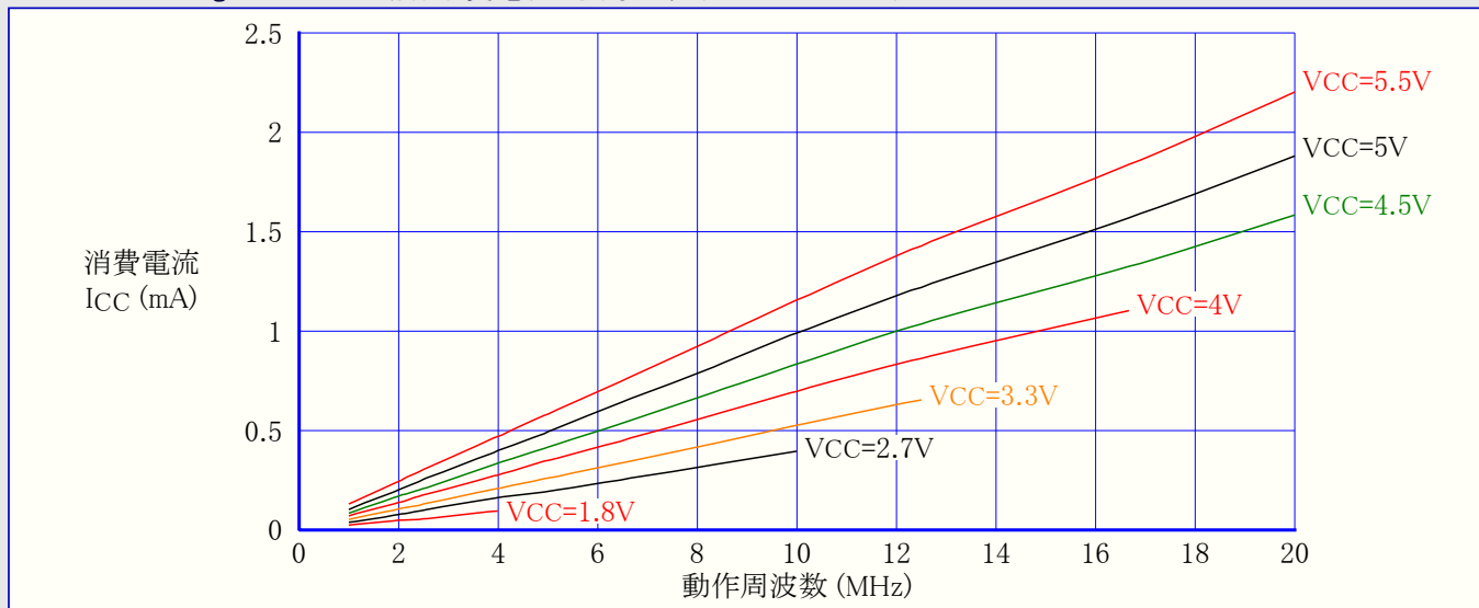
図31-101. ATmega88A: アイドル動作消費電流 対 周波数 (1MHz~20MHz)
