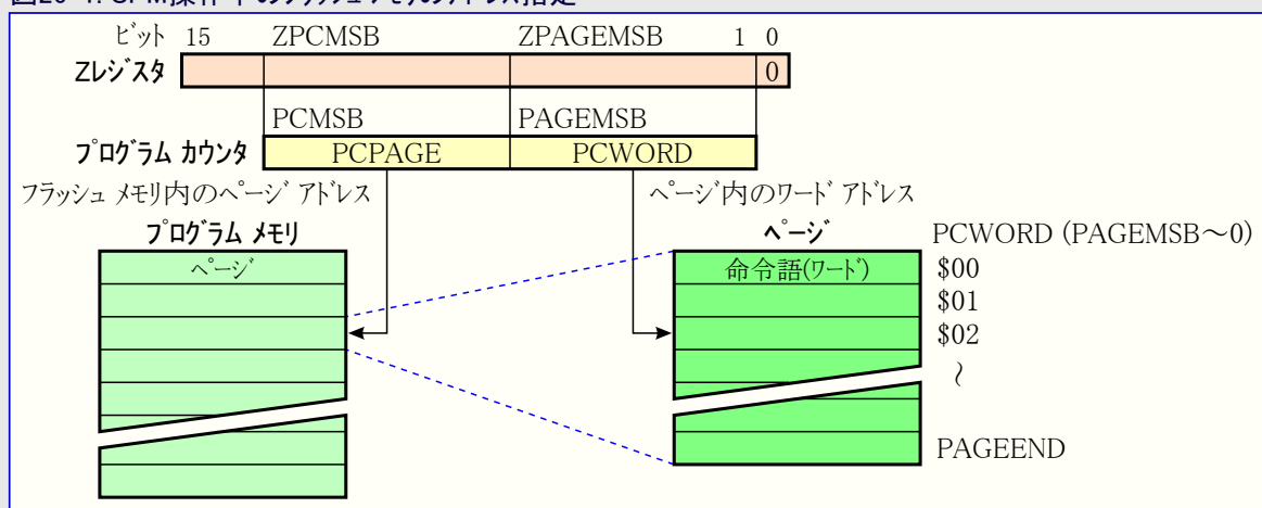
図26-1. SPM操作中のフラッシュメモリのアドレス指定
