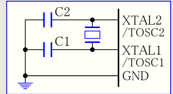
図9-3. クリスタル発振子接続図
