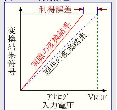
図24-11. 利得誤差
