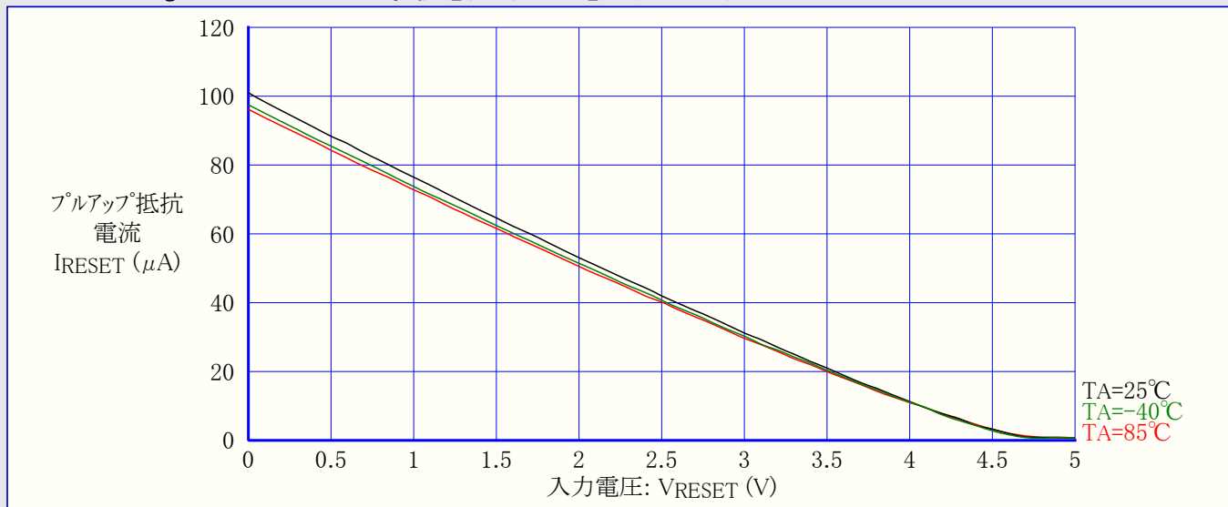
図31-20. ATmega48A: RESETプルアップ抵抗電流 対 入力電圧 (VCC=5V)
