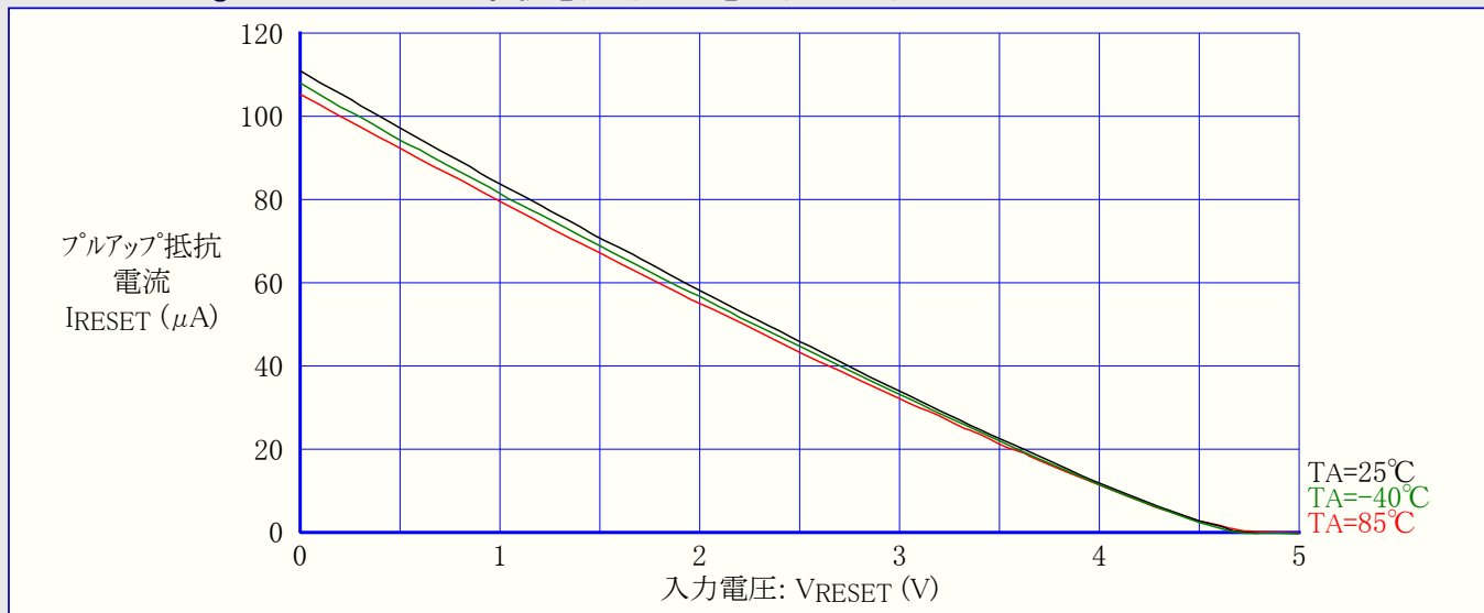
図31-114. ATmega88A: RESETプルアップ抵抗電流 対 入力電圧 (VCC=5V)
