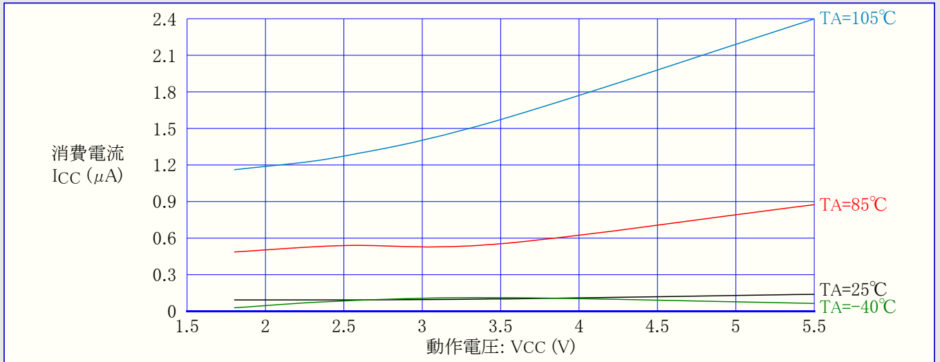
図32-102. ATmega168PA:パワーダウン動作消費電流 対 動作電圧 (ウォッチドッグ タイマ禁止)
