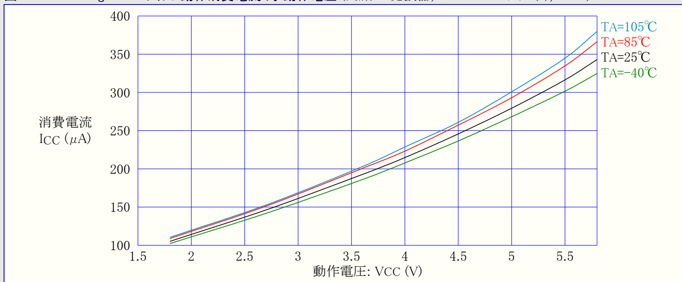
図31-340. ATmega328P: アイドル動作消費電流 対 動作電圧 (内蔵RC発振器, CKDIV8=プログラム(0), 1MHz)
