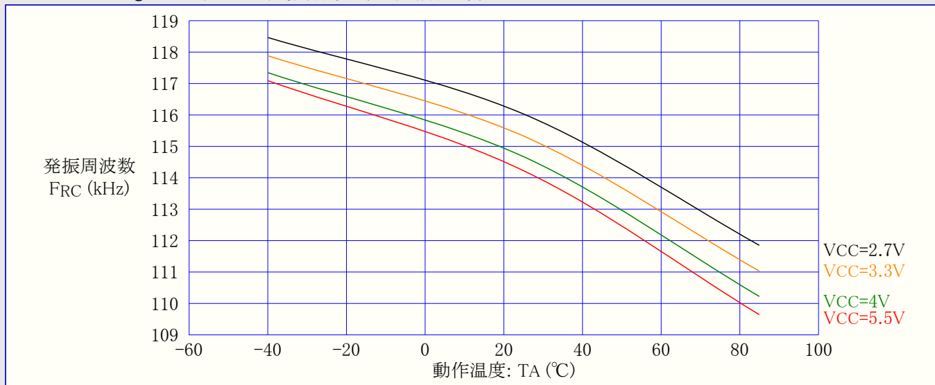
図31-319. ATmega328: ウォッチドッグ発振器周波数 対 動作温度
