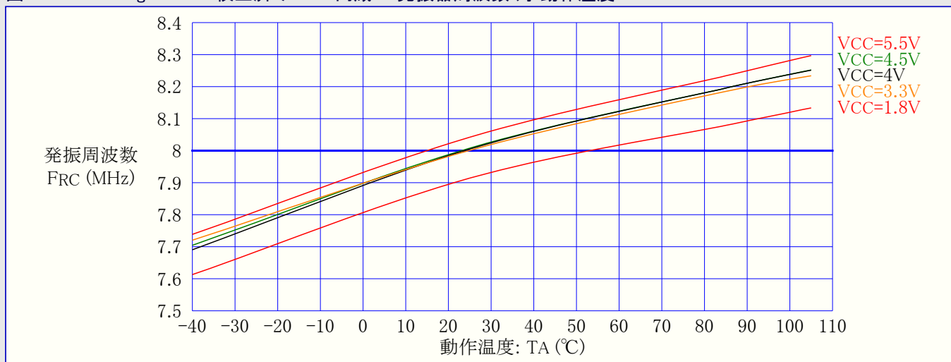
図32-130. ATmega168PA: 校正済み8MHz内蔵RC発振器周波数 対 動作温度
