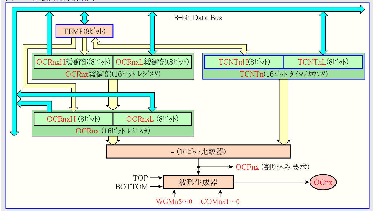
図16-4. 比較出力部構成図
