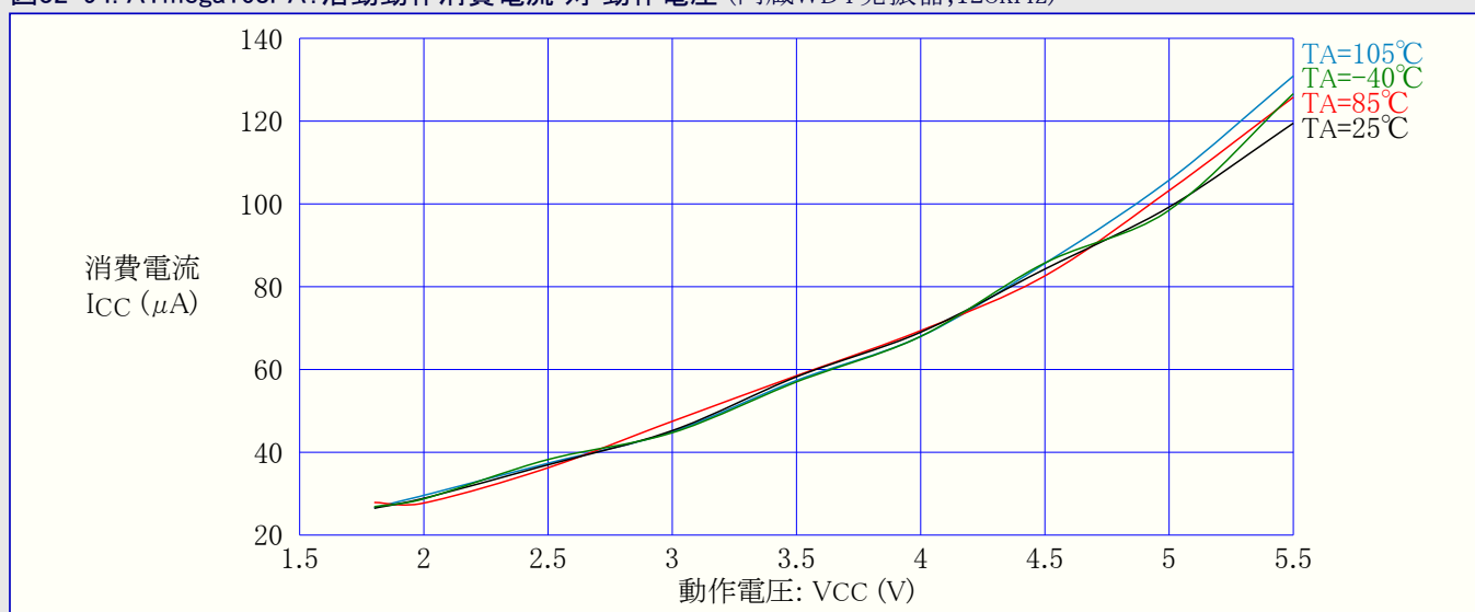
図32-94. ATmega168PA: 活動動作消費電流 対 動作電圧 (内蔵WDT発振器, 128kHz)
