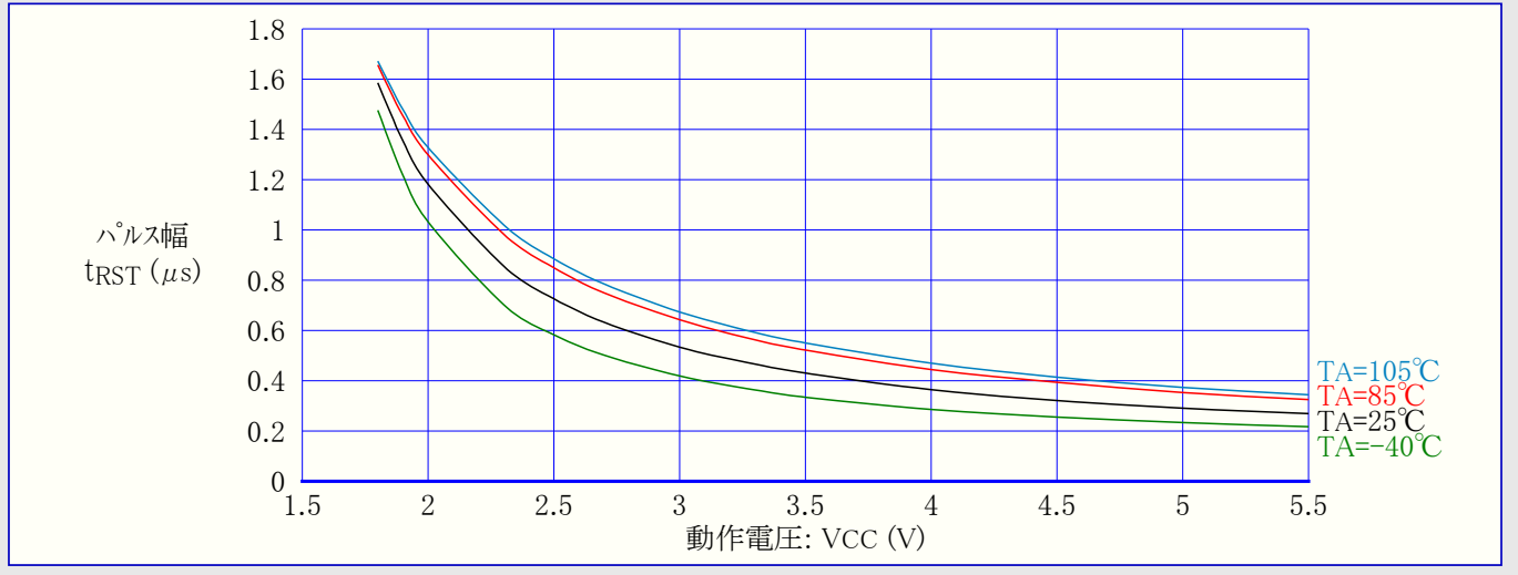
図31-378. ATmega328P: 最小リセットパルス幅 対 動作電圧
