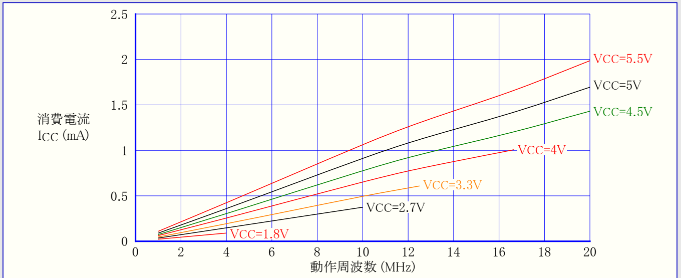
図32-90. ATmega88PA: リセット消費(供給)電流 対 周波数 (1MHz~20MHz)
