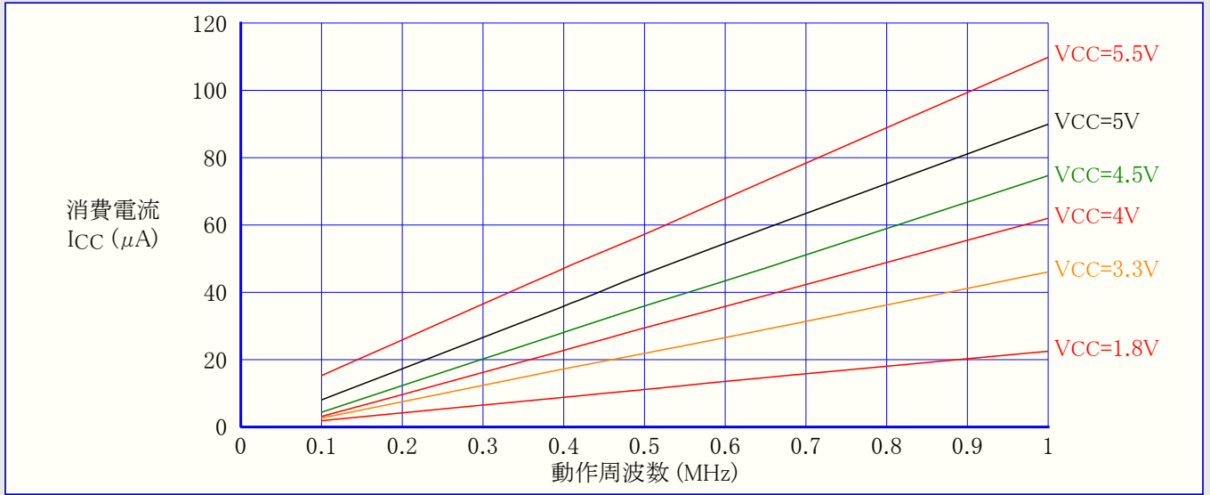
図32-89. ATmega88PA: リセット消費(供給)電流 対 周波数 (100kHz~1MHz)
