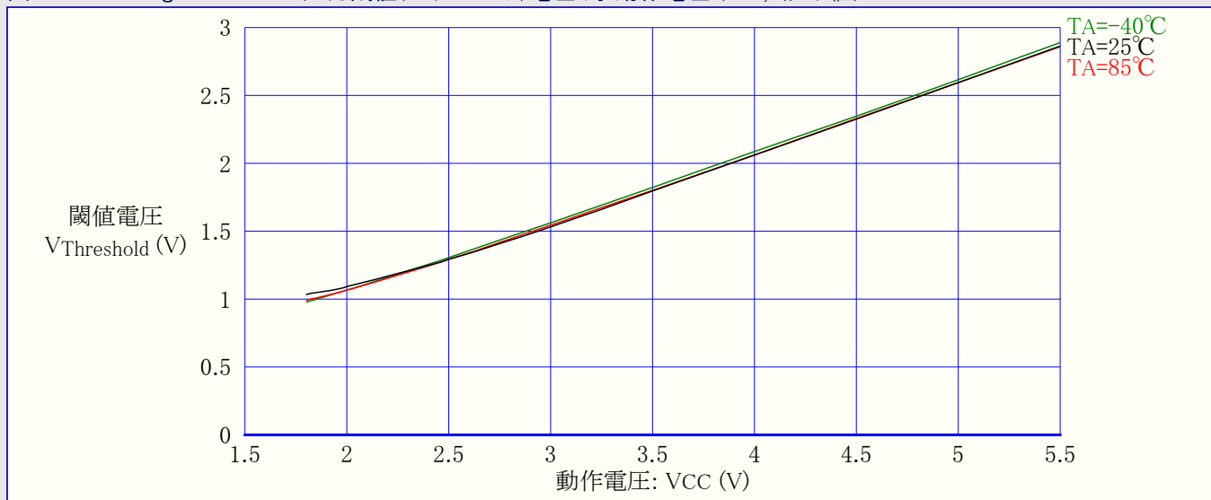
図31-25. ATmega48A:I/Oピン入力閾値(スレッシュホールド)電圧 対 動作電圧 ( V_{IH,1} 読み値)
