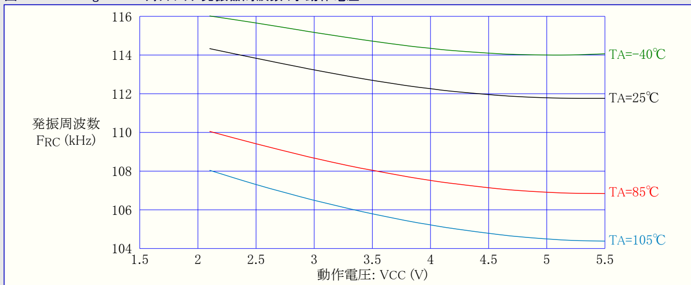
図32-35. ATmega48PA: ウォッチドッグ発振器周波数 対 動作電圧
