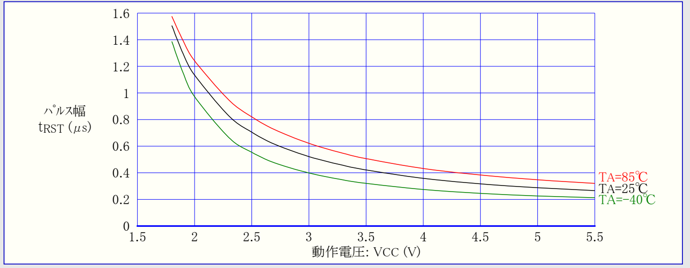
図31-141. ATmega88A: 最小リセットパルス幅 対 動作電圧
