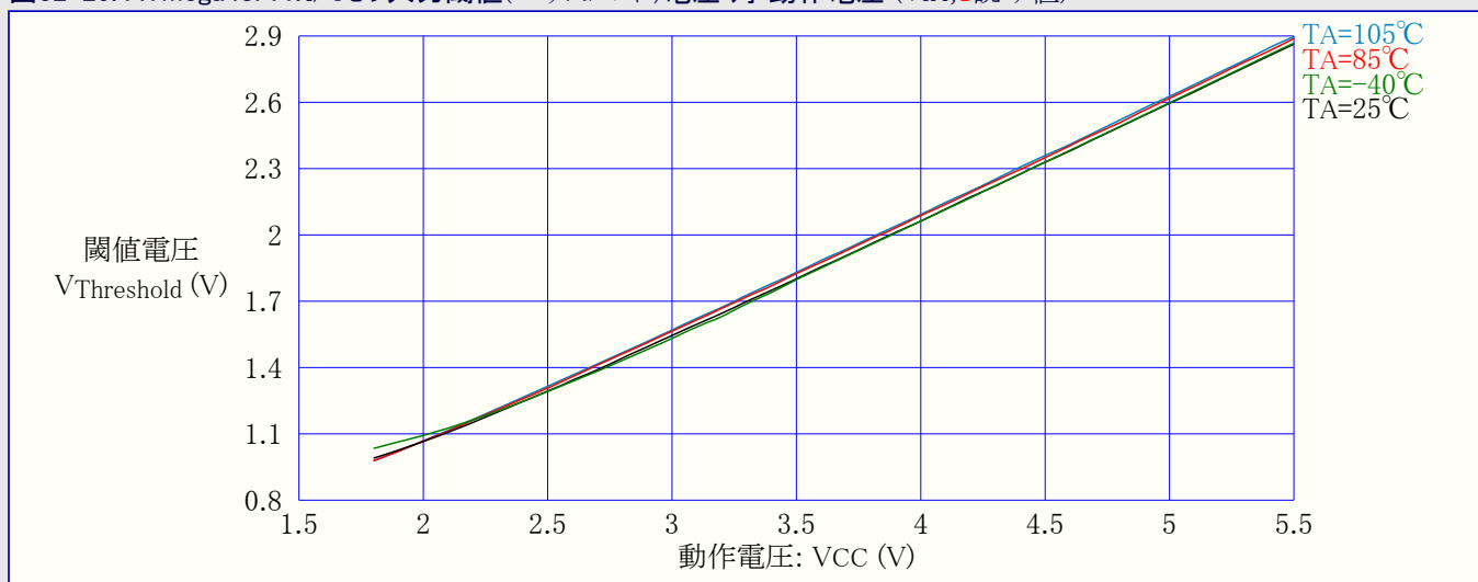
図32-26. ATmega48PA:I/Oピン入力閾値(スレッショルド)電圧 対 動作電圧 (VIL,0読み値)
