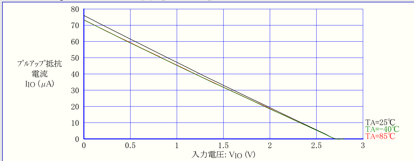
図31-205. ATmega168A:I/Oピンプルアップ抵抗電流 対 入力電圧 (VCC=2.7V)
