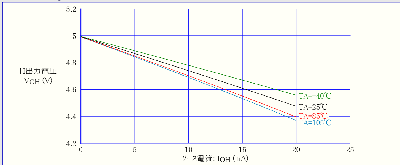
図31-165. ATmega88PA:I/Oピン出力電圧 対 ソース電流 (VCC=5V)
