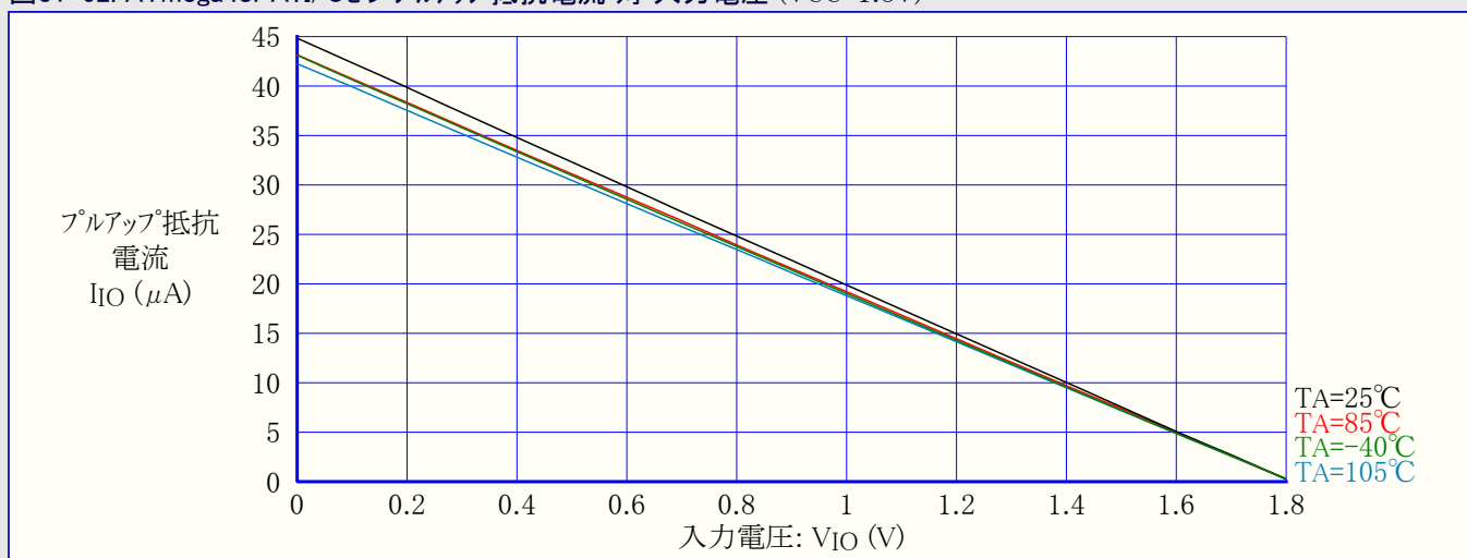
図31-62. ATmega48PA:I/Oピンプルアップ抵抗電流 対 入力電圧 ( V_{CC}=1.8V )
