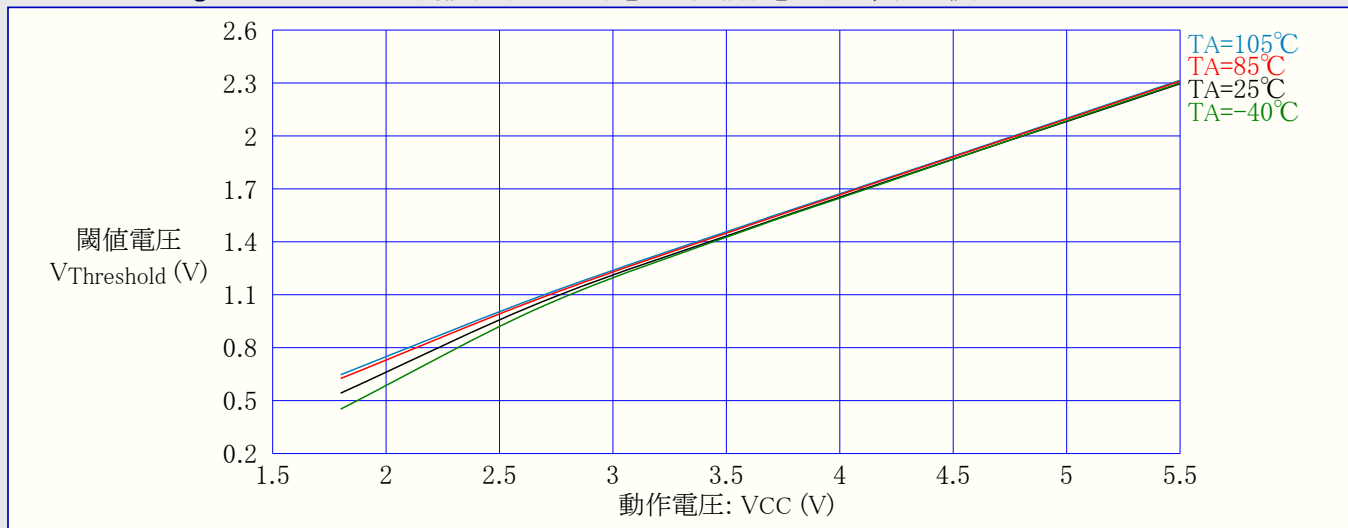
図31-357. ATmega328P:I/Oピン入力閾値(スレッショールド)電圧 対 動作電圧 (VIL,0読み値)
