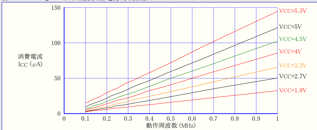
図31-329. ATmega328:リセット消費(供給)電流 対 周波数 (100kHz~1MHz)
