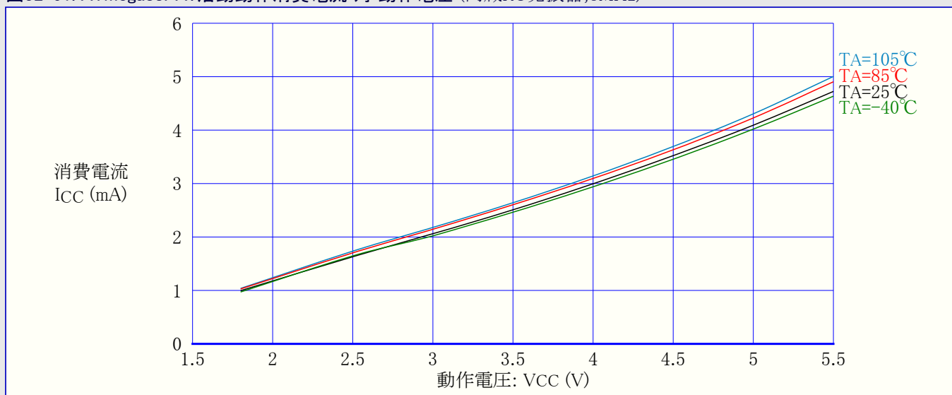
図32-51. ATmega88PA: 活動動作消費電流 対 動作電圧 (内蔵RC発振器, 8MHz)
