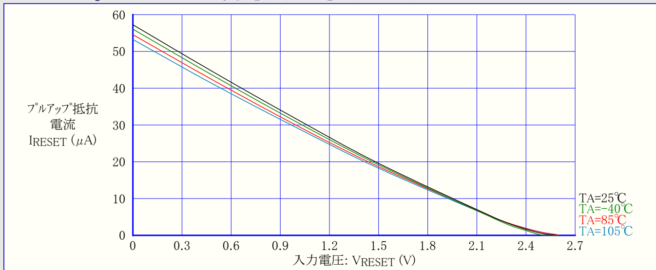
図32-158. ATmega328P: RESETプルアップ抵抗電流 対 入力電圧 (VCC=2.7V)
