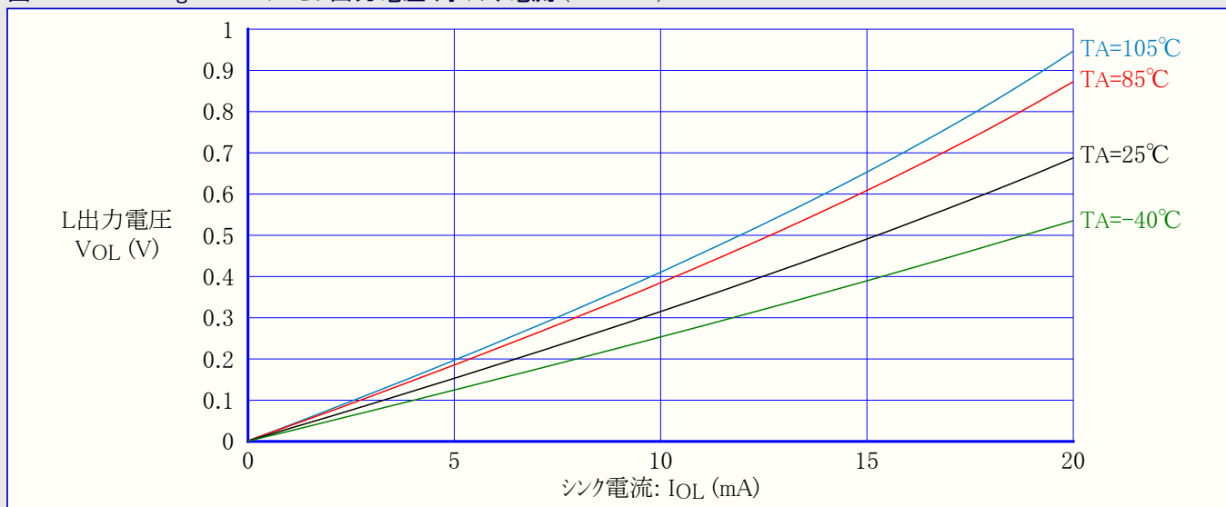
図31-352. ATmega328P: I/Oピン出力電圧 対 シンク電流 (VCC=3V)
