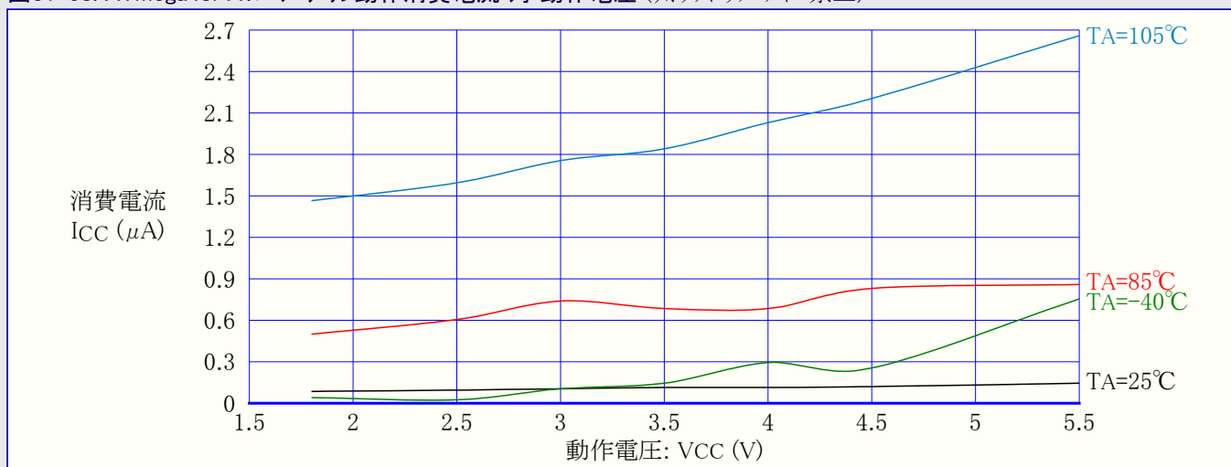
図31-58. ATmega48PA: パワーダウン動作消費電流 対 動作電圧 (ウォッチドッグ タイマ禁止)
