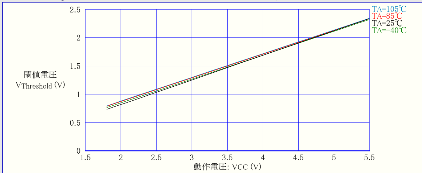
図31-170. ATmega88PA: RESET入力閾値(スレッショルド)電圧 対 動作電圧 (VIL,0読み値)
