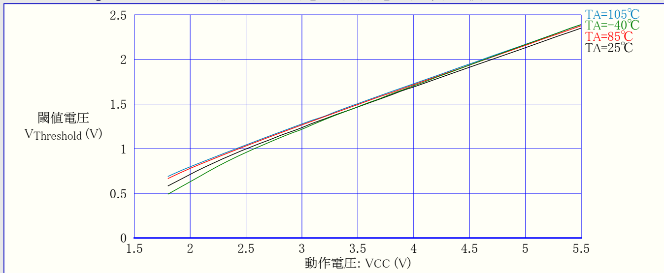
図31-167. ATmega88PA:I/Oピン入力閾値(スレッシュホールド)電圧 対 動作電圧 (VIL,0読み値)
