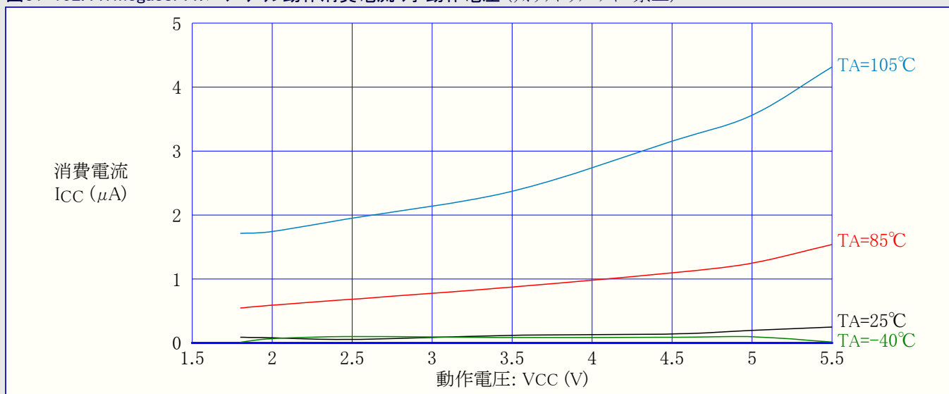
図31-152. ATmega88PA: パワーダウン動作消費電流 対 動作電圧 (ウォッチドッグ タイマ禁止)
