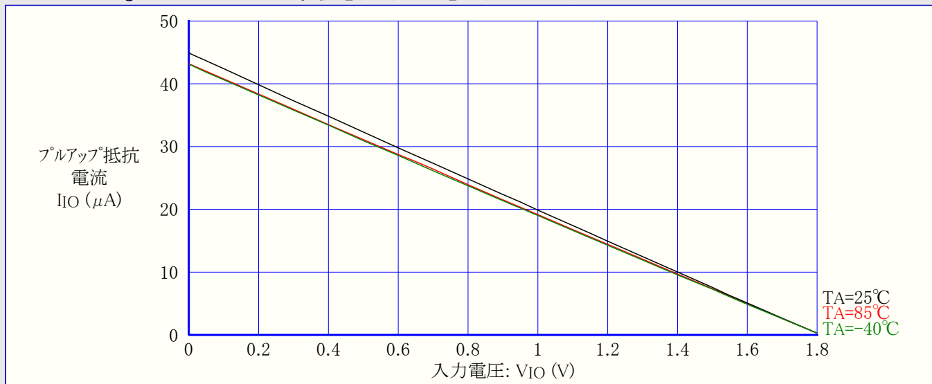
図31-15. ATmega48A:I/Oピンプルアップ抵抗電流 対 入力電圧 ( V_{CC}=1.8V )
