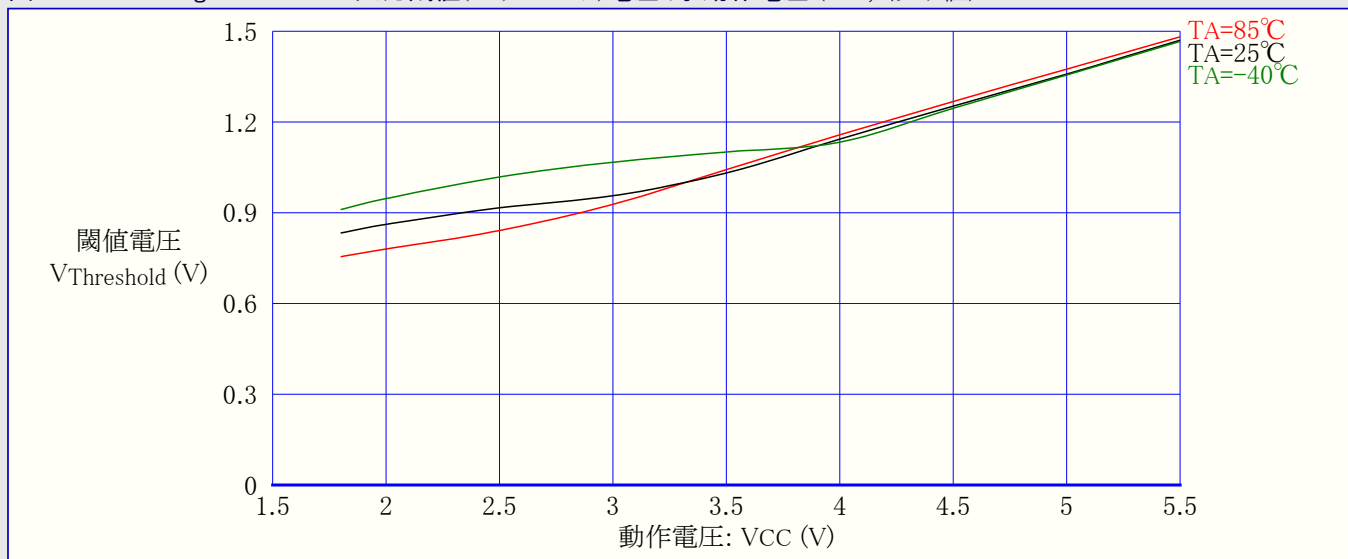
図31-122. ATmega88A:RESET入力閾値(スレッショルド)電圧 対 動作電圧 (VIH,1読み値)
