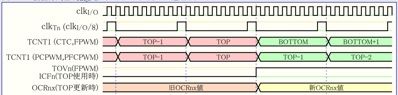
図16-13. 前置分周器( f_{clk_{I/O}/8} )のタイマ/カウンタ、TOP近辺 タイミング
