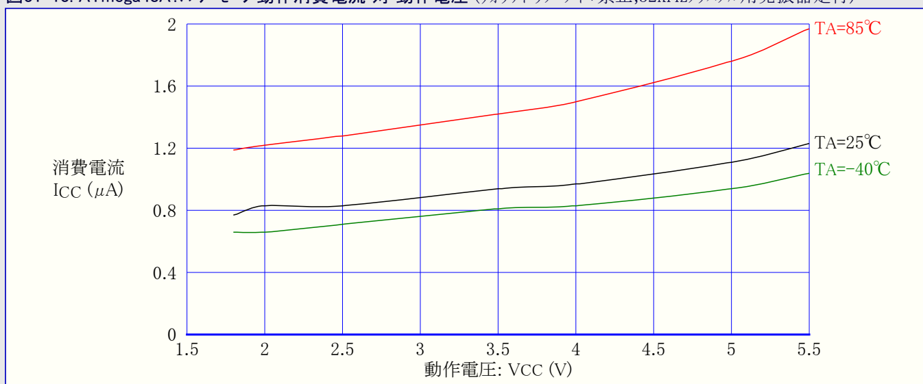
図31-13. ATmega48A: パワーセーブ動作消費電流 対 動作電圧 (ウォッチドッグ タイマ禁止, 32kHzクリスタル用発振器走行)
