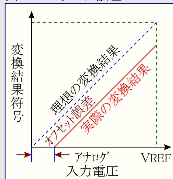
図24-10. オフセット誤差
