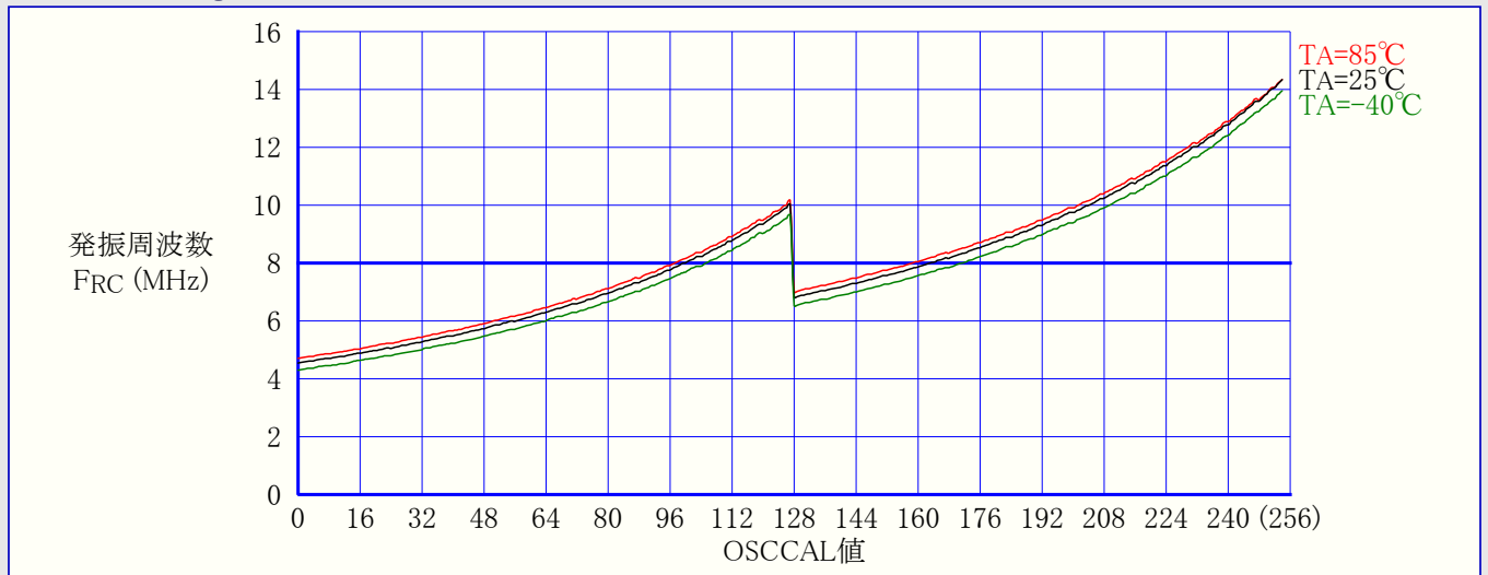
図31-228. ATmega168A: 校正付き8MHz内蔵RC発振器周波数 対 発振校正(OSCCAL)値
