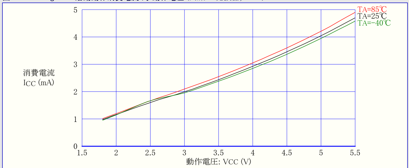
図31-5. ATmega48A: 活動動作消費電流 対 動作電圧 (内蔵RC発振器, 8MHz)
