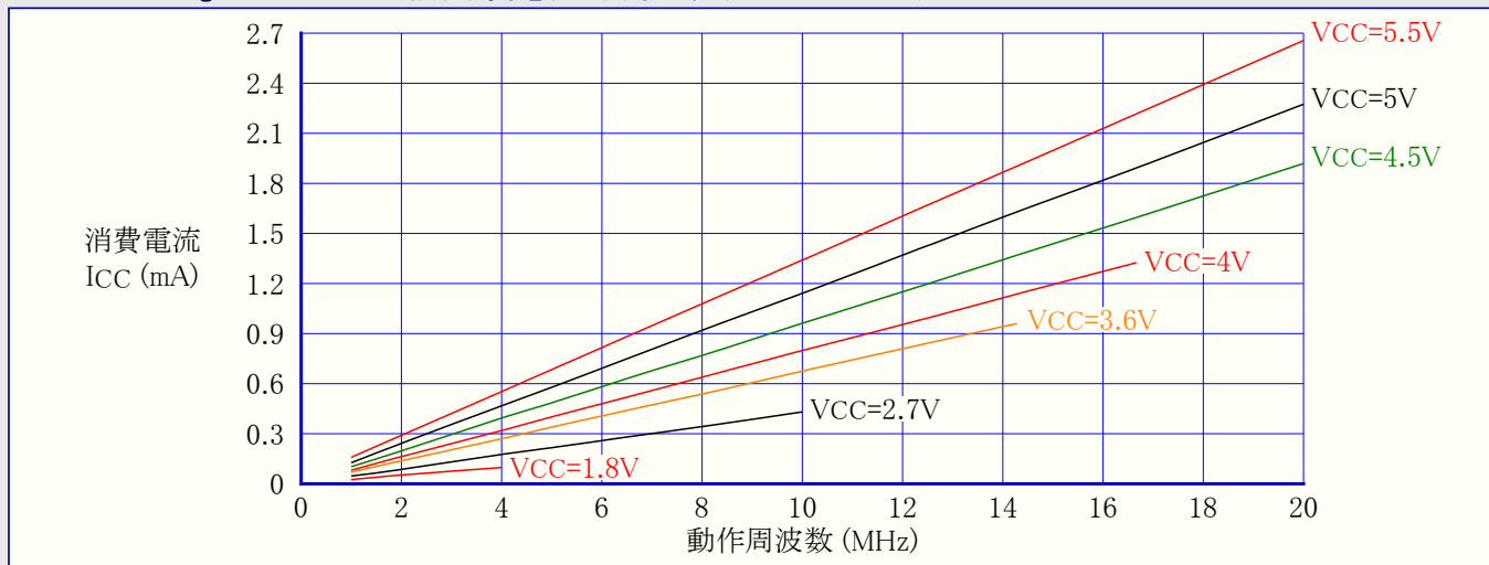
図32-98. ATmega168PA: アイドル動作消費電流 対 周波数 (1MHz~20MHz)
