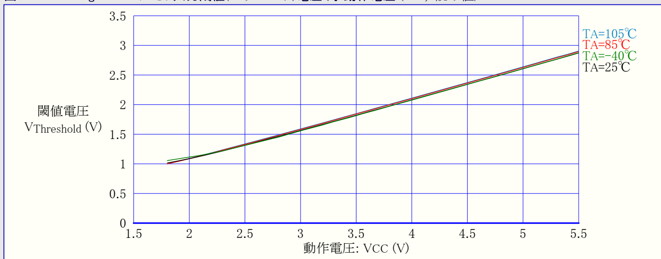
図32-70. ATmega88PA:I/Oピン入力閾値(スレッショルド)電圧 対 動作電圧 (VIH, 1読み値)
