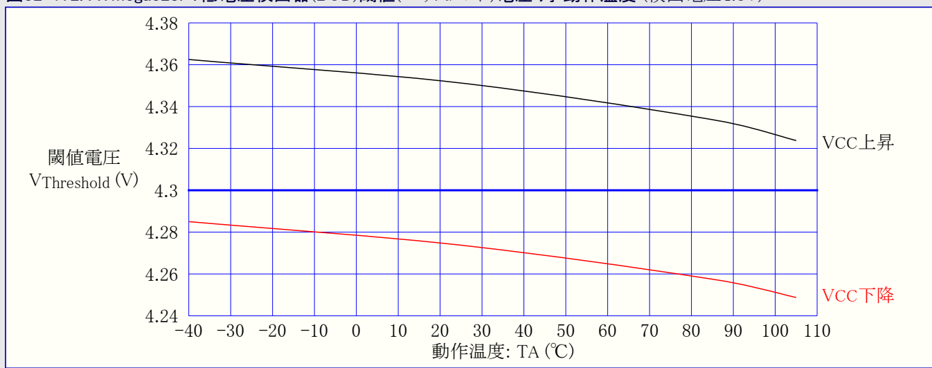
図32-172. ATmega328P: 低電圧検出器(BOD)閾値(スレッシュホールド)電圧 対 動作温度 (検出電圧4.3V)
