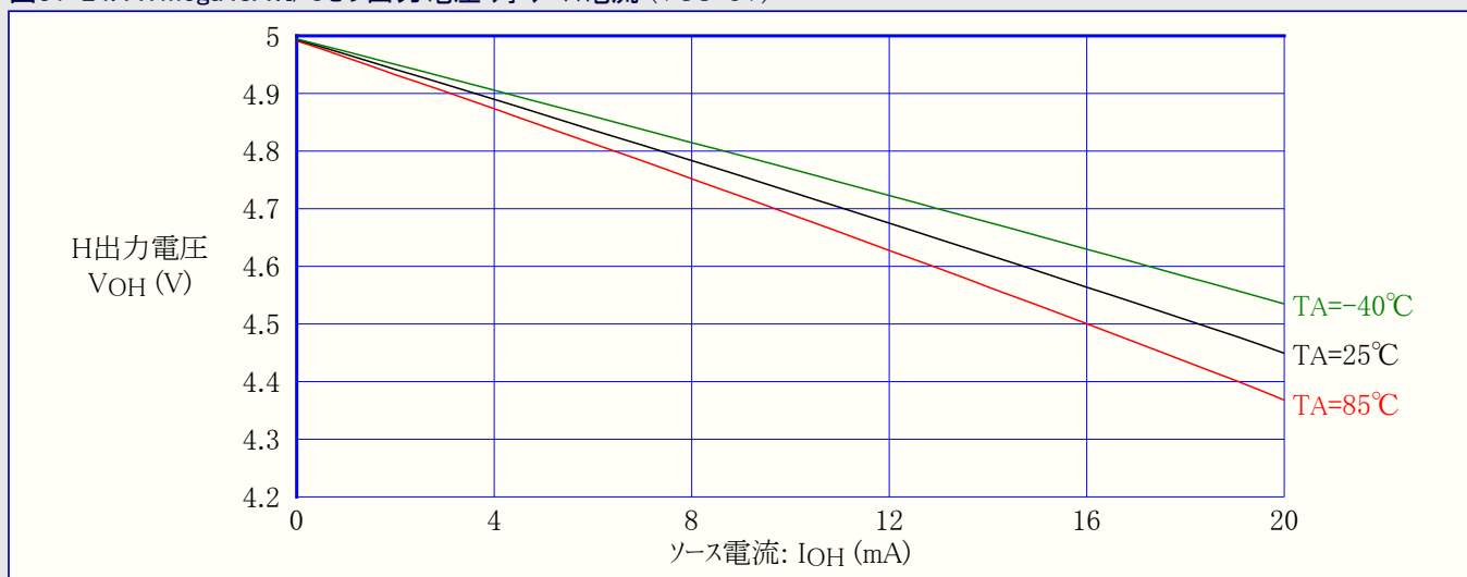
図31-24. ATmega48A:I/Oピン出力電圧 対 ソース電流 (VCC=5V)
