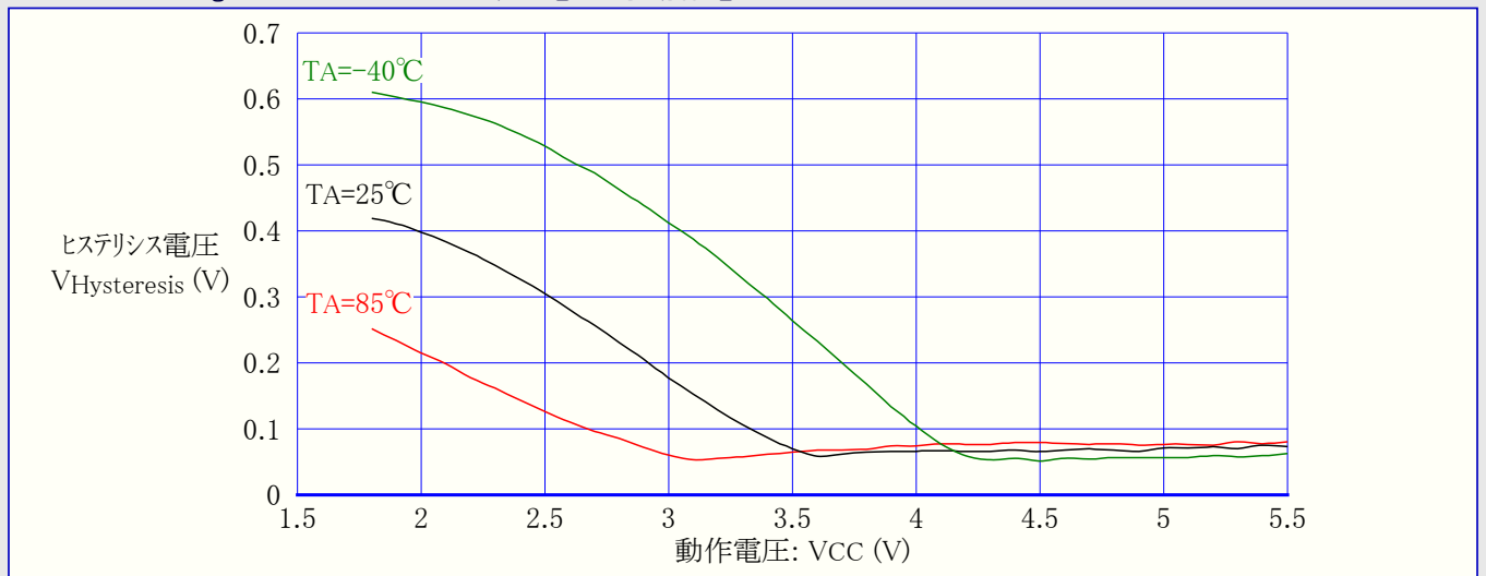
図31-314. ATmega328: RESET入力ヒステリシス電圧 対 動作電圧
