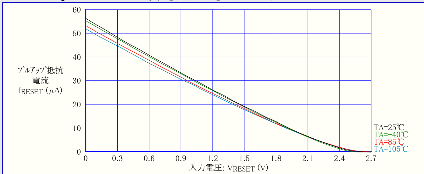
図31-255. ATmega168PA:RESETプルアップ抵抗電流 対 入力電圧 (VCC=2.7V)
