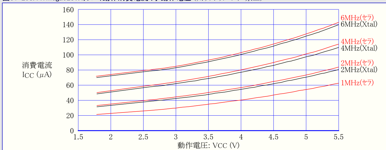
図31-298. ATmega328:スタンバイ動作消費電流 対 動作電圧 (ウォッチドッグ タイマ禁止)
