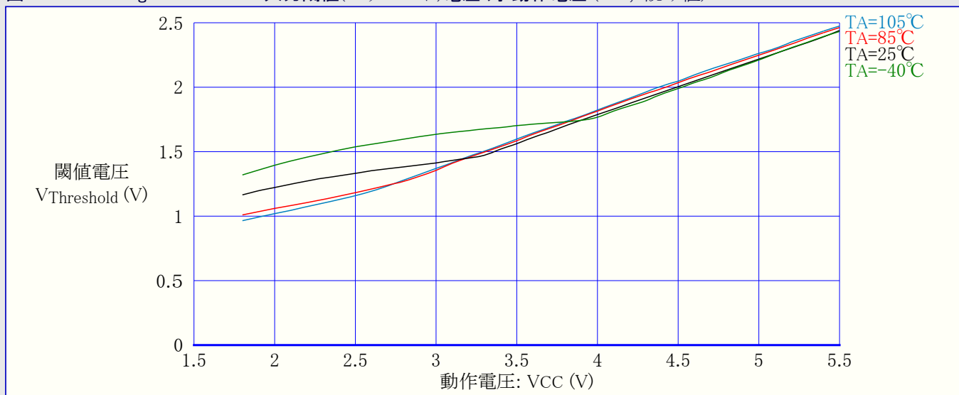
図31-169. ATmega88PA:RESET入力閾値(スレッシュホールド)電圧 対 動作電圧 (VIH,1読み値)
