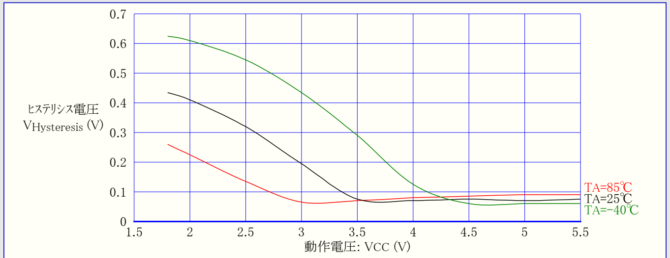
図31-219. ATmega168A: RESET入力ヒステリシス電圧 対 動作電圧
