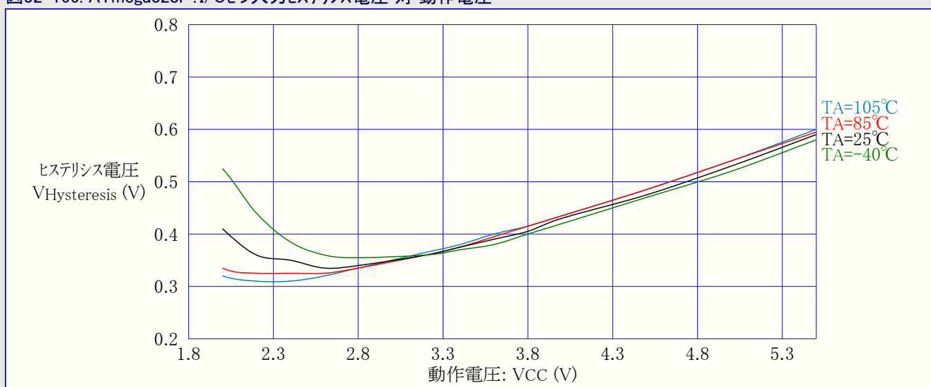
図32-166. ATmega328P:I/Oピン入力ヒステリシス電圧 対 動作電圧
