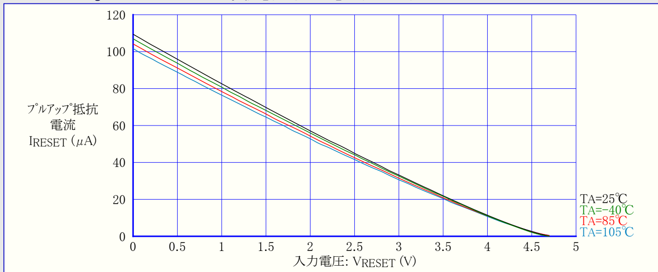
図32-111. ATmega168PA: RESETプルアップ抵抗電流 対 入力電圧 (VCC=5V)
