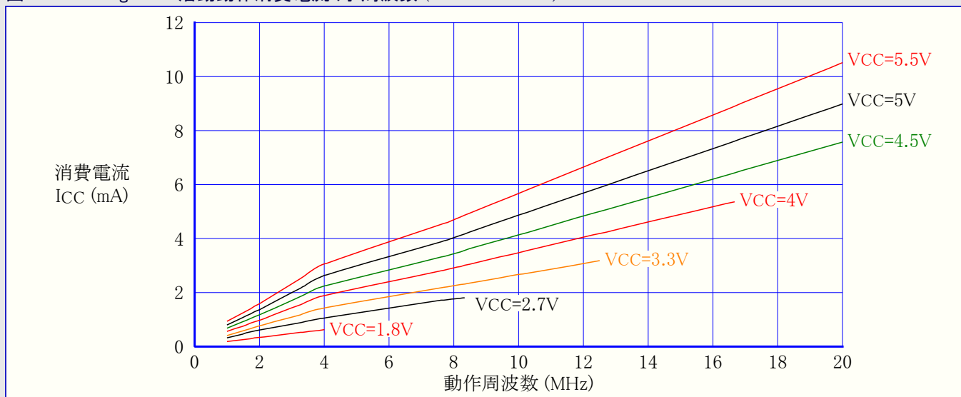
図31-2. ATmega48A: 活動動作消費電流 対 周波数 (1MHz~20MHz)
