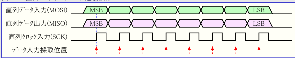
図28-9. 直列プログラミングバイト通信波形
