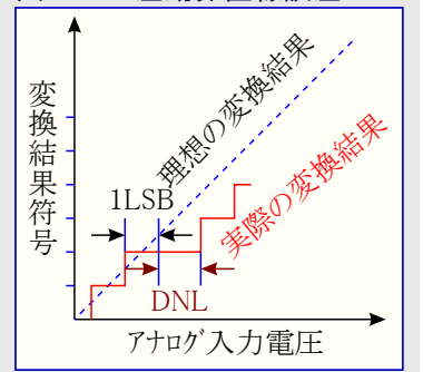
図24-13. 差動非直線誤差
