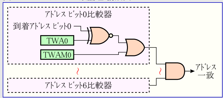
図22-22. TWIアドレス一致論理 構成図
