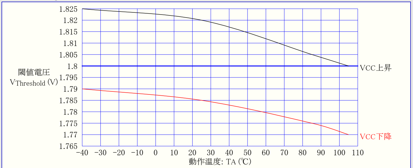
図32-31. ATmega48PA: 低電圧検出器(BOD)閾値(スレッショルド)電圧 対 動作温度 (検出電圧1.8V)
