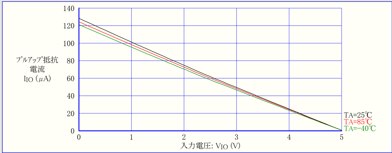
図31-17. ATmega48A: I/Oピンプルアップ抵抗電流 対 入力電圧 (VCC=5V)
