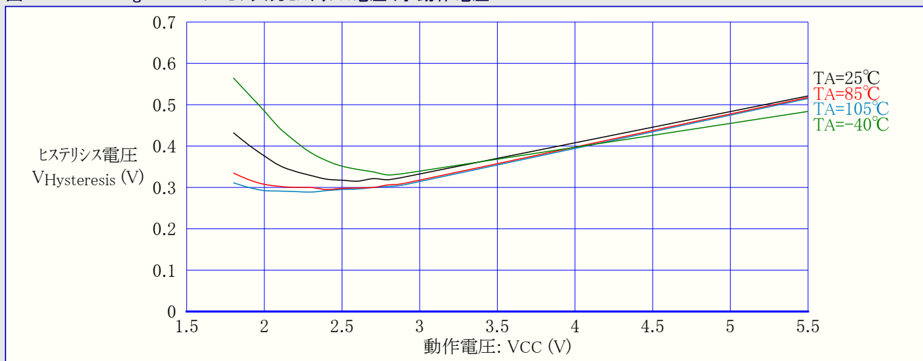
図31-168. ATmega88PA:I/Oピン入力ヒステリシス電圧 対 動作電圧
