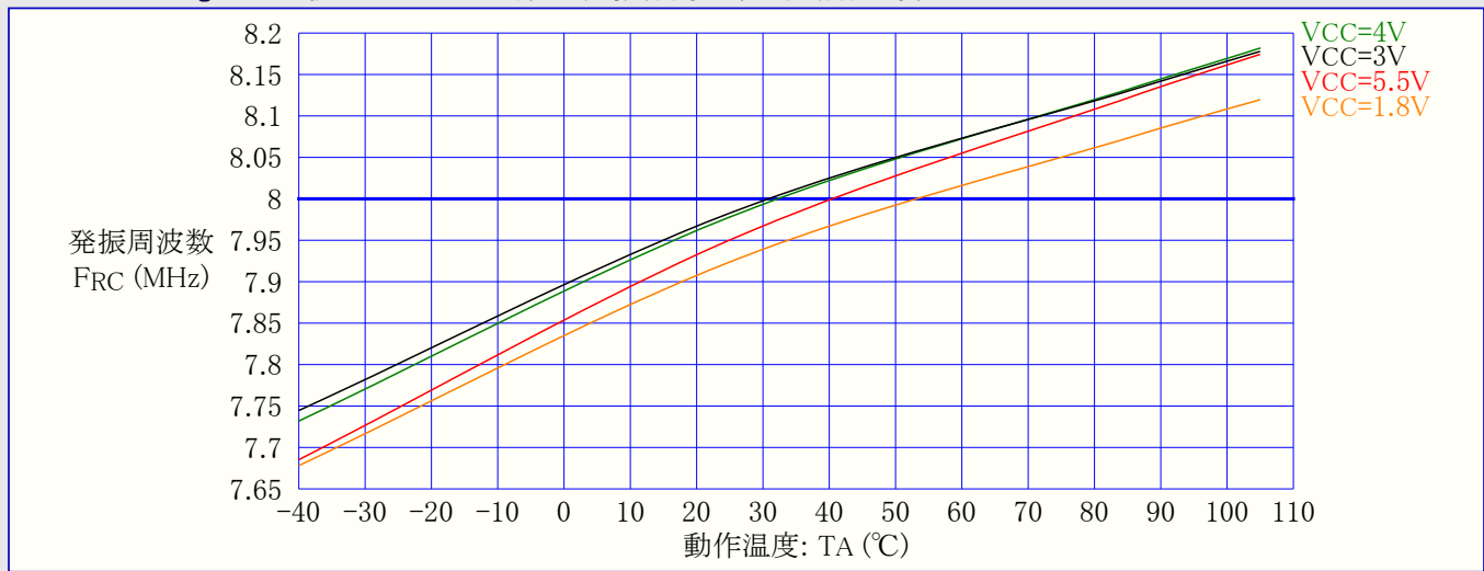
図32-37. ATmega48PA: 校正付き8MHz内蔵RC発振器周波数 対 動作温度
