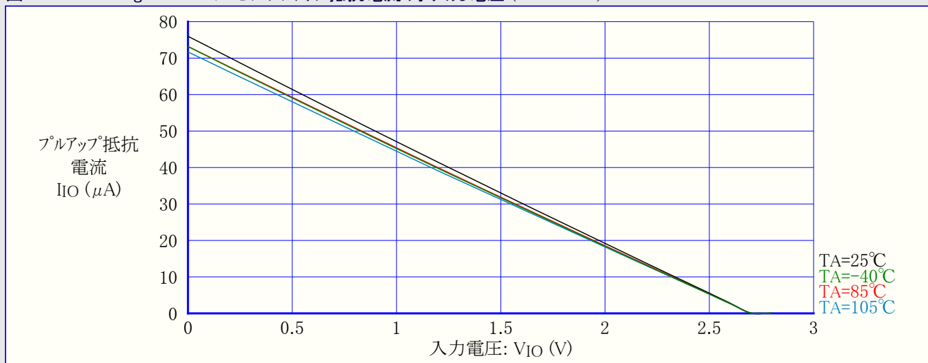
図31-252. ATmega168PA:I/Oピンプルアップ抵抗電流 対 入力電圧 ( V_{CC}=2.7V )
