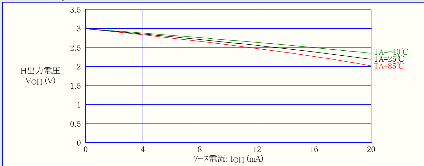
図31-212. ATmega168A:I/Oピン出力電圧 対 ソース電流 (VCC=3V)
