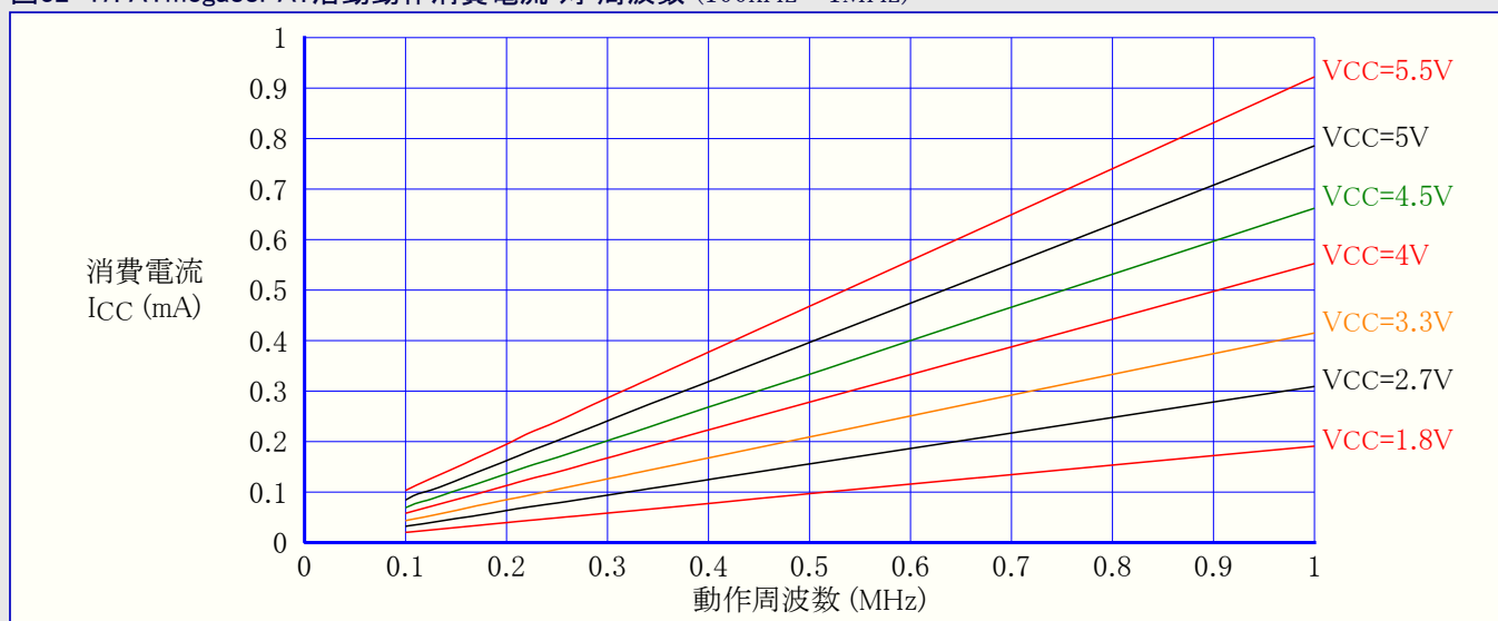
図32-47. ATmega88PA: 活動動作消費電流 対 周波数 (100kHz~1MHz)
