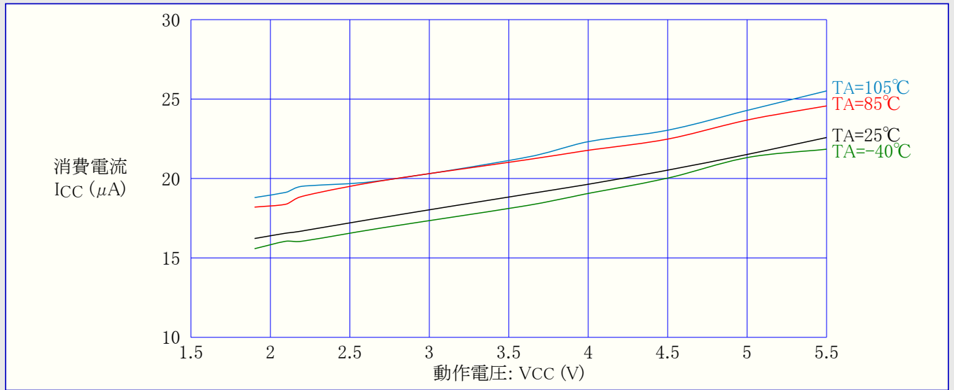
図32-182. ATmega328P: 低電圧検出器(BOD)消費電流 対 動作電圧
