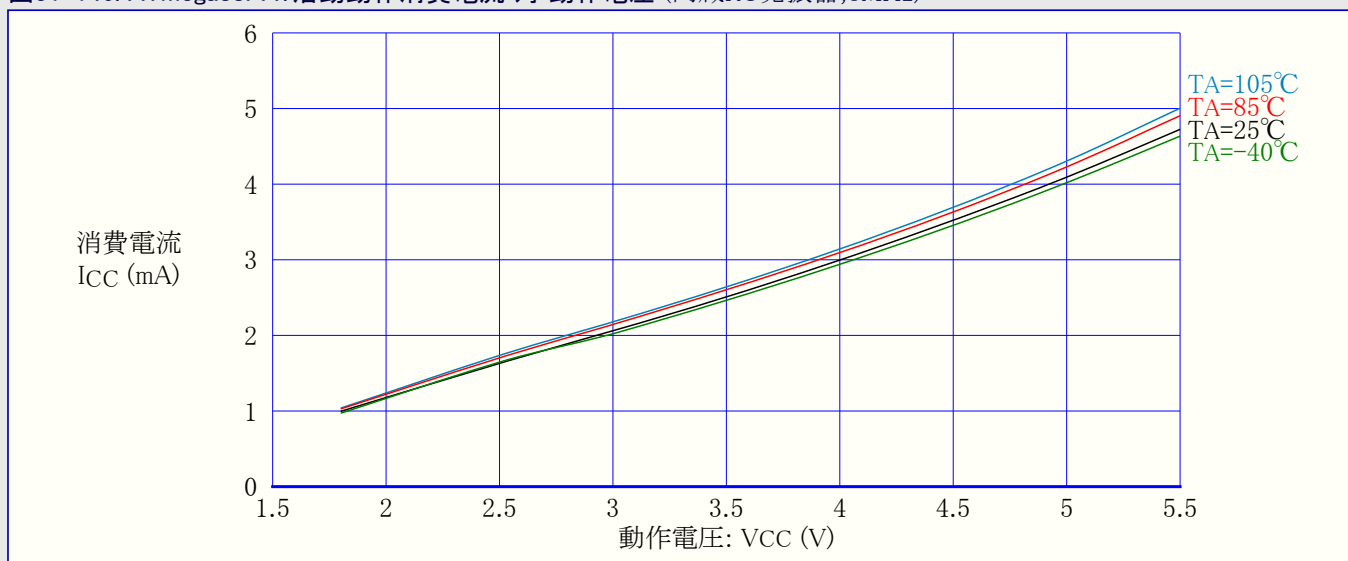
図31-146. ATmega88PA: 活動動作消費電流 対 動作電圧 (内蔵RC発振器, 8MHz)
