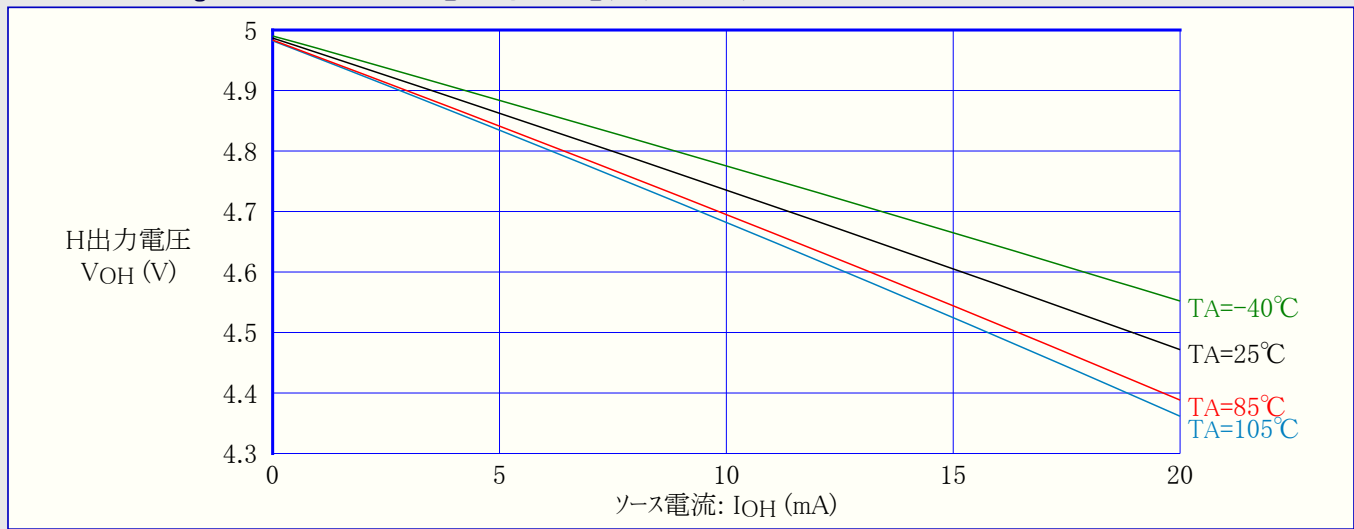
図32-115. ATmega168PA:I/Oピン出力電圧 対 ソース電流 (VCC=5V)
