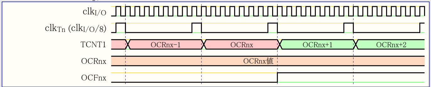
図16-11. 前置分周器( f_{clk_{I/O}/8} )のタイマ/カウンタ、 OCF1x 設定 タイミング
