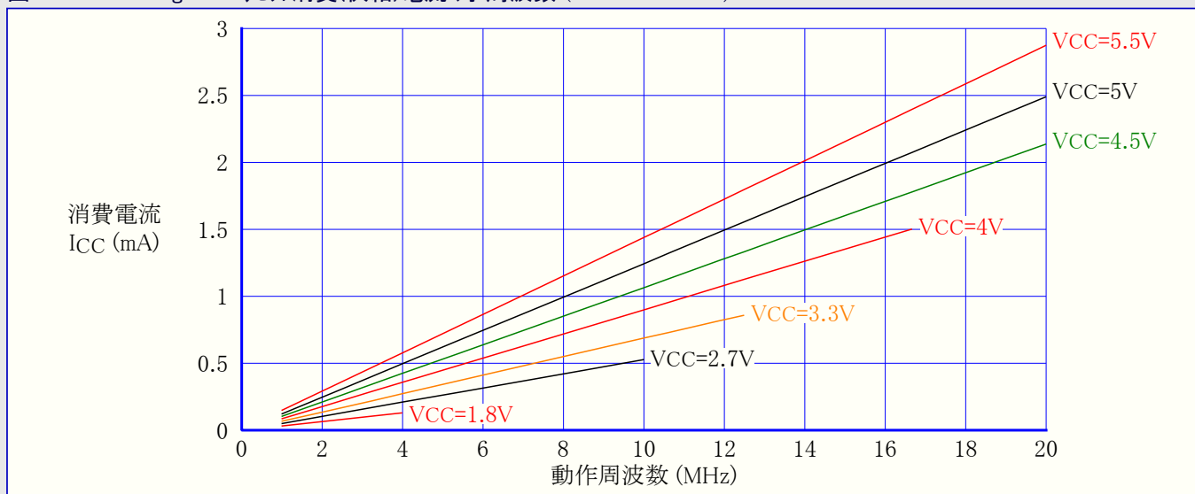
図31-330. ATmega328:リセット消費(供給)電流 対 周波数 (1MHz~20MHz)
