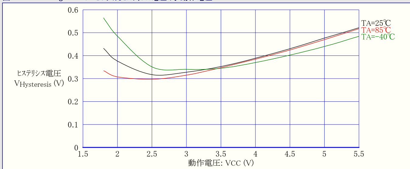
図31-121. ATmega88A:I/Oピン入力ヒステリシス電圧 対 動作電圧
