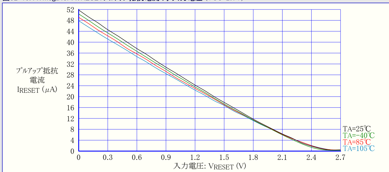
図32-19. ATmega48PA: RESETプルアップ抵抗電流 対 入力電圧 (VCC=2.7V)
