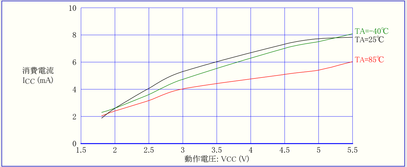
図31-233. ATmega168A:プログラミング電流 対 動作電圧
