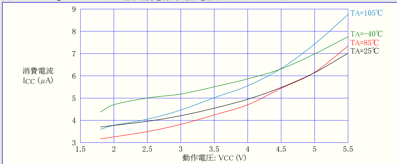
図31-248. ATmega168PA: パワーダウン動作消費電流 対 動作電圧 (ウォッチドッグ タイマ許可)
