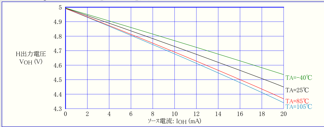
図32-24. ATmega48PA:I/Oピン出力電圧 対 ソース電流 (VCC=5V)
