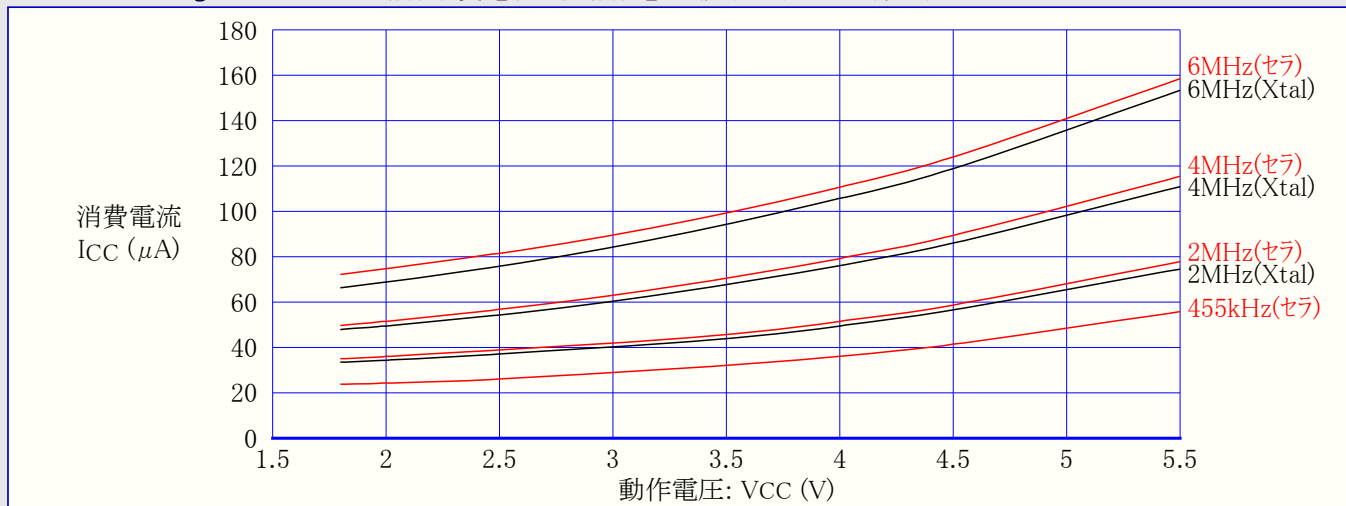
図31-155. ATmega88PA:スタンバイ動作消費電流 対 動作電圧 (ウォッチドッグ タイマ禁止)
