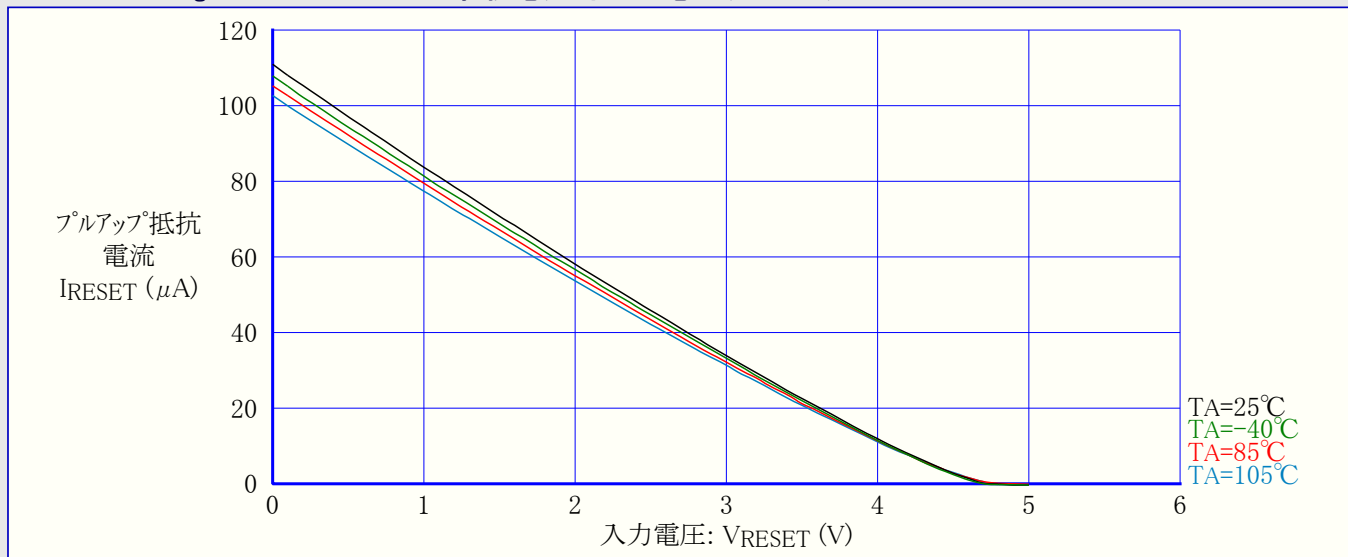
図31-161. ATmega88PA: RESETプルアップ抵抗電流 対 入力電圧 (VCC=5V)
