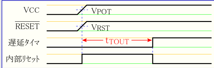
図11-2. 内蔵電源ONリセット ( \overline{RESET} はVCCに接続)
