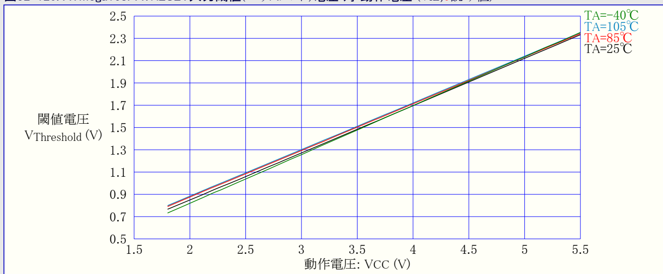
図32-120. ATmega168PA: RESET入力閾値(スレッシュホールド)電圧 対 動作電圧 (VIL,0読み値)
