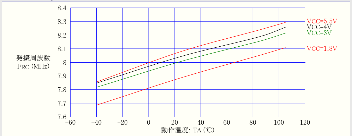
図31-180. ATmega88PA: 校正済み8MHz内蔵RC発振器周波数 対 動作温度
