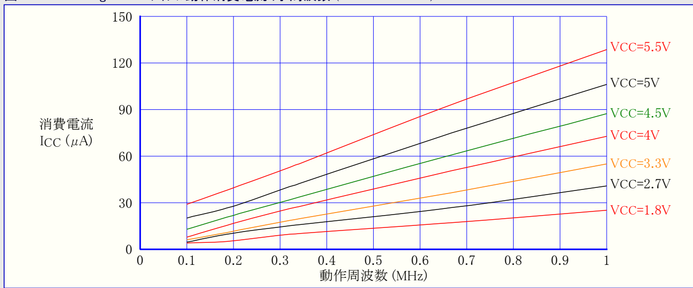
図31-147. ATmega88PA: アイドル動作消費電流 対 周波数 (100kHz~1MHz)
