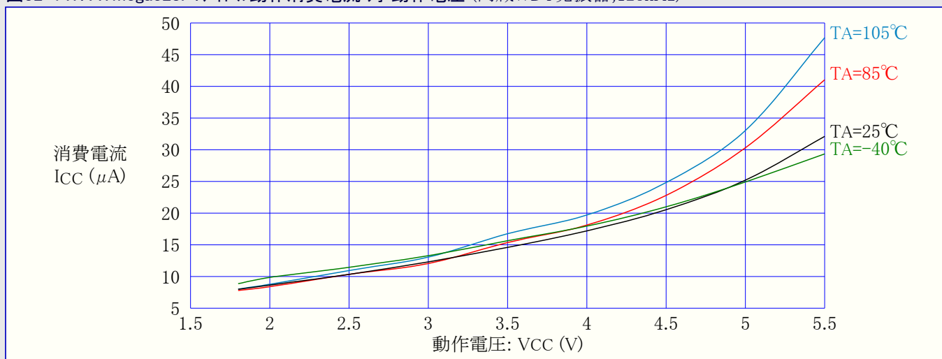
図32-147. ATmega328P: アイドル動作消費電流 対 動作電圧 (内蔵WDT発振器, 128kHz)
