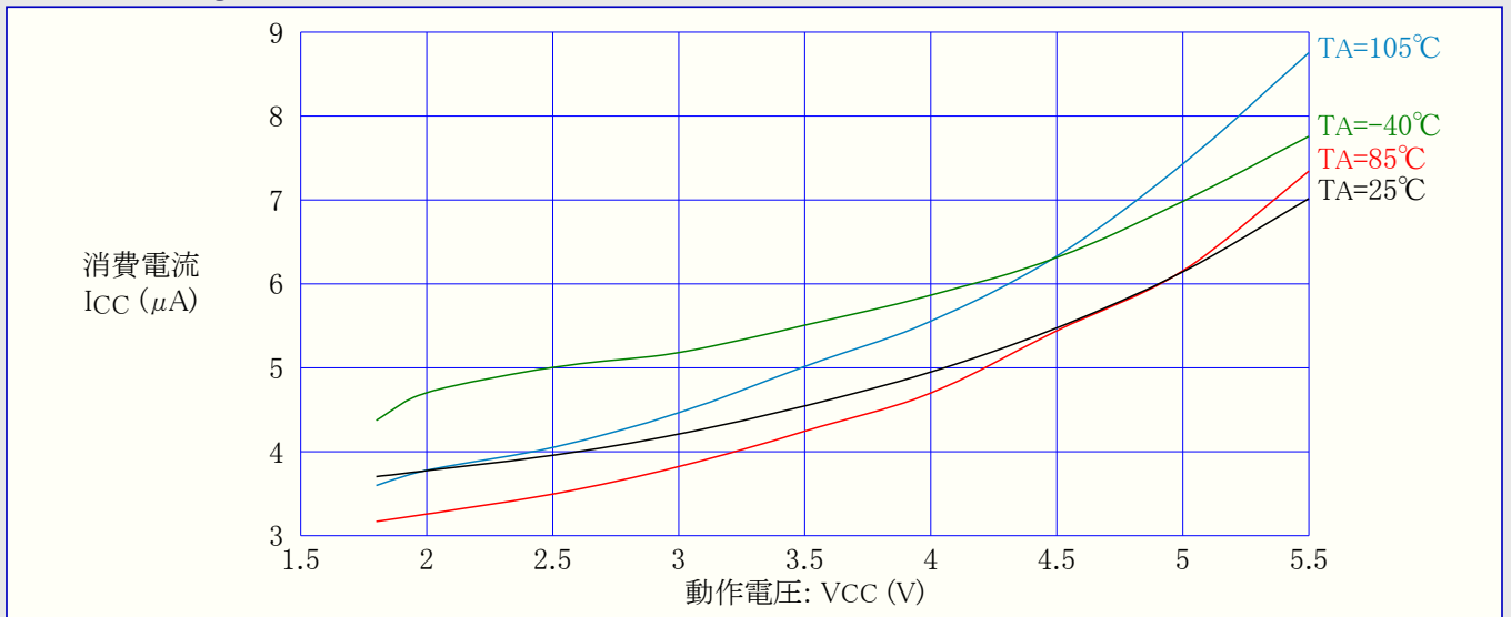
図32-103. ATmega168PA:パワーダウン動作消費電流 対 動作電圧 (ウォッチドッグ タイマ許可)
