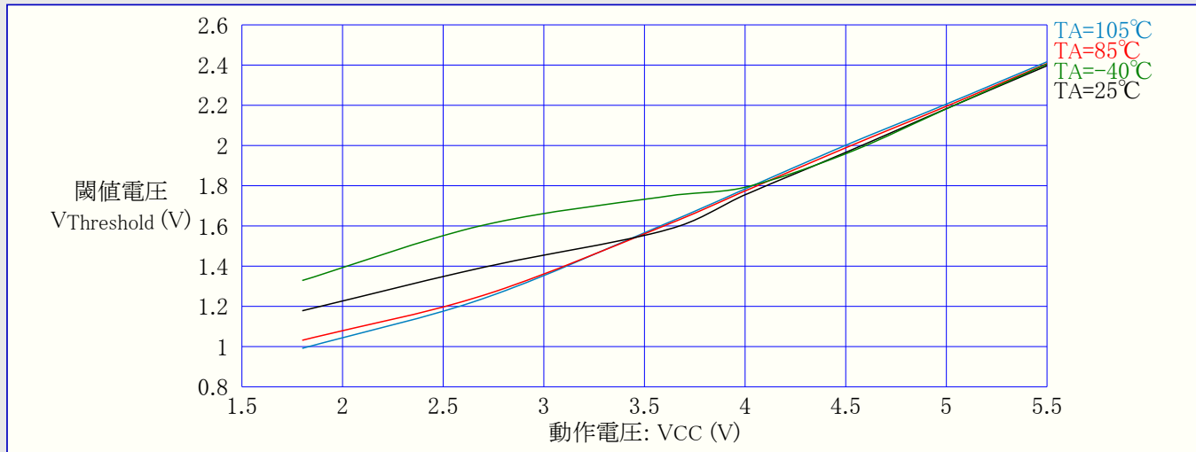
図32-167. ATmega328P: RESET入力閾値(スレッショルド)電圧 対 動作電圧 (VIH,1読み値)
