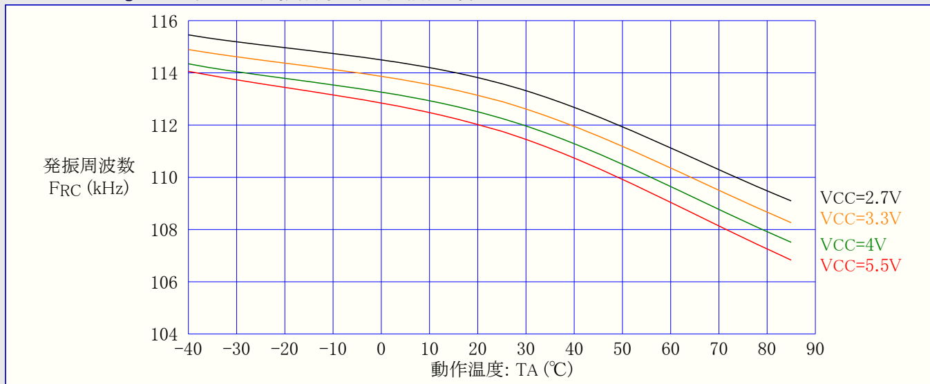
図31-35. ATmega48A: ウォッチドッグ発振器周波数 対 動作温度
