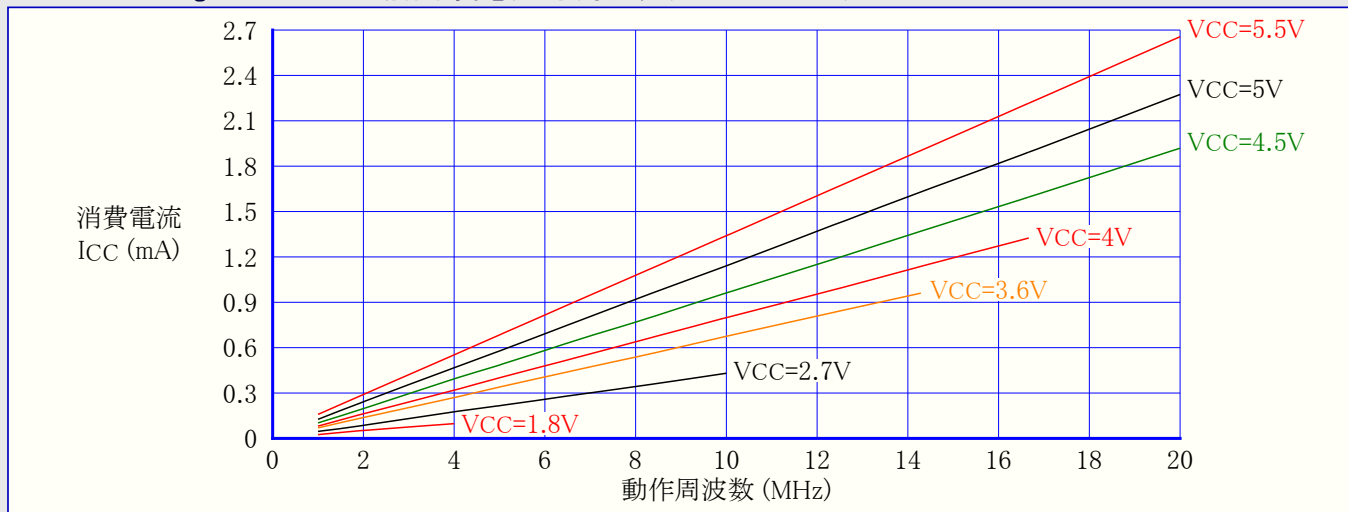
図31-243. ATmega168PA: アイドル動作消費電流 対 周波数 (1MHz~20MHz)
