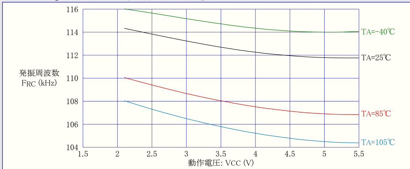
図31-83. ATmega48PA: ウォッチドッグ発振器周波数 対 動作電圧
