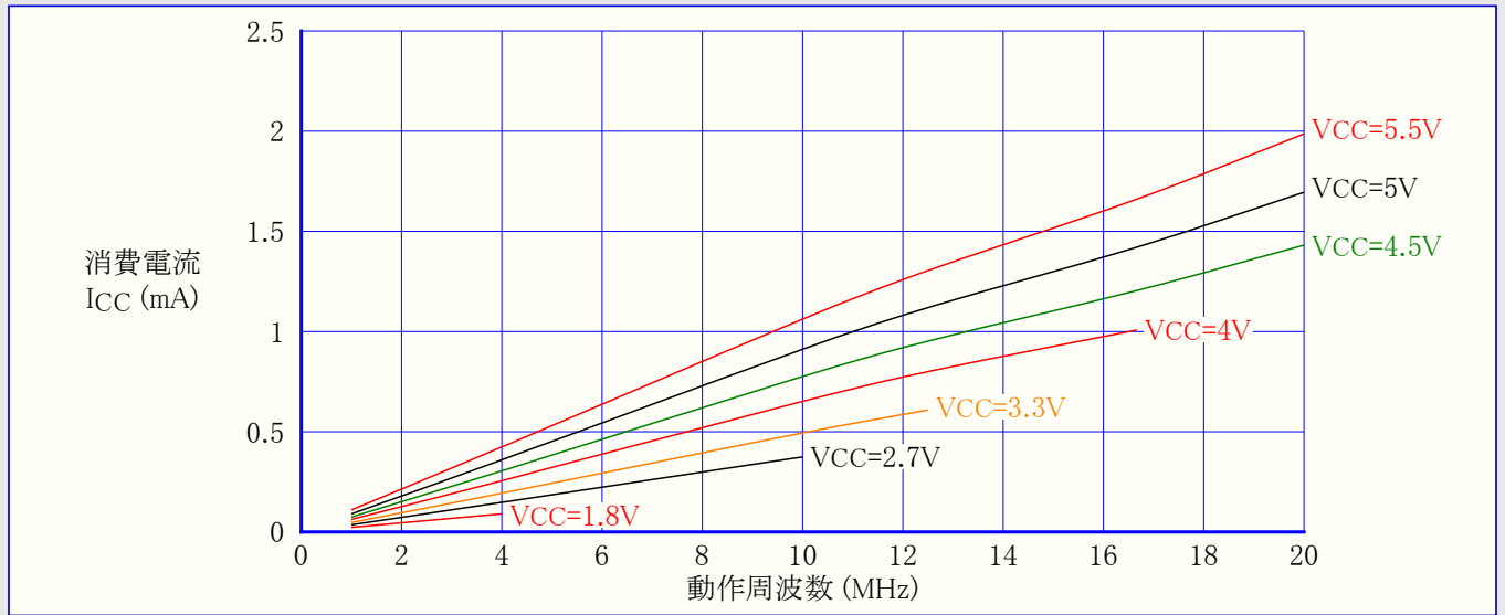
図31-188. ATmega88PA:リセット消費(供給)電流 対 周波数 (1MHz~20MHz)
