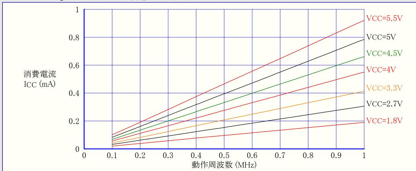
図31-190. ATmega168A: 活動動作消費電流 対 周波数 (100kHz~1MHz)
