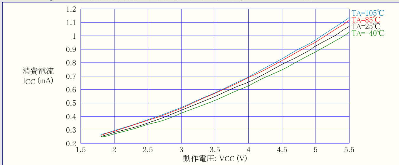
図32-4. ATmega48PA: 活動動作消費電流 対 動作電圧 (内蔵RC発振器, CKDIV8=プログラム(0), 1MHz)
