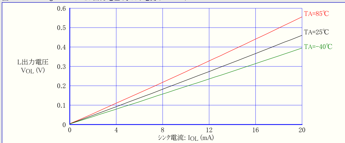
図31-211. ATmega168A:I/Oピン出力電圧 対 シンク電流 (VCC=5V)
