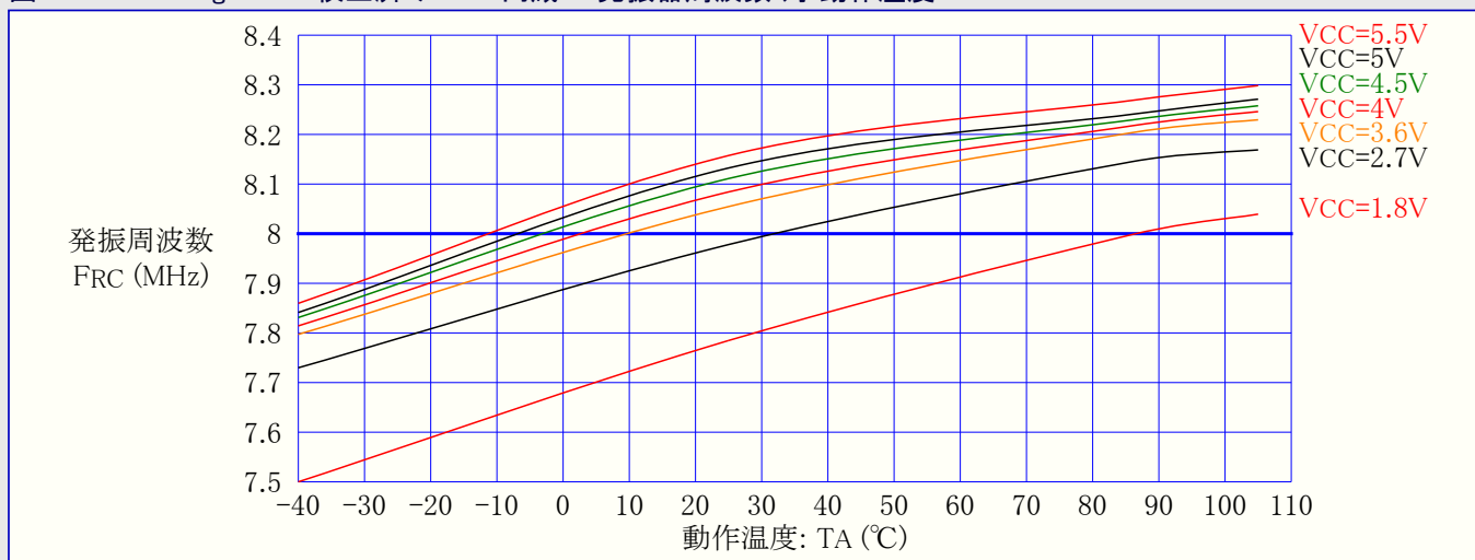
図32-177. ATmega328P: 校正済み8MHz内蔵RC発振器周波数 対 動作温度
