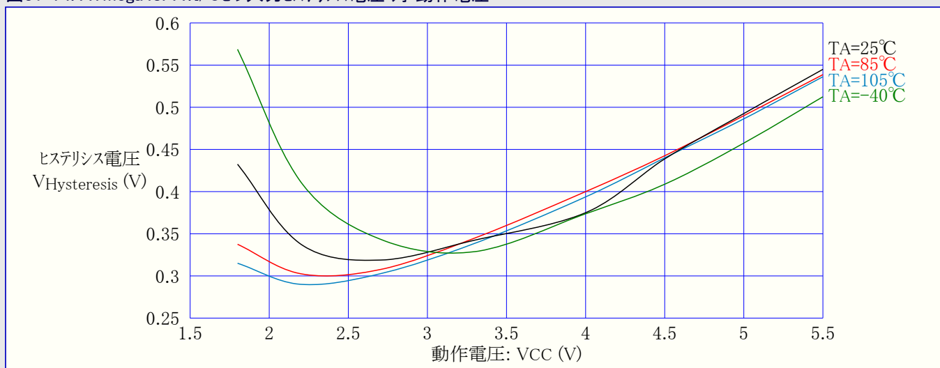
図31-74. ATmega48PA:I/Oピン入力ヒステリシス電圧 対 動作電圧
