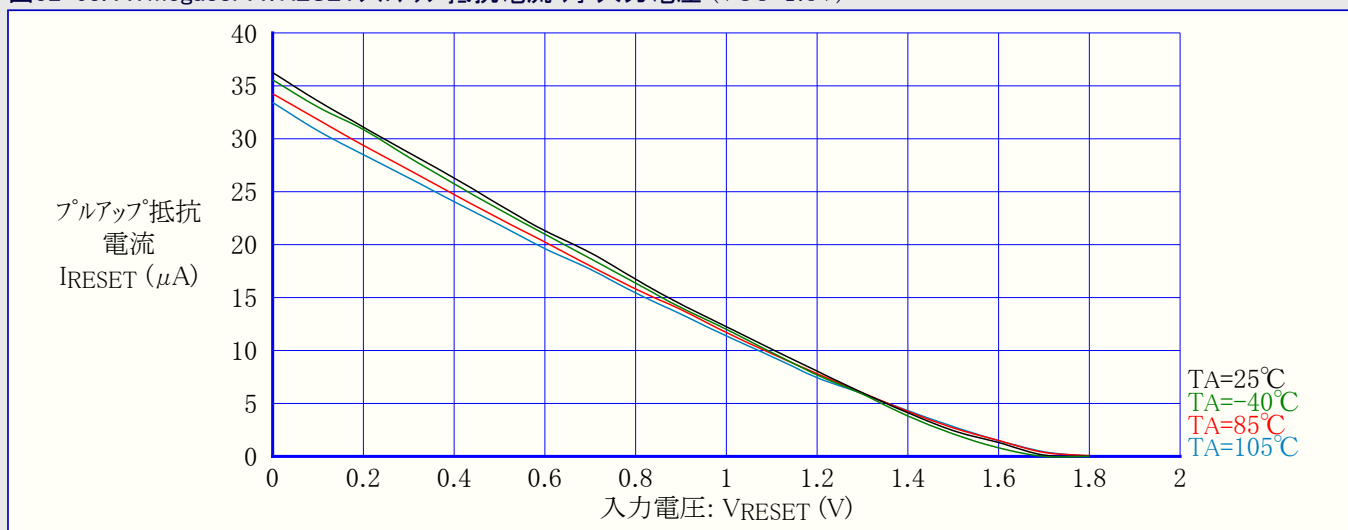
図32-63. ATmega88PA: RESETプルアップ抵抗電流 対 入力電圧 (VCC=1.8V)
