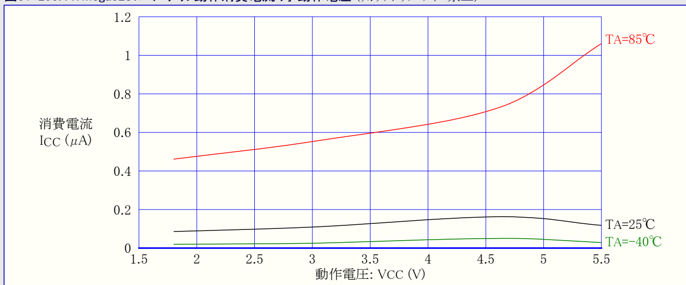
図31-295. ATmega328: パワーダウン動作消費電流 対 動作電圧 (ウォッチドッグ タイマ禁止)
