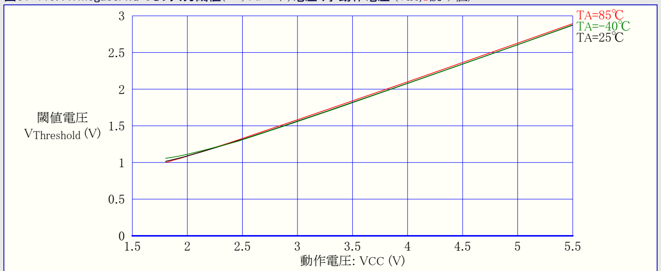
図31-119. ATmega88A:I/Oピン入力閾値(スレッシュホールド)電圧 対 動作電圧 (VIH,1読み値)
