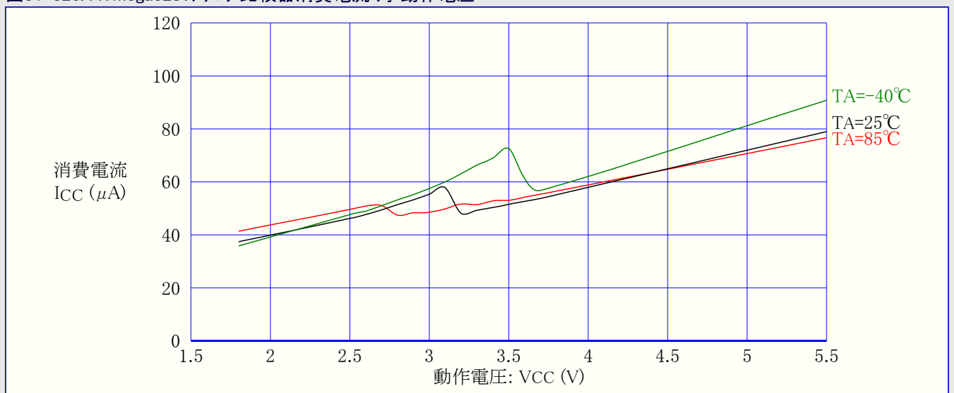
図31-327. ATmega328: 低電圧検出器(BOD)消費電流 対 動作電圧
