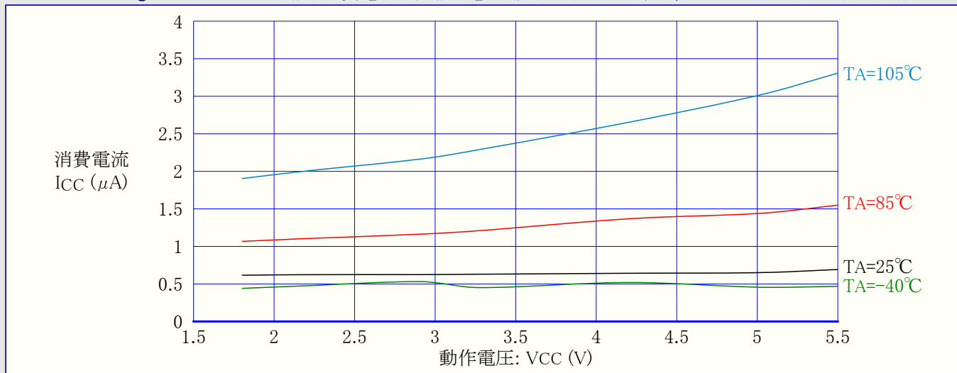
図32-152. ATmega328P: パワーセーブ動作消費電流 対 動作電圧 (ウォッチドッグ タイマ禁止, 32kHzクリスタル用発振器走行)
