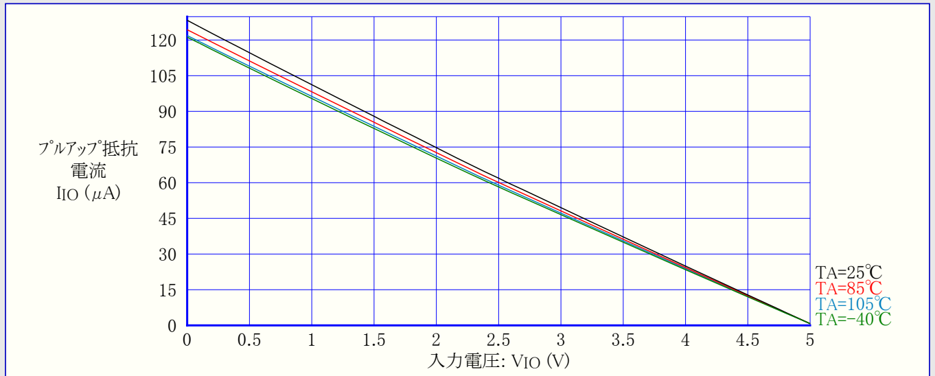
図31-64. ATmega48PA: I/Oピンプルアップ抵抗電流 対 入力電圧 (VCC=5V)
