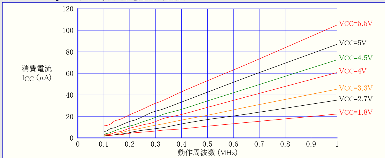
図31-139. ATmega88A:リセット消費(供給)電流 対 周波数 (100kHz~1MHz)
