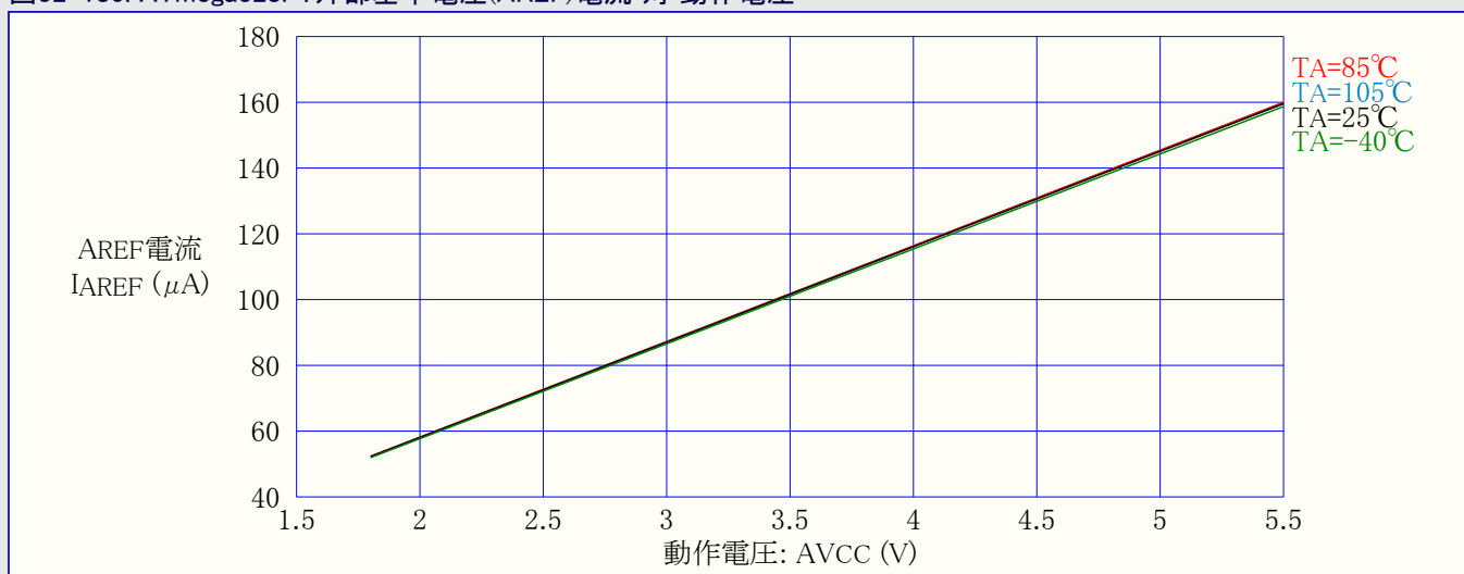
図32-180. ATmega328P: 外部基準電圧(AREF)電流 対 動作電圧
