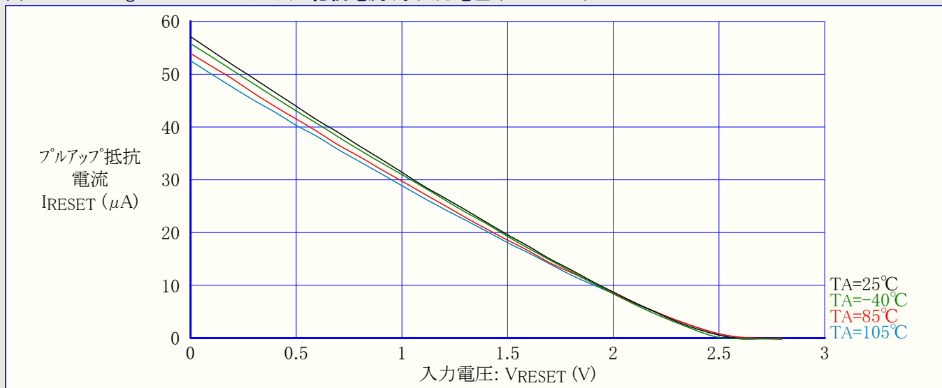
図32-64. ATmega88PA: RESETプルアップ抵抗電流 対 入力電圧 (VCC=2.7V)
