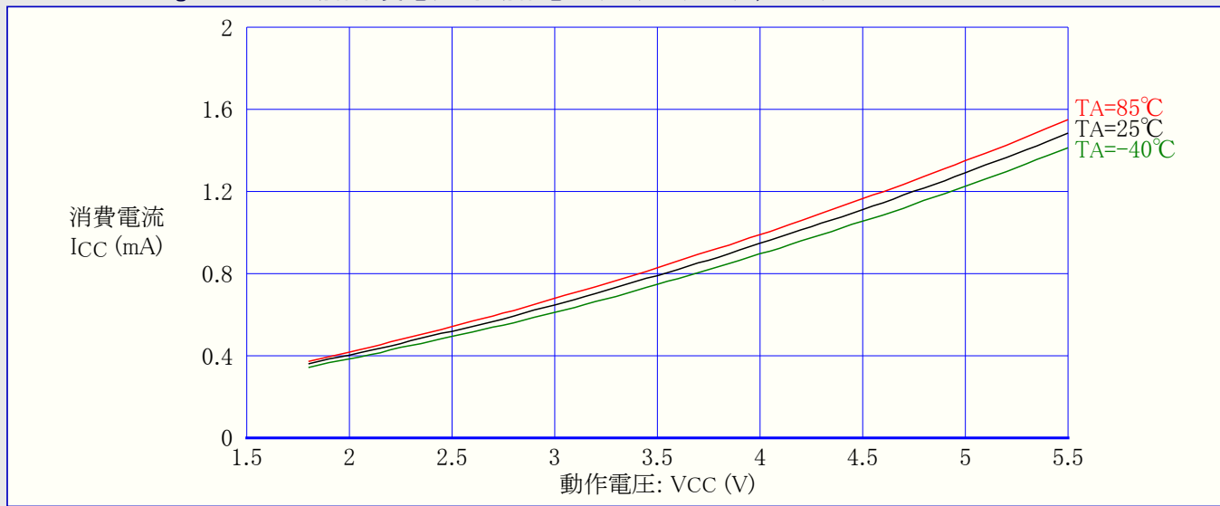
図31-294. ATmega328:アイドル動作消費電流 対 動作電圧 (内蔵RC発振器,8MHz)
