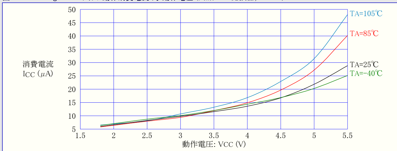
図31-56. ATmega48PA: アイドル動作消費電流 対 動作電圧 (内蔵RC発振器, CKDIV8=プログラム(0), 1MHz)
