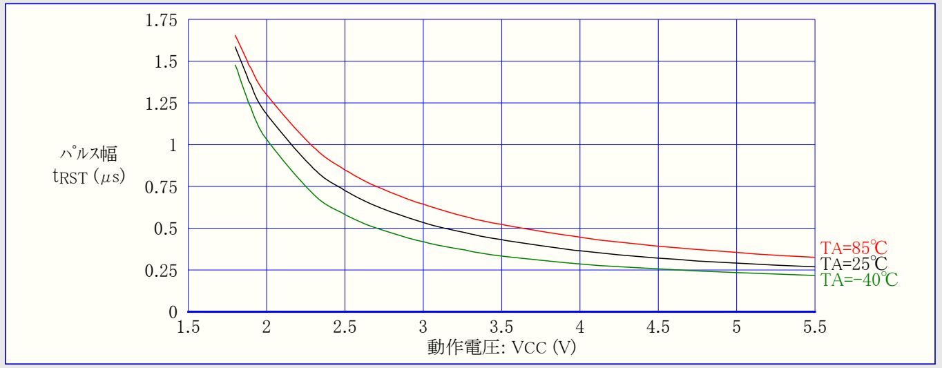
図31-236. ATmega168A: 最小リセットパルス幅 対 動作電圧
