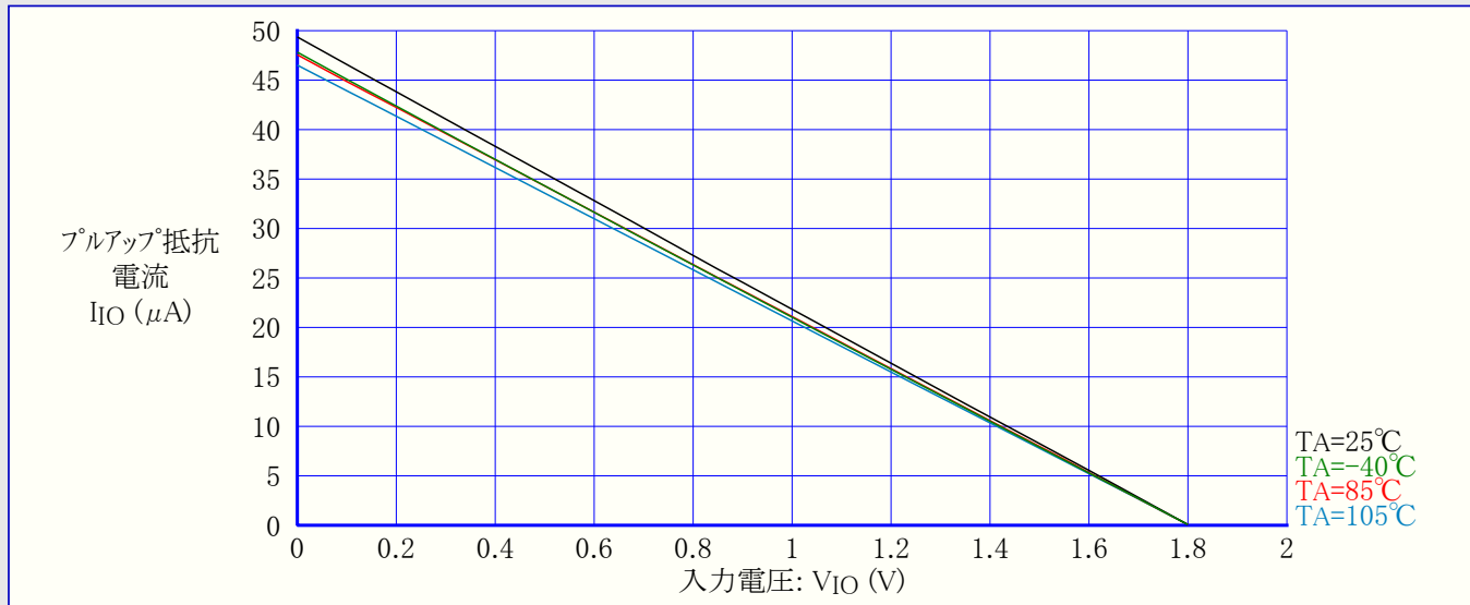
図32-154. ATmega328P: I/Oピンプルアップ抵抗電流 対 入力電圧 (VCC=1.8V)
