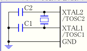
図9-2. クリスタル発振器接続図
