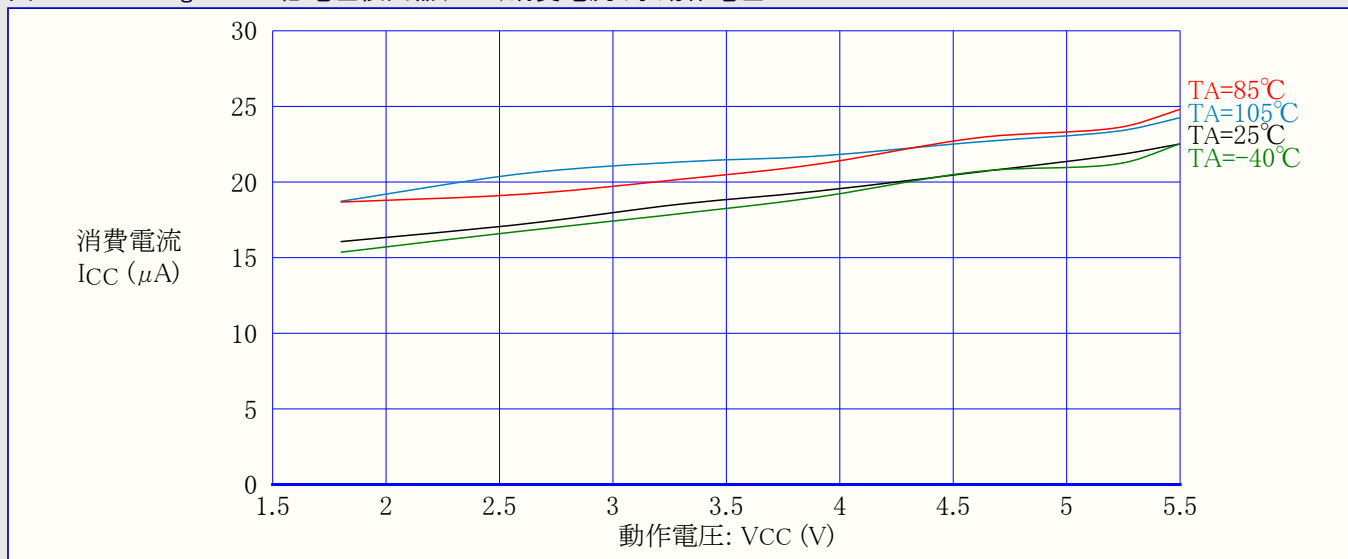
図32-87. ATmega88PA: 低電圧検出器(BOD)消費電流 対 動作電圧
