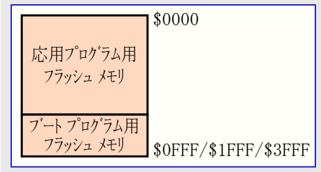
図8-2. ATmega88A/88PA/168A/168PA/328/328Pプログラムメモリ配置図
