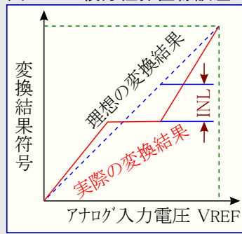
図24-12. 積分性非直線誤差
