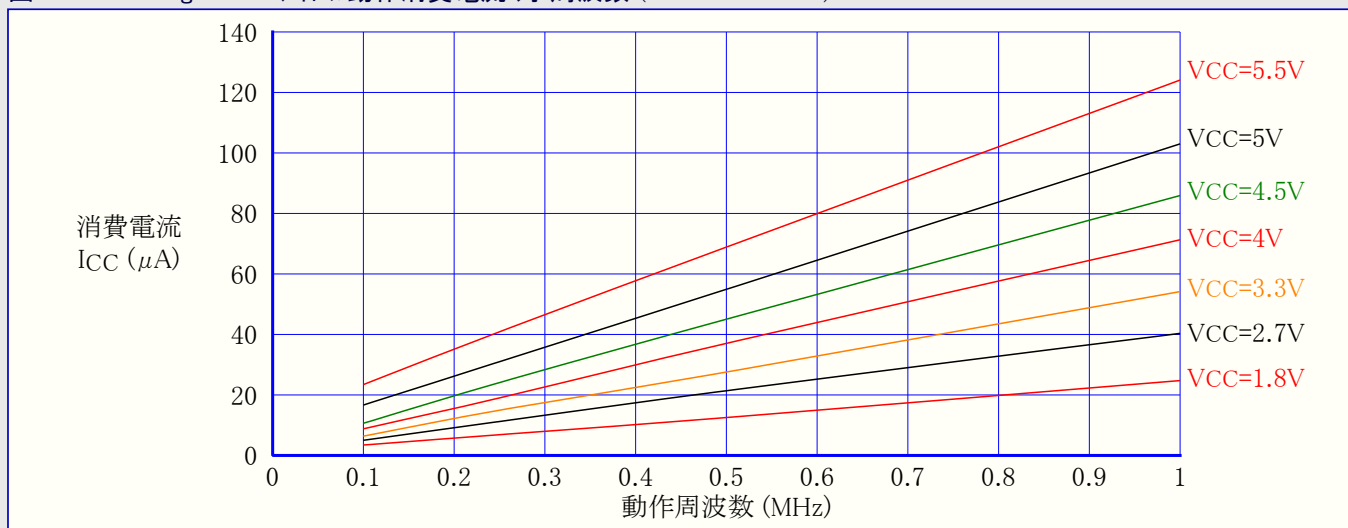
図32-52. ATmega88PA: アイドル動作消費電流 対 周波数 (100kHz~1MHz)
