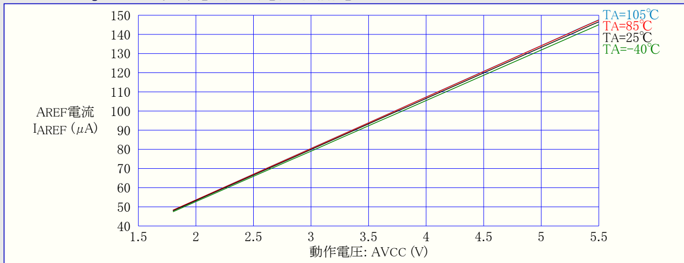
図31-88. ATmega48PA: 外部基準電圧(AREF)電流 対 動作電圧
