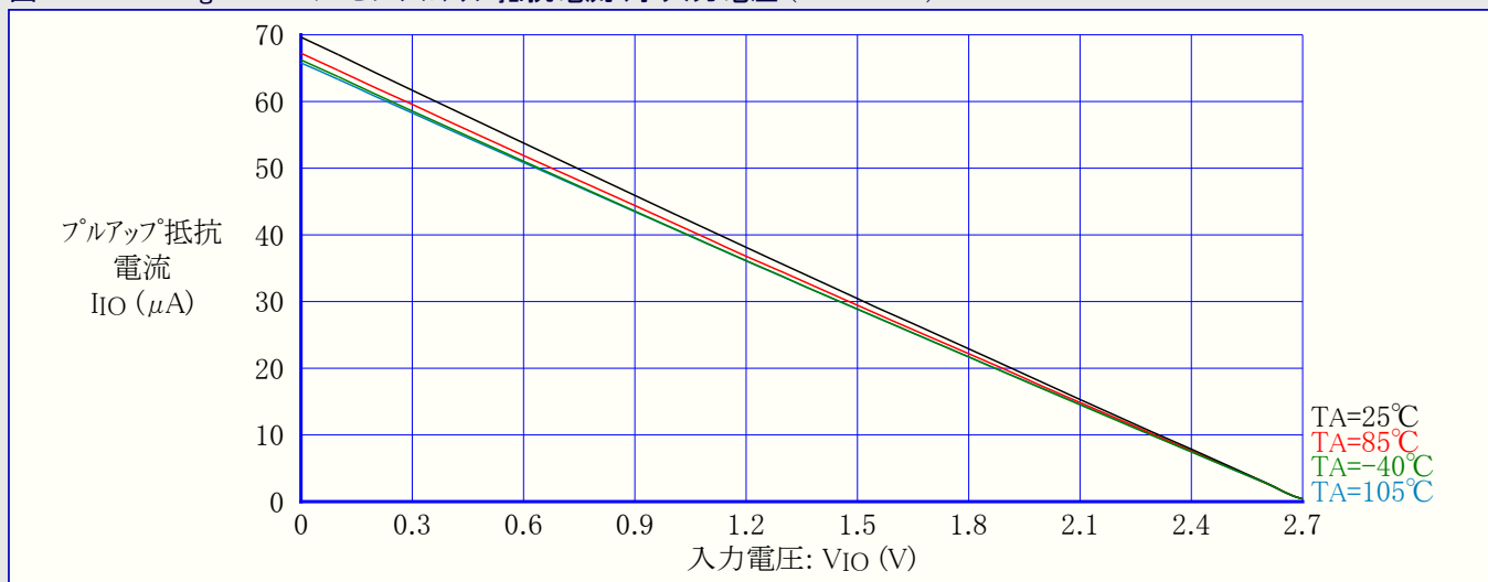
図32-16. ATmega48PA:I/Oピンプルアップ抵抗電流 対 入力電圧 (VCC=2.7V)
