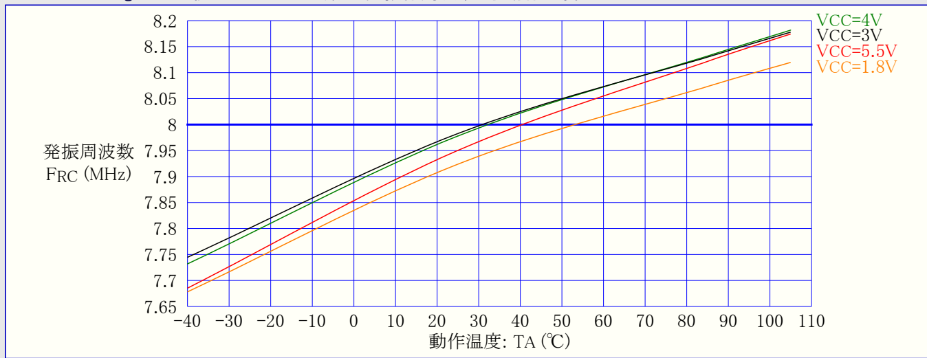
図31-85. ATmega48PA: 校正付き8MHz内蔵RC発振器周波数 対 動作温度
