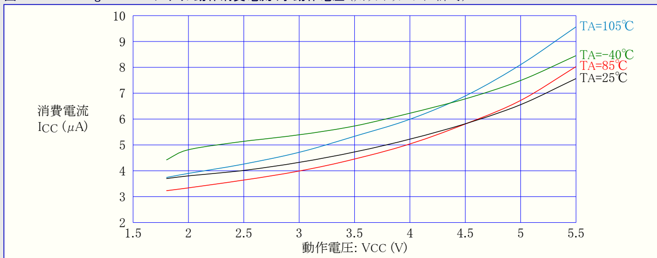
図31-343. ATmega328P: パワーダウン動作消費電流 対 動作電圧 (ウォッチドッグ タイマ許可)
