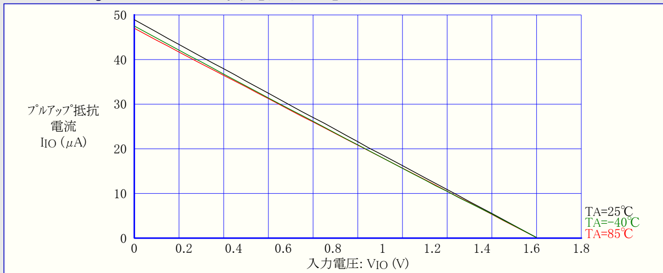
図31-204. ATmega168A:I/Oピンプルアップ抵抗電流 対 入力電圧 (VCC=1.8V)
