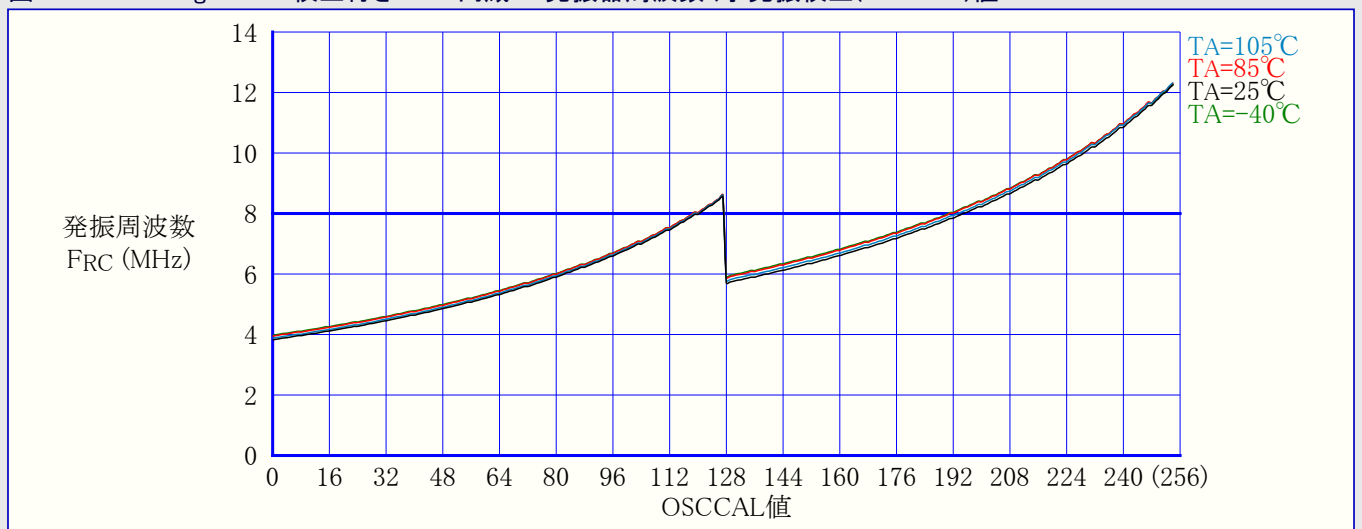
図31-181. ATmega88PA: 校正付き8MHz内蔵RC発振器周波数 対 発振校正(OSCCAL)値
