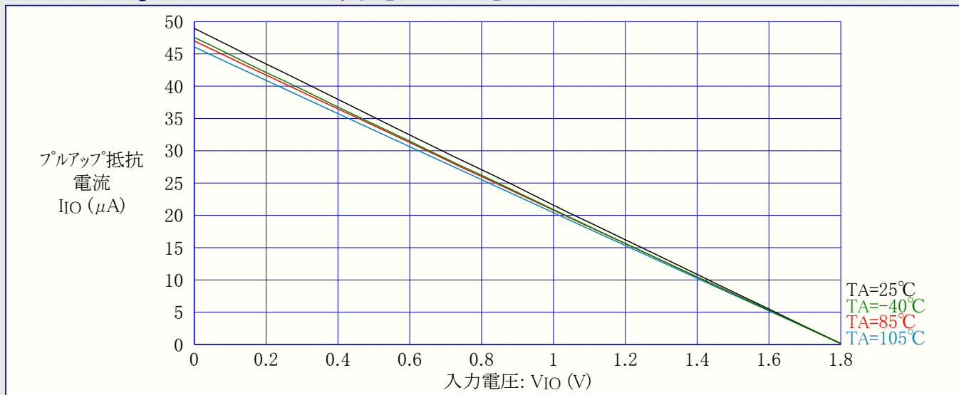
図31-251. ATmega168PA:I/Oピンプルアップ抵抗電流 対 入力電圧 ( V_{CC}=1.8V )
