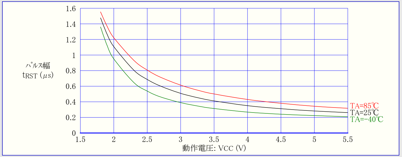
図31-47. ATmega48A: 最小リセットパルス幅 対 動作電圧
