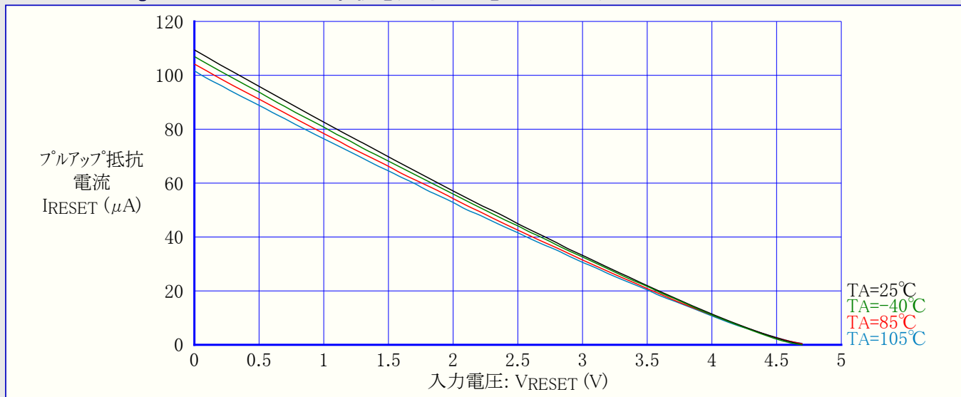
図31-256. ATmega168PA: RESETプルアップ抵抗電流 対 入力電圧 (VCC=5V)
