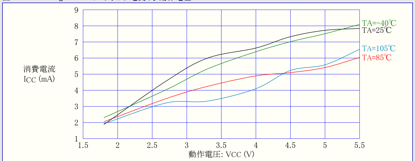
図32-136. ATmega168PA: プログラミング電流 対 動作電圧
