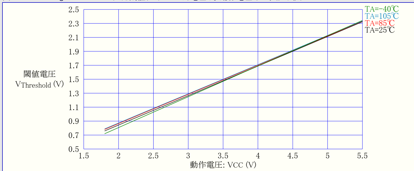
図32-168. ATmega328P: RESET入力閾値(スレッショルド)電圧 対 動作電圧 (VIL,0読み値)
