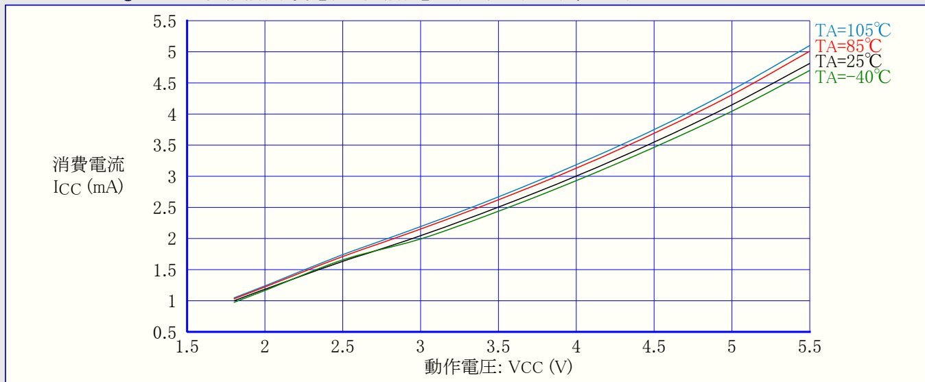
図32-96. ATmega168PA: 活動動作消費電流 対 動作電圧 (内蔵RC発振器, 8MHz)
