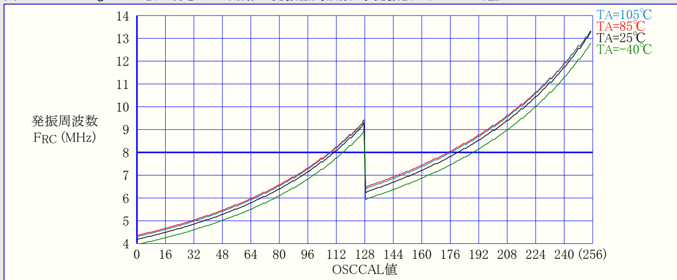
図32-178. ATmega328P: 校正付き8MHz内蔵RC発振器周波数 対 発振校正(OSCCAL)値
