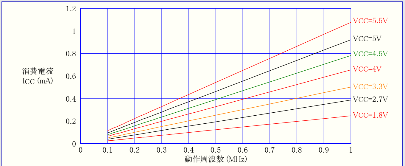
図32-140. ATmega328P: 活動動作消費電流 対 周波数 (100kHz~1MHz)
