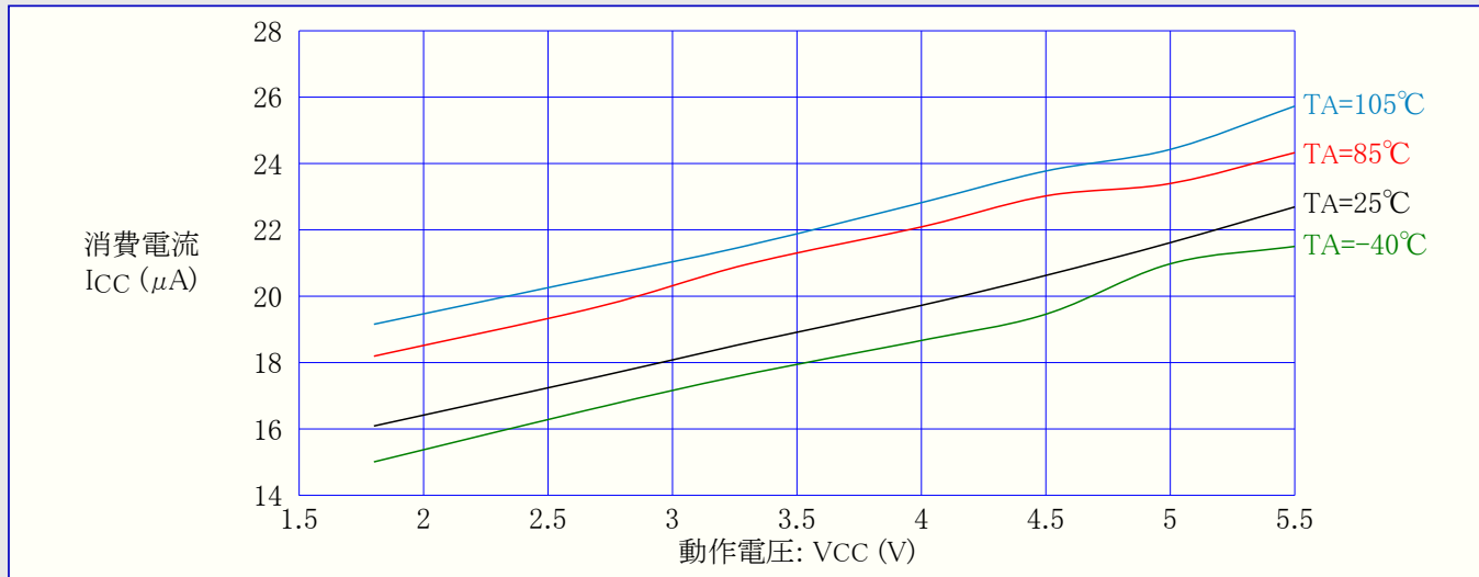
図31-280. ATmega168PA: 低電圧検出器(BOD)消費電流 対 動作電圧
