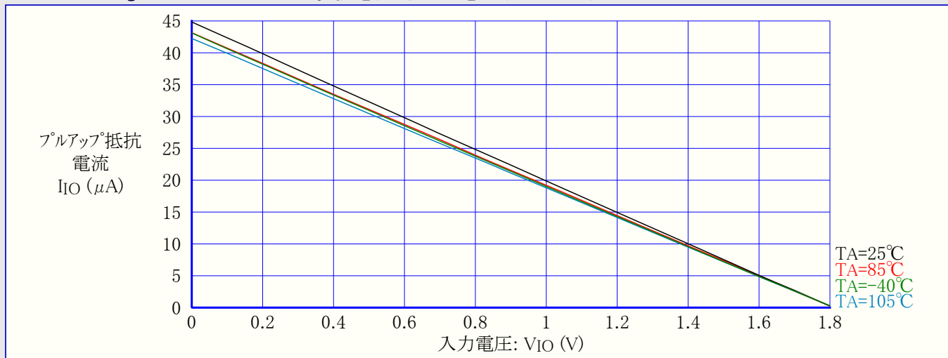
図32-15. ATmega48PA:I/Oピンプルアップ抵抗電流 対 入力電圧 (VCC=1.8V)
