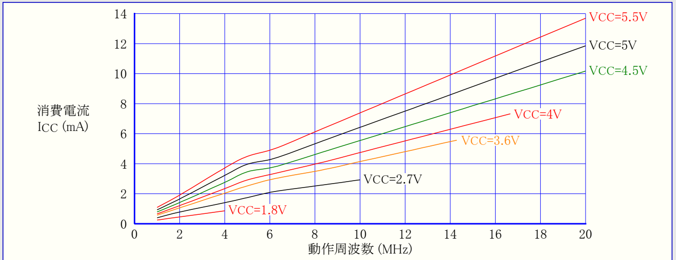
図32-141. ATmega328P: 活動動作消費電流 対 周波数 (1MHz~20MHz)
