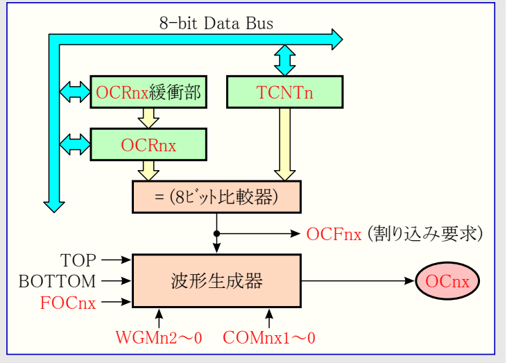
図18-3. 比較出力部構成図
