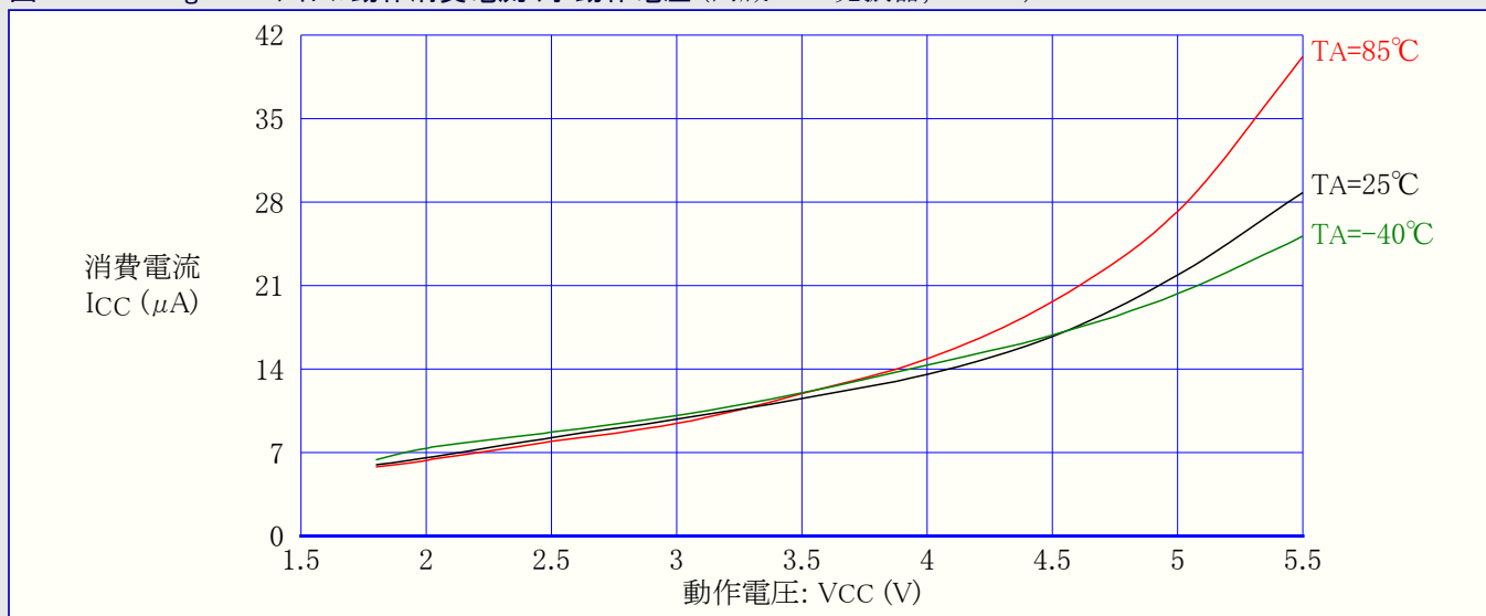
図31-8. ATmega48A: アイドル動作消費電流 対 動作電圧 (内蔵WDT発振器, 128kHz)
