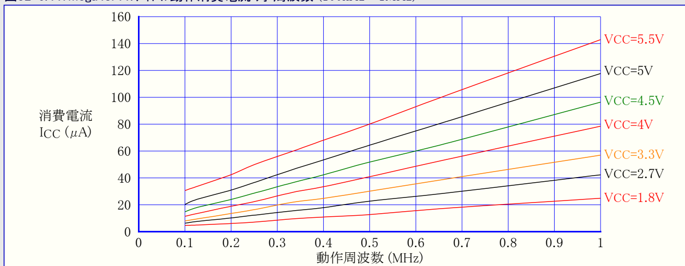
図32-6. ATmega48PA: アイドル動作消費電流 対 周波数 (100kHz~1MHz)
