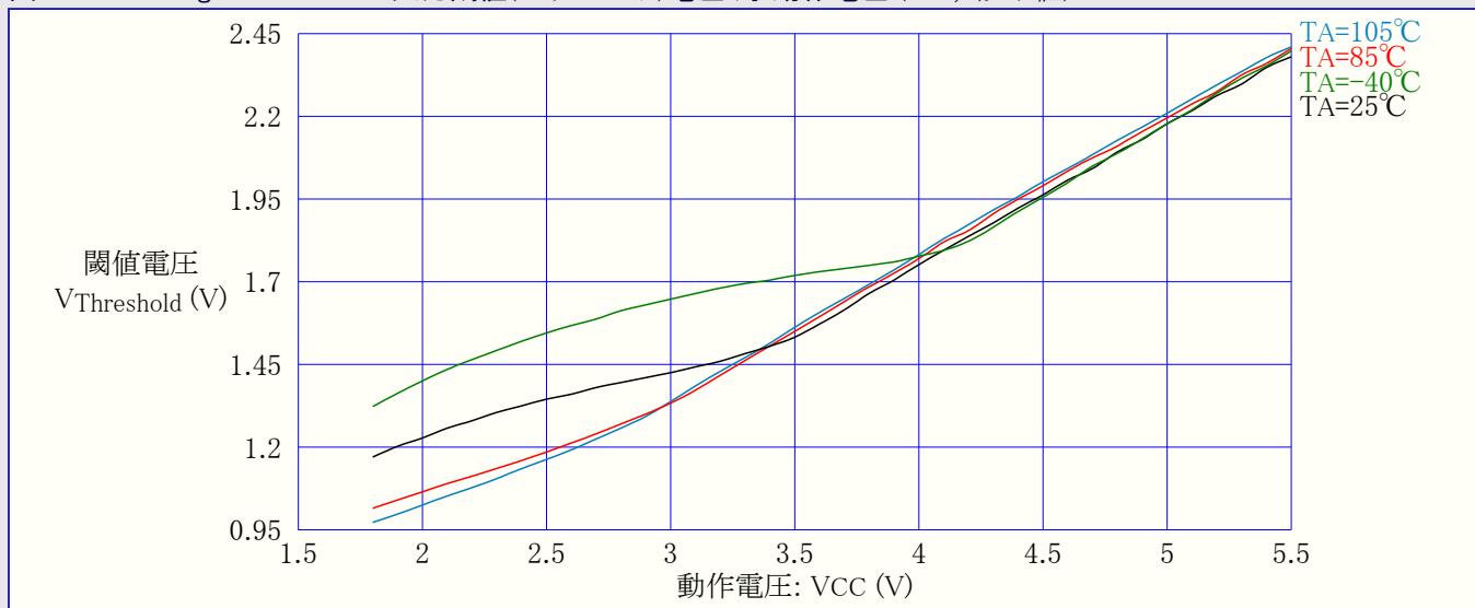
図31-75. ATmega48PA:RESET入力閾値(スレッショルド)電圧 対 動作電圧 (VIH,1読み値)
