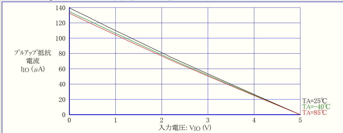
図31-111. ATmega88A:I/Oピンプルアップ抵抗電流 対 入力電圧 (VCC=5V)
