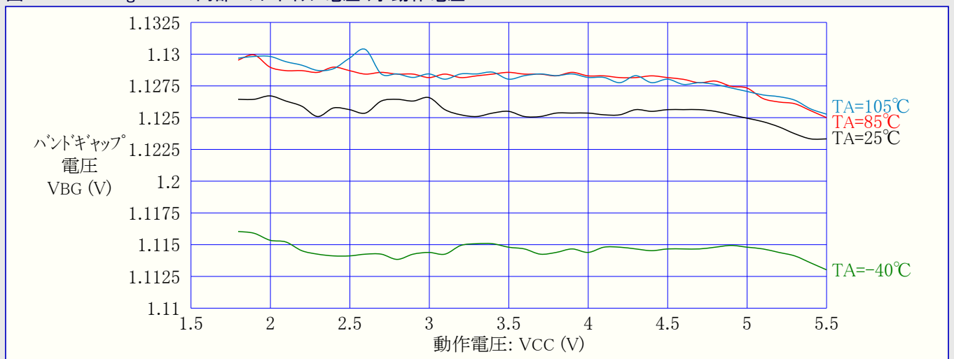
図31-81. ATmega48PA: 内部バンドギャップ電圧 対 動作電圧
