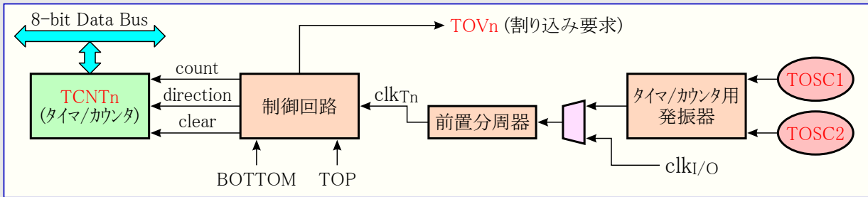
図18-2. カウンタ構成図
