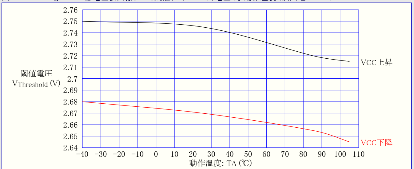
図32-32. ATmega48PA: 低電圧検出器(BOD)閾値(スレッショルド)電圧 対 動作温度 (検出電圧2.7V)
