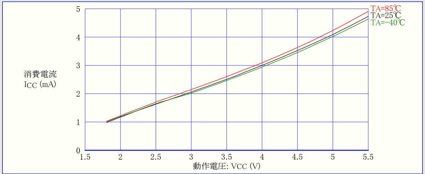
図31-99. ATmega88A: 活動動作消費電流 対 動作電圧 (内蔵RC発振器,8MHz)
