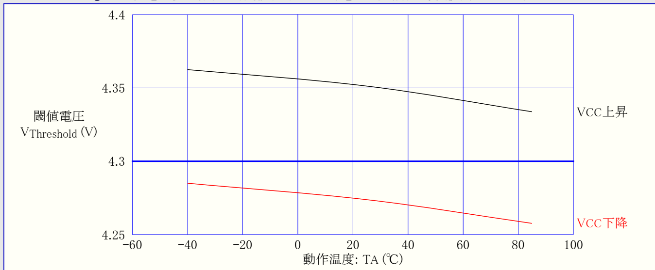
図31-317. ATmega328: 低電圧検出器(BOD)閾値(スレッシュホールド)電圧 対 動作温度 (検出電圧4.3V)
