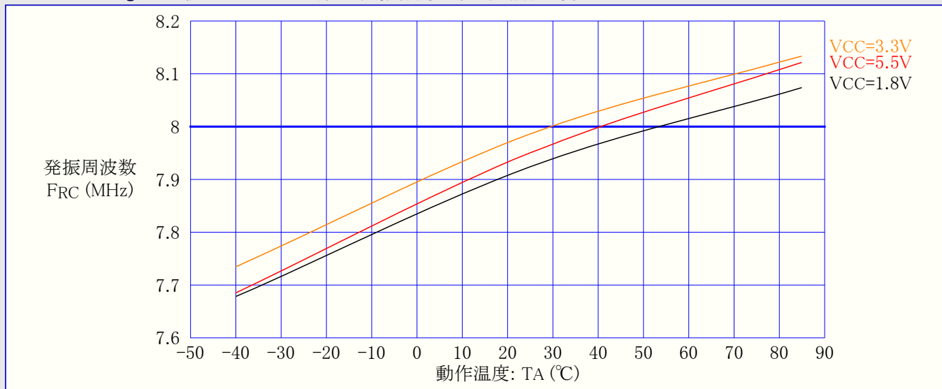
図31-38. ATmega48A: 校正付き8MHz内蔵RC発振器周波数 対 動作温度
