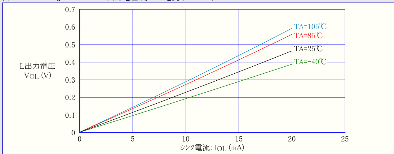
図31-163. ATmega88PA:I/Oピン出力電圧 対 シンク電流 (VCC=5V)
