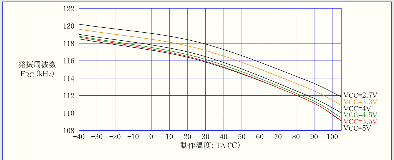
図31-272. ATmega168PA: ウォッチドッグ発振器周波数 対 動作温度
