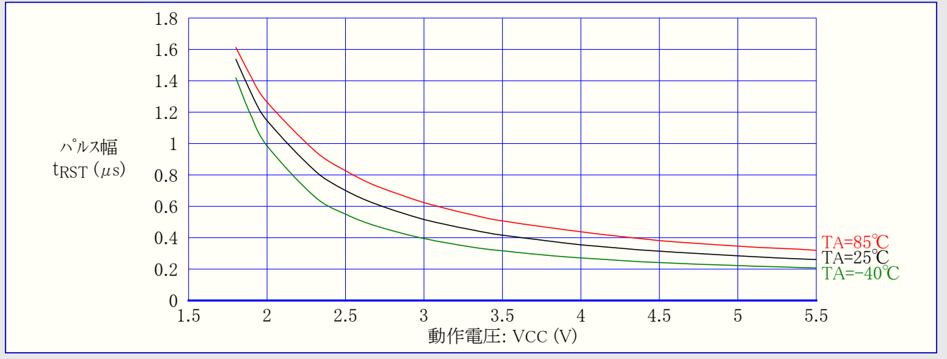
図31-331. ATmega328: 最小リセットパルス幅 対 動作電圧
