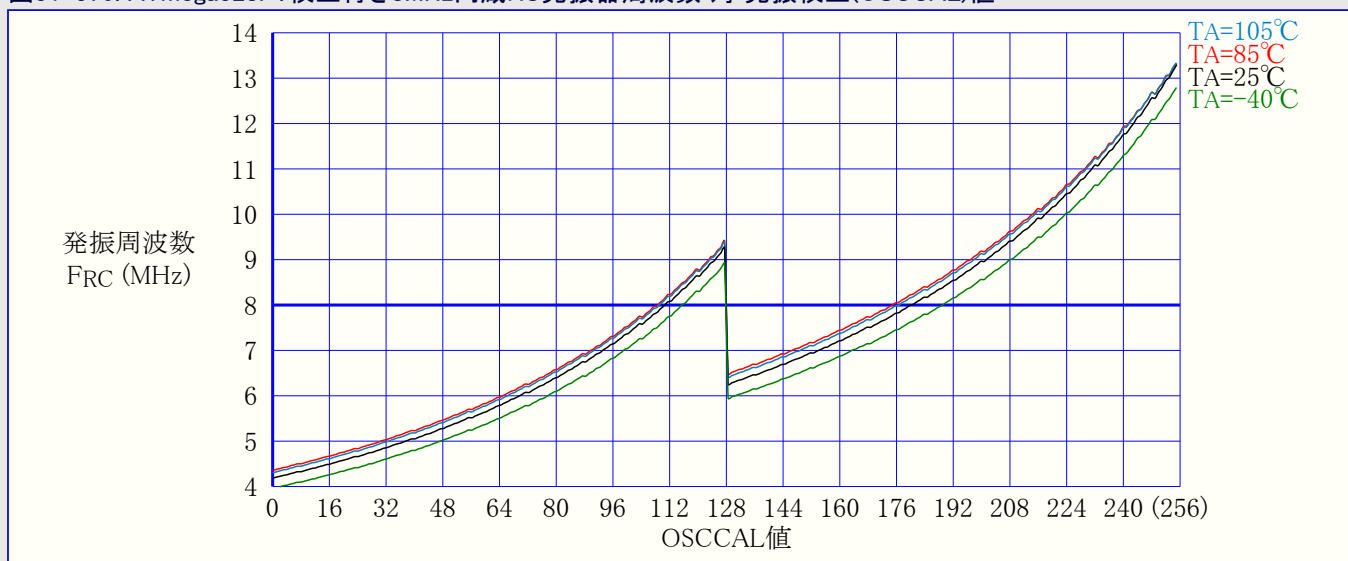
図31-370. ATmega328P: 校正付き8MHz内蔵RC発振器周波数 対 発振校正(OSCCAL)値
