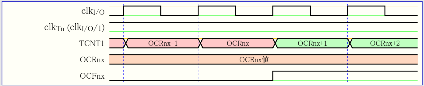
図16-10. 前置分周なし(1/1)のタイマ/カウンタ、 OCF1x 設定 タイミング
