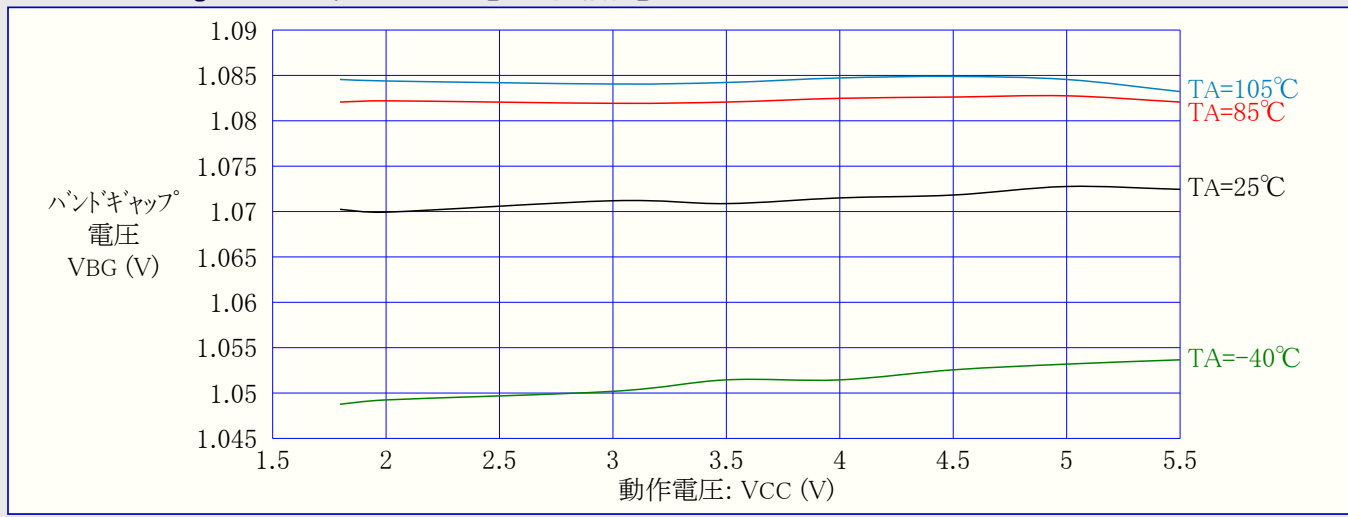
図31-176. ATmega88PA: 内部バンドギャップ電圧 対 動作電圧
