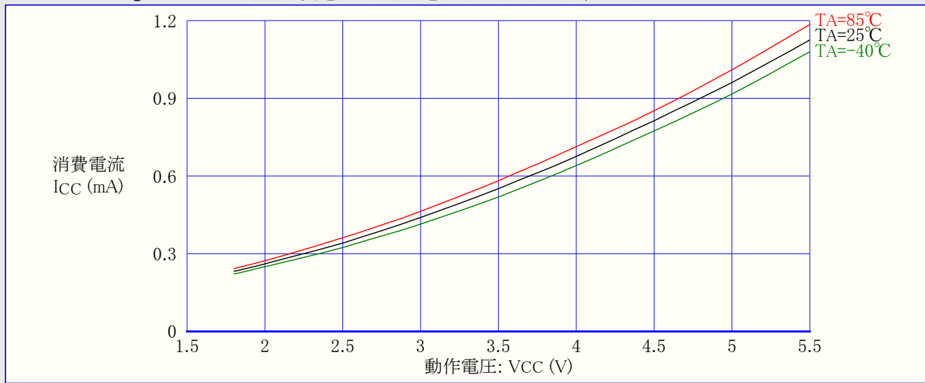
図31-199. ATmega168A:アイドル動作消費電流 対 動作電圧 (内蔵RC発振器,8MHz)
