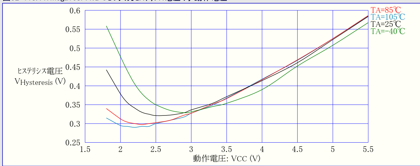
図32-118. ATmega168PA:I/Oピン入力ヒステリシス電圧 対 動作電圧
