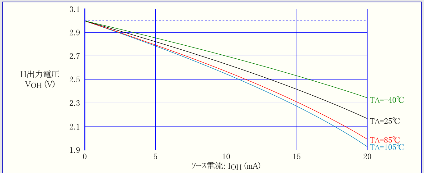
図32-162. ATmega328P:I/Oピン出力電圧 対 ソース電流 (VCC=3V)
