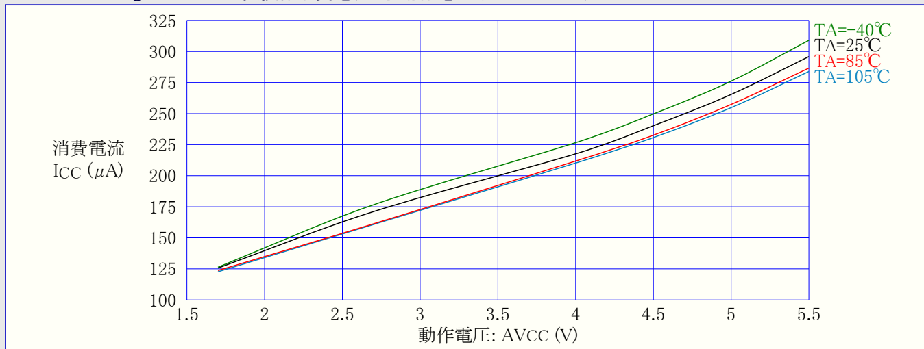
図31-277. ATmega168PA: A/D変換器消費電流 対 動作電圧 (AREF=AVCC)
