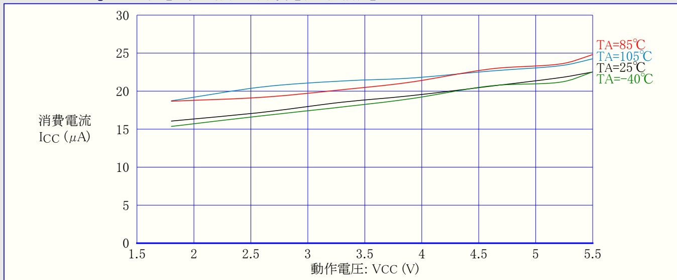
図31-185. ATmega88PA: 低電圧検出器(BOD)消費電流 対 動作電圧
