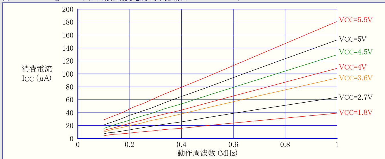
図32-145. ATmega328P: アイドル動作消費電流 対 周波数 (100kHz~1MHz)
