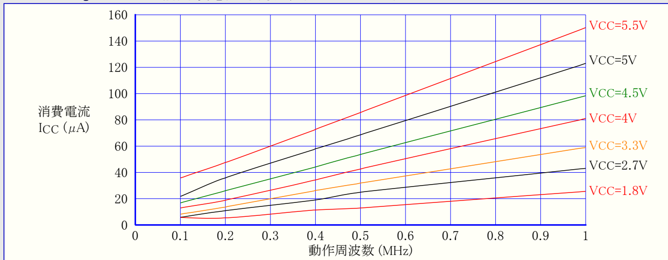
図31-6. ATmega48A: アイドル動作消費電流 対 周波数 (100kHz~1MHz)
