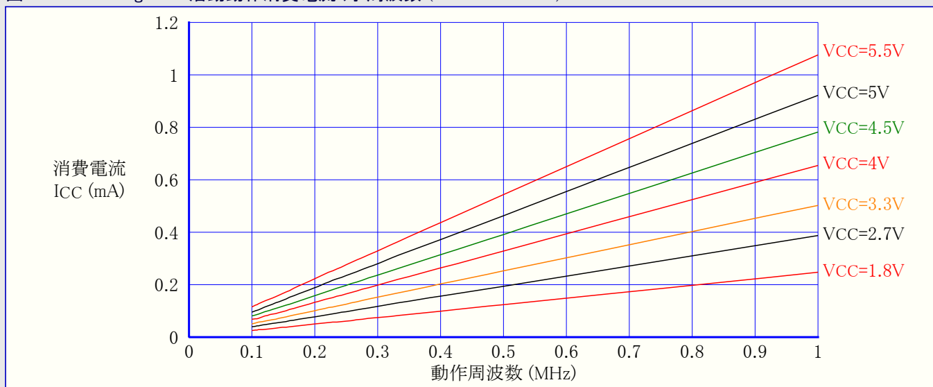
図31-285. ATmega328: 活動動作消費電流 対 周波数 (100kHz~1MHz)
