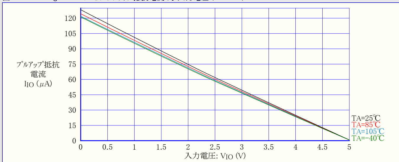
図32-17. ATmega48PA:I/Oピンプルアップ抵抗電流 対 入力電圧 (VCC=5V)
