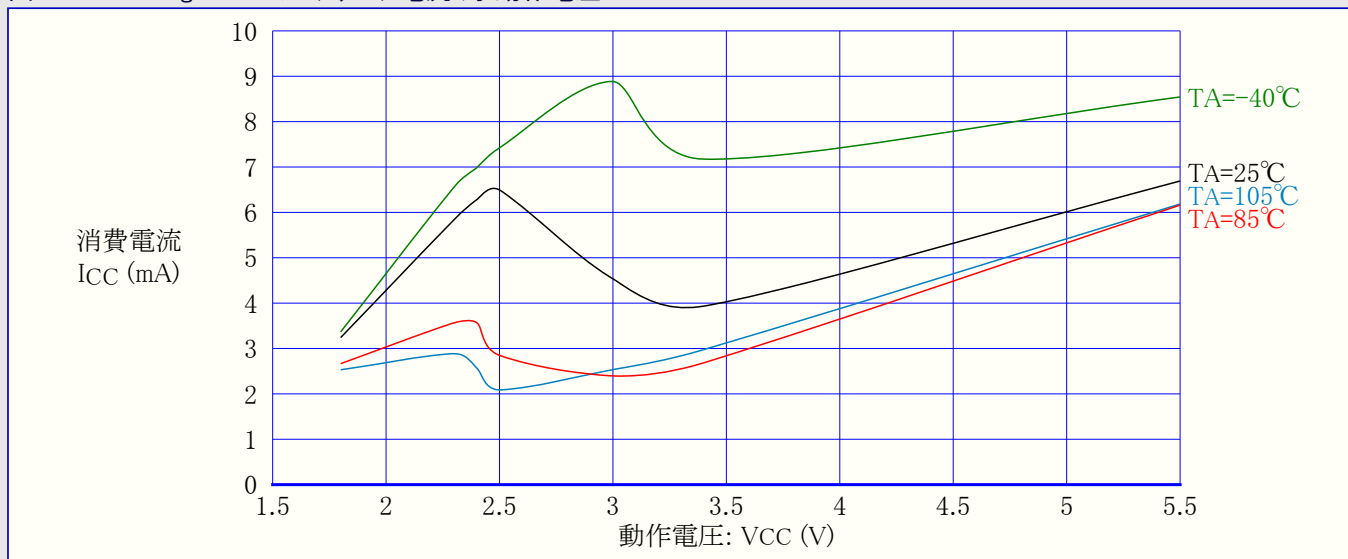
図32-88. ATmega88PA: プログラミング電流 対 動作電圧
