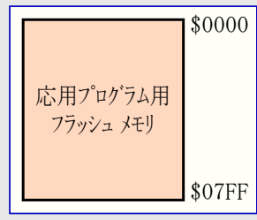
図8-1. ATmega48A/48PAプログラムメモリ配置図
