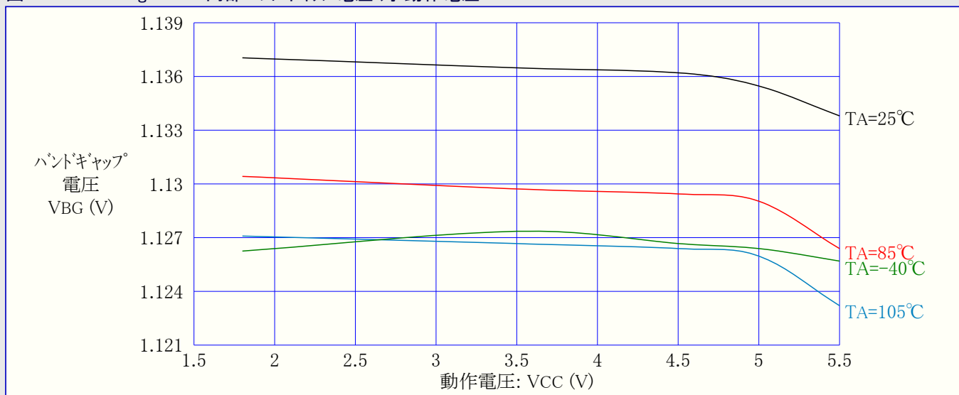
図31-365. ATmega328P: 内部バンドギャップ電圧 対 動作電圧
