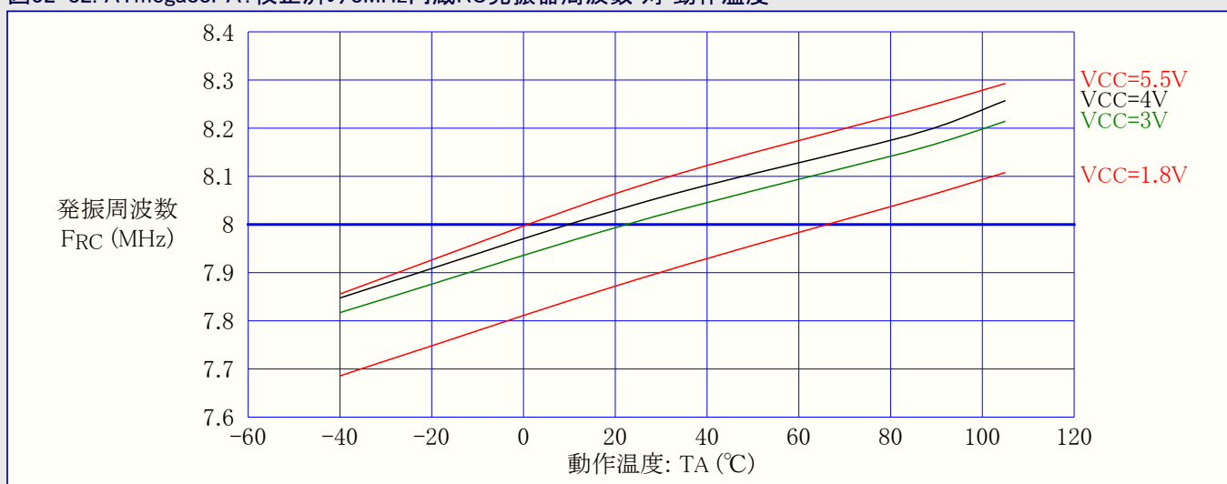
図32-82. ATmega88PA: 校正済み8MHz内蔵RC発振器周波数 対 動作温度
