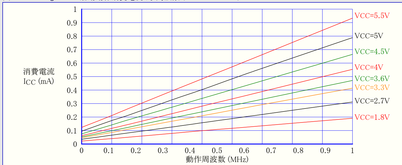
図32-1. ATmega48PA: 活動動作消費電流 対 周波数 (100kHz~1MHz)
