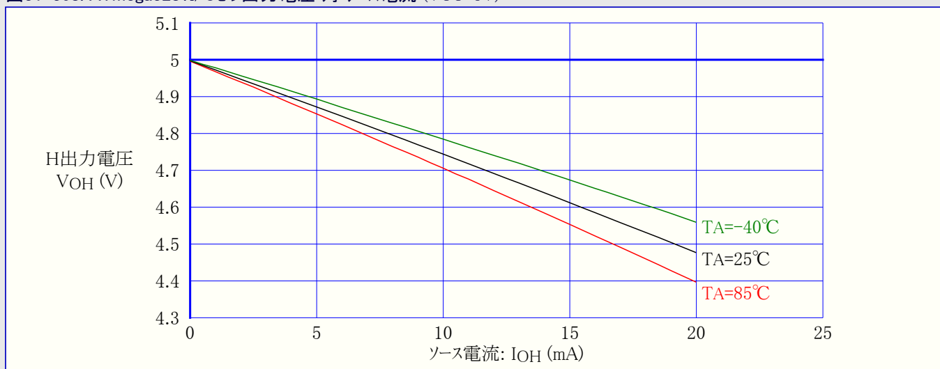
図31-308. ATmega328:I/Oピン出力電圧 対 ソース電流 (VCC=5V)
