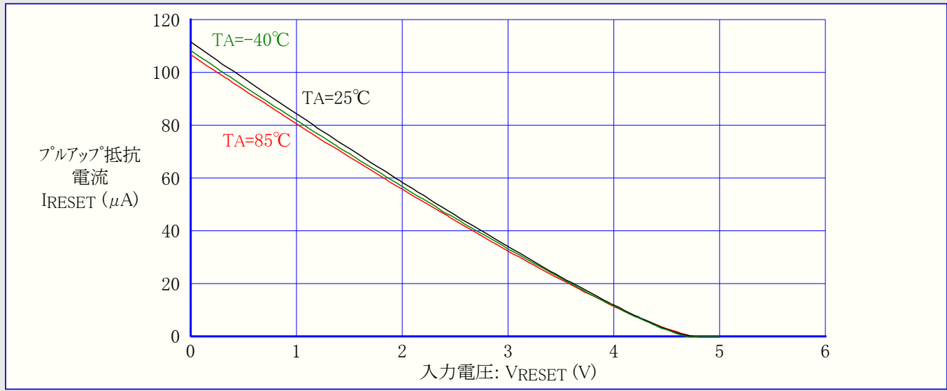
図31-304. ATmega328: RESETプルアップ抵抗電流 対 入力電圧 (VCC=5V)
