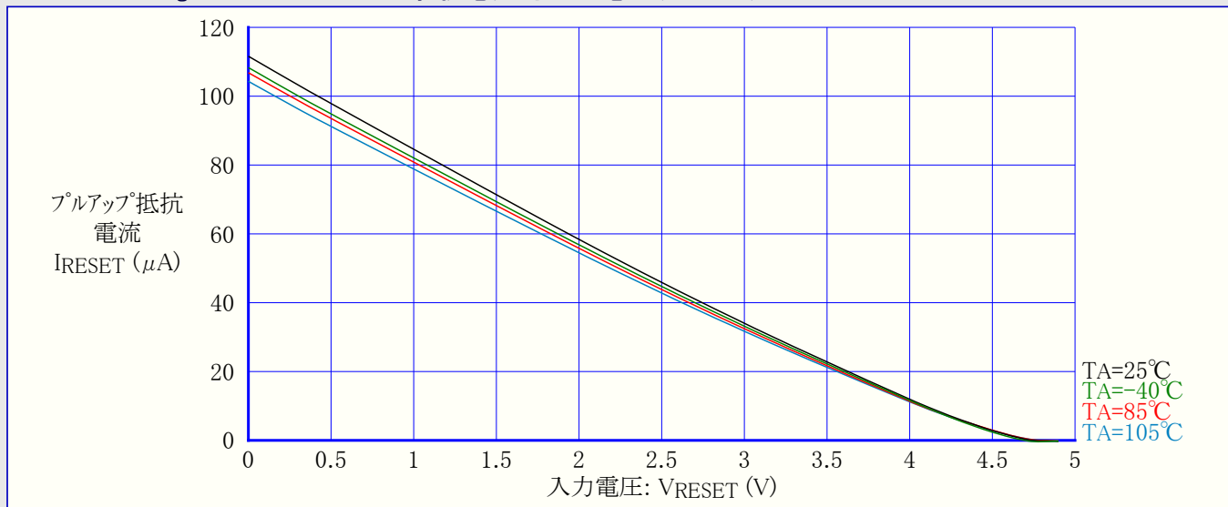
図31-351. ATmega328P: RESETフルアップ抵抗電流 対 入力電圧 (VCC=5V)
