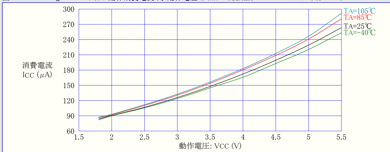
図32-100. ATmega168PA: アイドル動作消費電流 対 動作電圧 (内蔵RC発振器, CKDIV8=プログラム(0), 1MHz)
