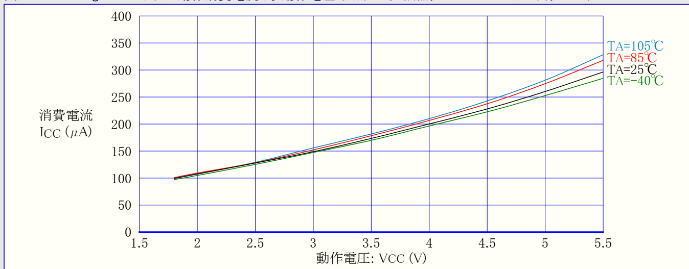
図32-55. ATmega88PA:アイドル動作消費電流 対 動作電圧 (内蔵RC発振器,CKDIV8=プログラム(0),1MHz)
