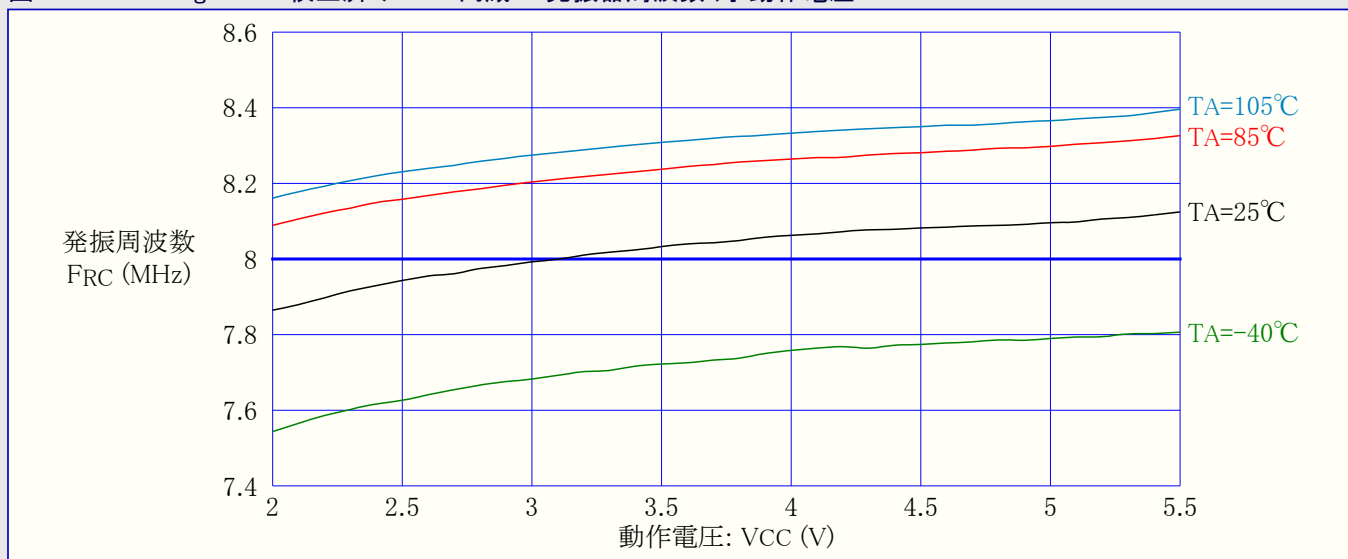
図31-368. ATmega328P: 校正済み8MHz内蔵RC発振器周波数 対 動作電圧
