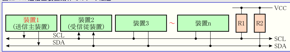
図22-11. 送信主装置動作でのデータ転送
