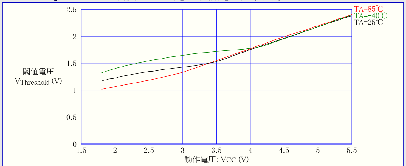
図31-28. ATmega48A:RESET入力閾値(スレッショルド)電圧 対 動作電圧 (VIH,1読み値)
