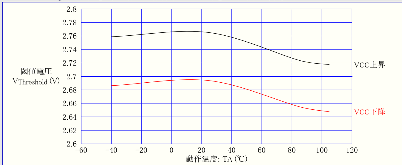
図31-173. ATmega88PA: 低電圧検出器(BOD)閾値(スレッショルド)電圧 対 動作温度 (検出電圧2.7V)
