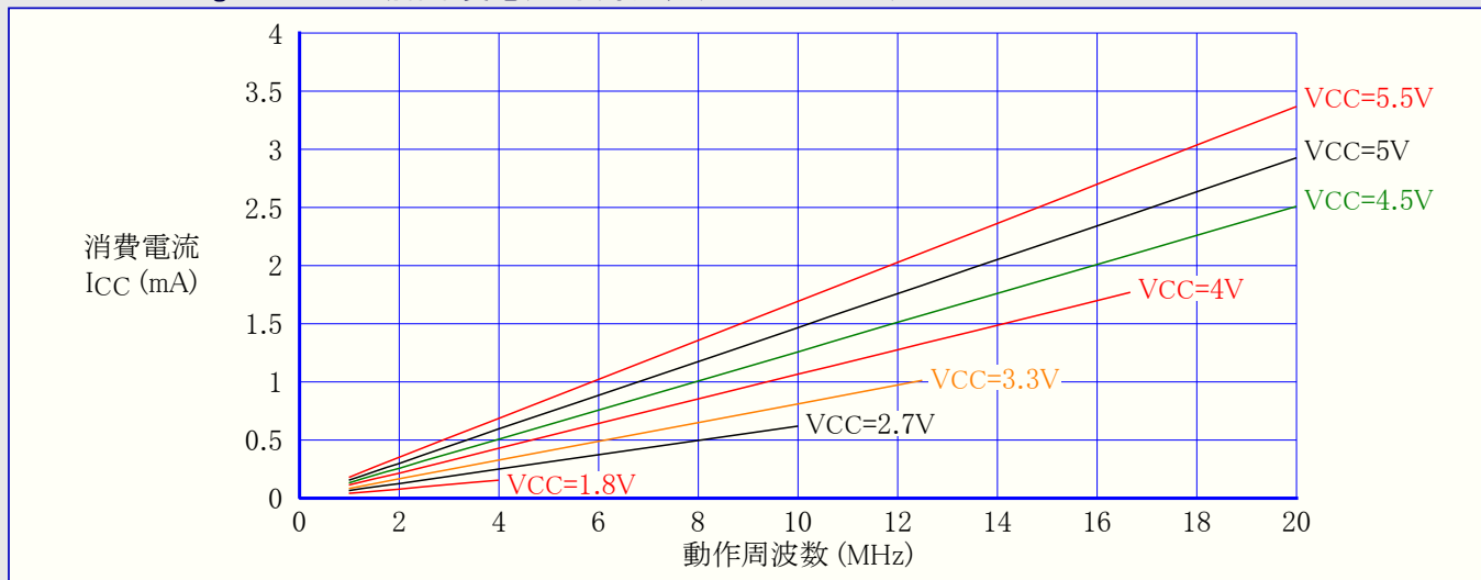
図31-291. ATmega328:アイドル動作消費電流 対 周波数 (1MHz~20MHz)
