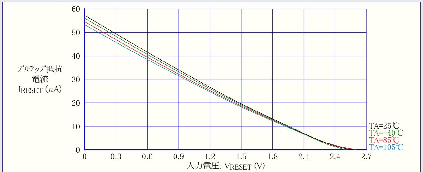
図31-350. ATmega328P: RESETプルアップ抵抗電流 対 入力電圧 (VCC=2.7V)
