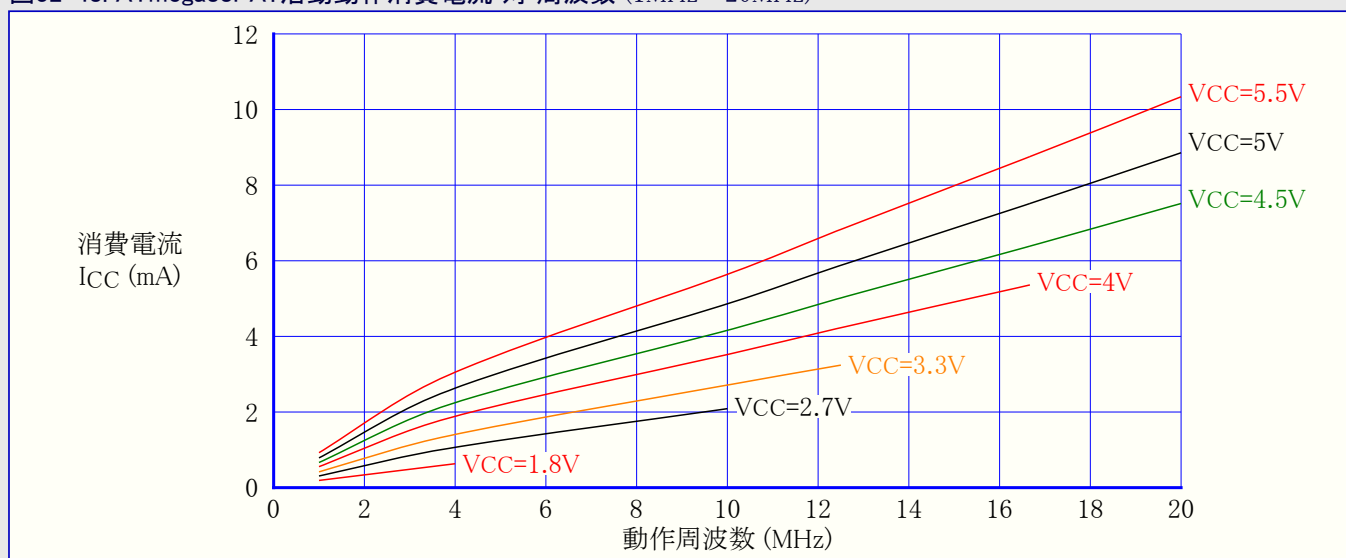
図32-48. ATmega88PA: 活動動作消費電流 対 周波数 (1MHz~20MHz)
