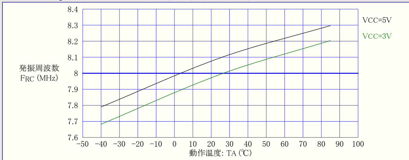
図31-322. ATmega328: 校正済み8MHz内蔵RC発振器周波数 対 動作温度
