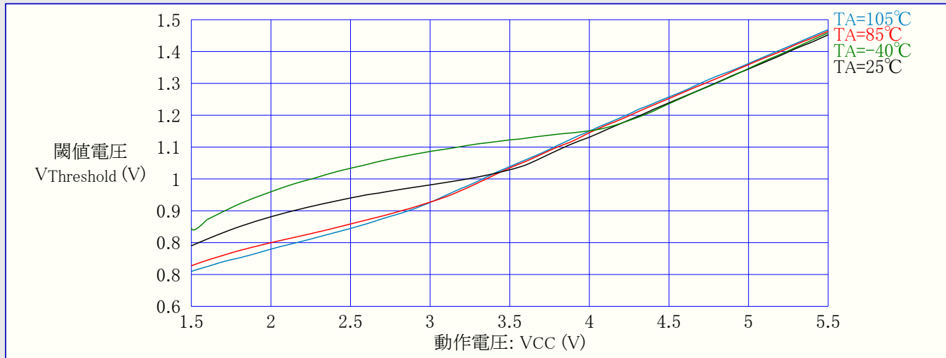
図32-119. ATmega168PA: RESET入力閾値(スレッシュホールド)電圧 対 動作電圧 (VIH,1読み値)
