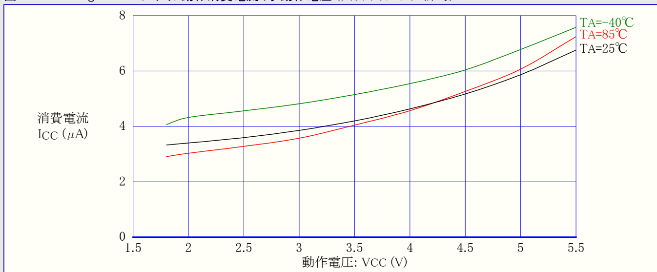
図31-12. ATmega48A: パワーダウン動作消費電流 対 動作電圧 (ウォッチドッグ タイマ許可)
