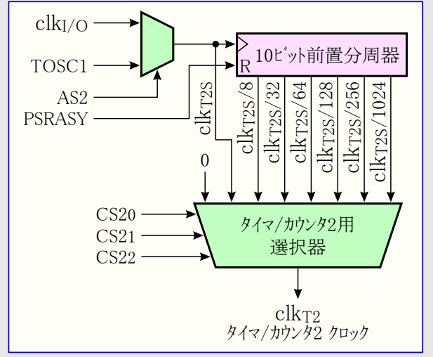
図18-12. タイマ/カウンタ2前置分周器部構成
