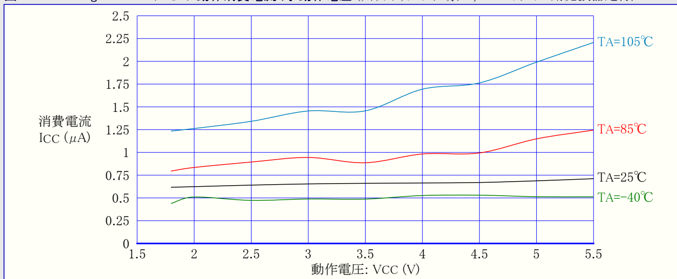
図31-60. ATmega48PA: パワーセーブ動作消費電流 対 動作電圧 (ウォッチドッグ タイマ禁止, 32kHzクリスタル用発振器走行)
