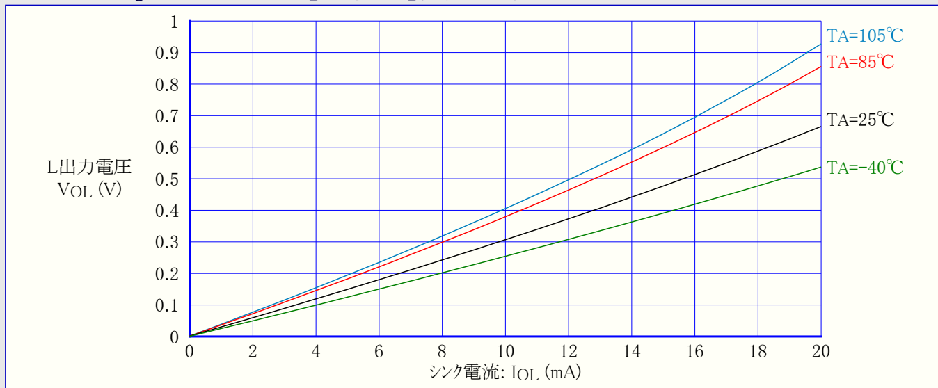
図32-112. ATmega168PA: I/Oピン出力電圧 対 シンク電流 (VCC=3V)
