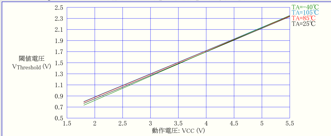
図31-265. ATmega168PA: RESET入力閾値(スレッショルト)電圧 対 動作電圧 (VIL,0読み値)
