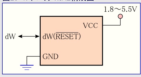
図25-1. デバッグWIRE構成図
