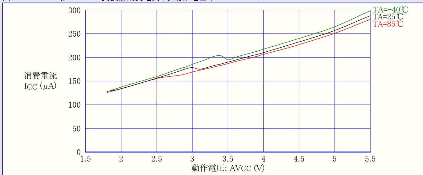
図31-134. ATmega88A: A/D変換器消費電流 対 動作電圧 (AREF=AVCC)
