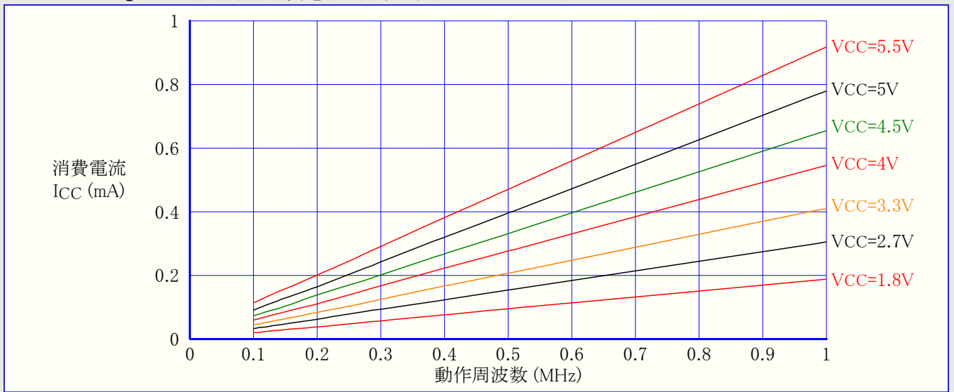
図31-48. ATmega48PA: 活動動作消費電流 対 周波数 (100kHz~1MHz)
