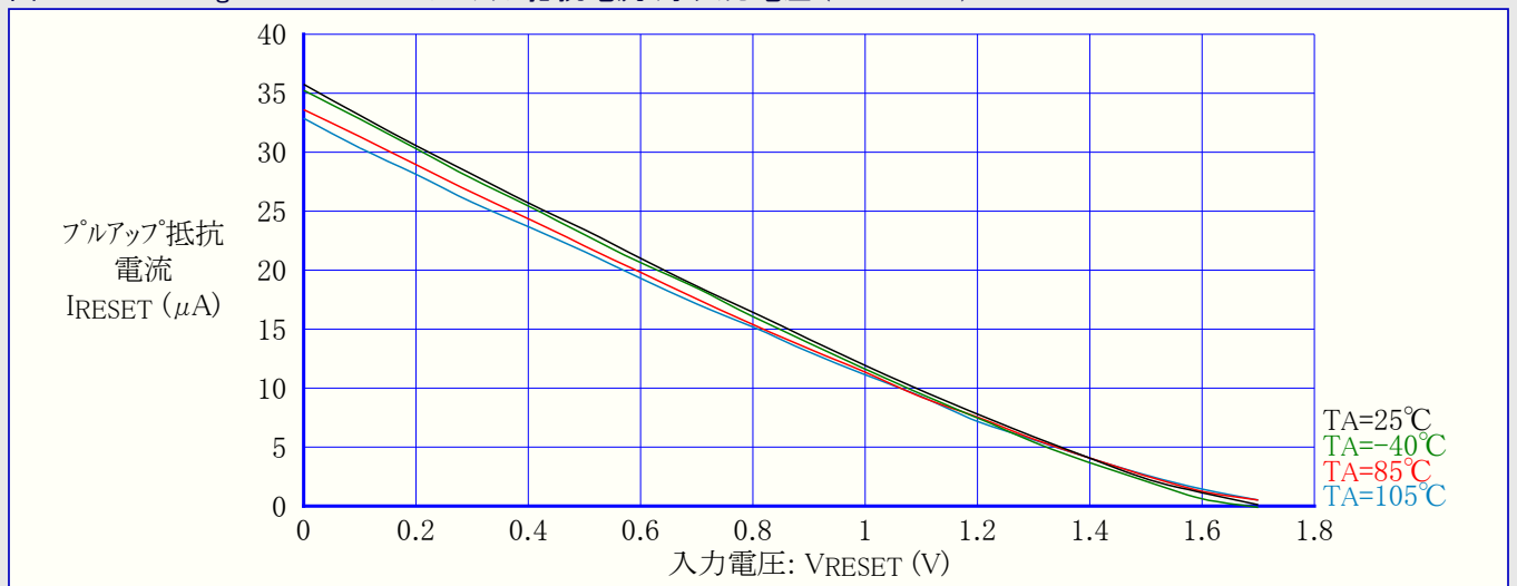
図32-109. ATmega168PA:RESETプルアップ抵抗電流 対 入力電圧 (VCC=1.8V)
