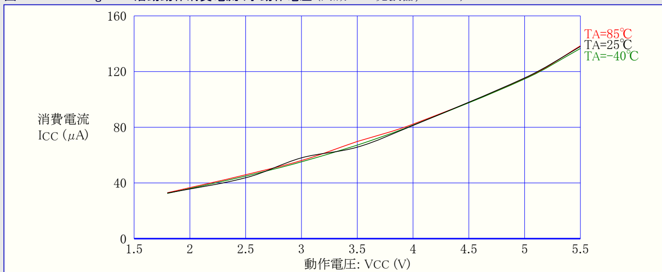
図31-287. ATmega328: 活動動作消費電流 対 動作電圧 (内蔵WDT発振器, 128kHz)
