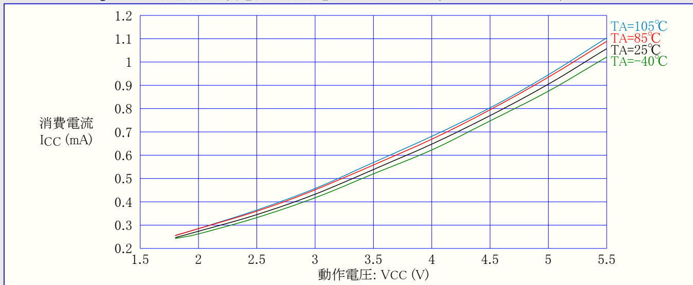
図31-240. ATmega168PA: 活動動作消費電流 対 動作電圧 (内蔵RC発振器, CKDIV8=プログラム(0), 1MHz)
