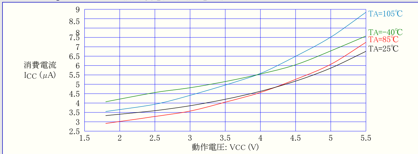
図32-12. ATmega48PA:パワーダウン動作消費電流 対 動作電圧 (ウォッチドッグ タイマ許可)
