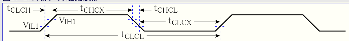
図29-2. 外部クロック駆動波形
