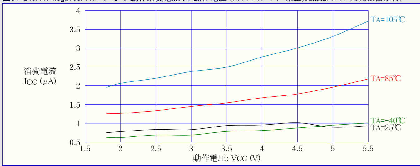
図31-249. ATmega168PA: パワーセーブ動作消費電流 対 動作電圧 (ウォッチドッグ タイマ禁止, 32kHzクリスタル用発振器走行)
