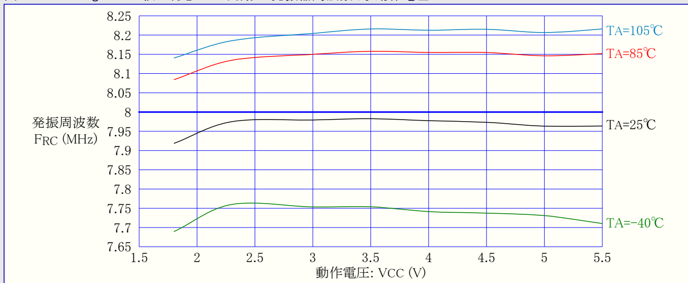
図31-84. ATmega48PA: 校正付き8MHz内蔵RC発振器周波数 対 動作電圧
