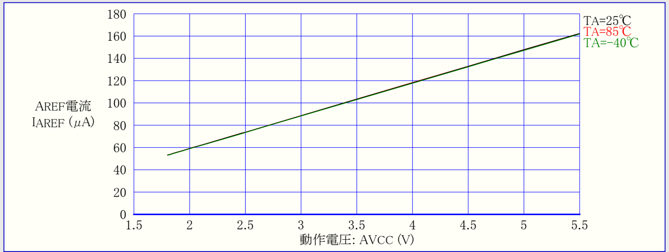
図31-231. ATmega168A: アナログ比較器消費電流 対 動作電圧
