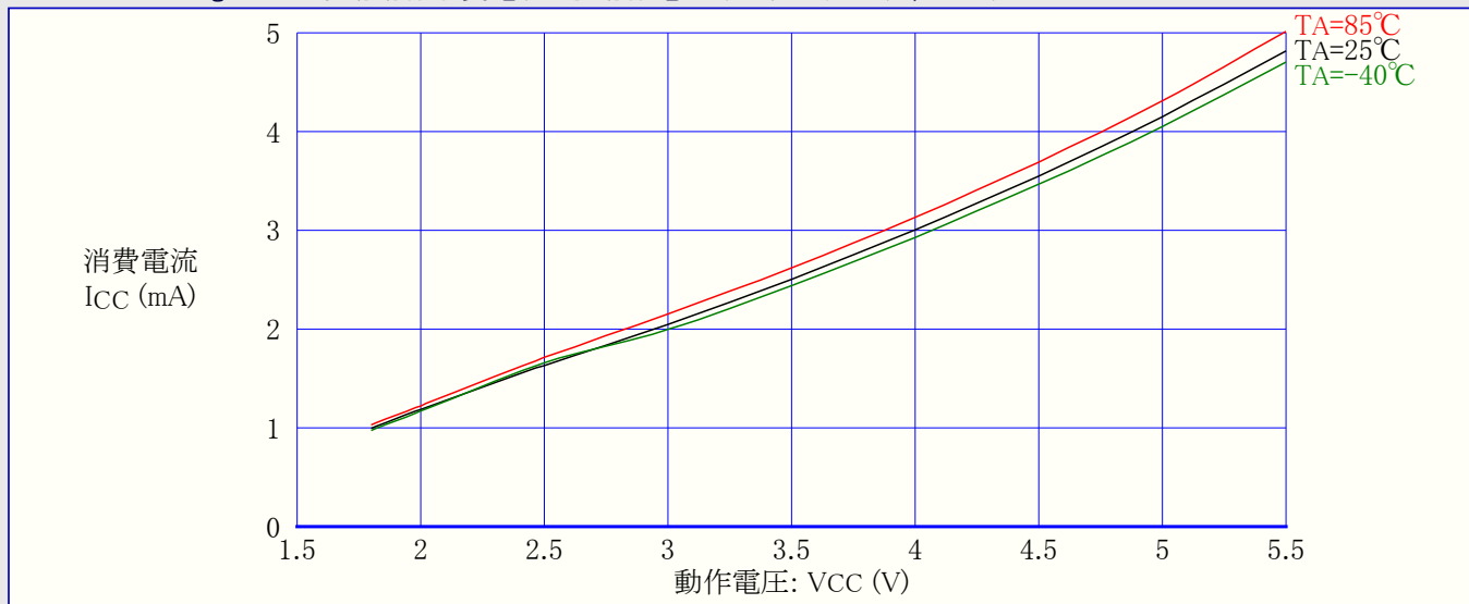
図31-194. ATmega168A: 活動動作消費電流 対 動作電圧 (内蔵RC発振器, 8MHz)
