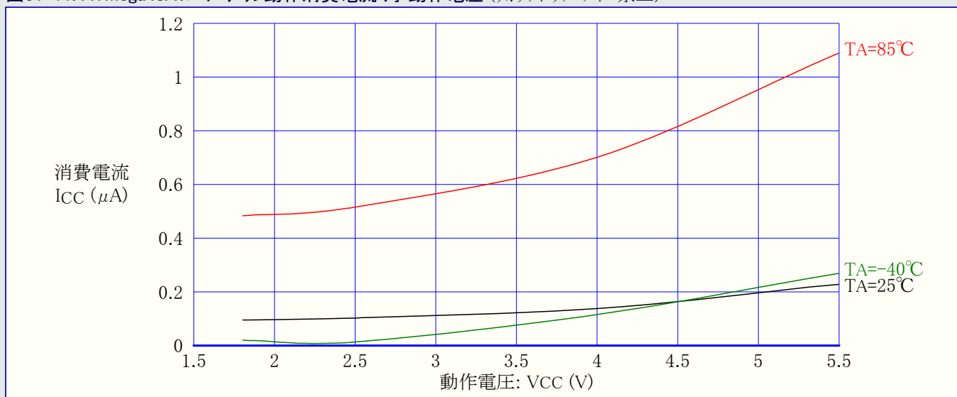
図31-11. ATmega48A: パワーダウン動作消費電流 対 動作電圧 (ウォッチドッグ タイマ禁止)
