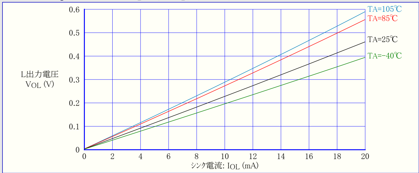
図32-113. ATmega168PA:I/Oピン出力電圧 対 シンク電流 (VCC=5V)
