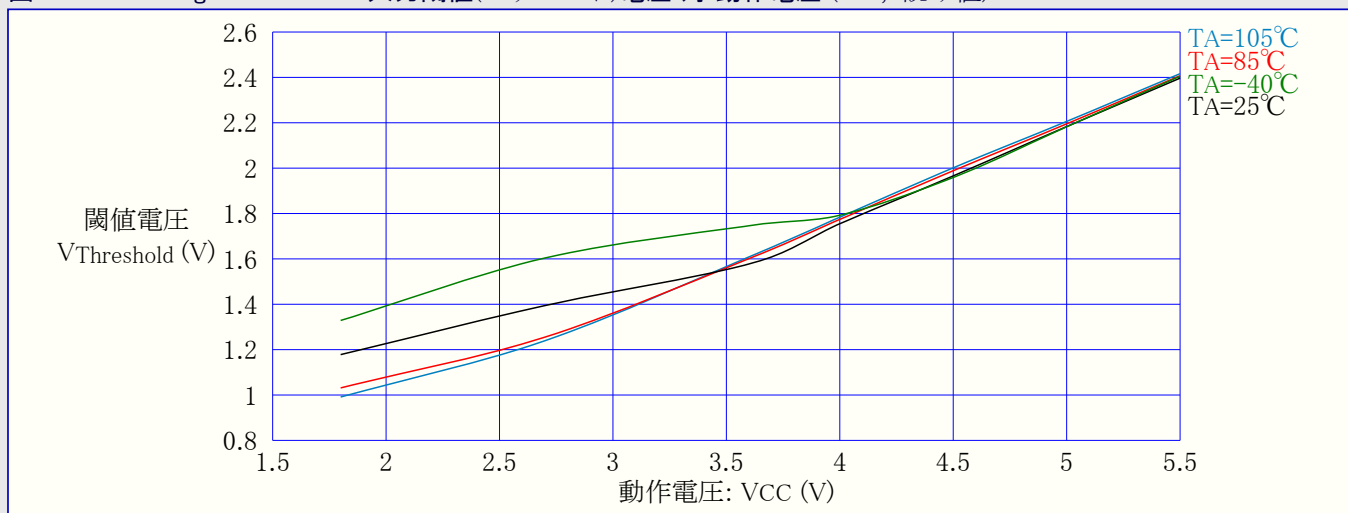
図31-359. ATmega328P:RESET入力閾値(スレッショールド)電圧 対 動作電圧 (VIH,1読み値)
