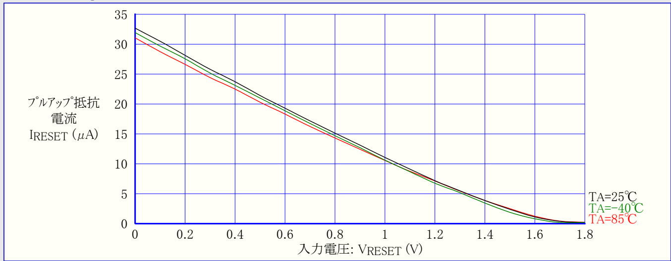
図31-18. ATmega48A: RESETプルアップ抵抗電流 対 入力電圧 (VCC=1.8V)
