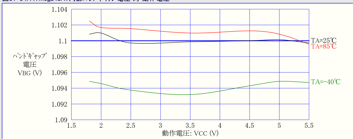
図31-34. ATmega48A: 内部バンドギャップ電圧 対 動作電圧
