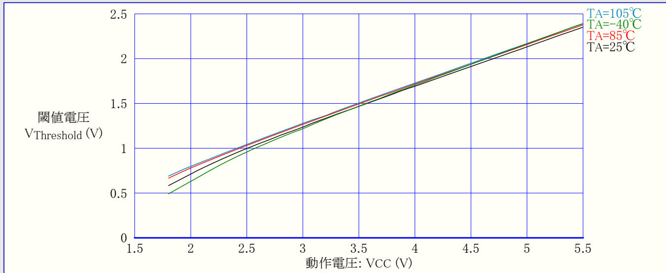
図32-71. ATmega88PA:I/Oピン入力閾値(スレッショルド)電圧 対 動作電圧 (VIL,0読み値)
