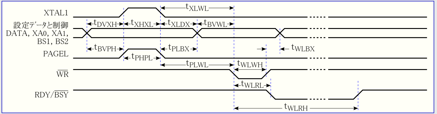
図29-7. 並列プログラミング タイミング (ページ設定での必要条件)
