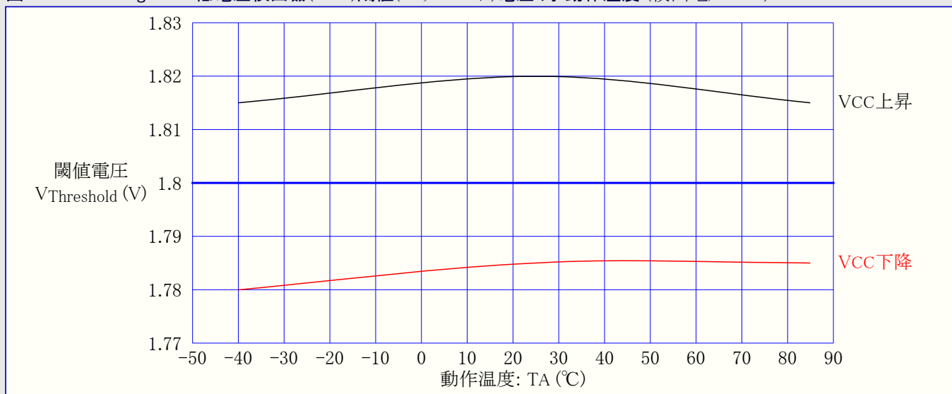
図31-125. ATmega88A: 低電圧検出器(BOD)閾値(スレッショルド)電圧 対 動作温度 (検出電圧1.8V)
