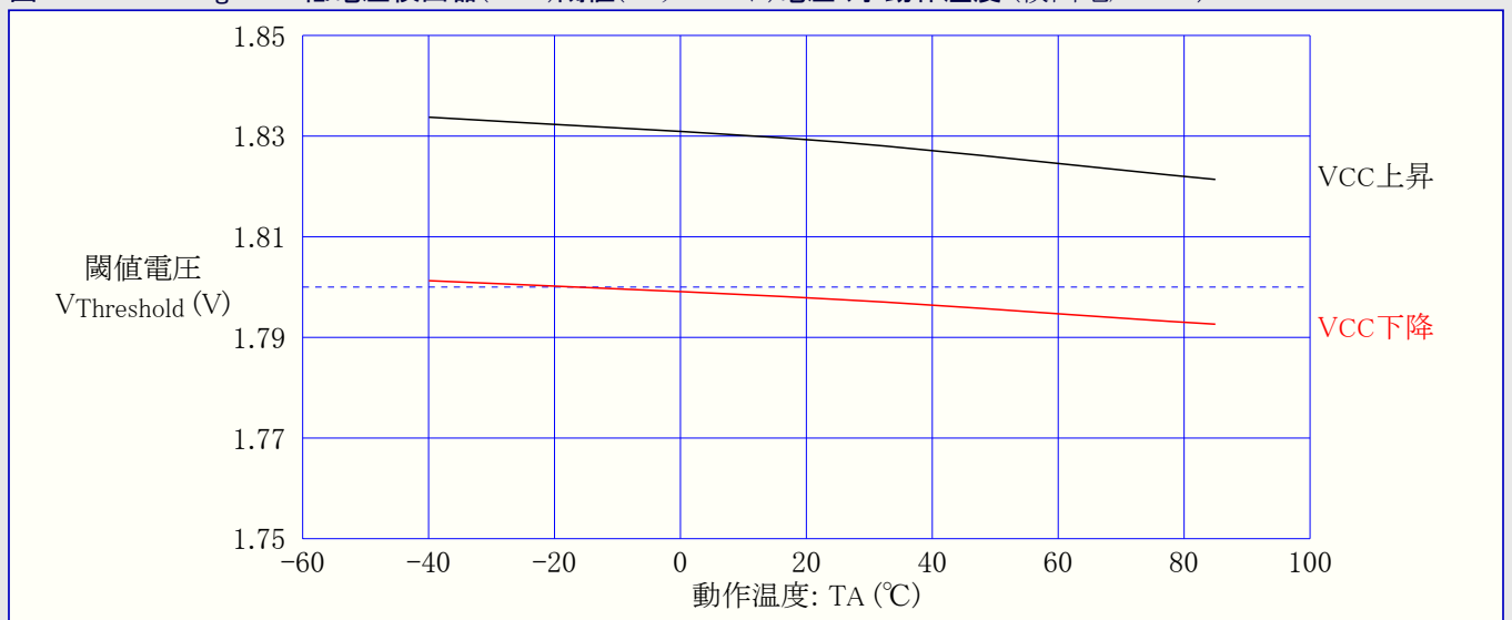
図31-315. ATmega328: 低電圧検出器(BOD)閾値(スレッショルド)電圧 対 動作温度 (検出電圧1.8V)
