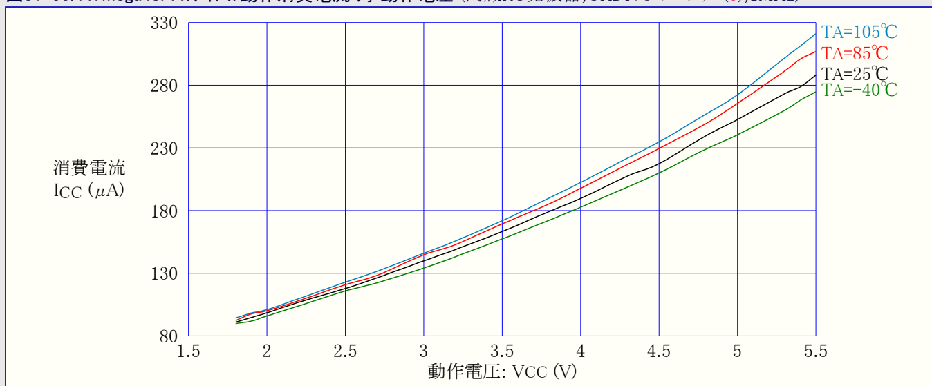
図31-56. ATmega48PA: アイドル動作消費電流 対 動作電圧 (内蔵RC発振器, CKDIV8=プログラム(0), 1MHz)
