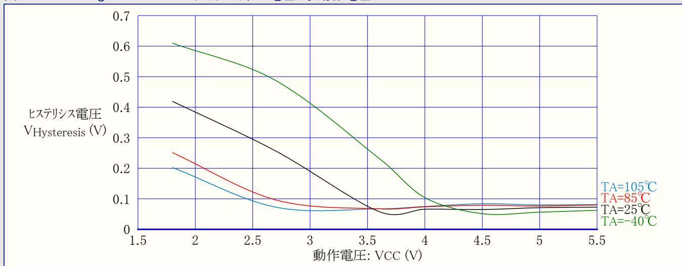
図32-121. ATmega168PA: RESET入力ヒステリシス電圧 対 動作電圧
