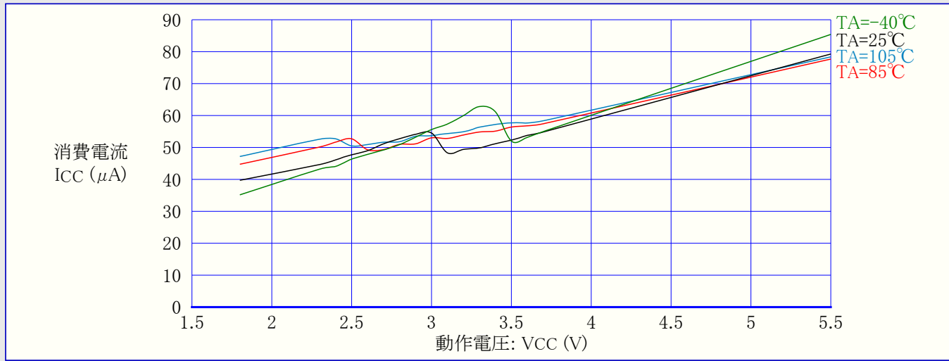
図32-86. ATmega88PA: アナログ比較器消費電流 対 動作電圧
