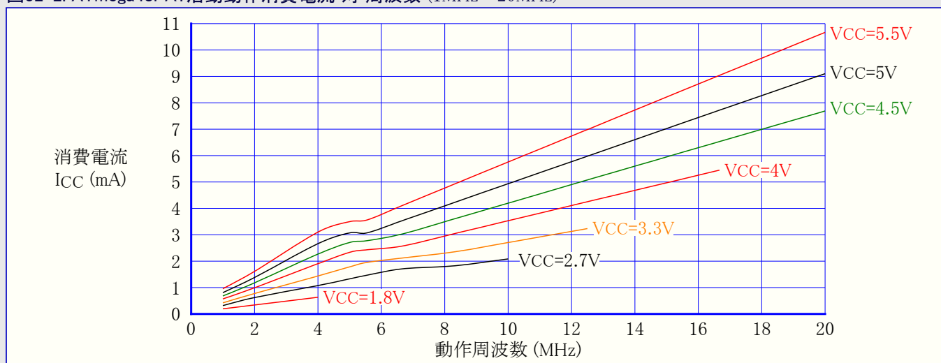
図32-2. ATmega48PA: 活動動作消費電流 対 周波数 (1MHz~20MHz)
