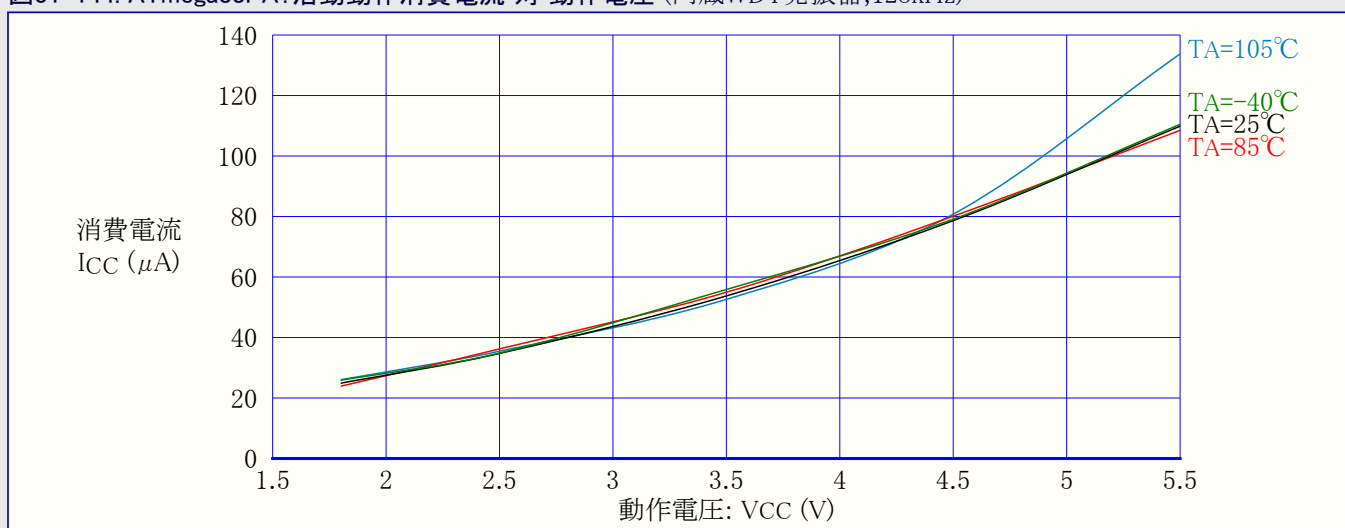
図31-144. ATmega88PA: 活動動作消費電流 対 動作電圧 (内蔵WDT発振器, 128kHz)
