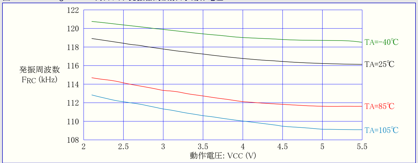
図31-273. ATmega168PA: ウォッチドッグ発振器周波数 対 動作電圧
