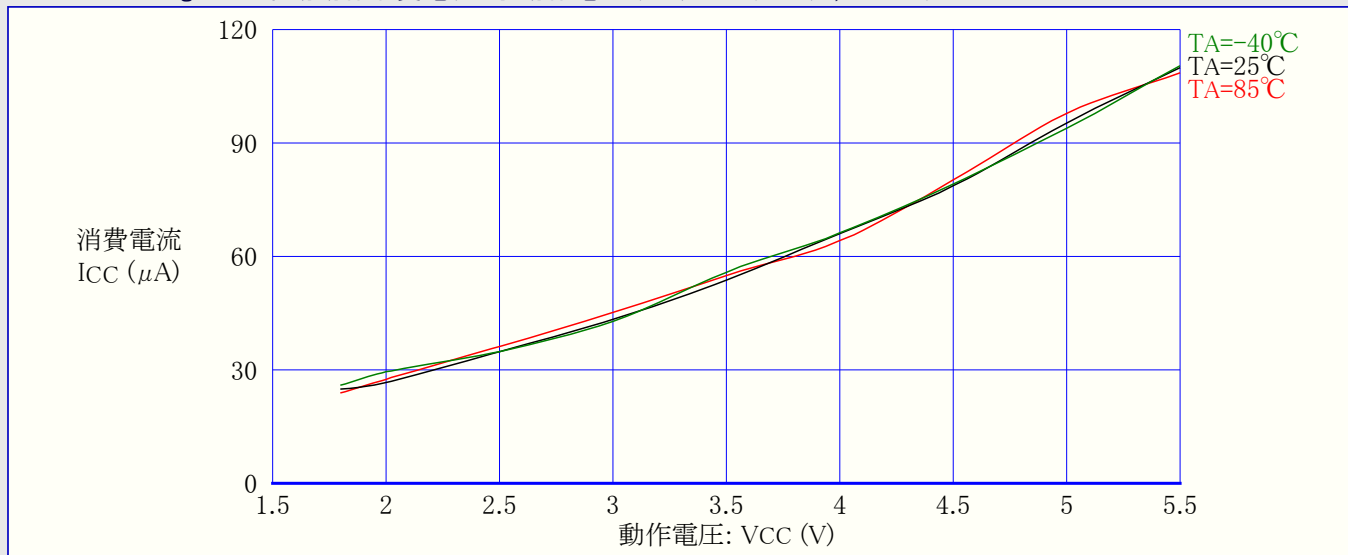
図31-97. ATmega88A: 活動動作消費電流 対 動作電圧 (内蔵WDT発振器, 128kHz)
