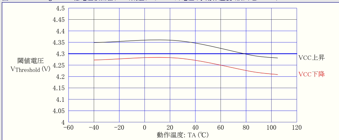
図31-174. ATmega88PA: 低電圧検出器(BOD)閾値(スレッショルド)電圧 対 動作温度 (検出電圧4.3V)
