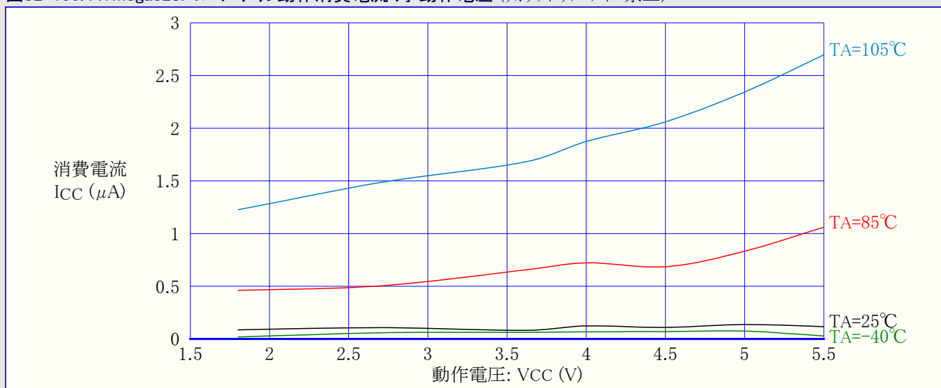
図32-150. ATmega328P:パワーダウン動作消費電流 対 動作電圧 (ウォッチドッグ タイマ禁止)
