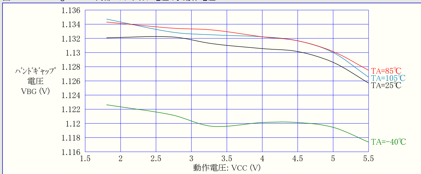
図32-126. ATmega168PA: 内部バンドギャップ電圧 対 動作電圧
