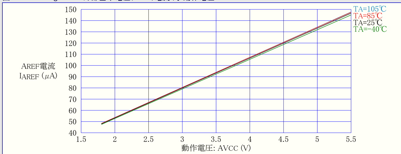
図32-40. ATmega48PA: 外部基準電圧(AREF)電流 対 動作電圧
