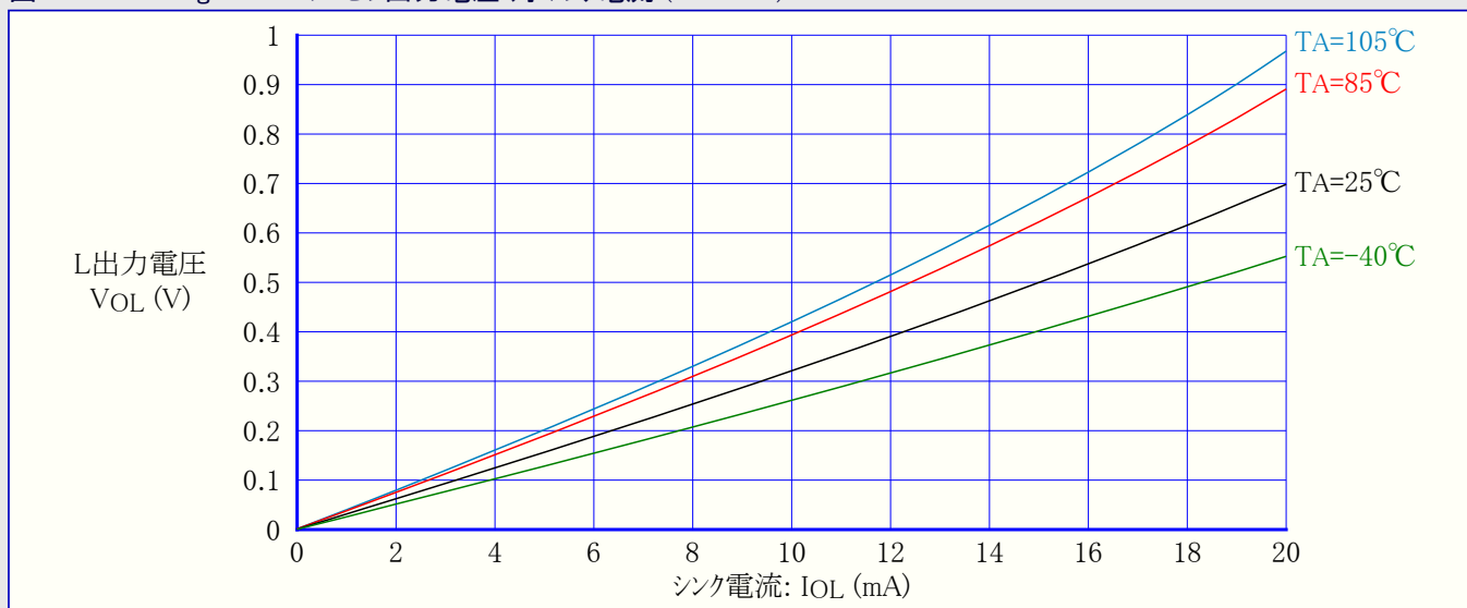
図31-68. ATmega48PA: I/Oピン出力電圧 対 シンク電流 (VCC=3V)
