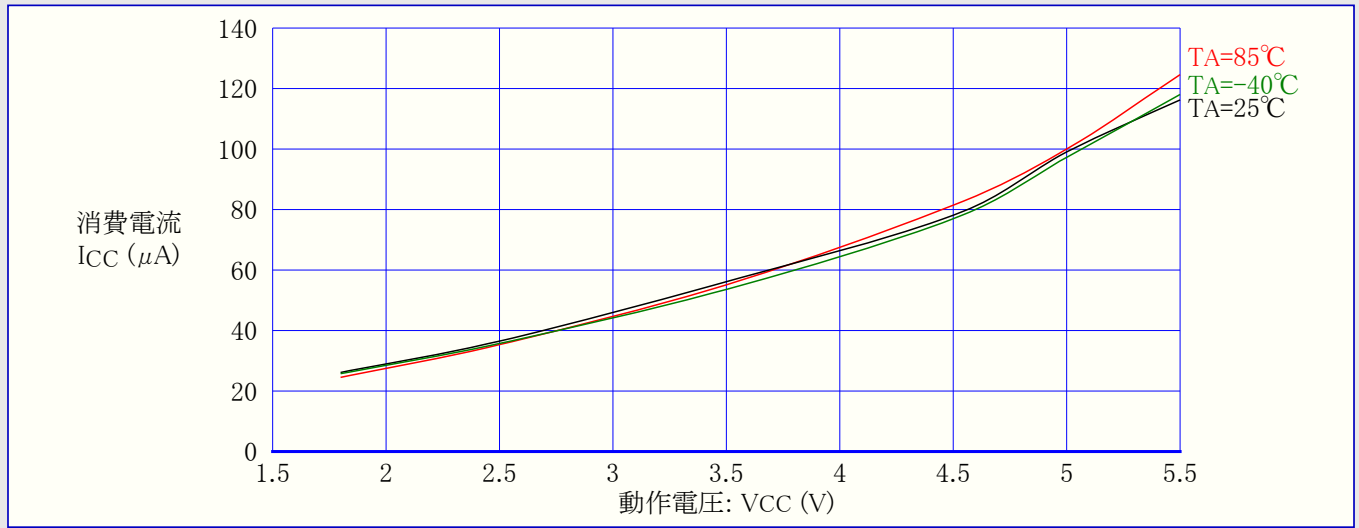
図31-4. ATmega48A: 活動動作消費電流 対 動作電圧 (内蔵RC発振器, CKDIV8=プログラム(0), 1MHz)
