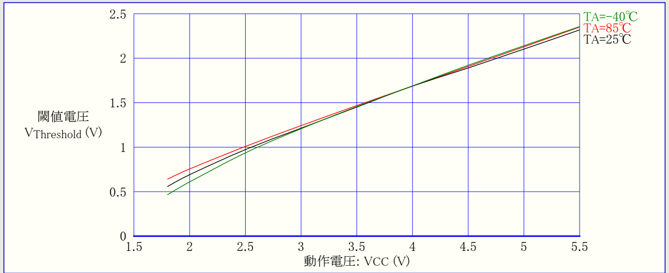
図31-27. ATmega48A:I/Oピン入力ヒステリシス電圧 対 動作電圧
