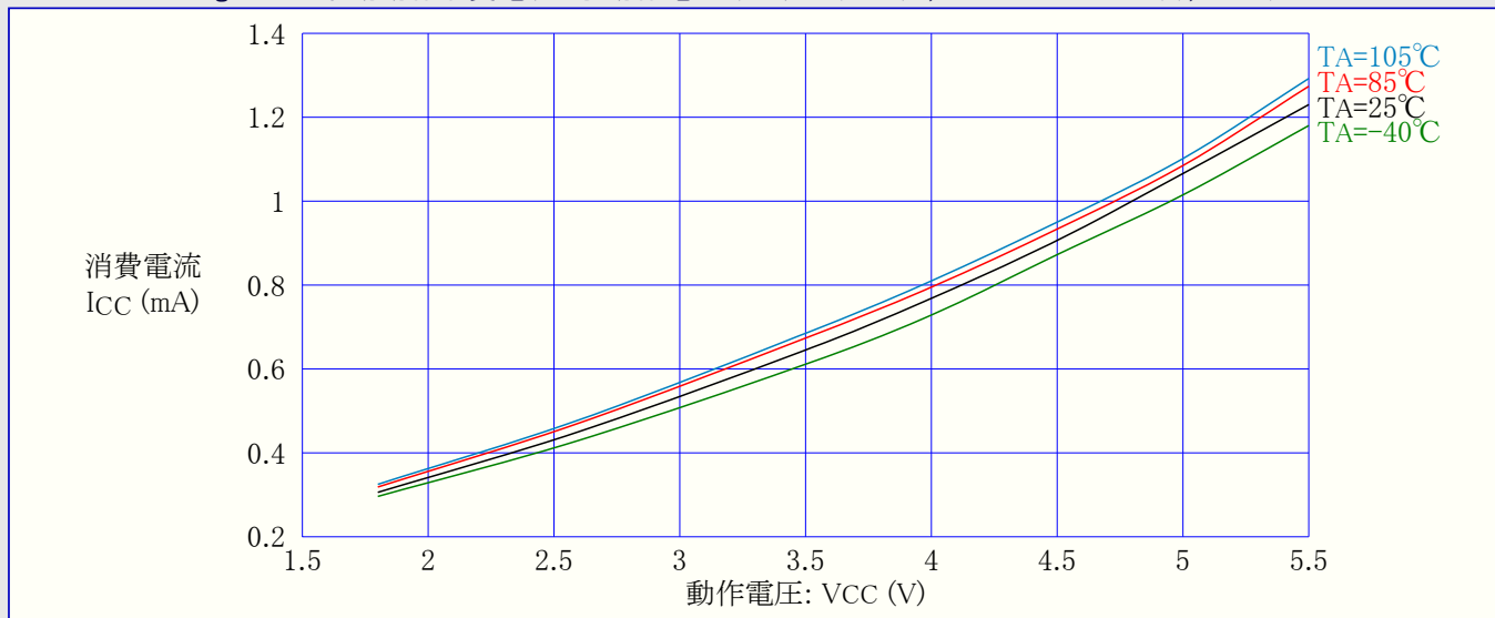
図31-335. ATmega328P: 活動動作消費電流 対 動作電圧 (内蔵RC発振器, CKDIV8=プログラム(0), 1MHz)
