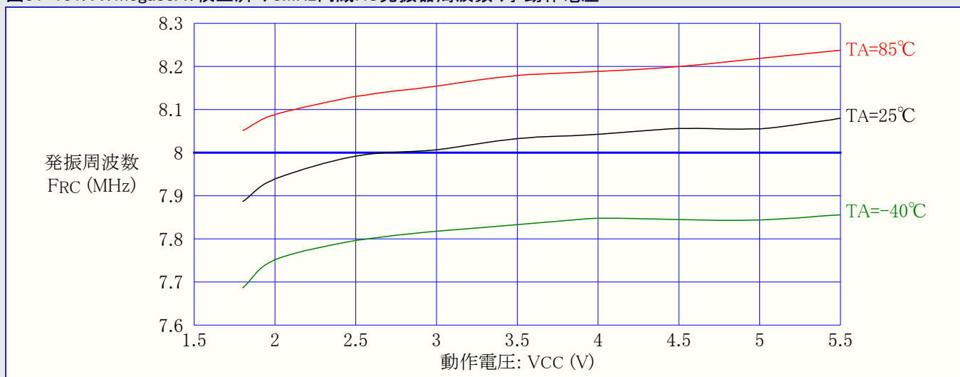
図31-131. ATmega88A: 校正済み8MHz内蔵RC発振器周波数 対 動作電圧
