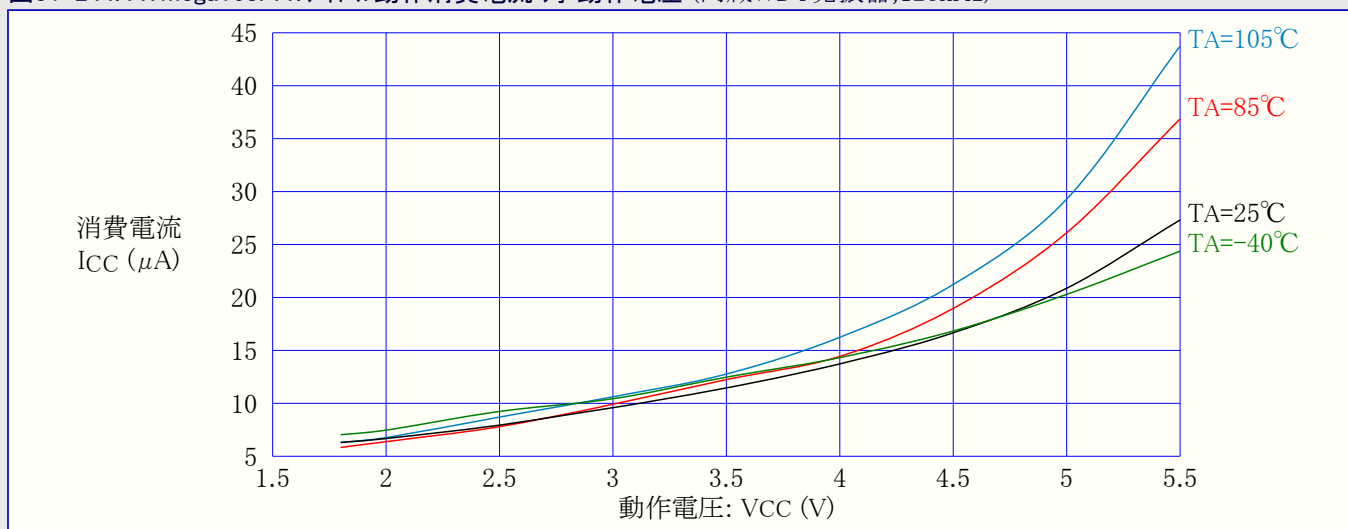
図31-244. ATmega168PA: アイドル動作消費電流 対 動作電圧 (内蔵WDT発振器, 128kHz)
