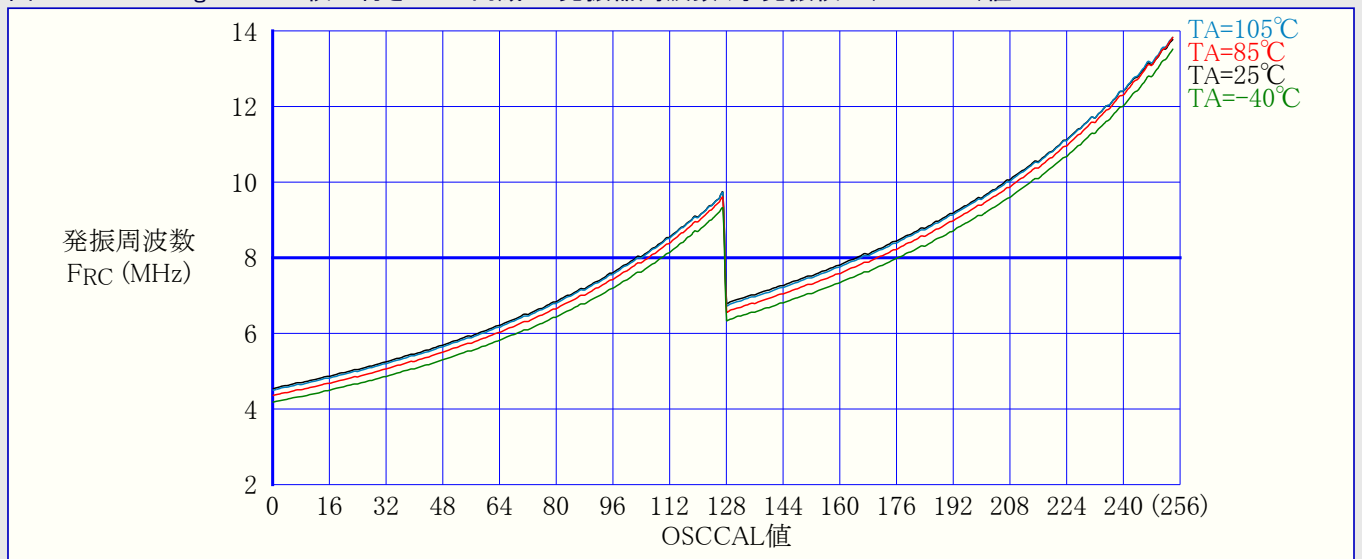
図31-276. ATmega168PA: 校正付き8MHz内蔵RC発振器周波数 対 発振校正(OSCCAL)値
