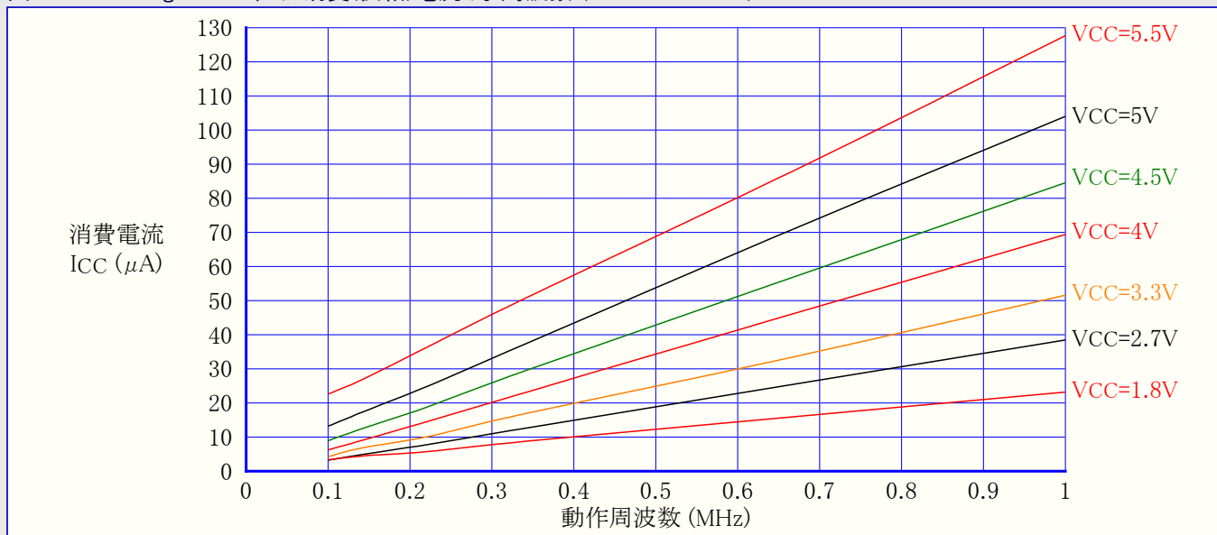
図31-92. ATmega48PA:リセット消費(供給)電流 対 周波数 (100kHz~1MHz)
