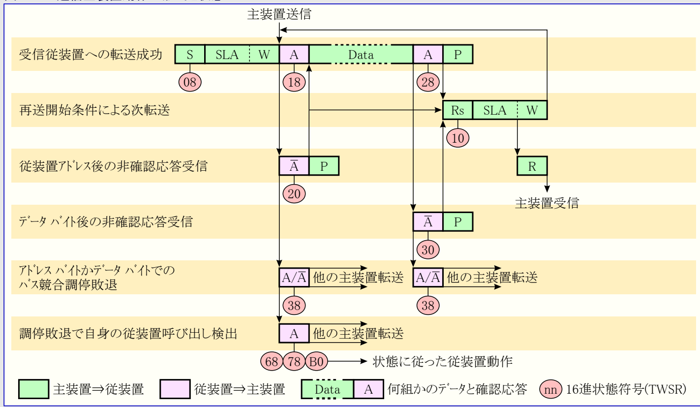
図22-12. 送信主装置動作の形式と状態
