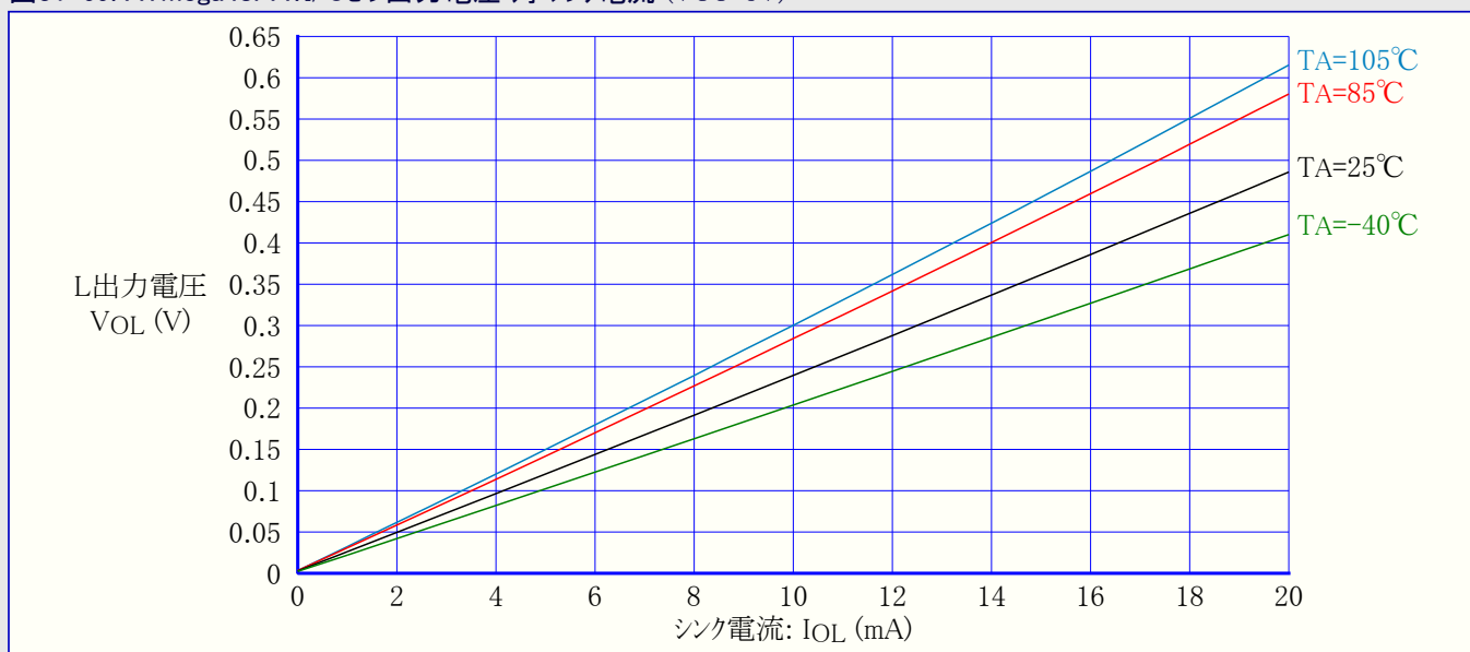
図31-69. ATmega48PA: I/Oピン出力電圧 対 シンク電流 (VCC=5V)
