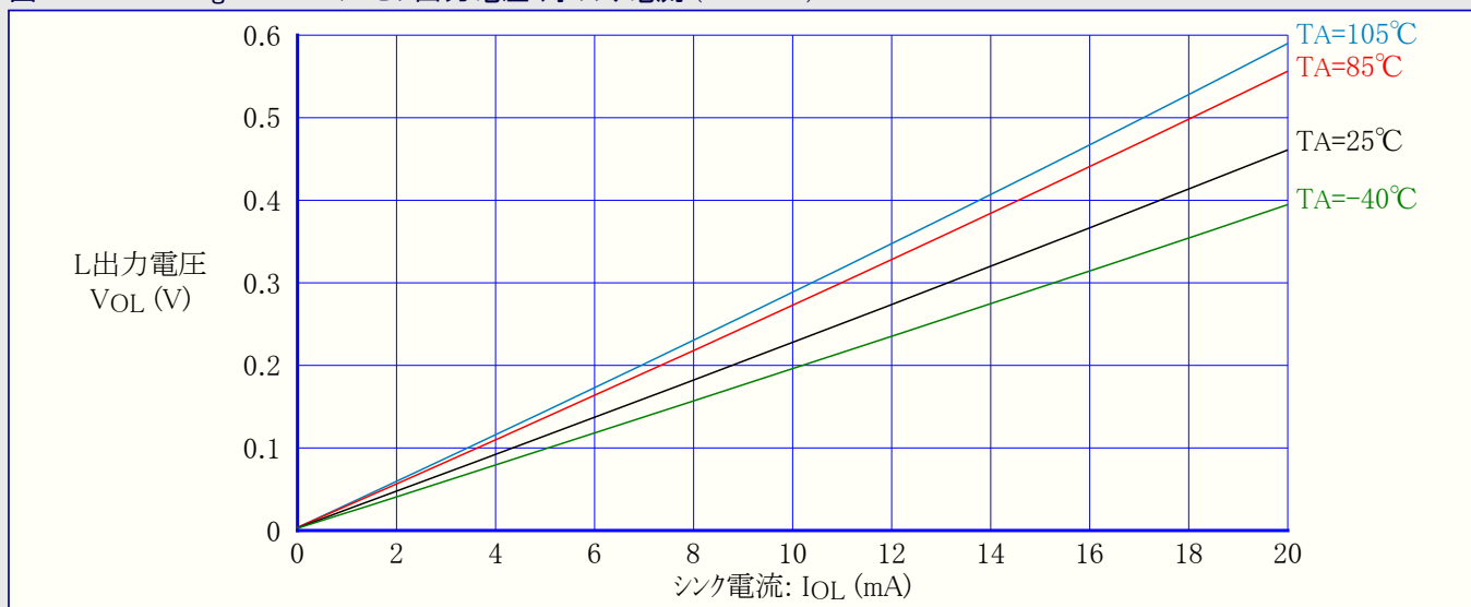
図31-258. ATmega168PA: I/Oピン出力電圧 対 シンク電流 (VCC=5V)
