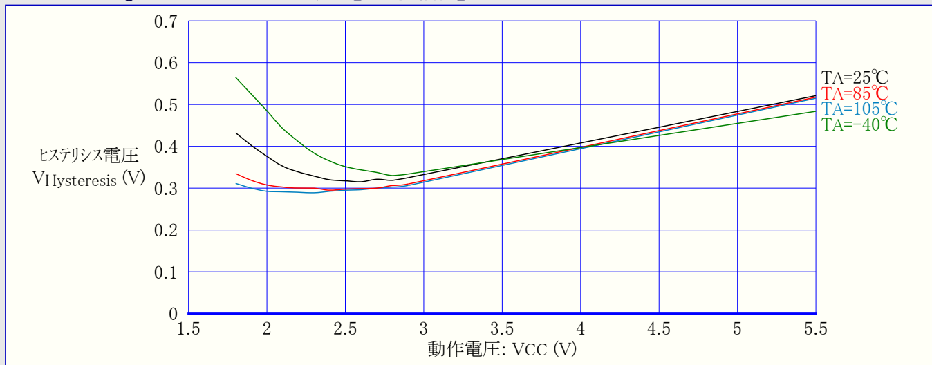
図32-72. ATmega88PA:I/Oピン入力ヒステリシス電圧 対 動作電圧
