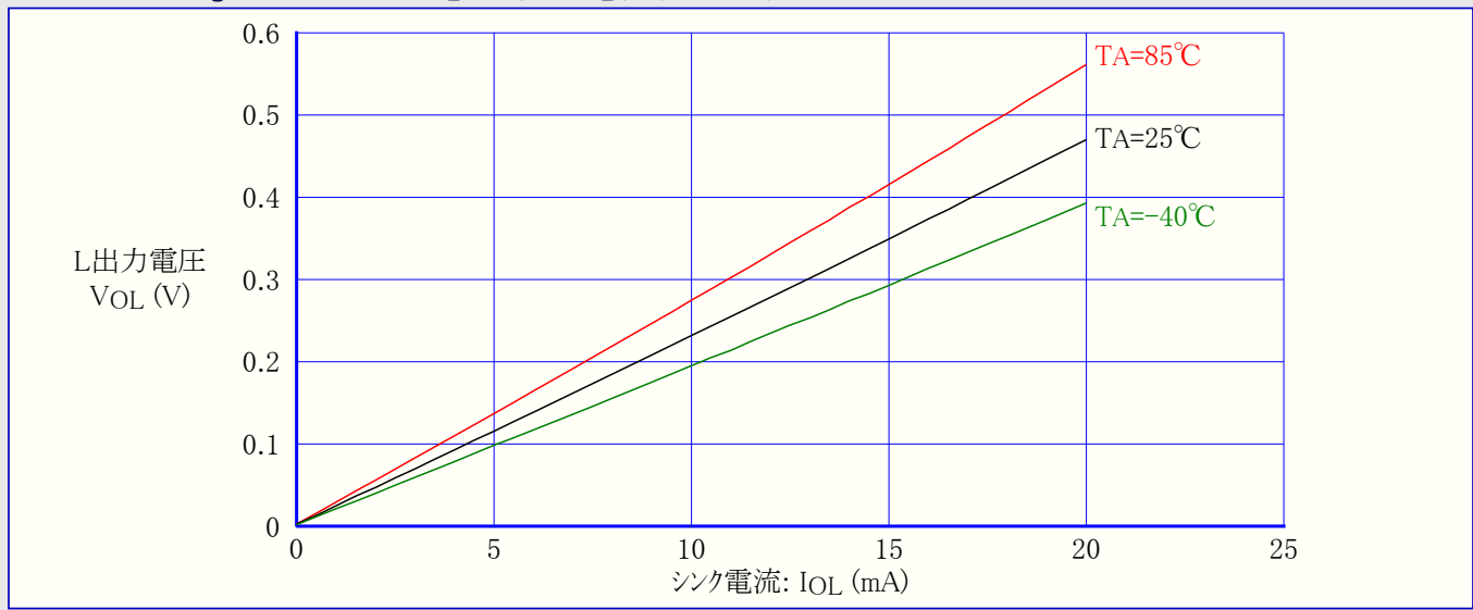
図31-306. ATmega328: I/Oピン出力電圧 対 シンク電流 (VCC=5V)
