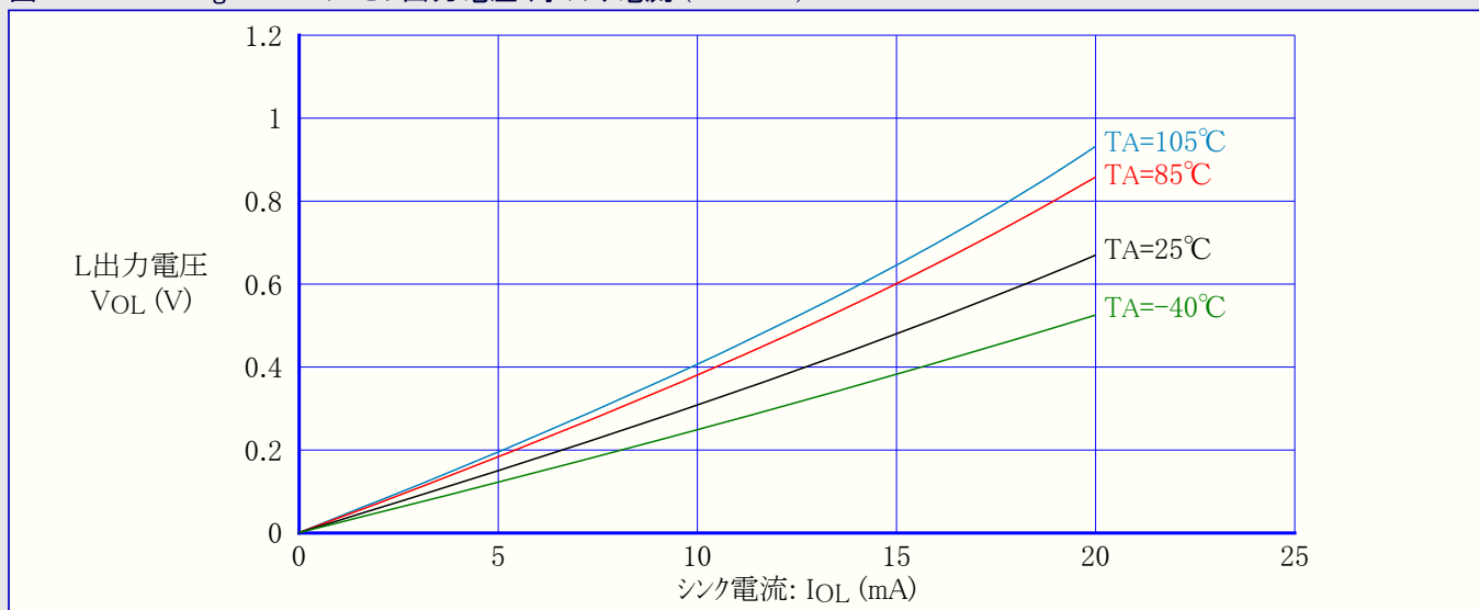
図31-162. ATmega88PA:I/Oピン出力電圧 対 シンク電流 (VCC=3V)
