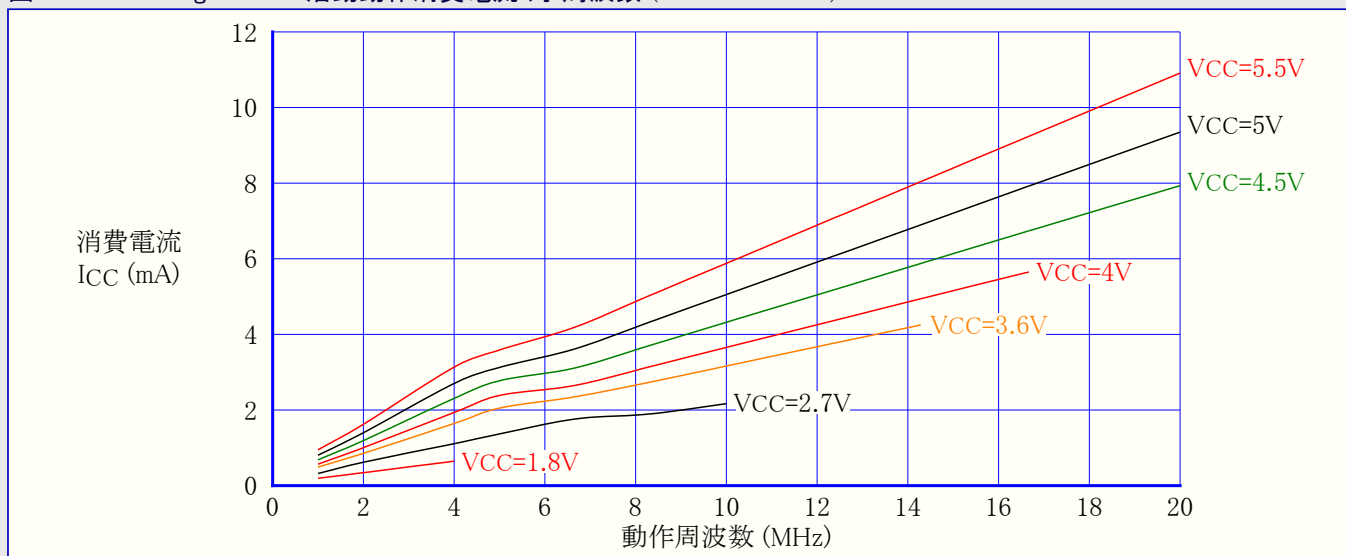
図31-238. ATmega168PA: 活動動作消費電流 対 周波数 (1MHz~20MHz)
