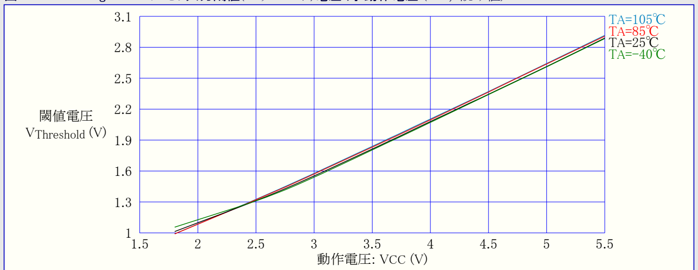
図31-356. ATmega328P:I/Oピン入力閾値(スレッシュホールド)電圧 対 動作電圧 ( V_{IH,1} 読み値)
