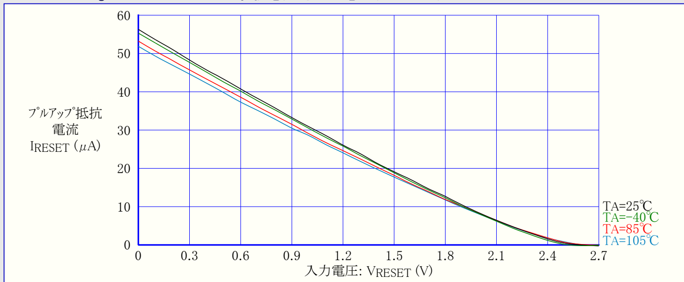
図32-110. ATmega168PA: RESETプルアップ抵抗電流 対 入力電圧 (VCC=2.7V)
