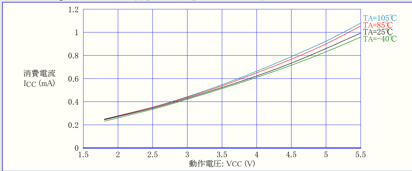
図31-151. ATmega88PA:アイドル動作消費電流 対 動作電圧 (内蔵RC発振器,8MHz)
