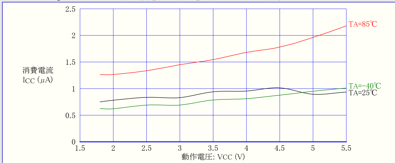
図31-202. ATmega168A: パワーセーブ動作消費電流 対 動作電圧 (ウォッチドッグ タイマ禁止, 32kHz クリスタル用発振器走行)
