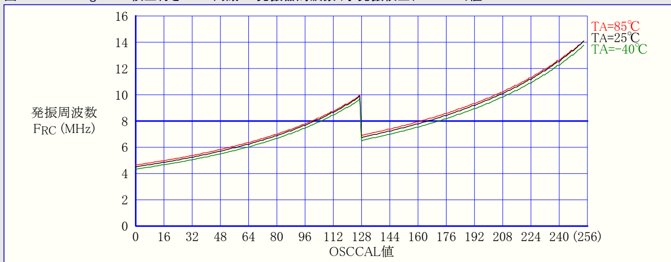
図31-39. ATmega48A: 校正付き8MHz内蔵RC発振器周波数 対 発振校正(OSCCAL)値
