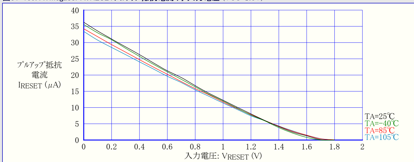
図31-159. ATmega88PA:RESETプルアップ抵抗電流 対 入力電圧 (VCC=1.8V)
