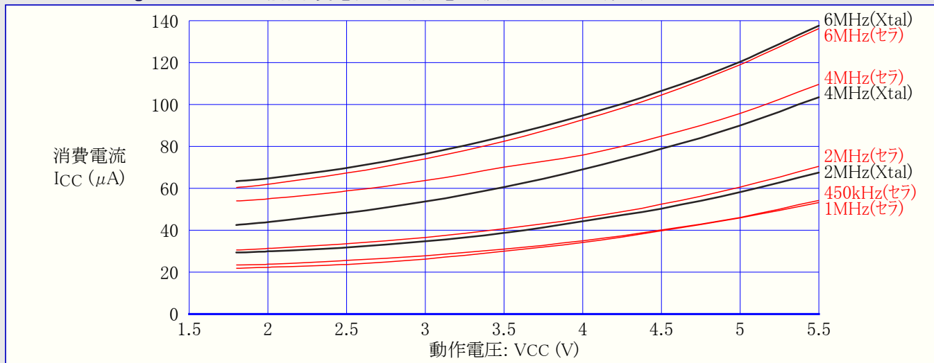
図31-203. ATmega168A:スタンバイ動作消費電流 対 動作電圧 (ウォッチドッグ タイマ禁止)
