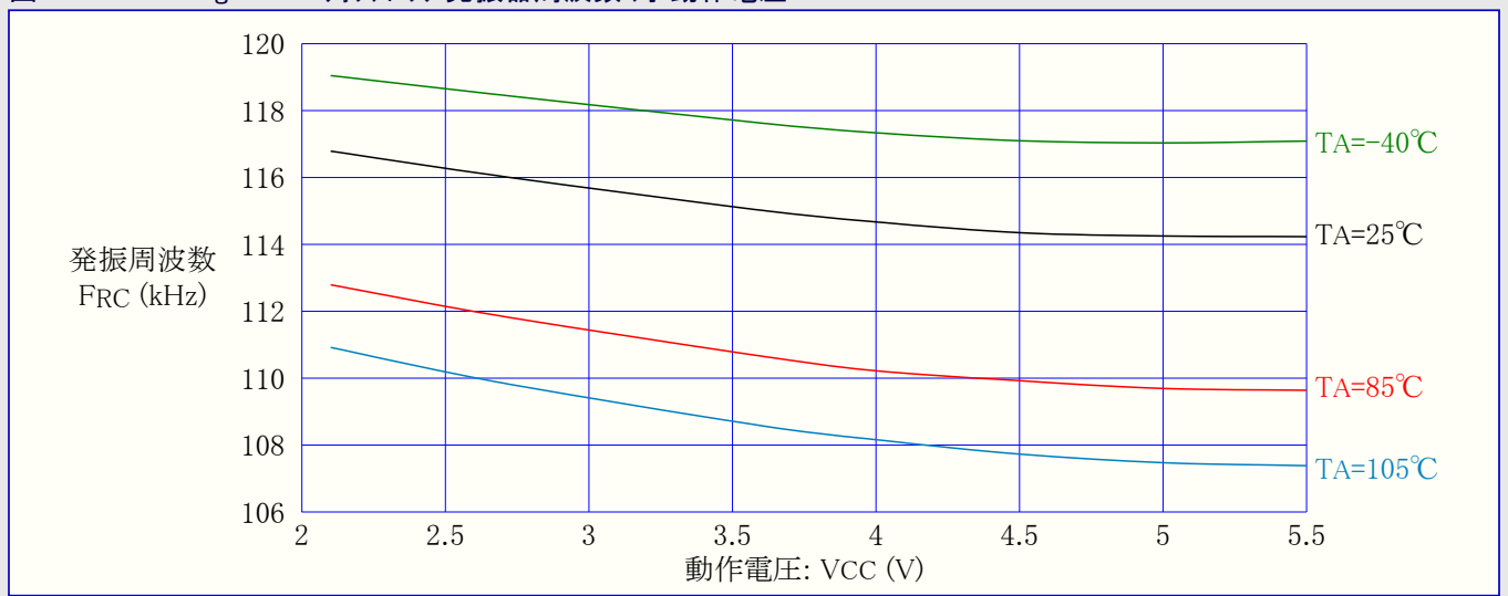
図32-175. ATmega328P: ウォッチドッグ発振器周波数 対 動作電圧
