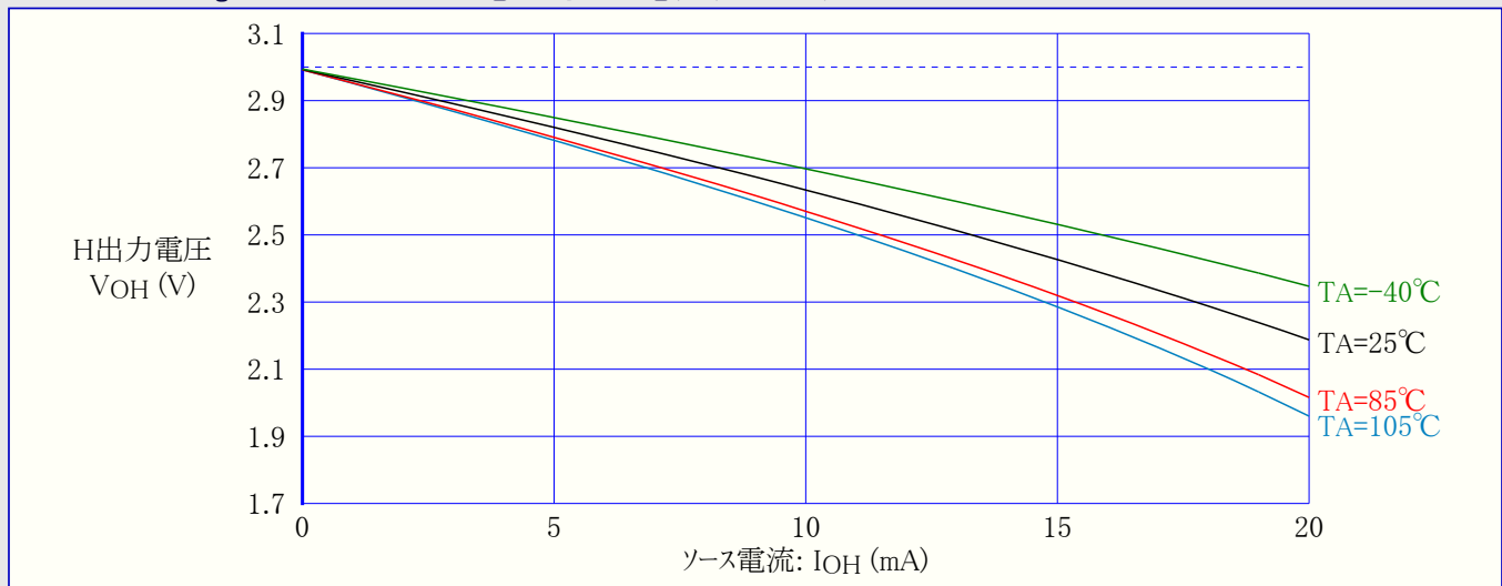
図32-114. ATmega168PA:I/Oピン出力電圧 対 ソース電流 (VCC=3V)
