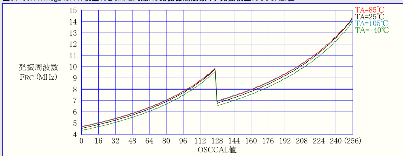
図31-86. ATmega48PA: 校正付き8MHz内蔵RC発振器周波数 対 発振校正(OSCCAL)値
