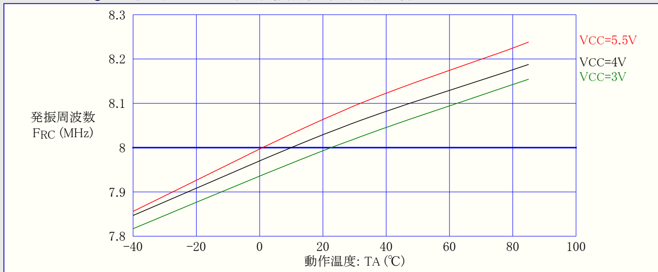
図31-132. ATmega88A: 校正済み8MHz内蔵RC発振器周波数 対 動作温度
