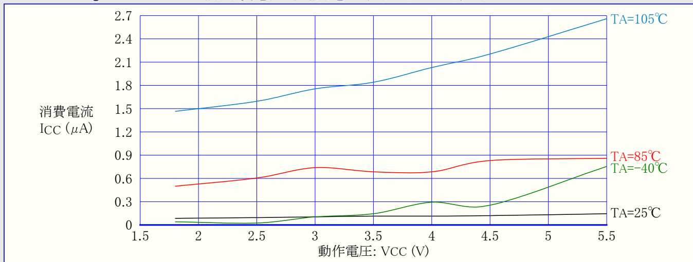
図32-11. ATmega48PA:パワーダウン動作消費電流 対 動作電圧 (ウォッチドッグ タイマ禁止)
