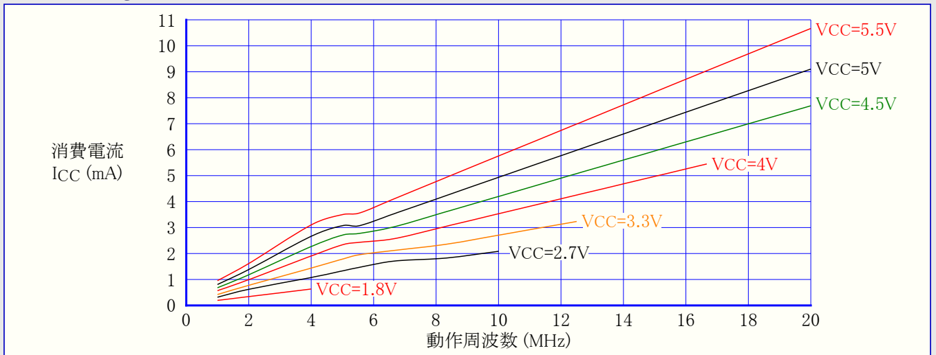
図31-49. ATmega48PA: 活動動作消費電流 対 周波数 (1MHz~20MHz)
