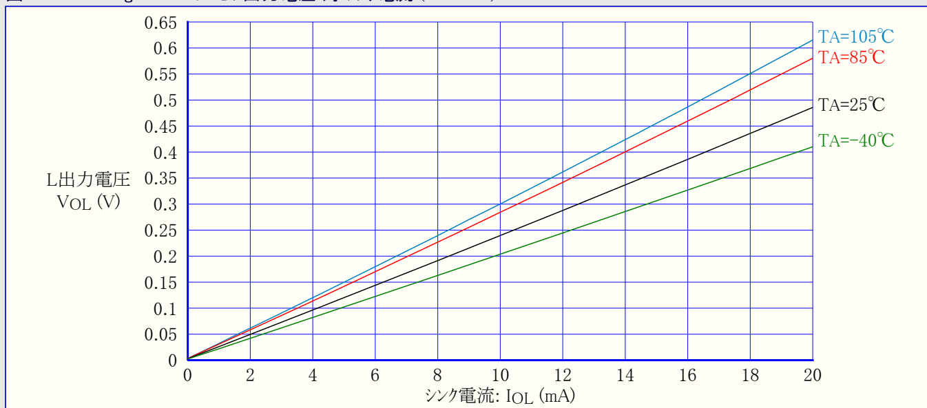
図32-22. ATmega48PA: I/Oピン出力電圧 対 シンク電流 (VCC=5V)
