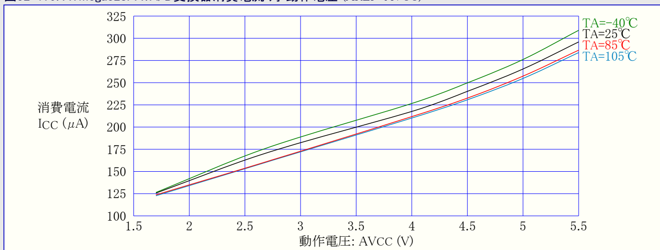
図32-179. ATmega328PA: A/D変換器消費電流 対 動作電圧 (AREF=AVCC)
