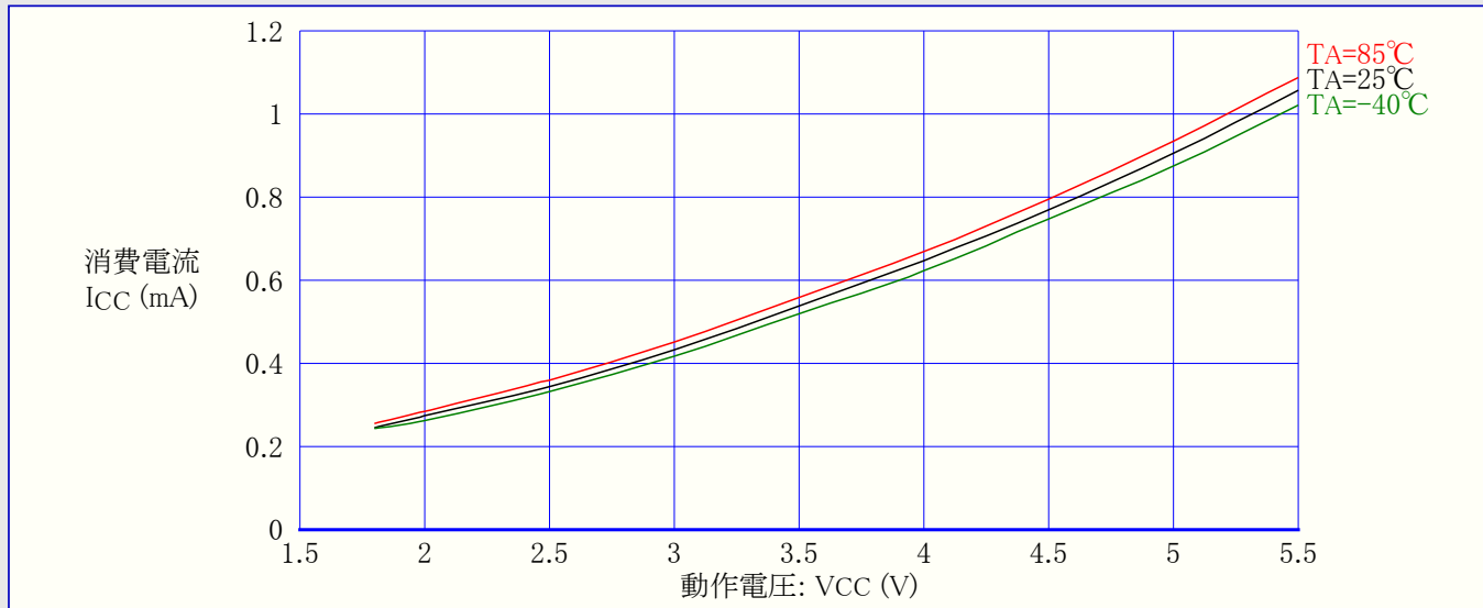
図31-193. ATmega168A: 活動動作消費電流 対 動作電圧 (内蔵RC発振器, CKDIV8=プログラム(0), 1MHz)
