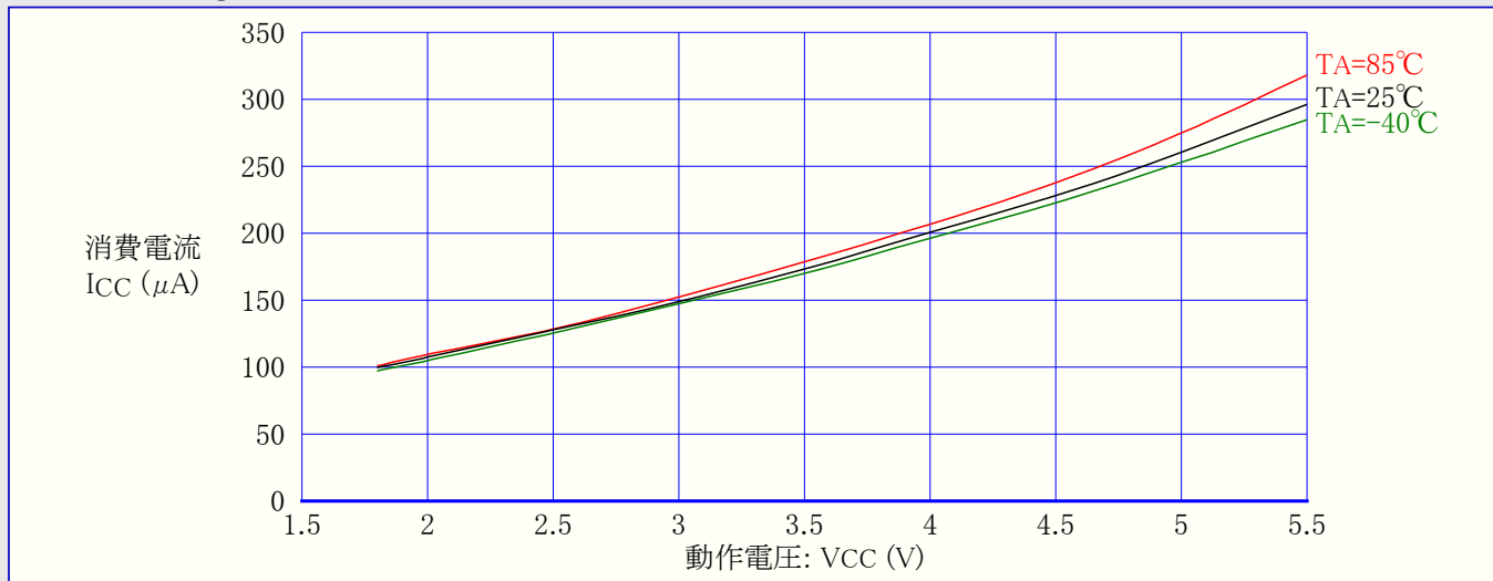
図31-103. ATmega88A: アイドル動作消費電流 対 動作電圧 (内蔵RC発振器, CKDIV8=プログラム(0), 1MHz)
