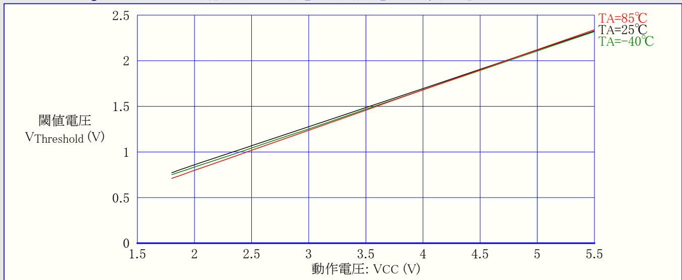
図31-29. ATmega48A: RESET入力閾値(スレッショルド)電圧 対 動作電圧 (VIL,0読み値)
