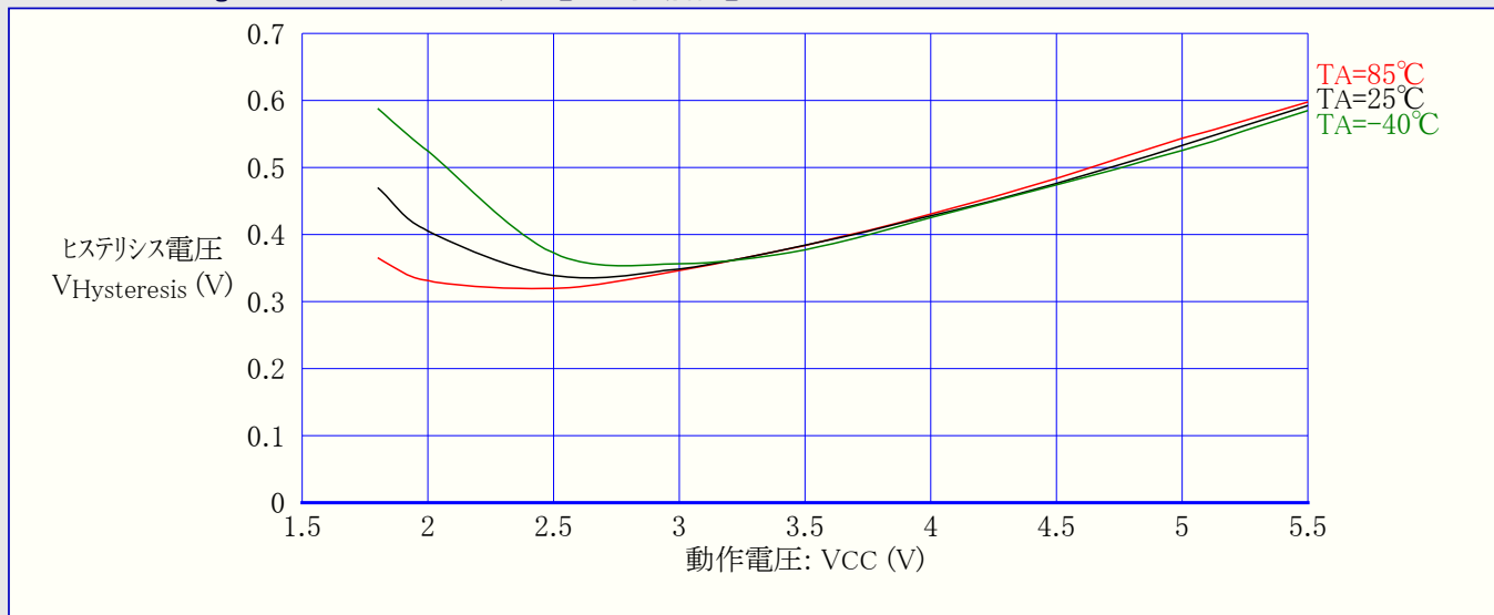
図31-311. ATmega328:I/Oピン入力ヒステリシス電圧 対 動作電圧
