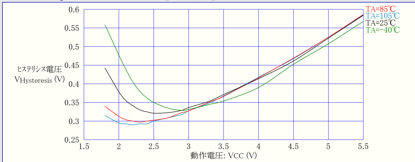
図31-263. ATmega168PA:I/Oピン入力ヒステリシス電圧 対 動作電圧
