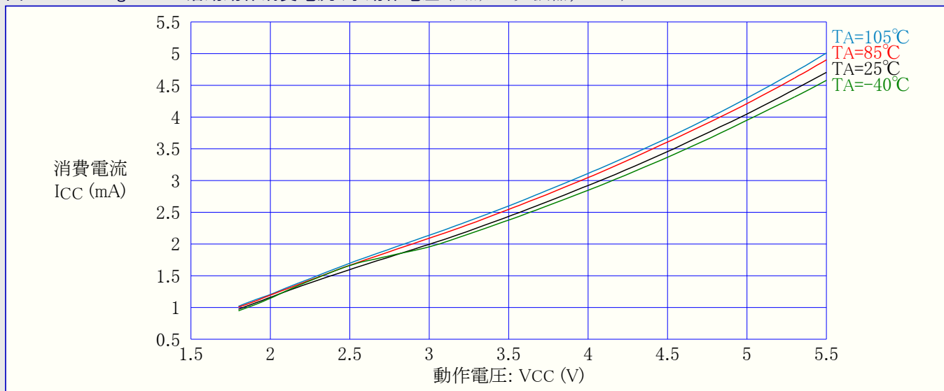
図32-5. ATmega48PA: 活動動作消費電流 対 動作電圧 (内蔵RC発振器, 8MHz)
