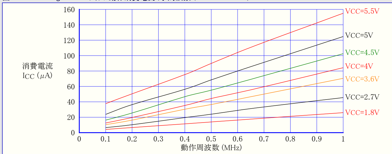
図31-242. ATmega168PA: アイドル動作消費電流 対 周波数 (100kHz~1MHz)
