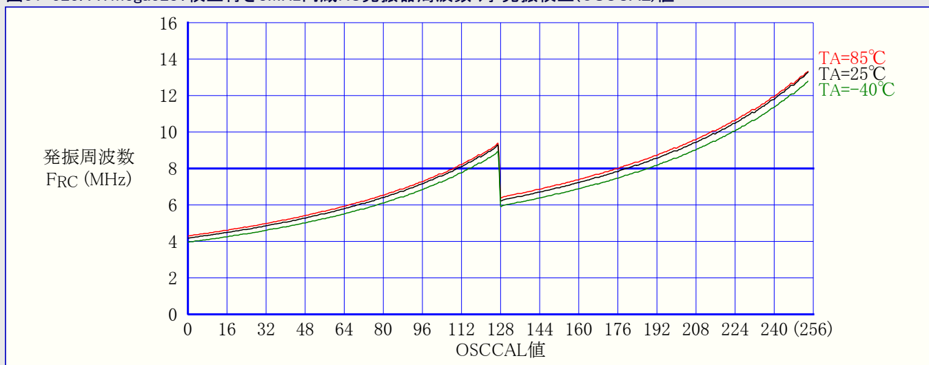
図31-323. ATmega328: 校正付き8MHz内蔵RC発振器周波数 対 発振校正(OSCCAL)値
