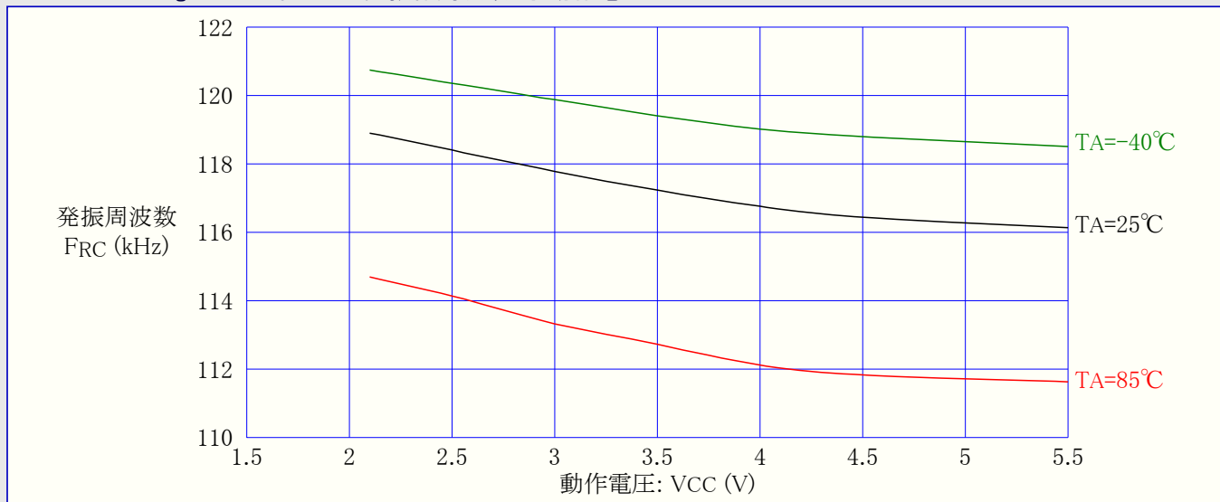
図31-225. ATmega168A: ウォッチドッグ発振器周波数 対 動作電圧
