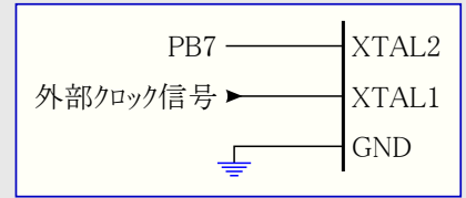
図9-4. 外部クロック信号駆動接続図
