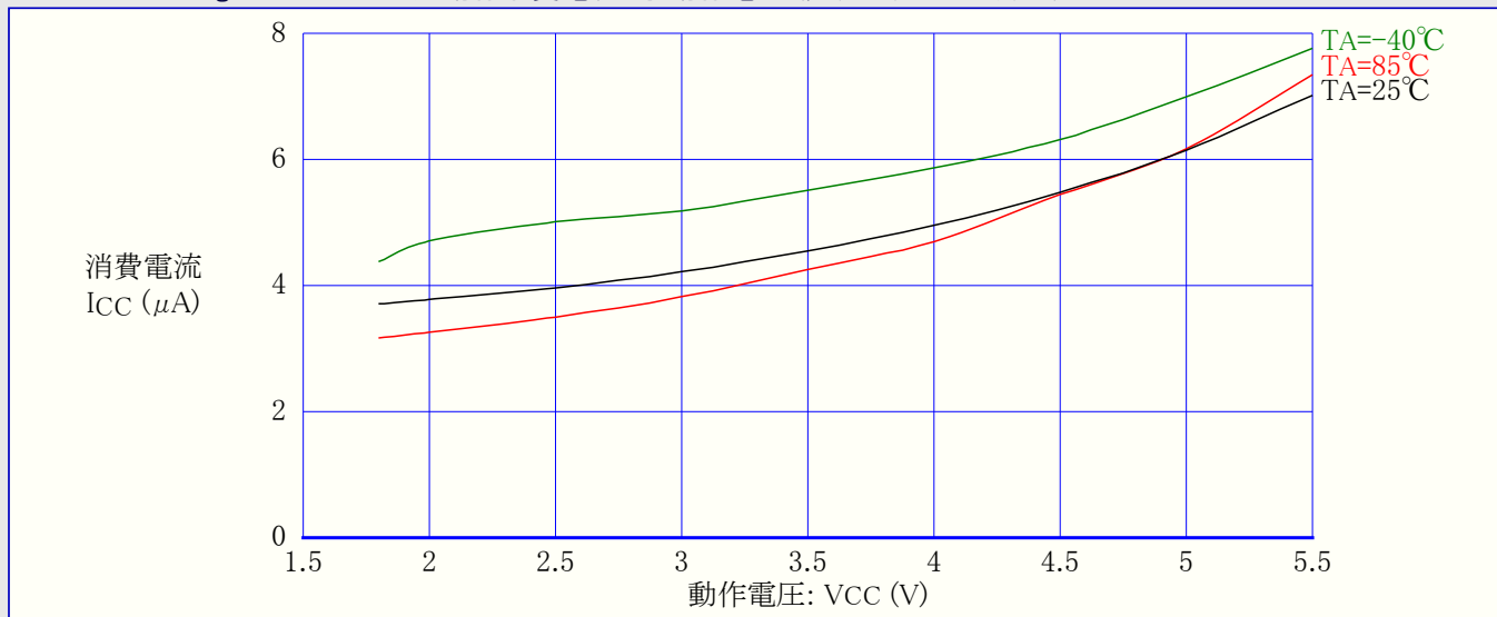
図31-201. ATmega168A: パワーダウン動作消費電流 対 動作電圧 (ウォッチドッグ タイマ許可)
