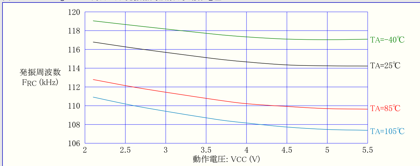
図31-367. ATmega328P: ウォッチドッグ発振器周波数 対 動作電圧
