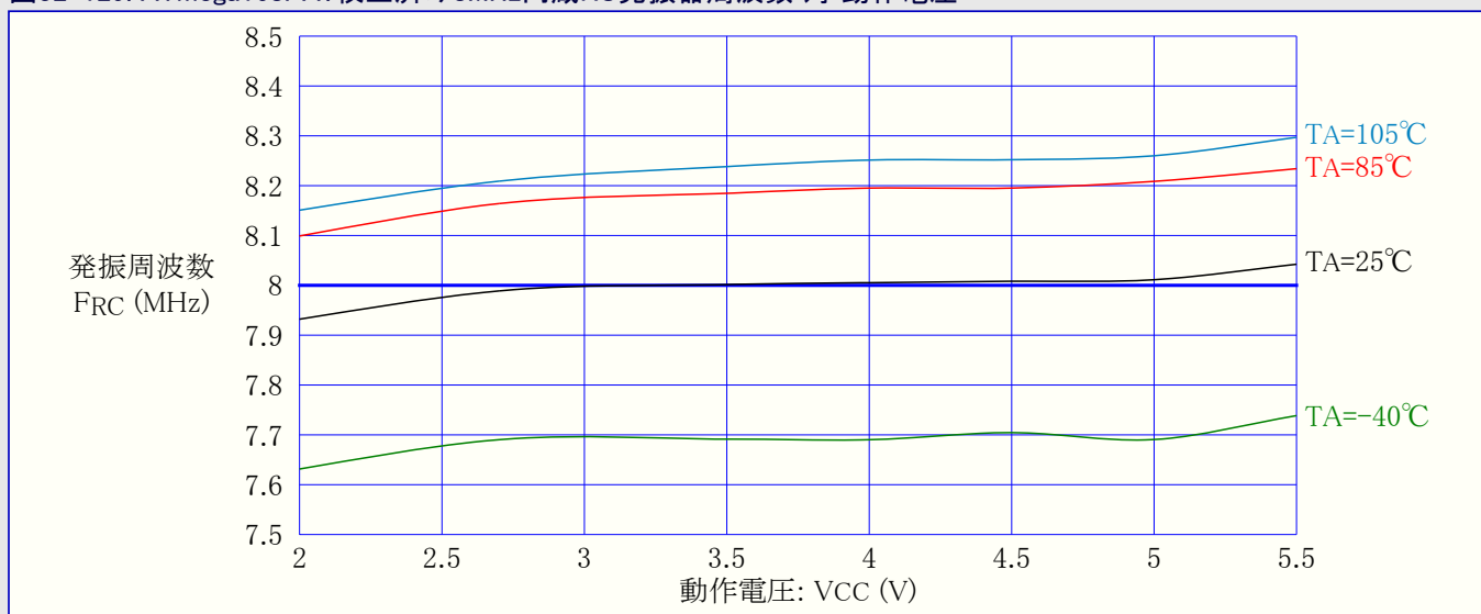
図32-129. ATmega168PA: 校正済み8MHz内蔵RC発振器周波数 対 動作電圧
