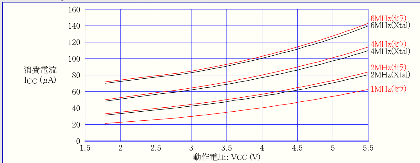
図31-345. ATmega328P:スタンバイ動作消費電流 対 動作電圧 (ウォッチドッグ タイマ禁止)
