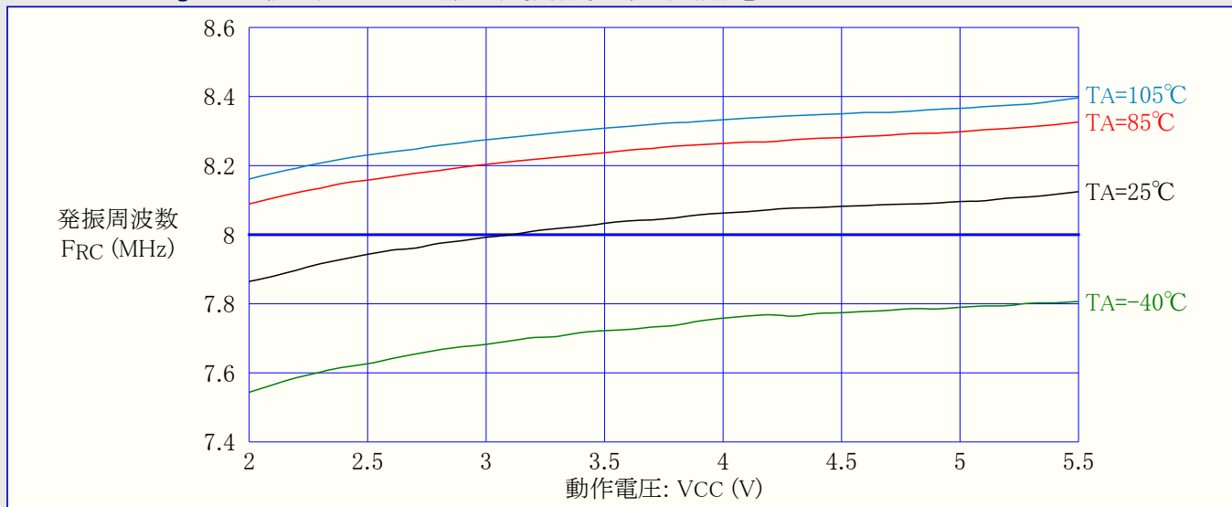
図32-176. ATmega328P: 校正済み8MHz内蔵RC発振器周波数 対 動作電圧
