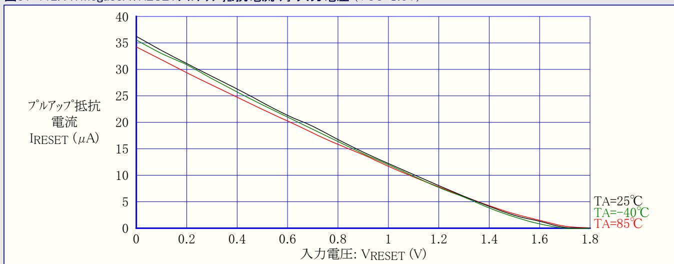
図31-112. ATmega88A:RESETプルアップ抵抗電流 対 入力電圧 (VCC=1.8V)
