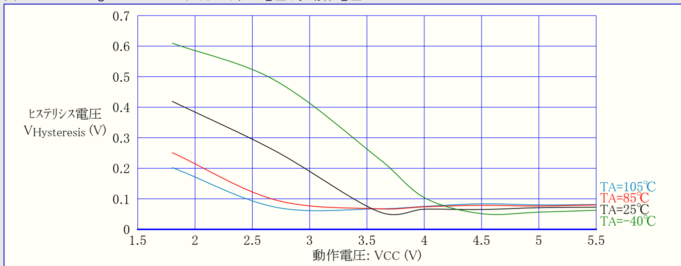
図32-169. ATmega328P: RESET入力ヒステリシス電圧 対 動作電圧
