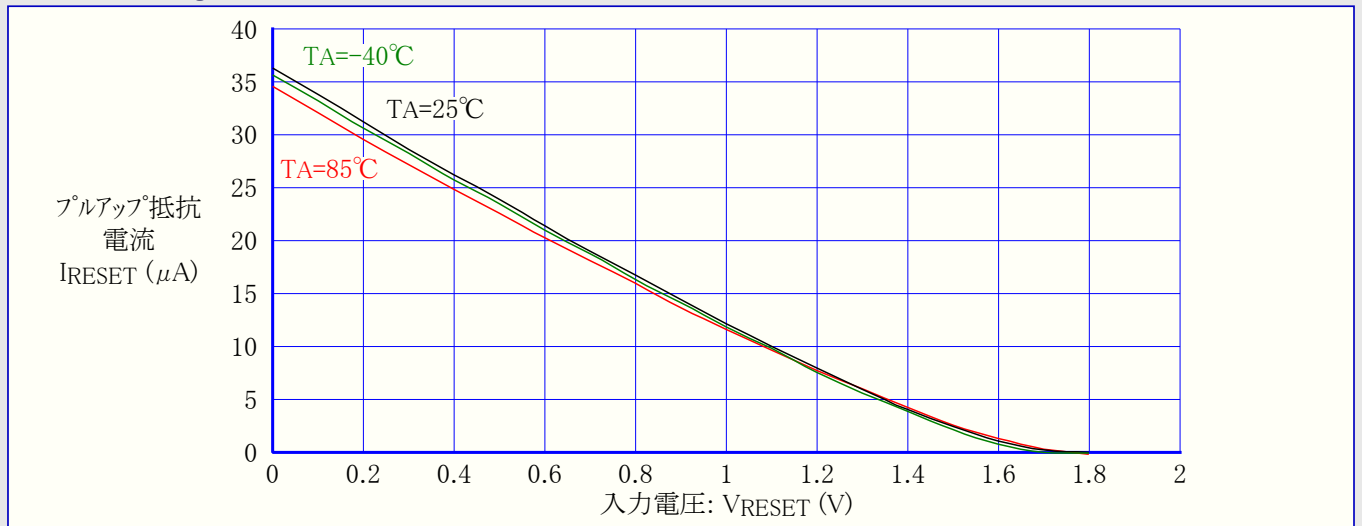
図31-302. ATmega328: RESETプルアップ抵抗電流 対 入力電圧 (VCC=1.8V)
