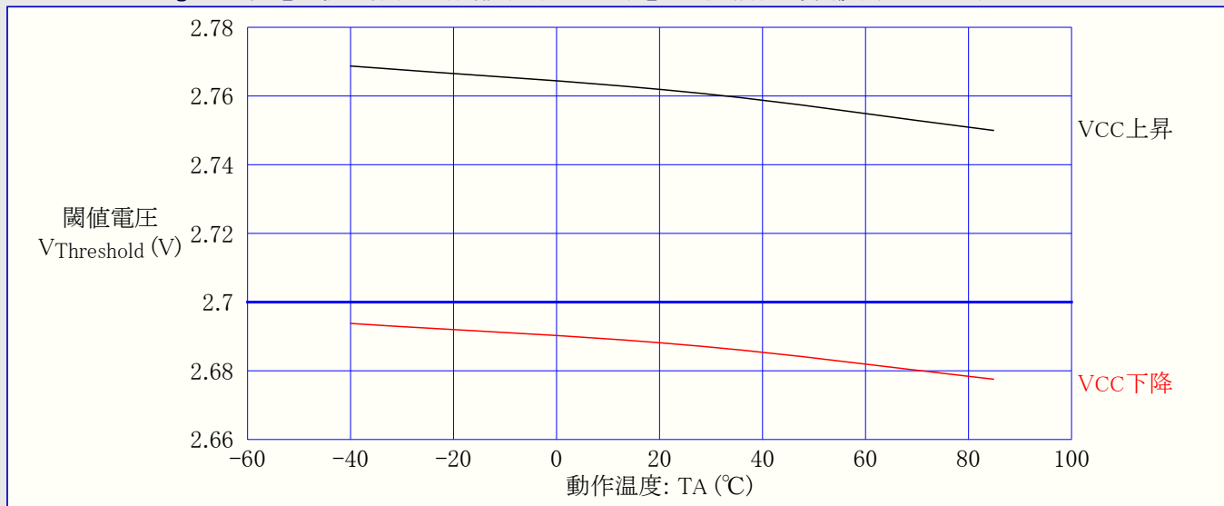
図31-316. ATmega328: 低電圧検出器(BOD)閾値(スレッシュホールド)電圧 対 動作温度 (検出電圧2.7V)
