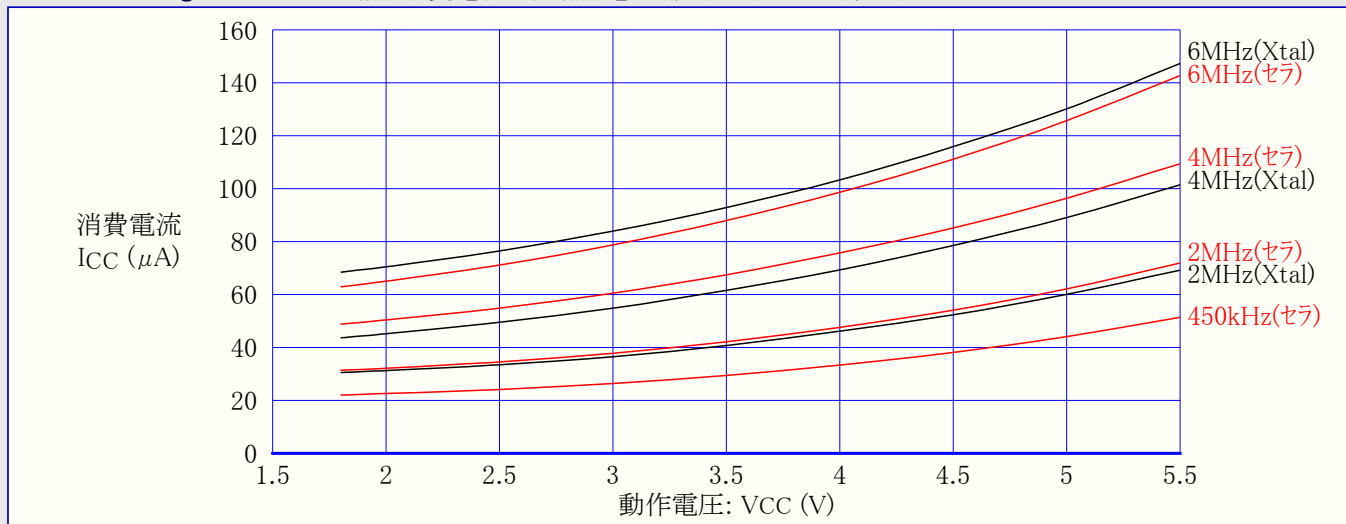
図31-14. ATmega48A:スタンバイ動作消費電流 対 動作電圧 (ウォッチドッグ タイマ禁止)
