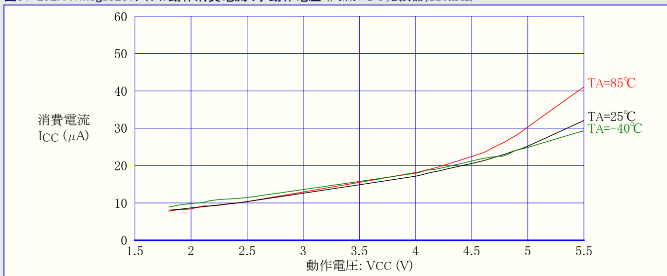
図31-292. ATmega328:アイドル動作消費電流 対 動作電圧 (内蔵WDT発振器,128kHz)
