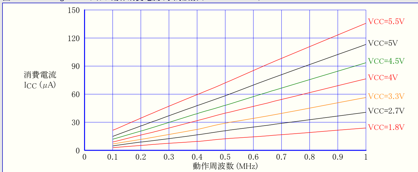
図31-195. ATmega168A: アイドル動作消費電流 対 周波数 (100kHz~1MHz)
