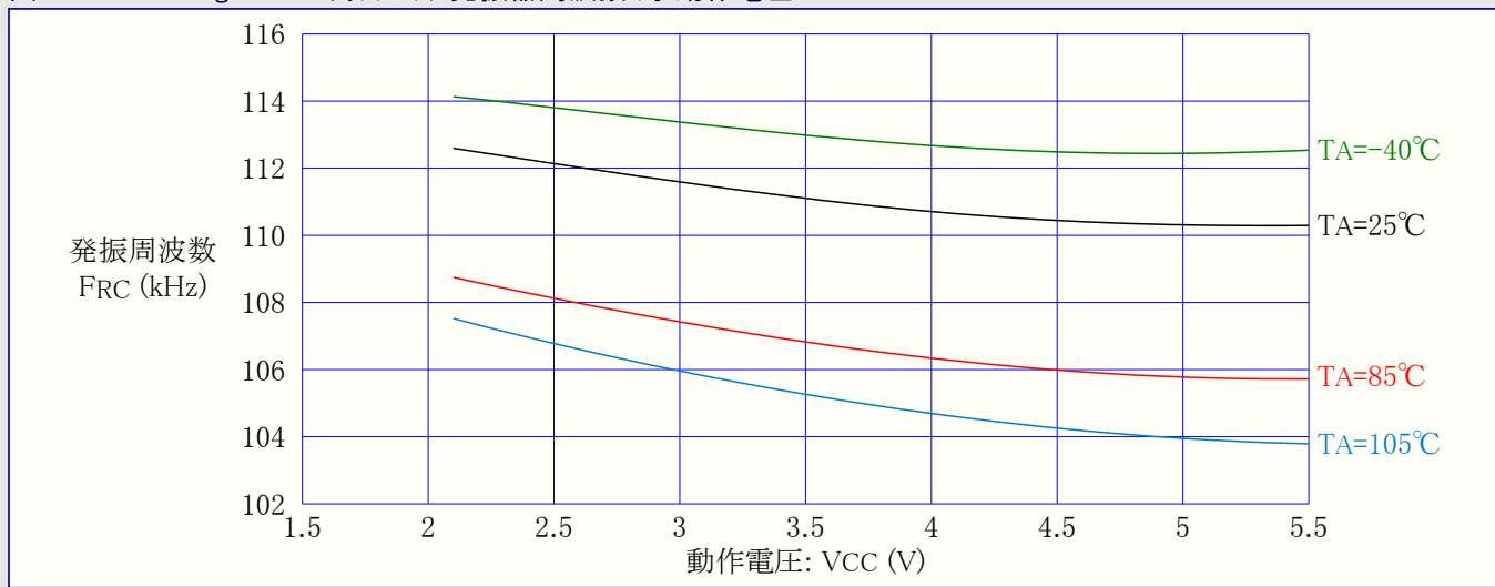
図31-178. ATmega88PA: ウォッチドッグ発振器周波数 対 動作電圧
