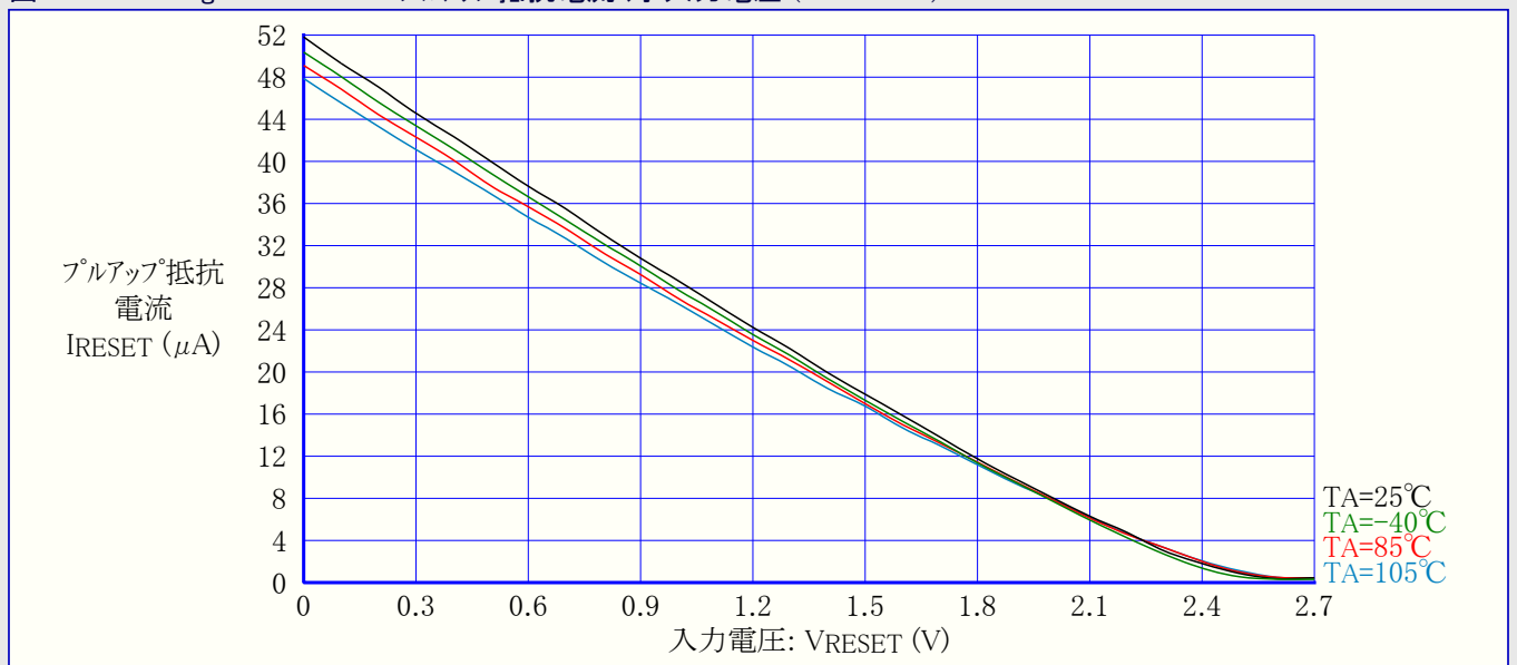
図31-66. ATmega48PA: RESETプルアップ抵抗電流 対 入力電圧 (VCC=2.7V)
