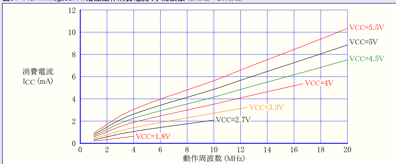
図31-143. ATmega88PA: 活動動作消費電流 対 周波数 (1MHz~20MHz)
