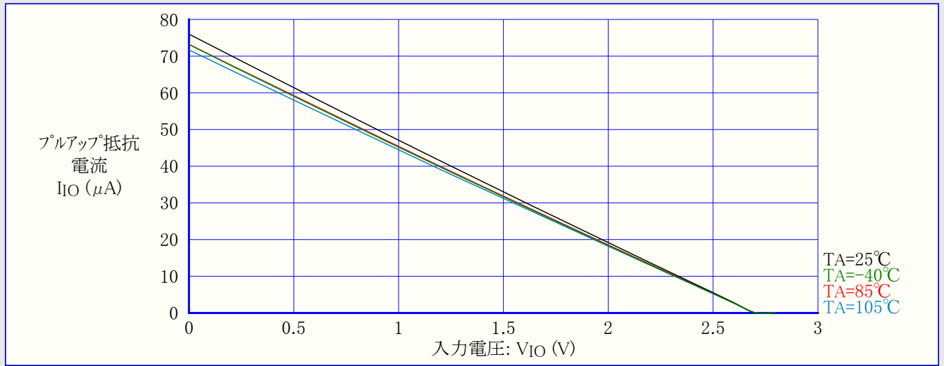
図32-108. ATmega168PA:I/Oピンプルアップ抵抗電流 対 入力電圧 (VCC=5V)
