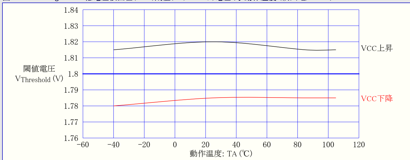
図32-76. ATmega88PA: 低電圧検出器(BOD)閾値(スレッショルド)電圧 対 動作温度 (検出電圧1.8V)
