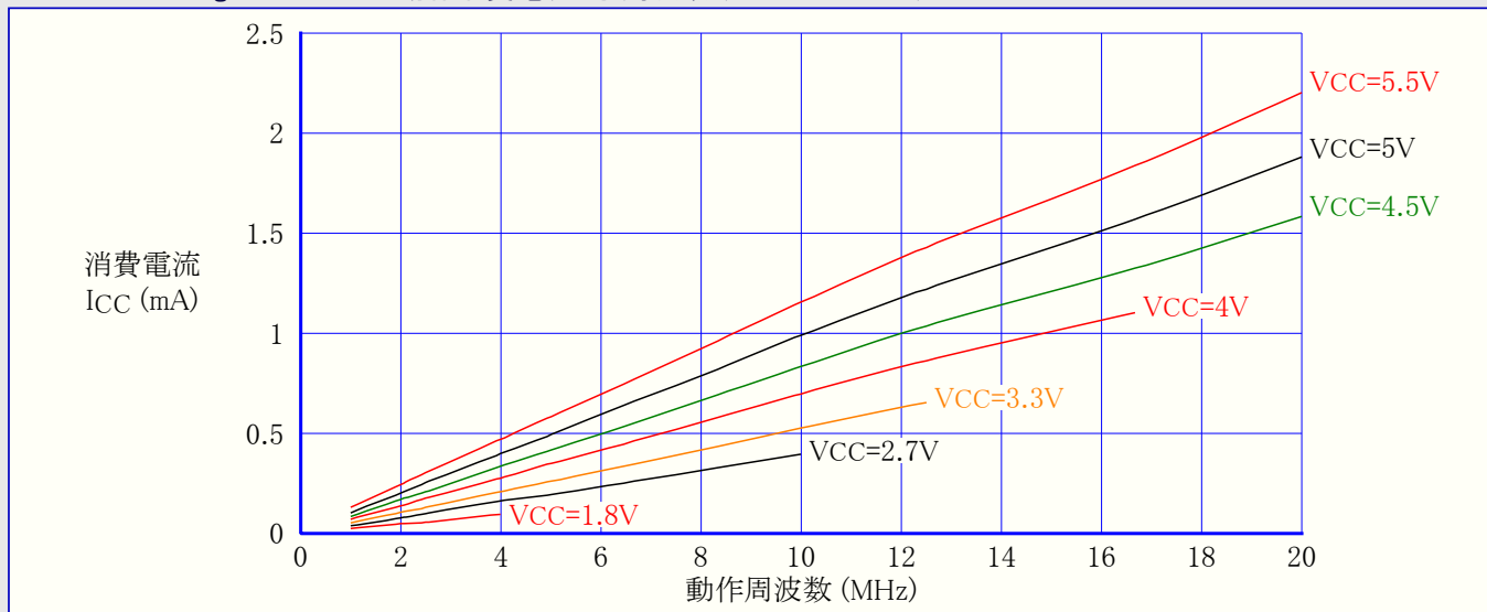
図31-148. ATmega88PA: アイドル動作消費電流 対 周波数 (1MHz~20MHz)
