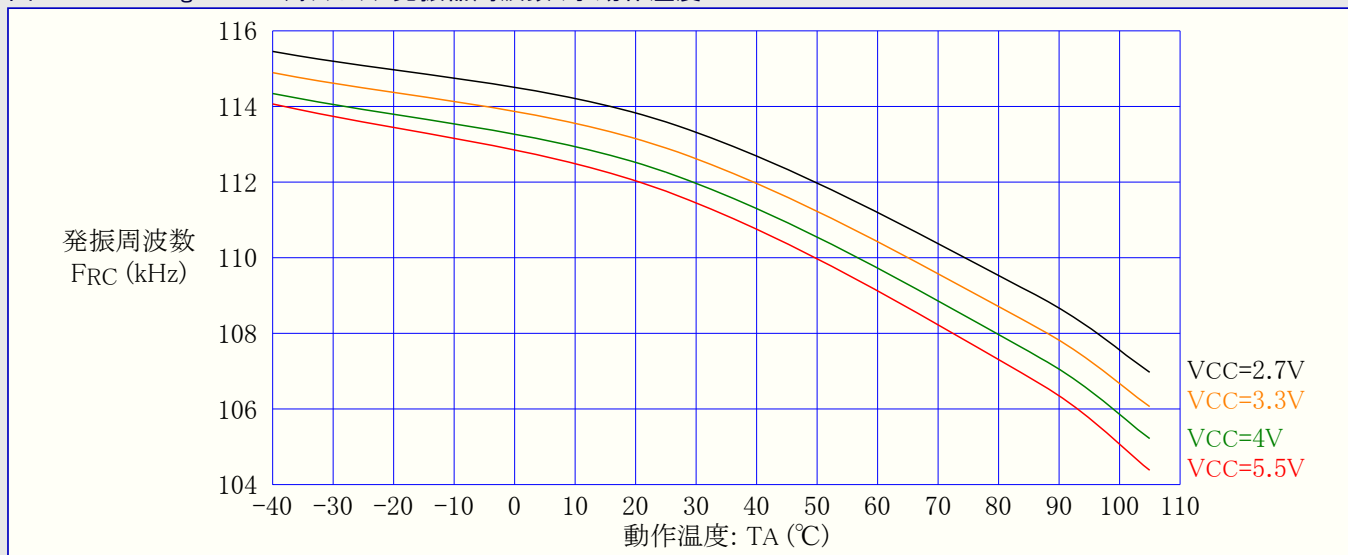
図32-34. ATmega48PA: ウォッチドッグ発振器周波数 対 動作温度
