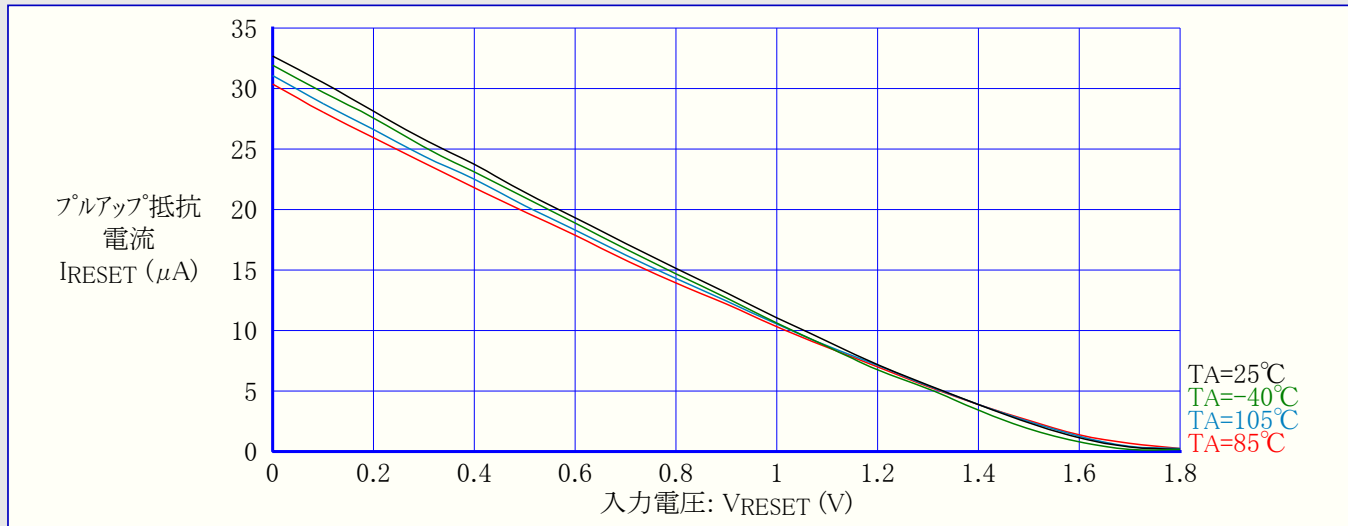
図32-18. ATmega48PA: RESETプルアップ抵抗電流 対 入力電圧 (VCC=1.8V)
