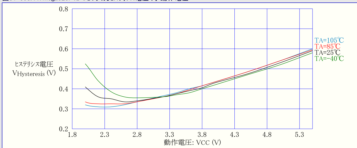
図31-358. ATmega328P:I/Oピン入力ヒステリシス電圧 対 動作電圧
