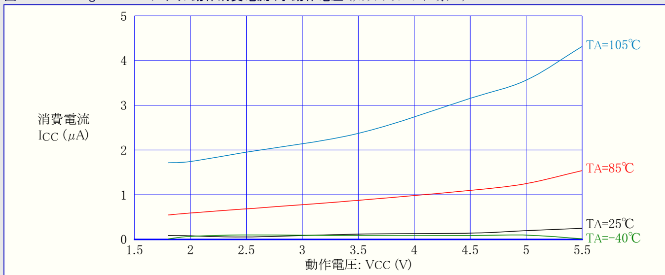
図32-57. ATmega88PA:パワーダウン動作消費電流 対 動作電圧 (ウォッチドッグ タイマ禁止)
