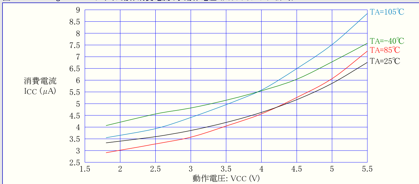
図31-59. ATmega48PA: パワーダウン動作消費電流 対 動作電圧 (ウォッチドッグ タイマ許可)
