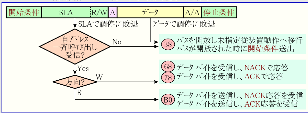
図22-21. バスの競合調停によって発生する利用可能な状態符号
