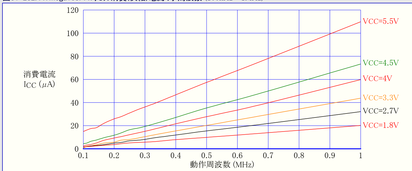
図31-282. ATmega168PA: リセット消費(供給)電流 対 周波数 (100kHz~1MHz)
