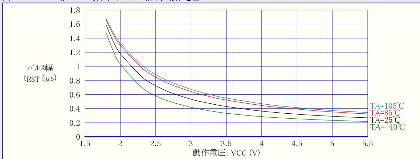
図32-186. ATmega328P:最小リセットパルス幅 対 動作電圧
