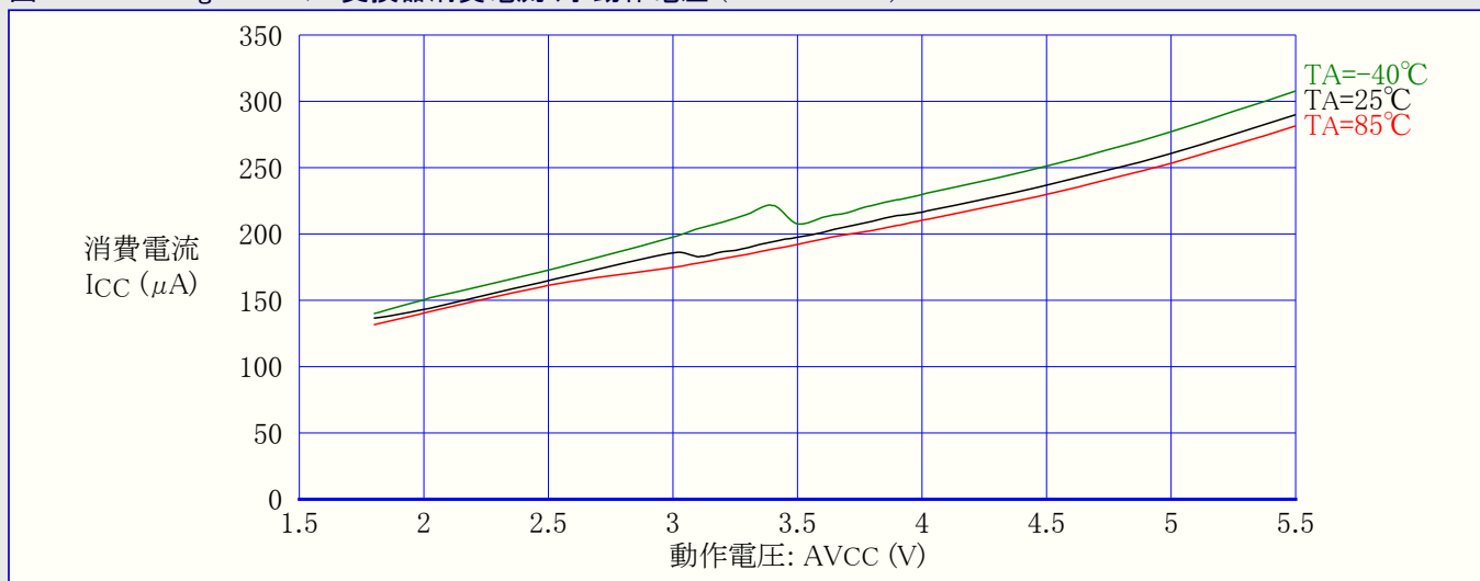
図31-40. ATmega48A: A/D変換器消費電流 対 動作電圧 (AREF=AVCC)
