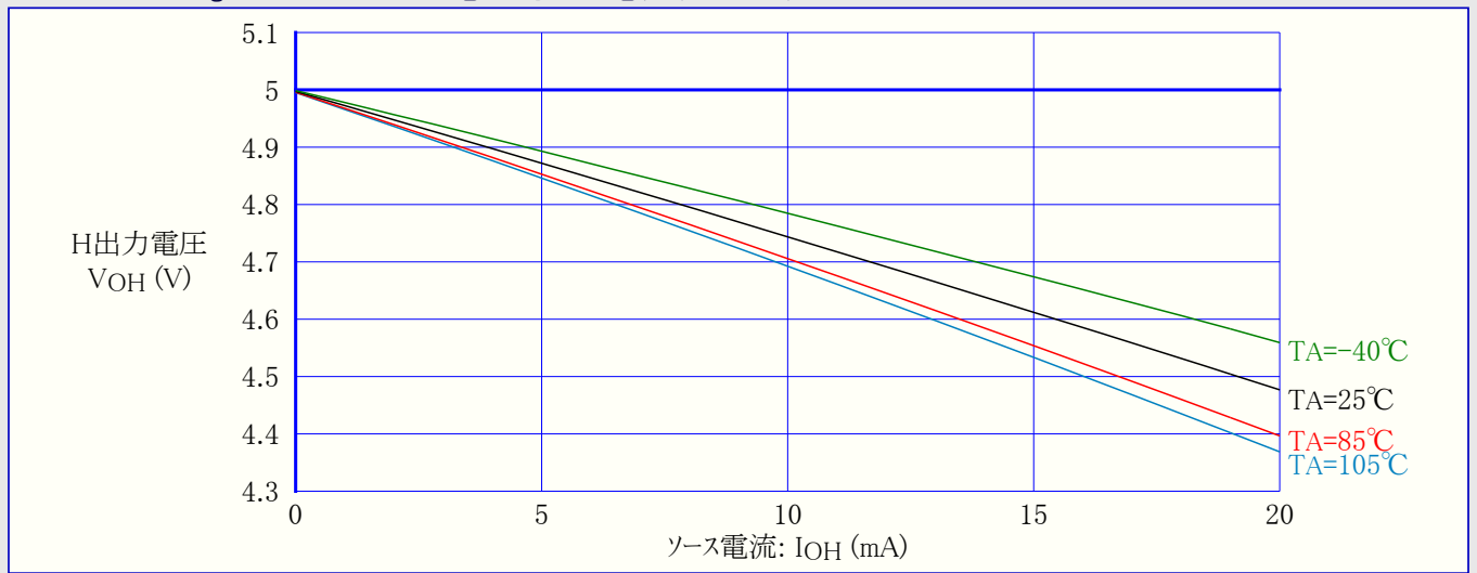
図32-163. ATmega328P:I/Oピン出力電圧 対 ソース電流 (VCC=5V)
