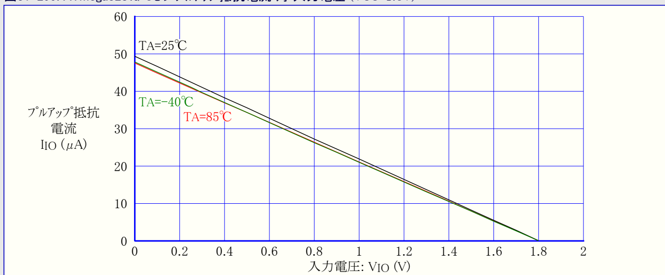
図31-299. ATmega328:I/Oピンプルアップ抵抗電流 対 入力電圧 ( V_{CC}=1.8V )
