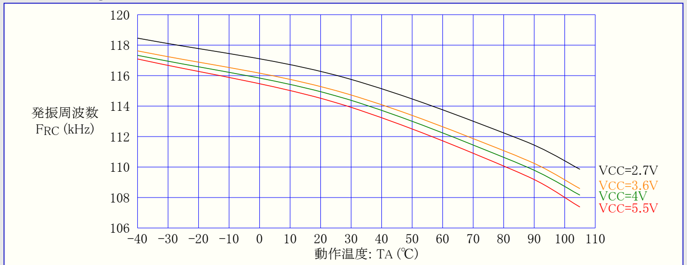
図32-174. ATmega328P: ウォッチドッグ発振器周波数 対 動作温度
