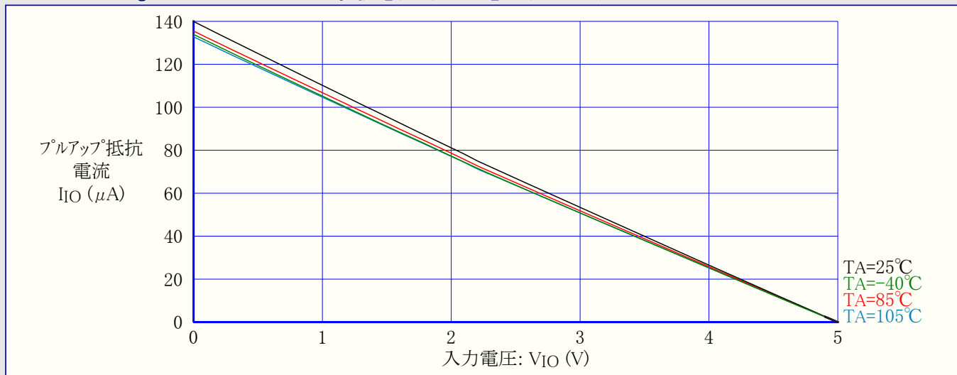
図31-253. ATmega168PA:I/Oピンプルアップ抵抗電流 対 入力電圧 (VCC=5V)
