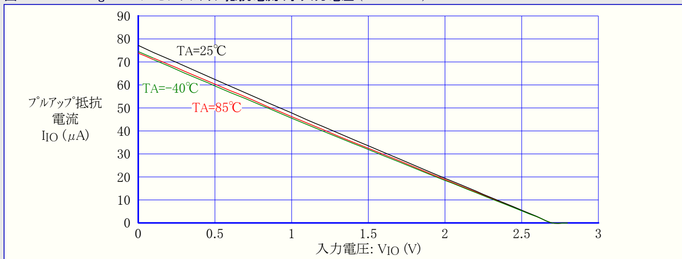
図31-300. ATmega328:I/Oピンプルアップ抵抗電流 対 入力電圧 ( V_{CC}=2.7V )
