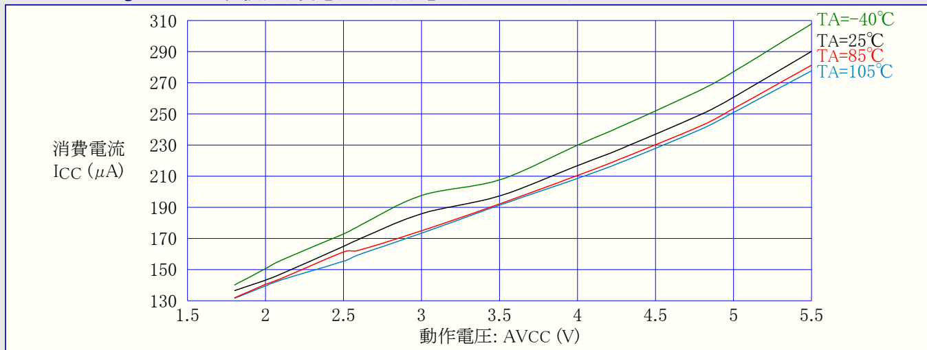
図32-39. ATmega48PA: A/D変換器消費電流 対 動作電圧 (AREF=AVCC)
