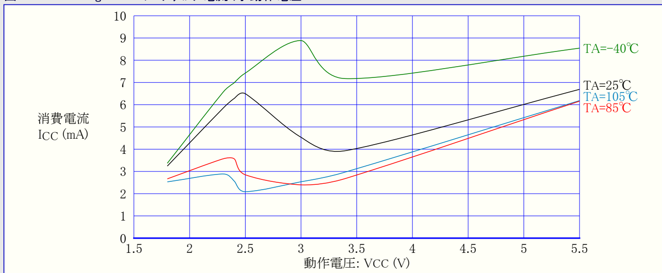
図31-186. ATmega88PA: プログラミング電流 対 動作電圧
