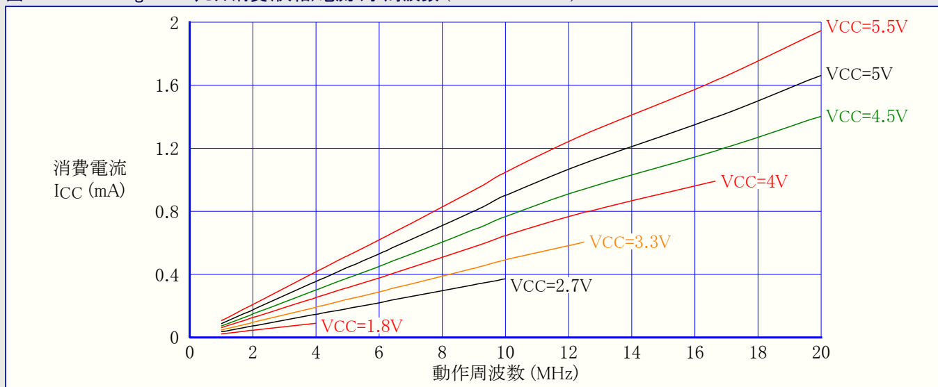
図31-140. ATmega88A:リセット消費(供給)電流 対 周波数 (1MHz~20MHz)
