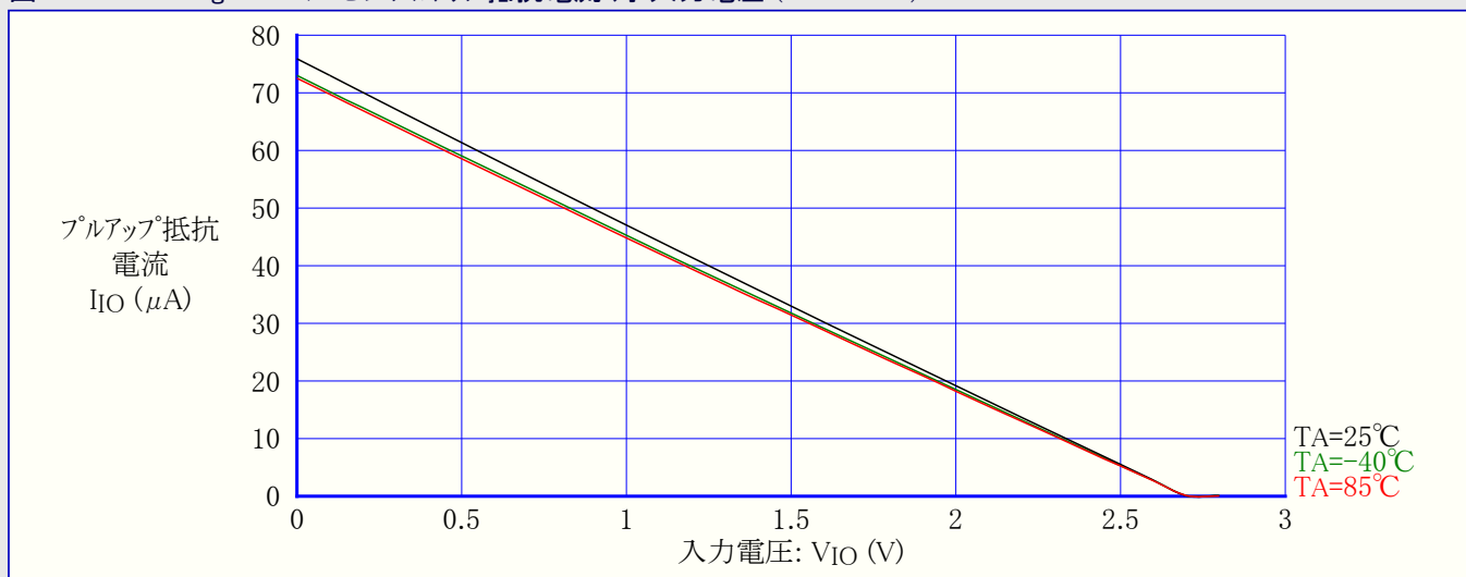
図31-110. ATmega88A:I/Oピンプルアップ抵抗電流 対 入力電圧 ( V_{CC}=2.7V )
