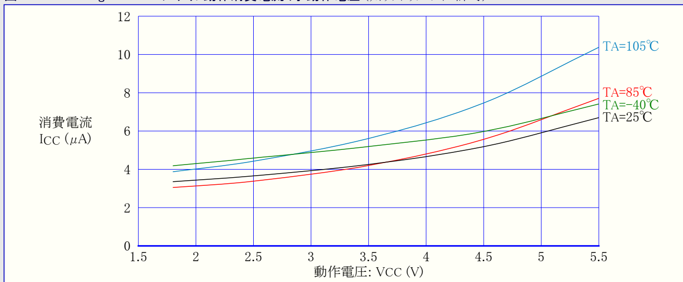
図31-153. ATmega88PA: パワーダウン動作消費電流 対 動作電圧 (ウォッチドッグ タイマ許可)
