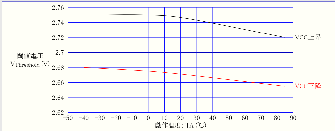
図31-32. ATmega48A: 低電圧検出器(BOD)閾値(スレッシュホールド)電圧 対 動作温度 (検出電圧2.7V)
