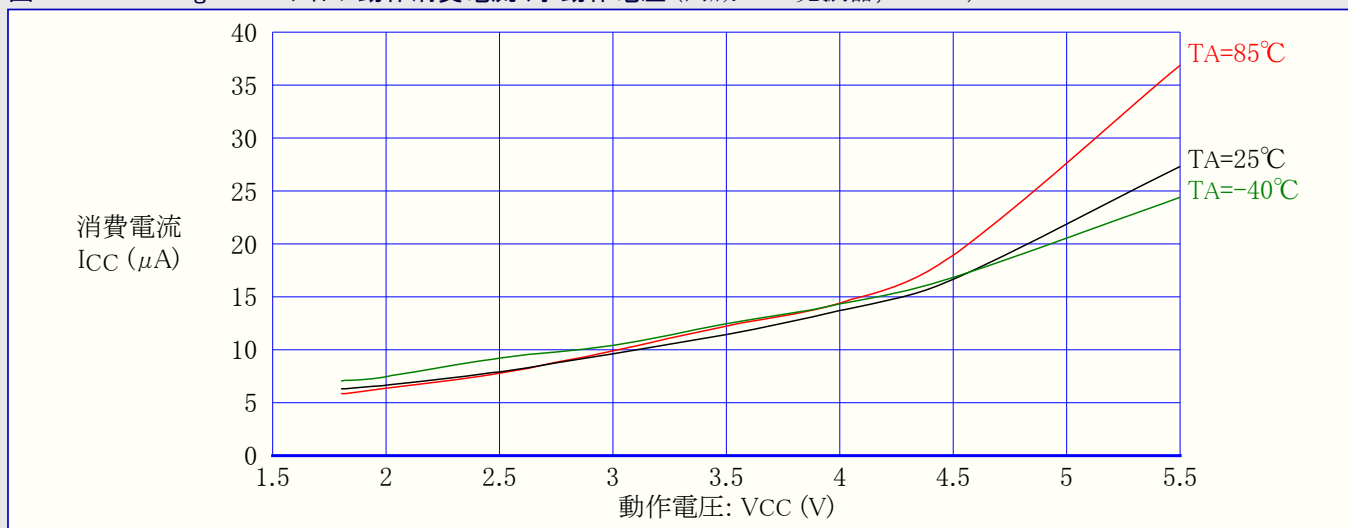
図31-197. ATmega168A: アイドル動作消費電流 対 動作電圧 (内蔵WDT発振器, 128kHz)
