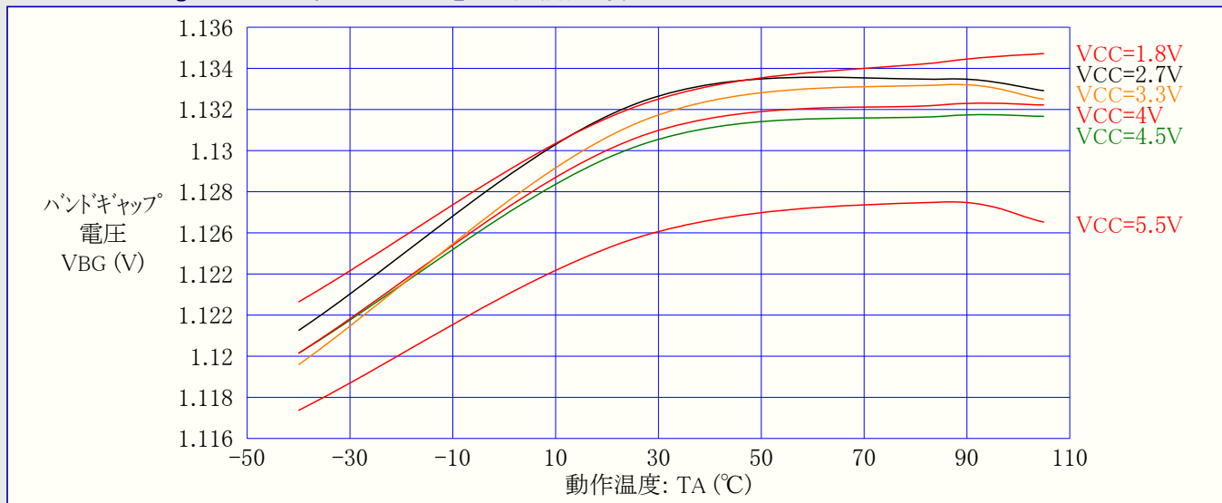
図32-125. ATmega168PA: 内部バンドギャップ電圧 対 動作温度
