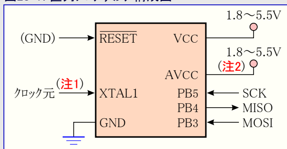
図28-7. 直列プログラミング構成図
