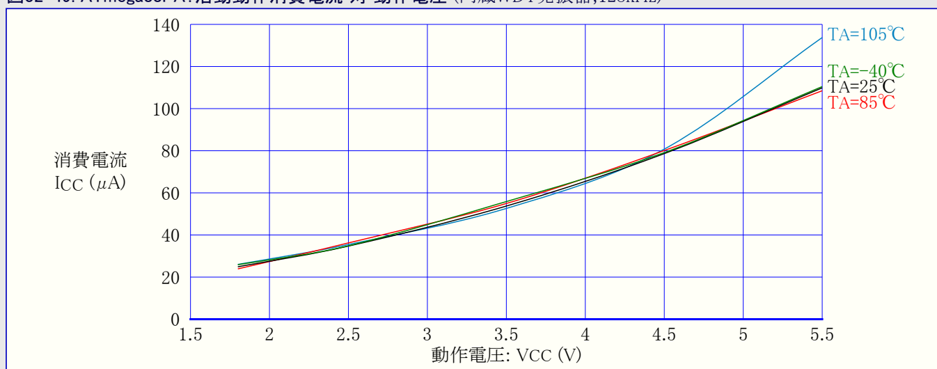
図32-49. ATmega88PA: 活動動作消費電流 対 動作電圧 (内蔵WDT発振器, 128kHz)
