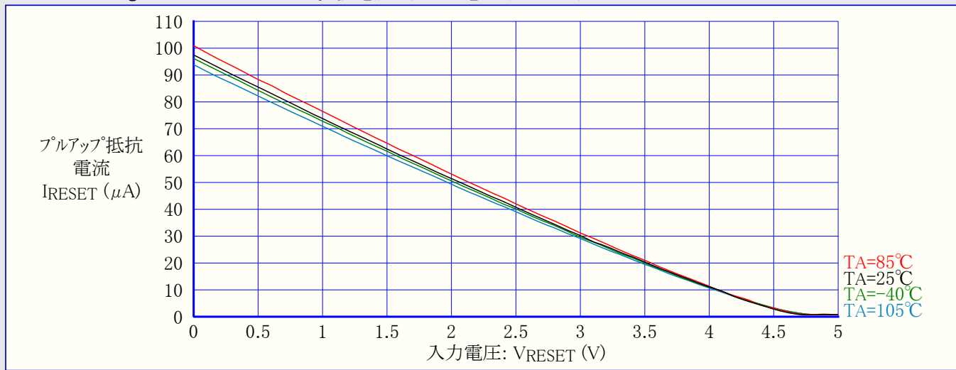
図31-67. ATmega48PA: RESETプルアップ抵抗電流 対 入力電圧 (VCC=5V)
