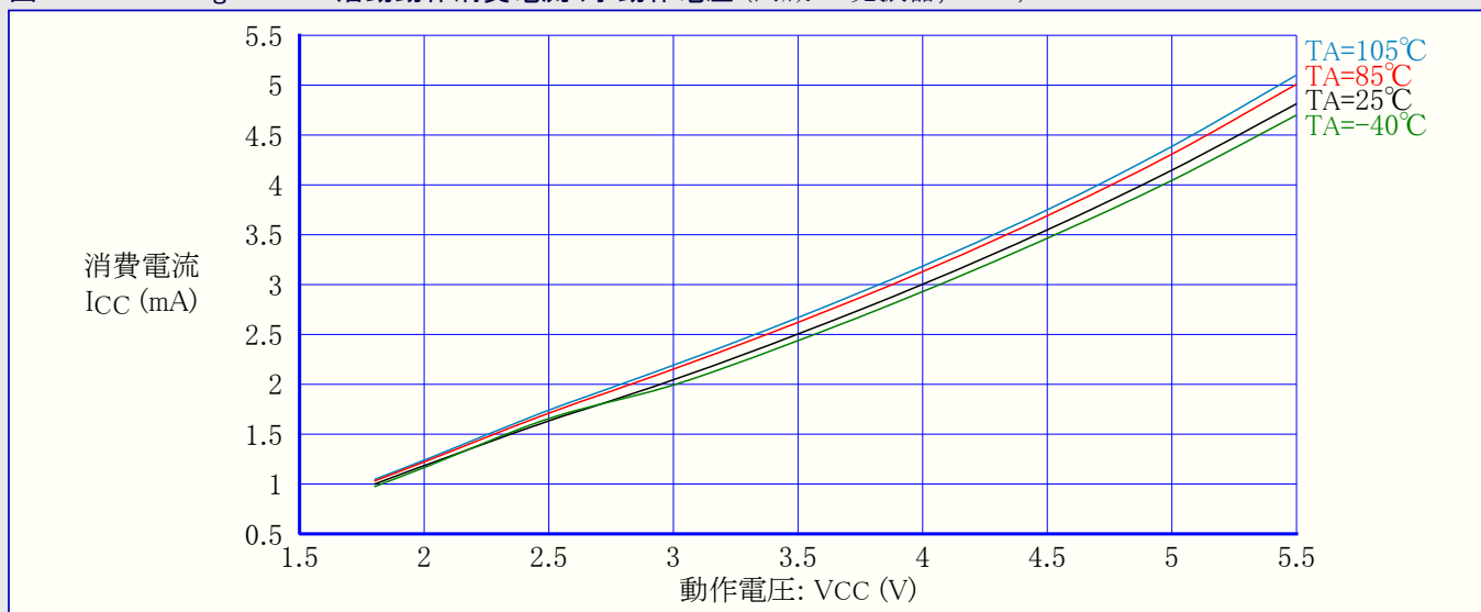
図31-241. ATmega168PA: 活動動作消費電流 対 動作電圧 (内蔵RC発振器, 8MHz)
