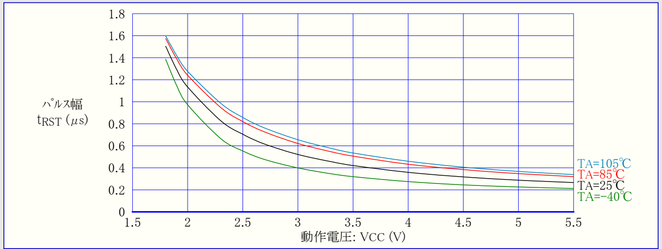
図31-189. ATmega88PA:最小リセットハルス幅 対 動作電圧
