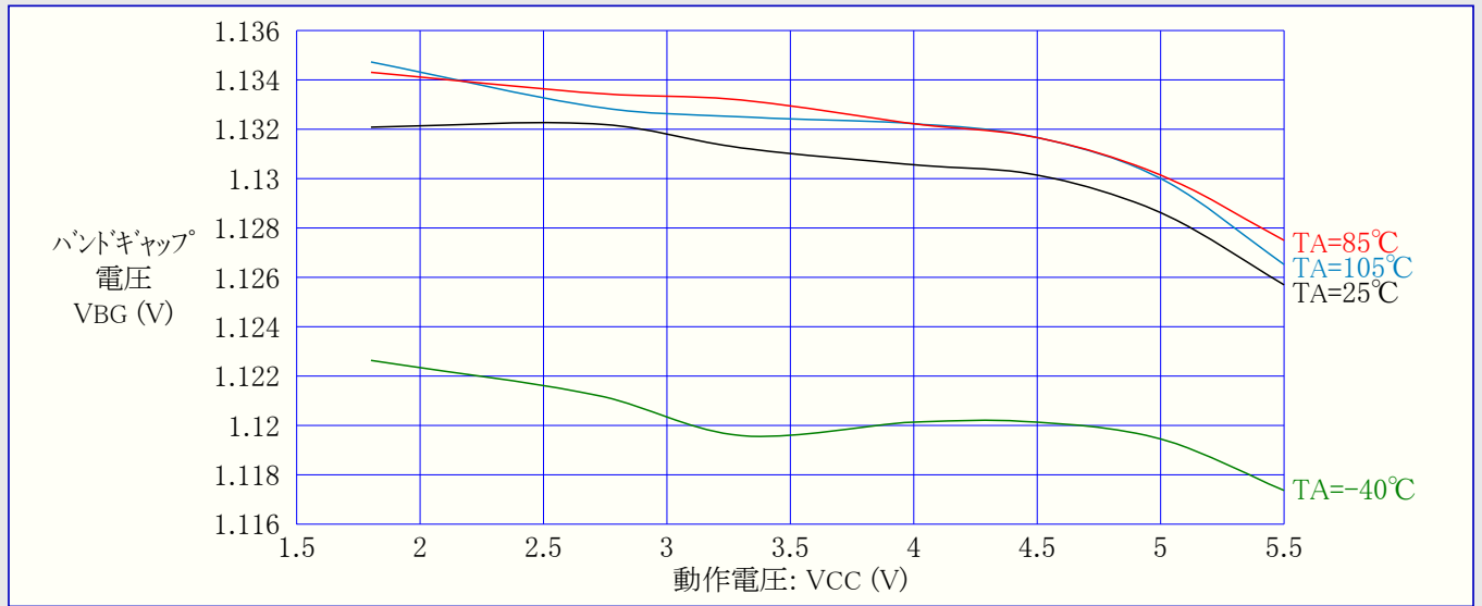
図31-271. ATmega168PA: 内部バンドギャップ電圧 対 動作電圧
