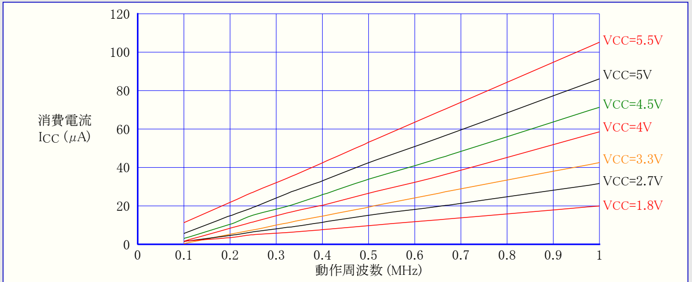
図31-234. ATmega168A:リセット消費(供給)電流 対 周波数 (100kHz~1MHz)
