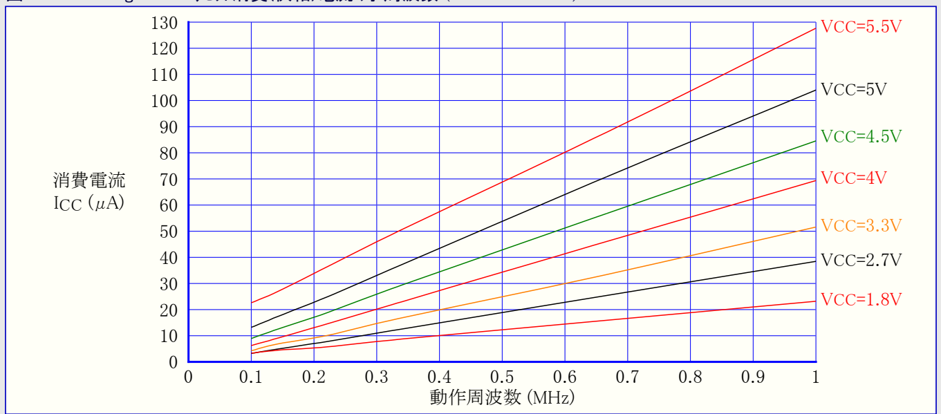
図32-44. ATmega48PA: リセット消費(供給)電流 対 周波数 (100kHz~1MHz)
