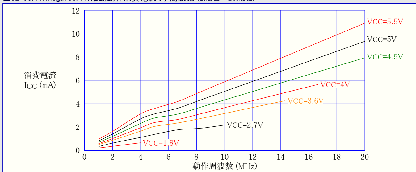
図32-93. ATmega168PA: 活動動作消費電流 対 周波数 (1MHz~20MHz)
