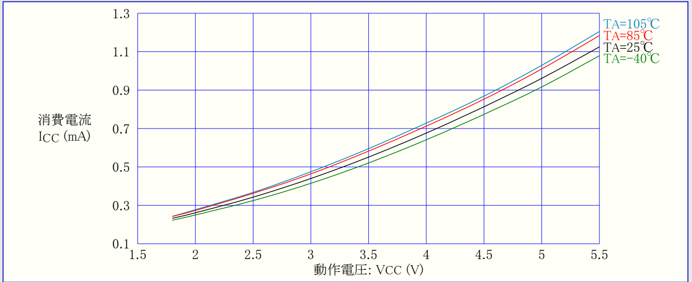
図32-101. ATmega168PA:アイドル動作消費電流 対 動作電圧 (内蔵RC発振器,8MHz)
