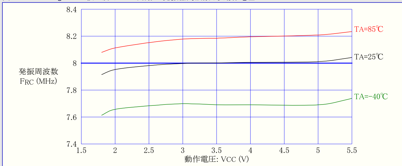
図31-226. ATmega168A: 校正済み8MHz内蔵RC発振器周波数 対 動作電圧
