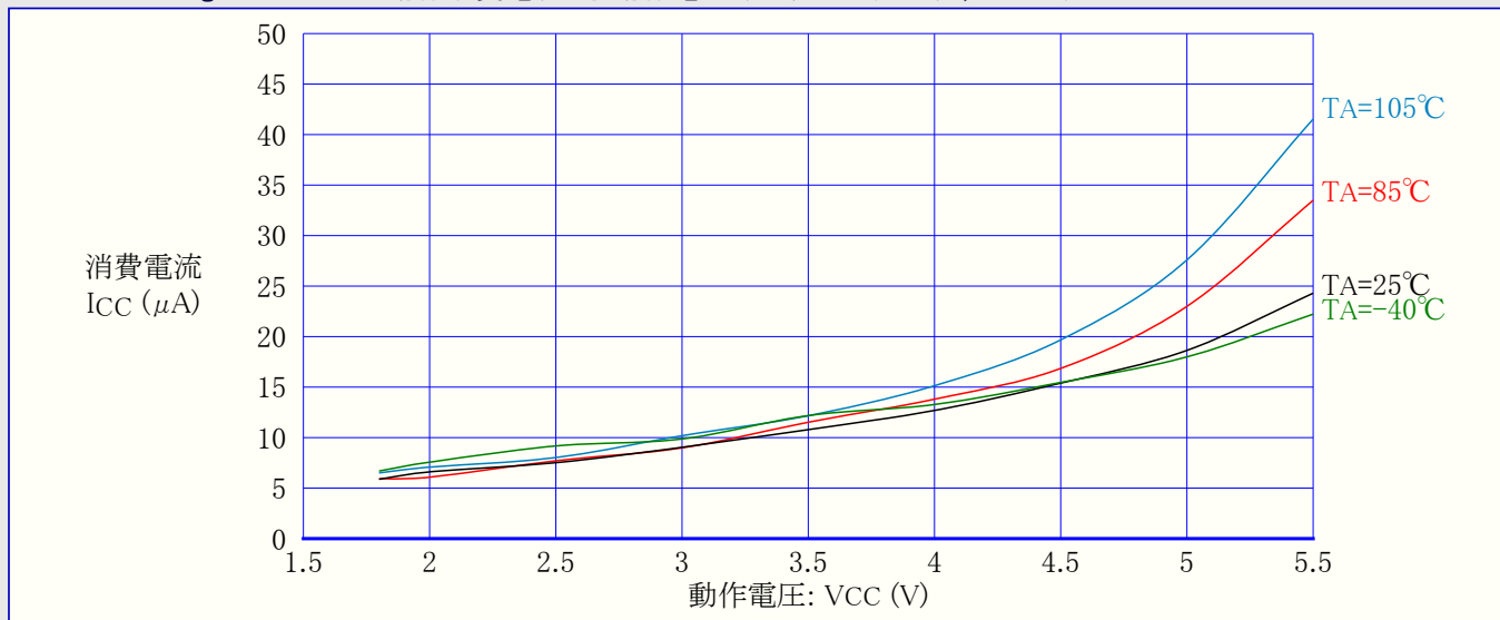
図32-54. ATmega88PA:アイドル動作消費電流 対 動作電圧 (内蔵WDT発振器,128kHz)
