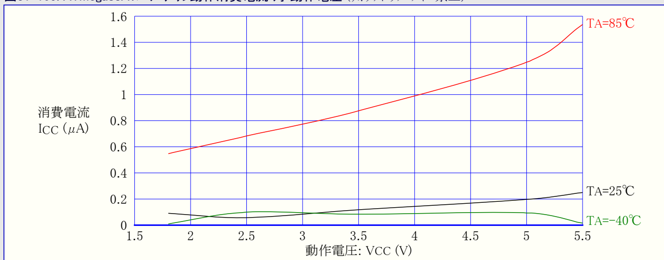
図31-105. ATmega88A: パワーダウン動作消費電流 対 動作電圧 (ウォッチドッグ タイマ禁止)
