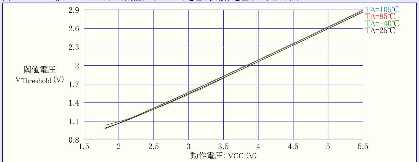
図31-72. ATmega48PA:I/Oピン入力閾値(スレッシュォルト)電圧 対 動作電圧 (VIH,1読み値)
