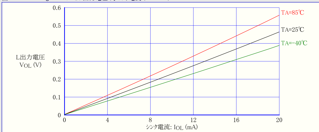
図31-116. ATmega88A: I/Oピン出力電圧 対 シンク電流 (VCC=5V)
