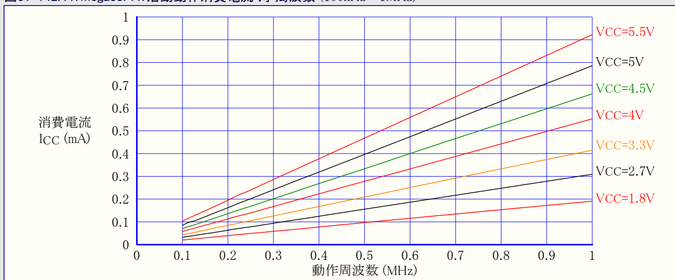
図31-142. ATmega88PA: 活動動作消費電流 対 周波数 (100kHz~1MHz)
