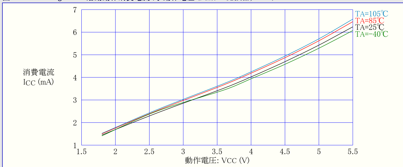
図32-144. ATmega328P: 活動動作消費電流 対 動作電圧 (内蔵RC発振器, 8MHz)
