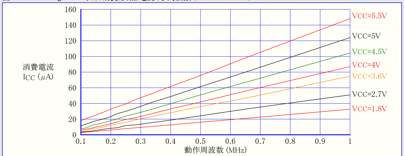
図32-184. ATmega328P: リセット消費(供給)電流 対 周波数 (100kHz~1MHz)
