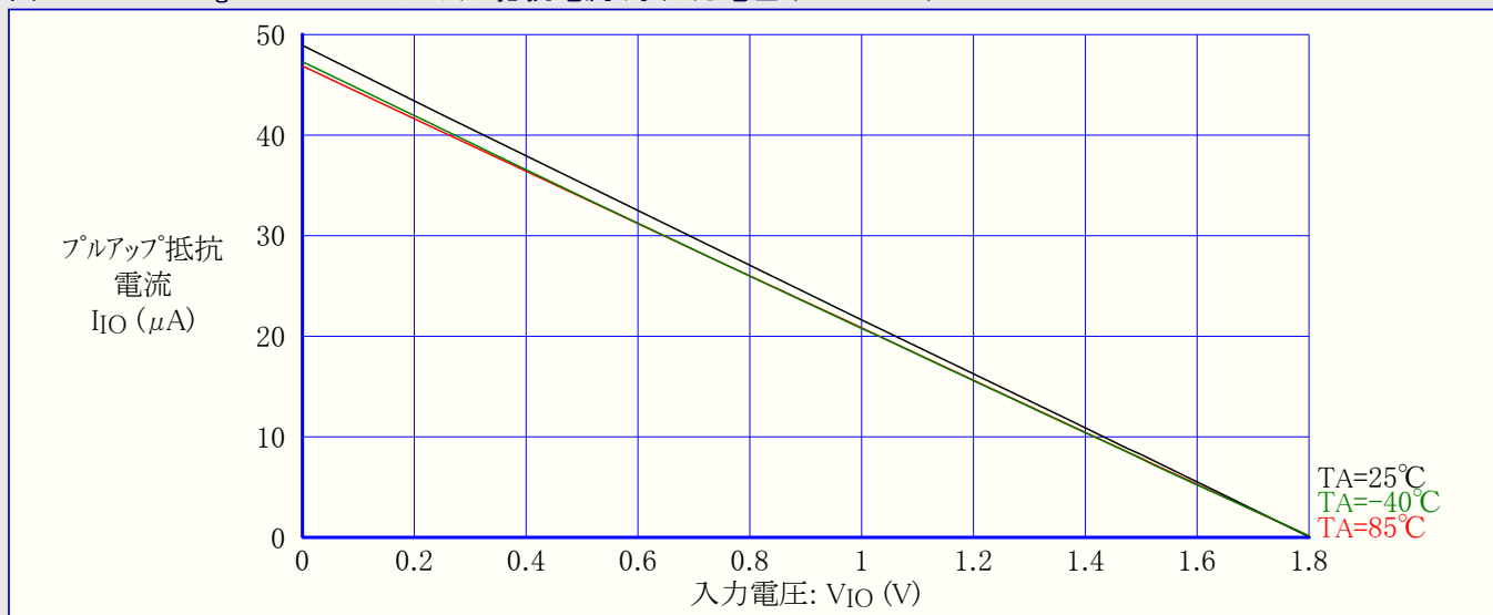
図31-109. ATmega88A:I/Oピンプルアップ抵抗電流 対 入力電圧 ( V_{CC}=1.8V )
