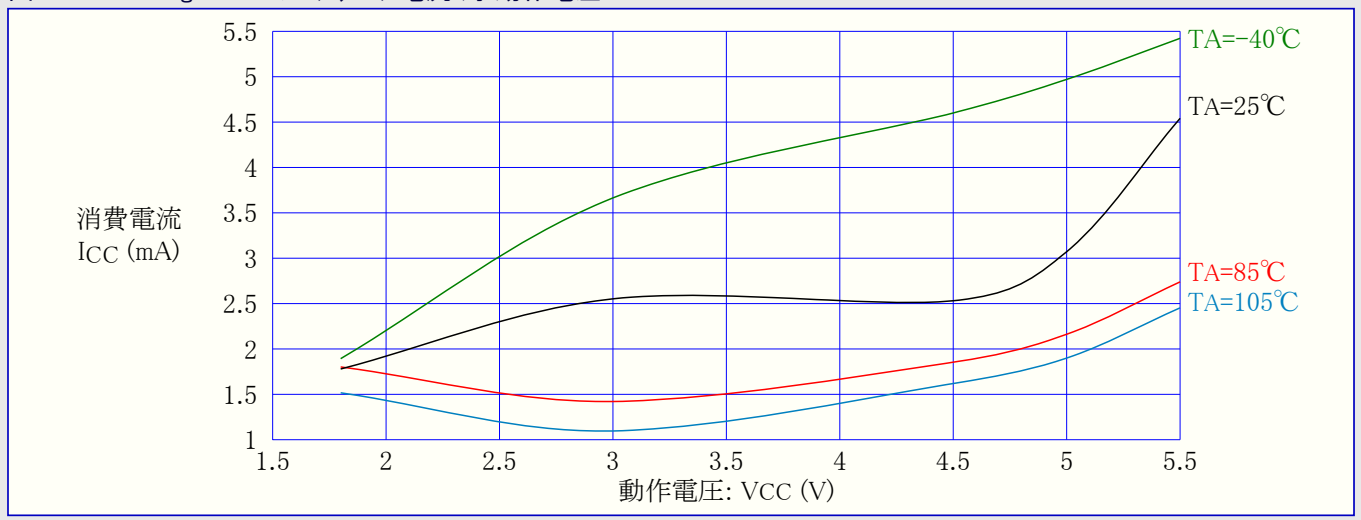
図32-43. ATmega48PA: プログラミング電流 対 動作電圧
