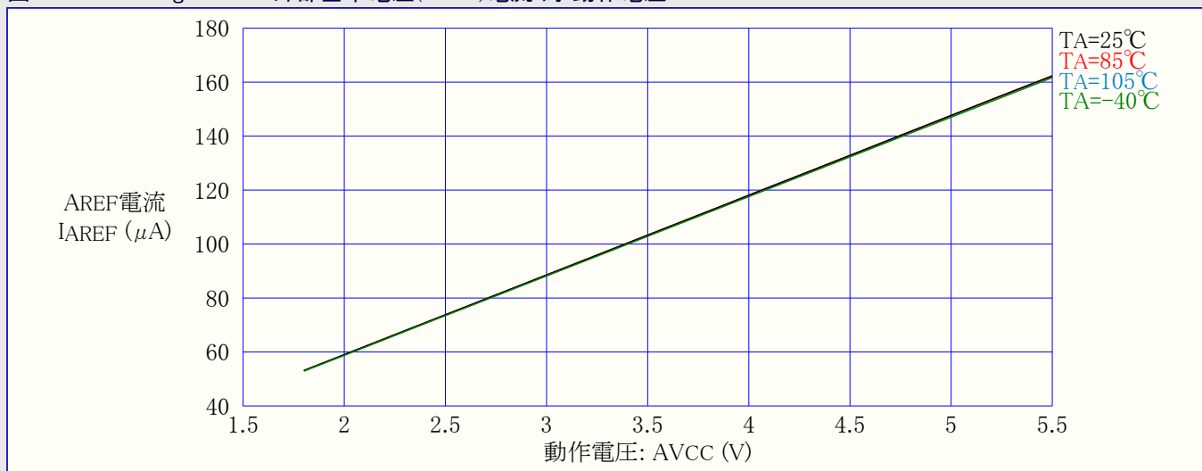
図31-278. ATmega168PA: 外部基準電圧(AREF)電流 対 動作電圧
