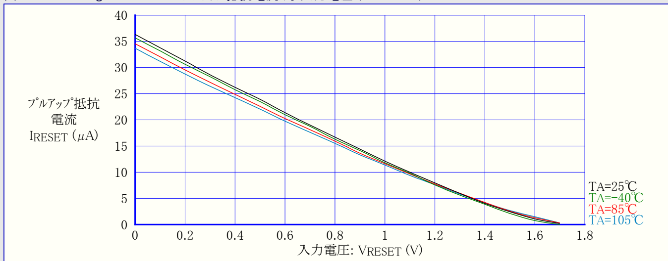
図32-157. ATmega328P:RESETプルアップ抵抗電流 対 入力電圧 (VCC=1.8V)
