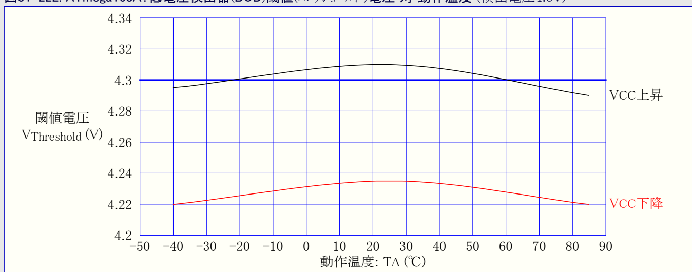
図31-222. ATmega168A: 低電圧検出器(BOD)閾値(スレッシュホールド)電圧 対 動作温度 (検出電圧4.3V)
