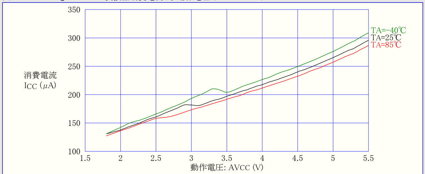
図31-229. ATmega168A: A/D変換器消費電流 対 動作電圧 (AREF=AVCC)
