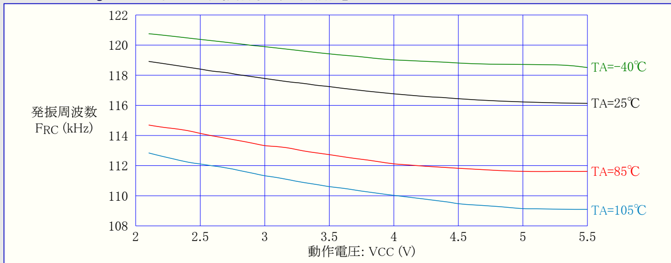
図32-128. ATmega168PA: ウォッチドッグ発振器周波数 対 動作電圧
