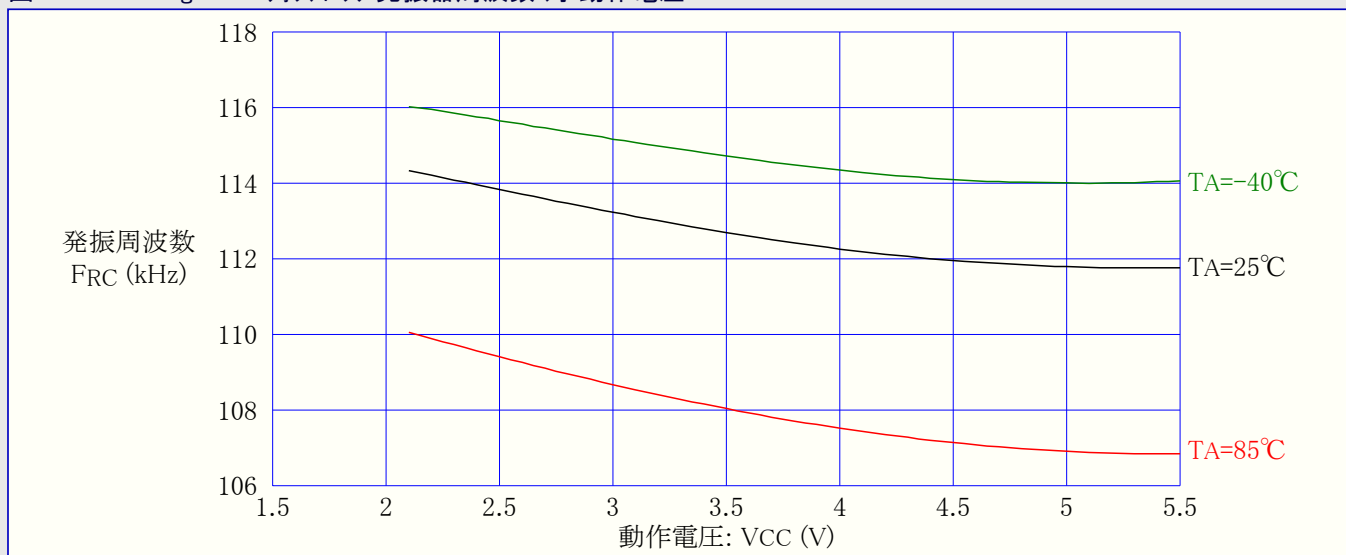
図31-36. ATmega48A: ウォッチドッグ発振器周波数 対 動作電圧
