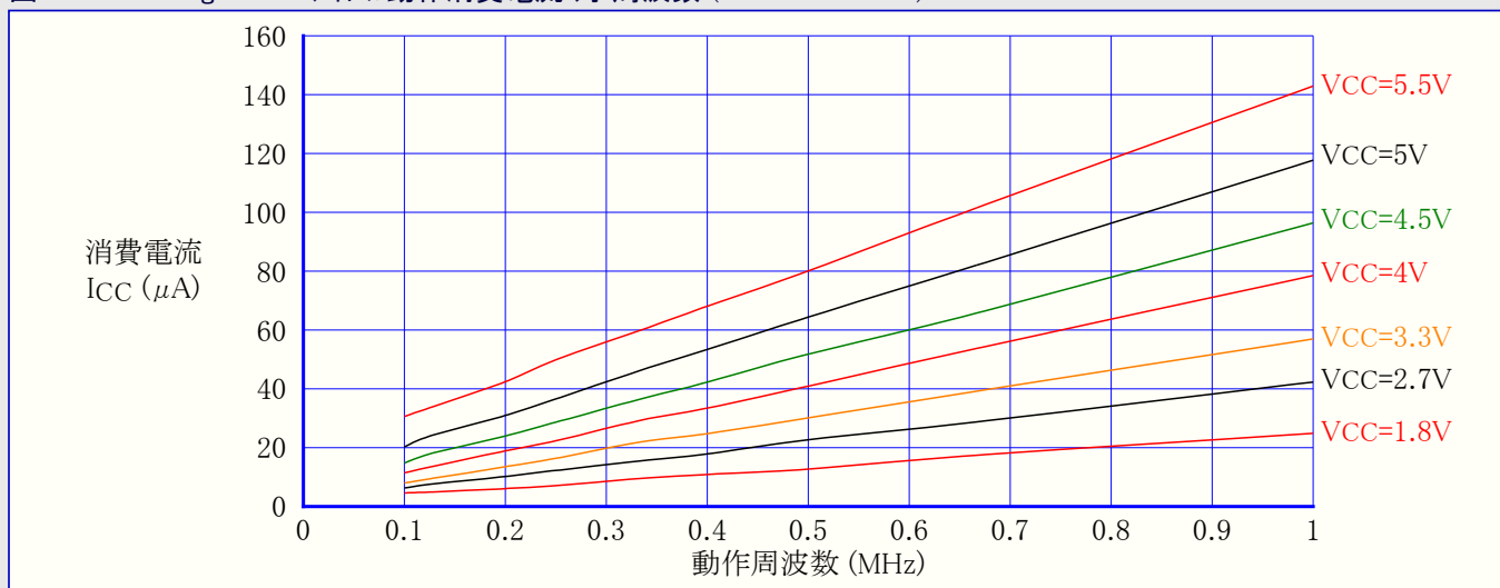
図31-53. ATmega48PA: アイドル動作消費電流 対 周波数 (100kHz~1MHz)
