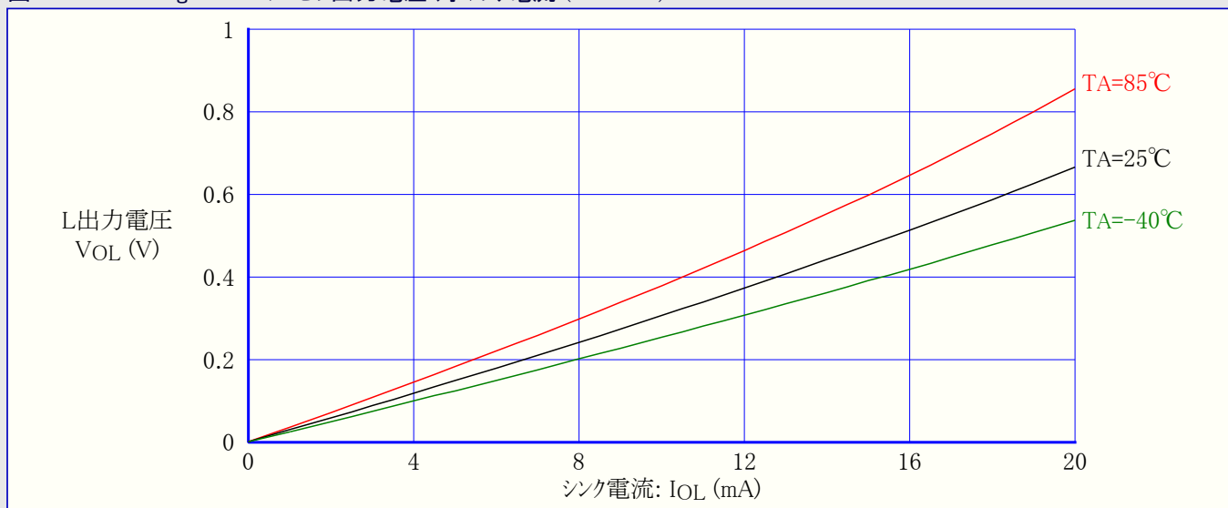
図31-210. ATmega168A:I/Oピン出力電圧 対 シンク電流 (VCC=3V)
