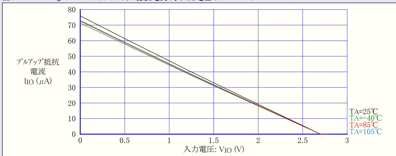
図31-157. ATmega88PA:I/Oピンプルアップ抵抗電流 対 入力電圧 (VCC=2.7V)
