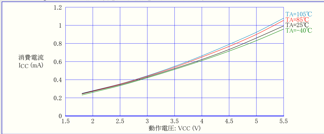
図32-56. ATmega88PA:アイドル動作消費電流 対 動作電圧 (内蔵RC発振器,8MHz)
