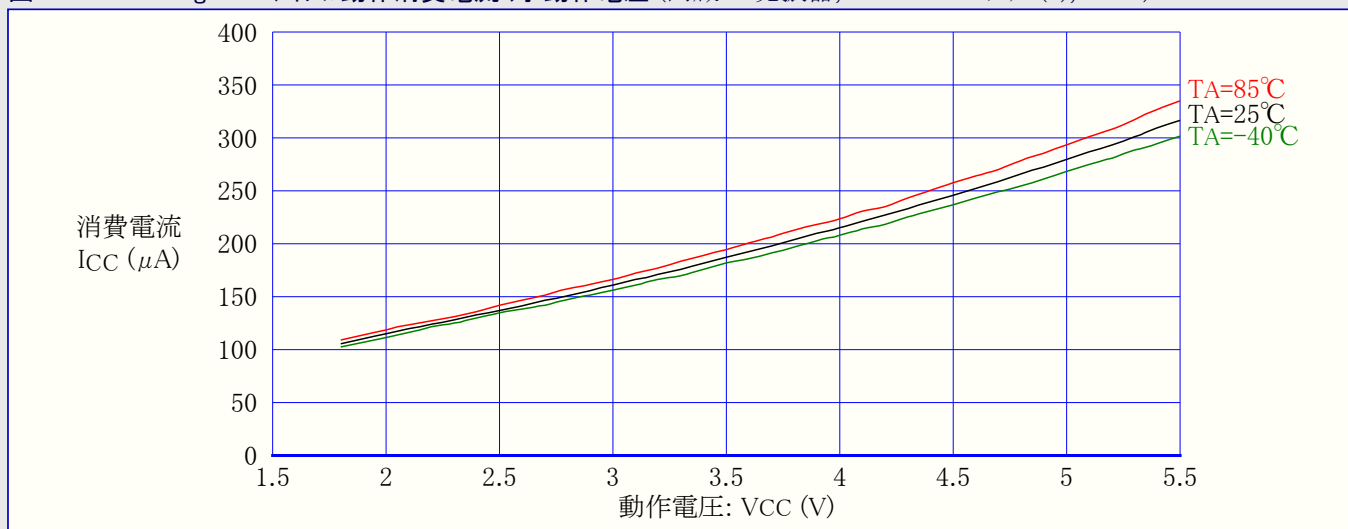
図31-293. ATmega328:アイドル動作消費電流 対 動作電圧 (内蔵RC発振器,CKDIV8=プログラム(0),1MHz)
