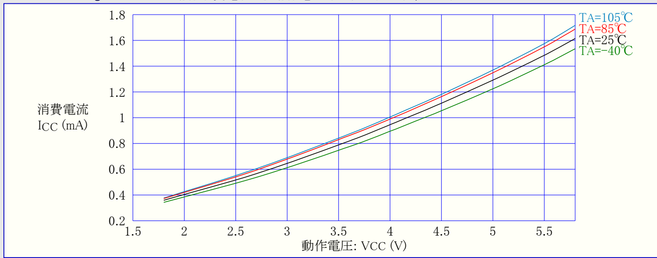
図31-341. ATmega328P:アイドル動作消費電流 対 動作電圧 (内蔵RC発振器,8MHz)
