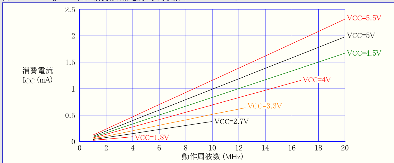
図31-46. ATmega48A:リセット消費(供給)電流 対 周波数 (1MHz~20MHz)
