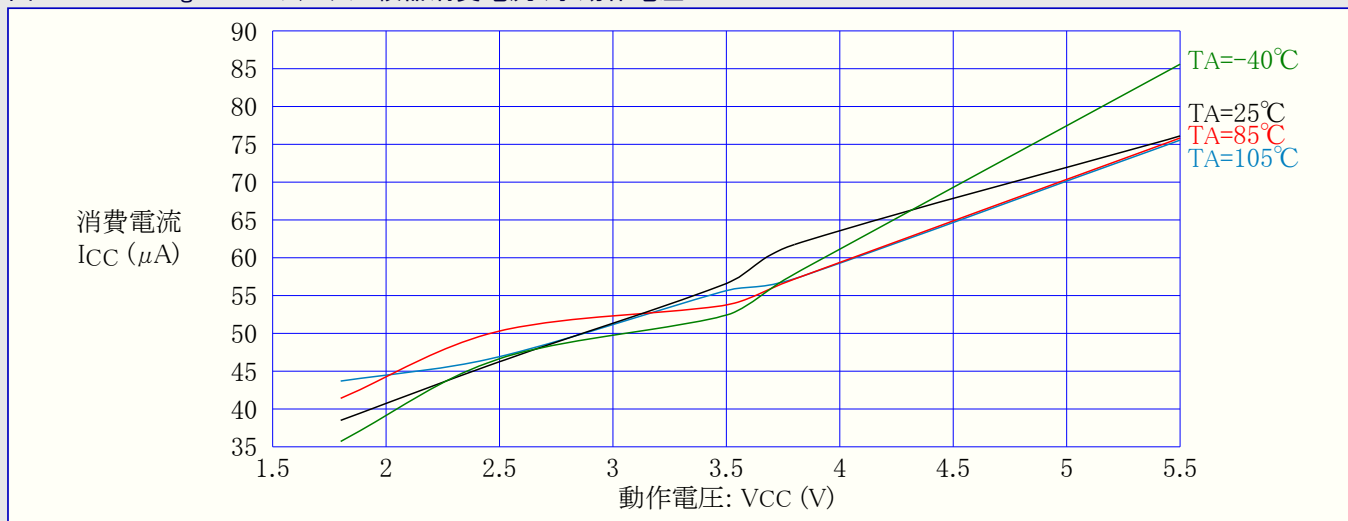
図32-41. ATmega48PA: アナログ比較器消費電流 対 動作電圧
