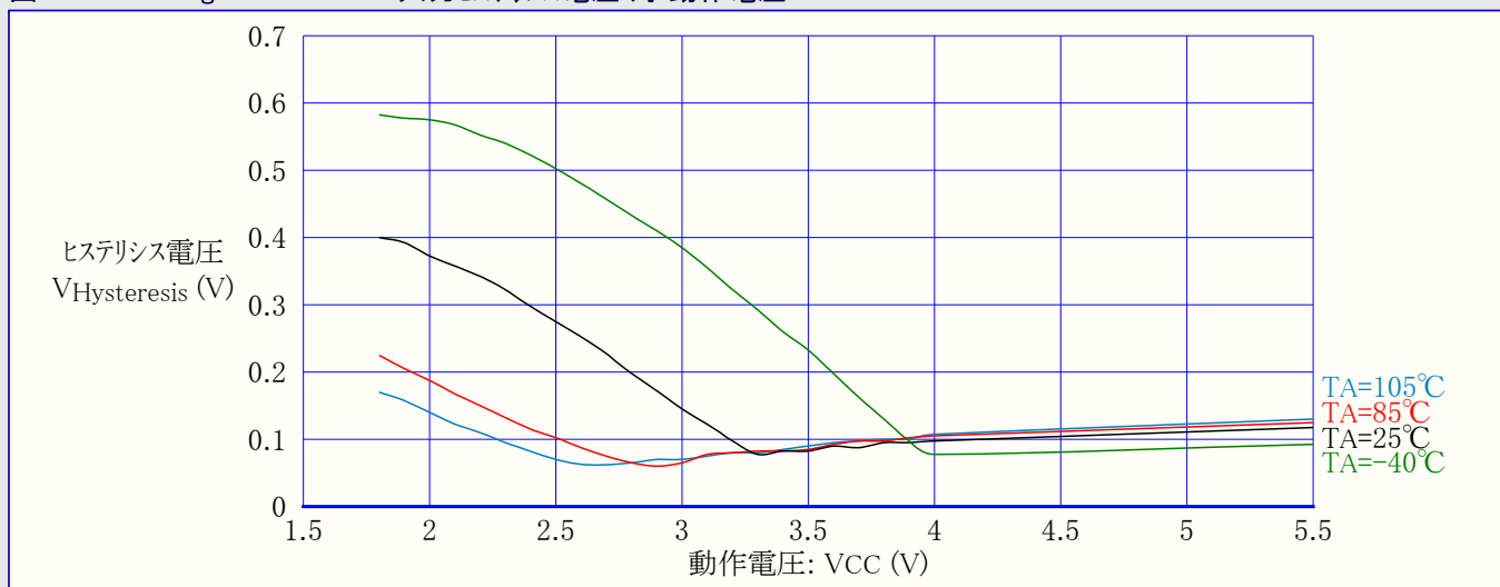
図32-75. ATmega88PA: RESET入力ヒステリシス電圧 対 動作電圧
