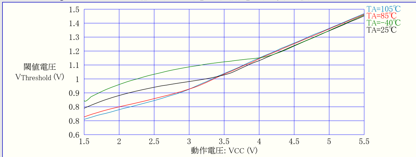
図31-264. ATmega168PA:RESET入力閾値(スレッショルド)電圧 対 動作電圧 (VIH,1読み値)
