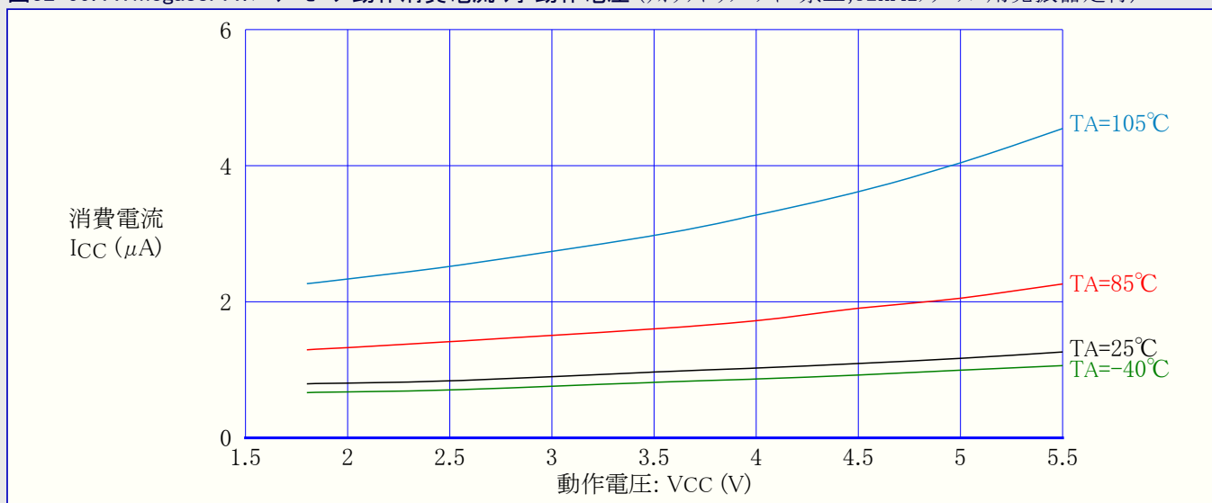
図32-59. ATmega88PA:ハワーセーフ動作消費電流 対 動作電圧 (ウォッチドッグ タイマ禁止,32kHzクリスタル用発振器走行)
