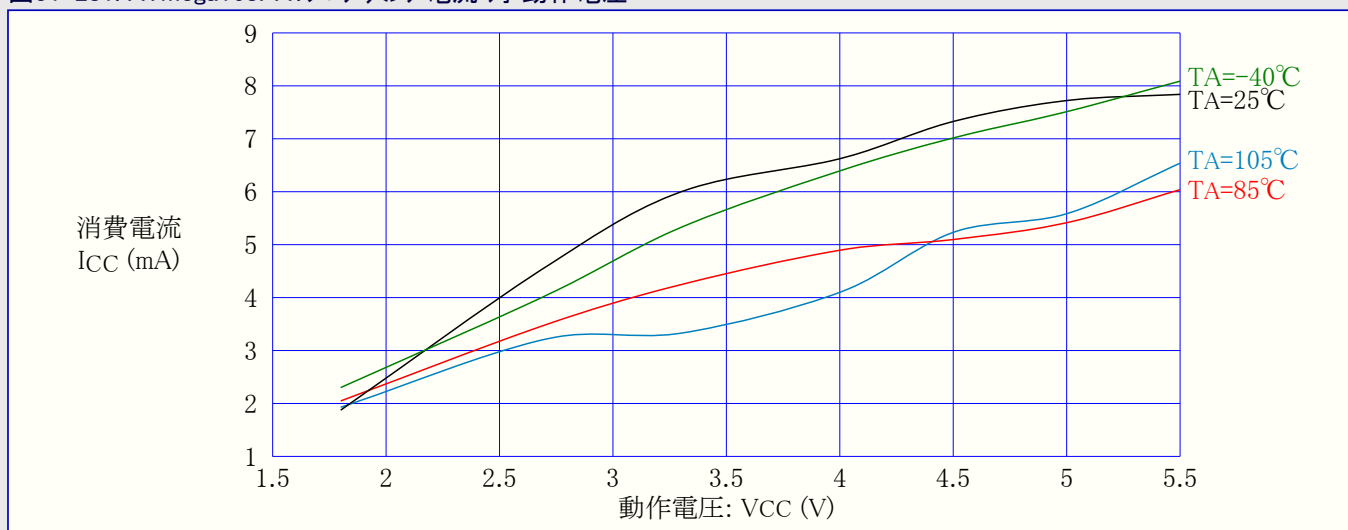
図31-281. ATmega168PA: フロタラシク電流 対 動作電圧
