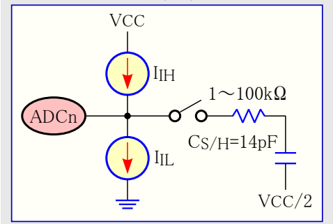
図24-8. アナログ入力回路
