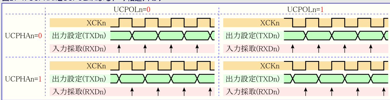
図21-1. UCPHAnとUCPOLnによるデータ転送タイミング
