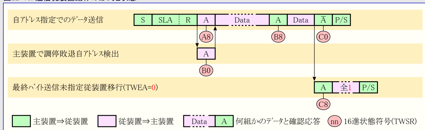
図22-18. 送信従装置動作の形式と状態
