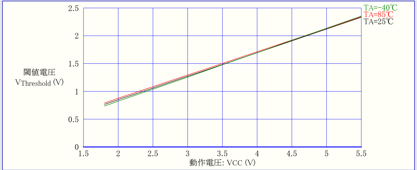
図31-218. ATmega168A: RESET入力閾値(スレッショルド)電圧 対 動作電圧 (VIL,0読み値)
