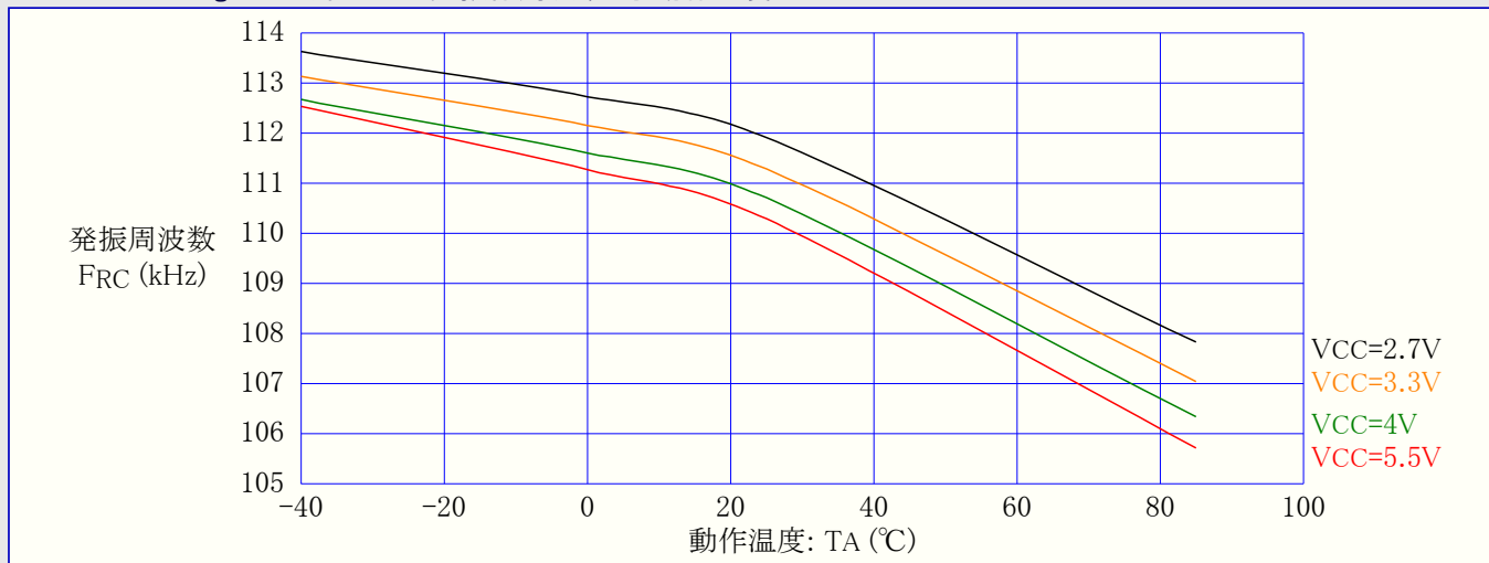
図31-129. ATmega88A: ウォッチドッグ発振器周波数 対 動作温度
