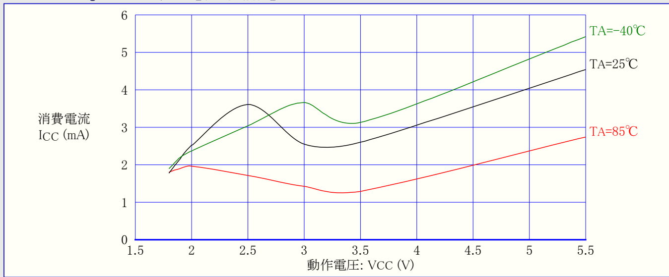
図31-44. ATmega48A:プログラミング電流 対 動作電圧
