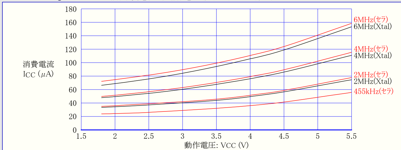
図31-108. ATmega88A:スタンバイ動作消費電流 対 動作電圧 (ウォッチドッグ タイマ禁止)
