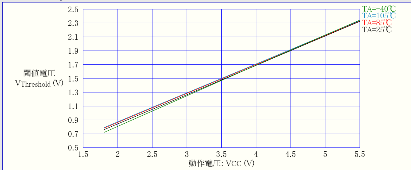
図31-360. ATmega328P: RESET入力閾値(スレッシュホールド)電圧 対 動作電圧 (VIL,0読み値)
