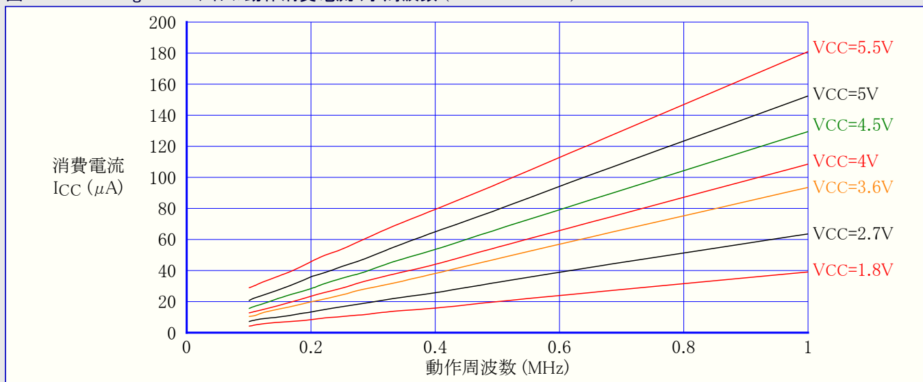
図31-337. ATmega328P: アイドル動作消費電流 対 周波数 (100kHz~1MHz)
