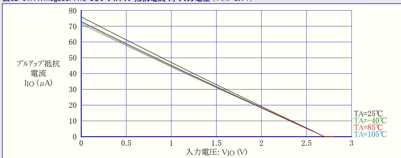
図32-61. ATmega88PA:I/Oピンプルアップ抵抗電流 対 入力電圧 (VCC=2.7V)
