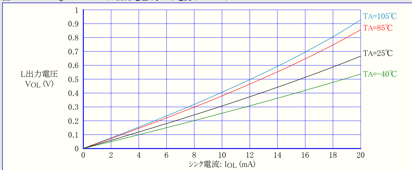
図31-257. ATmega168PA: I/Oピン出力電圧 対 シンク電流 (VCC=3V)
