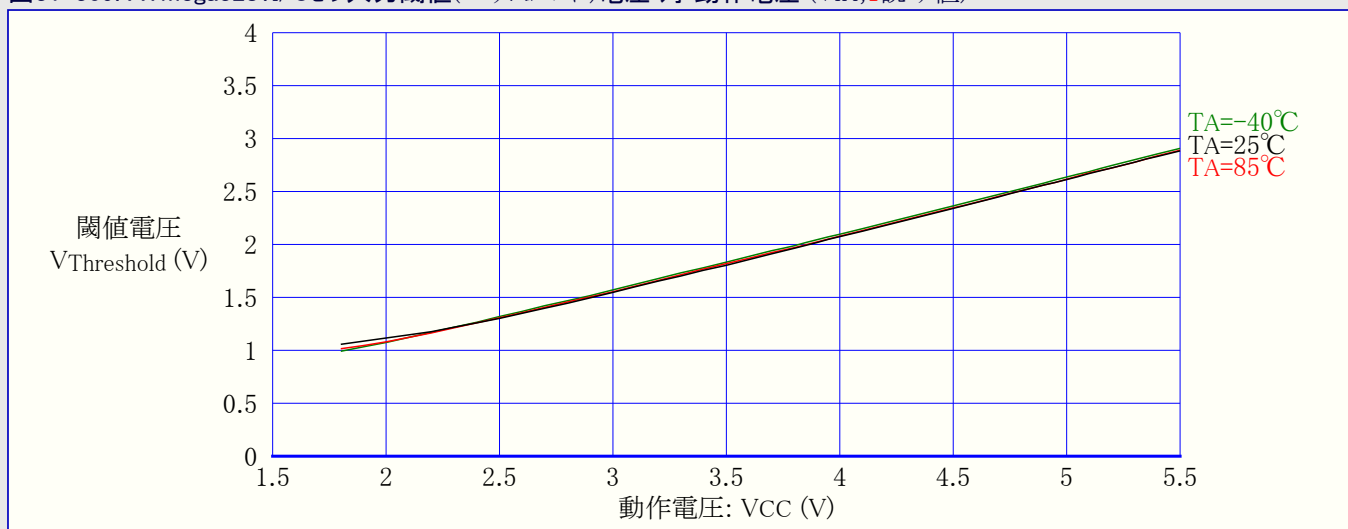
図31-309. ATmega328:I/Oピン入力閾値(スレッショルド)電圧 対 動作電圧 (VIH,1読み値)
