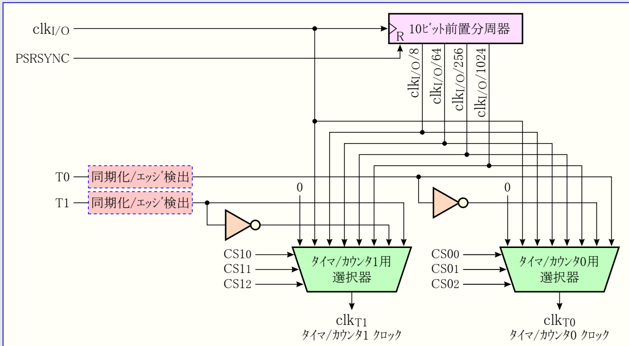
図17-2. タイマ/カウンタ0とタイマ/カウンタ1の前置分周器部構成図
