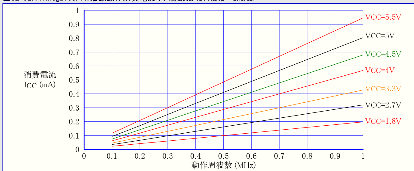
図32-92. ATmega168PA: 活動動作消費電流 対 周波数 (100kHz~1MHz)
