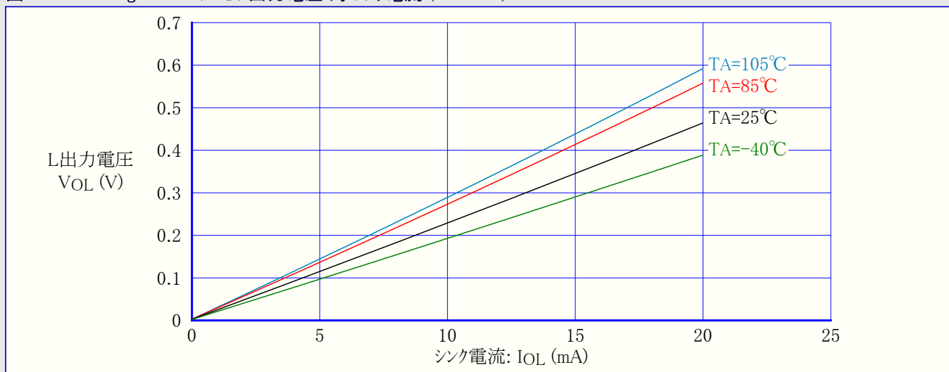
図32-67. ATmega88PA: I/Oピン出力電圧 対 シンク電流 (VCC=5V)
