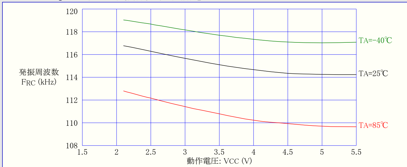
図31-320. ATmega328: ウォッチドッグ発振器周波数 対 動作電圧
