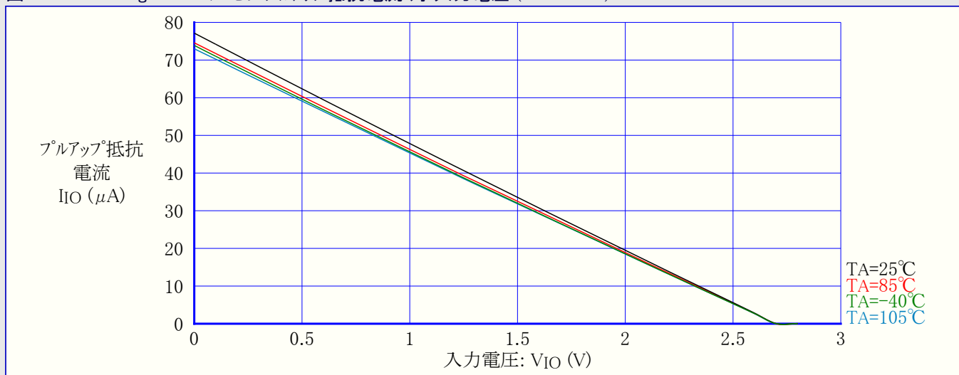
図31-347. ATmega328P:I/Oピンプルアップ抵抗電流 対 入力電圧 ( V_{CC}=2.7V )
