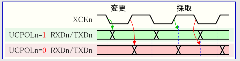
図20-3. 同期動作XCKnタイミング
