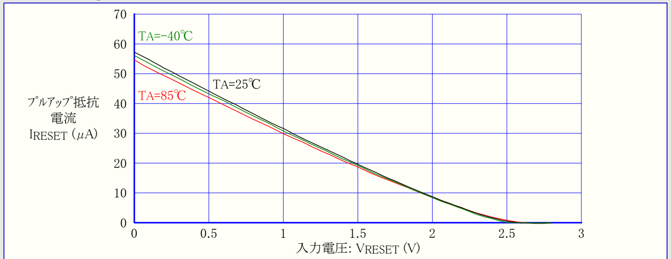
図31-303. ATmega328: RESETプルアップ抵抗電流 対 入力電圧 (VCC=2.7V)
