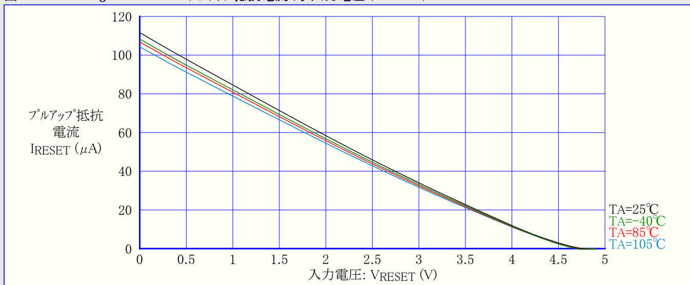
図32-159. ATmega328P: RESETプルアップ抵抗電流 対 入力電圧 (VCC=5V)
