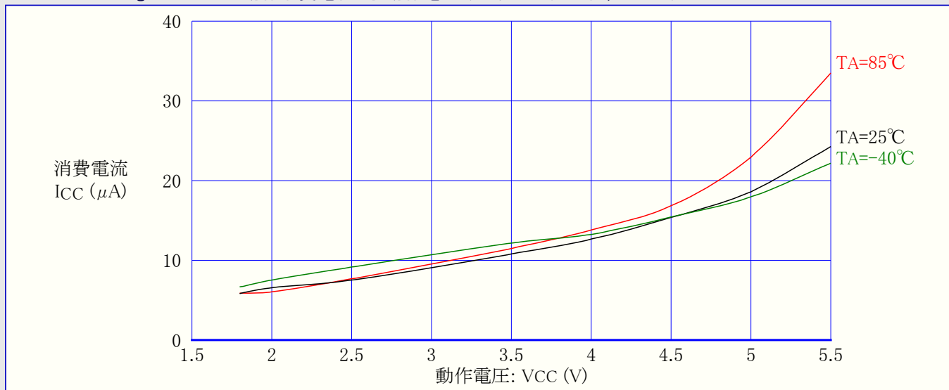
図31-102. ATmega88A: アイドル動作消費電流 対 動作電圧 (内蔵WDT発振器, 128kHz)
