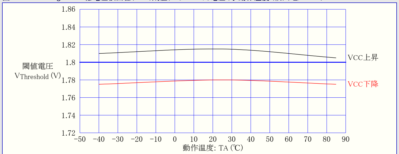
図31-220. ATmega168A: 低電圧検出器(BOD)閾値(スレッショルド)電圧 対 動作温度 (検出電圧1.8V)
