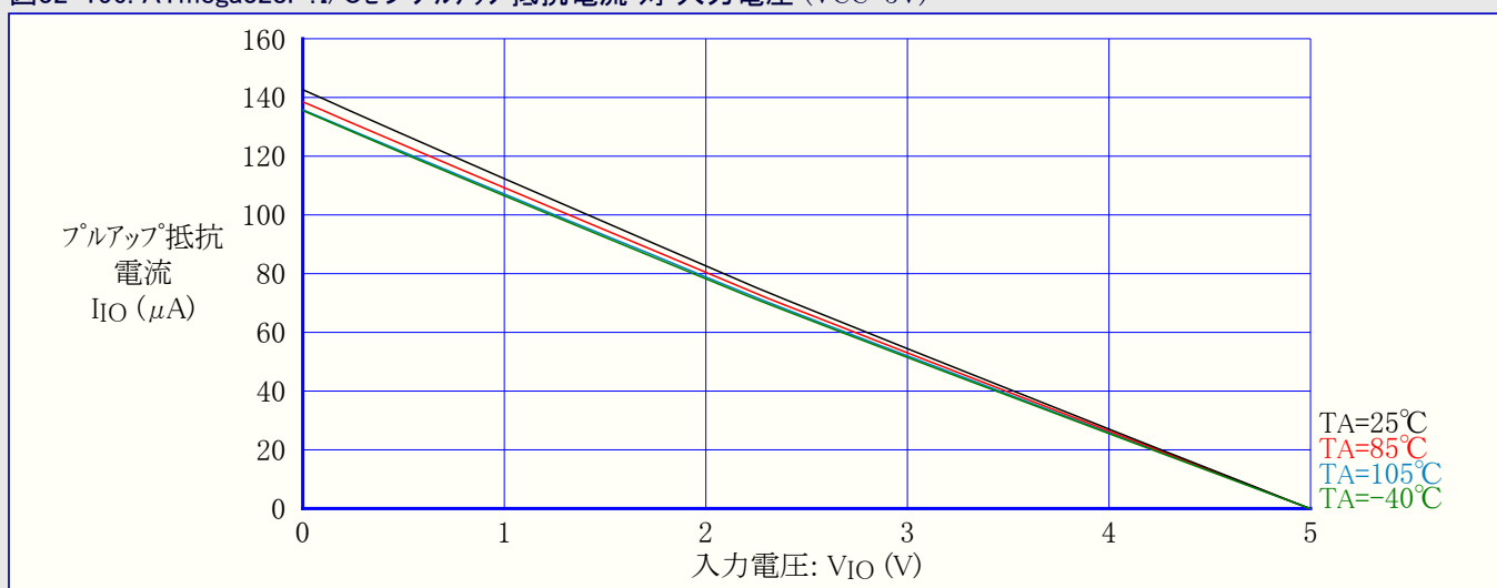
図32-156. ATmega328P:I/Oピンプルアップ抵抗電流 対 入力電圧 (VCC=5V)
