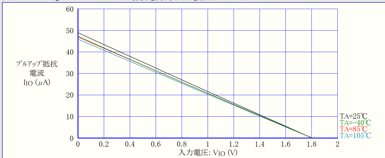
図31-156. ATmega88PA:I/Oピンプルアップ抵抗電流 対 入力電圧 (VCC=1.8V)
