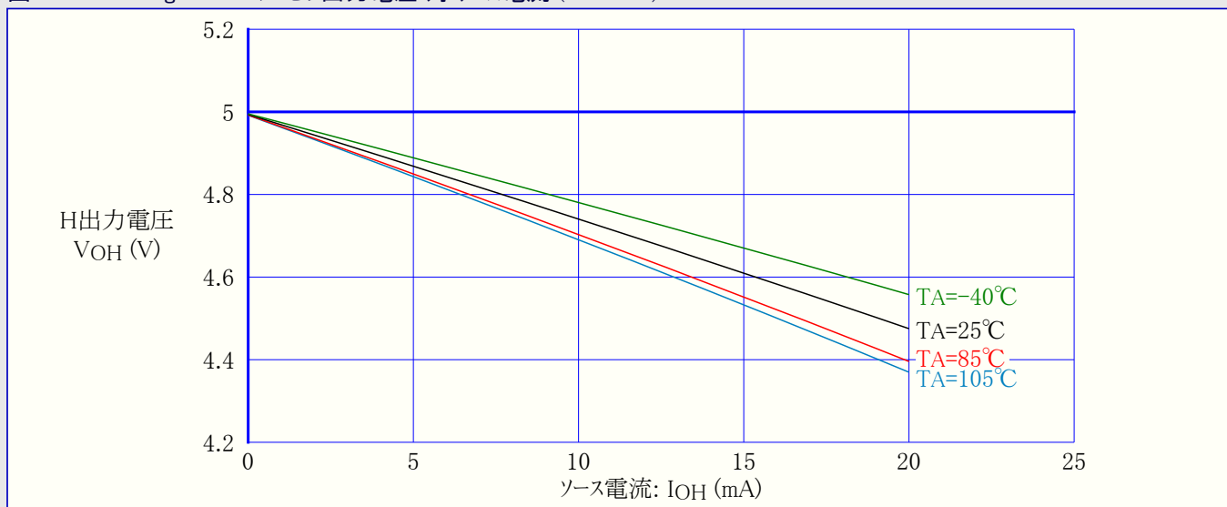
図32-69. ATmega88PA:I/Oピン出力電圧 対 ソース電流 (VCC=5V)
