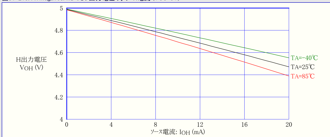
図31-213. ATmega168A:I/Oピン出力電圧 対 ソース電流 (VCC=5V)
