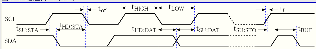
図29-5. 2線直列バス タイミング
