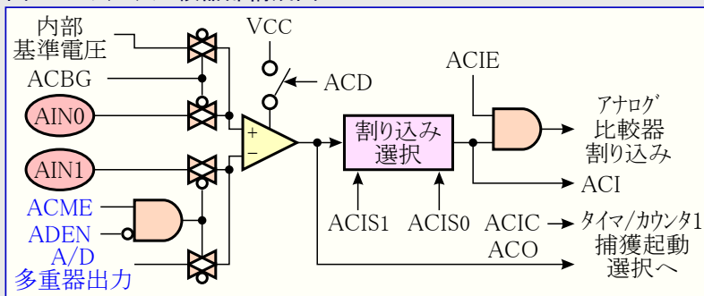
図23-1. アナログ比較器部構成図
