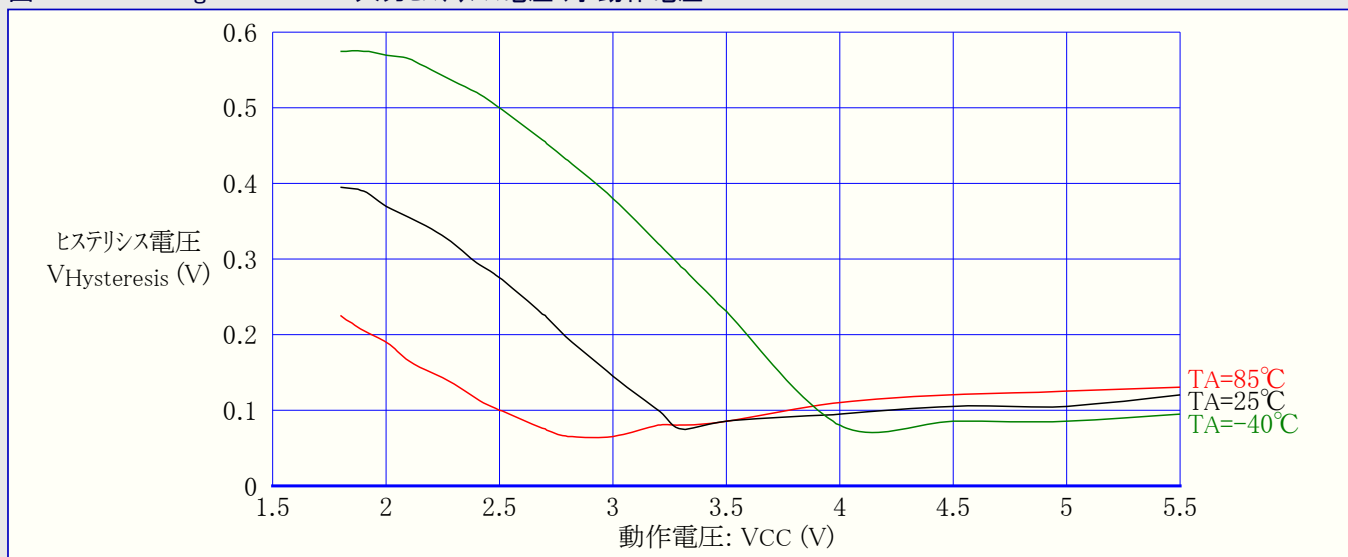
図31-124. ATmega88A: RESET入力ヒステリシス電圧 対 動作電圧
