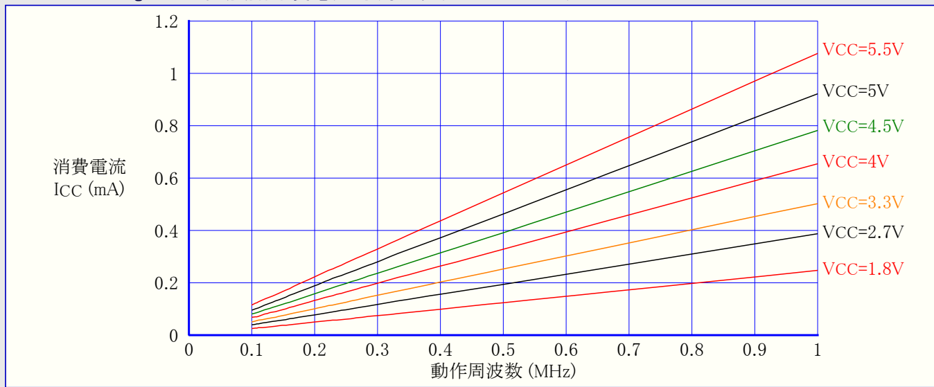
図31-332. ATmega328P: 活動動作消費電流 対 周波数 (100kHz~1MHz)
