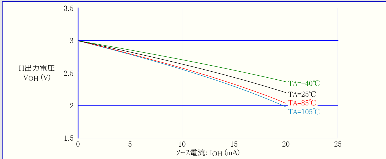
図31-164. ATmega88PA:I/Oピン出力電圧 対 ソース電流 (VCC=3V)
