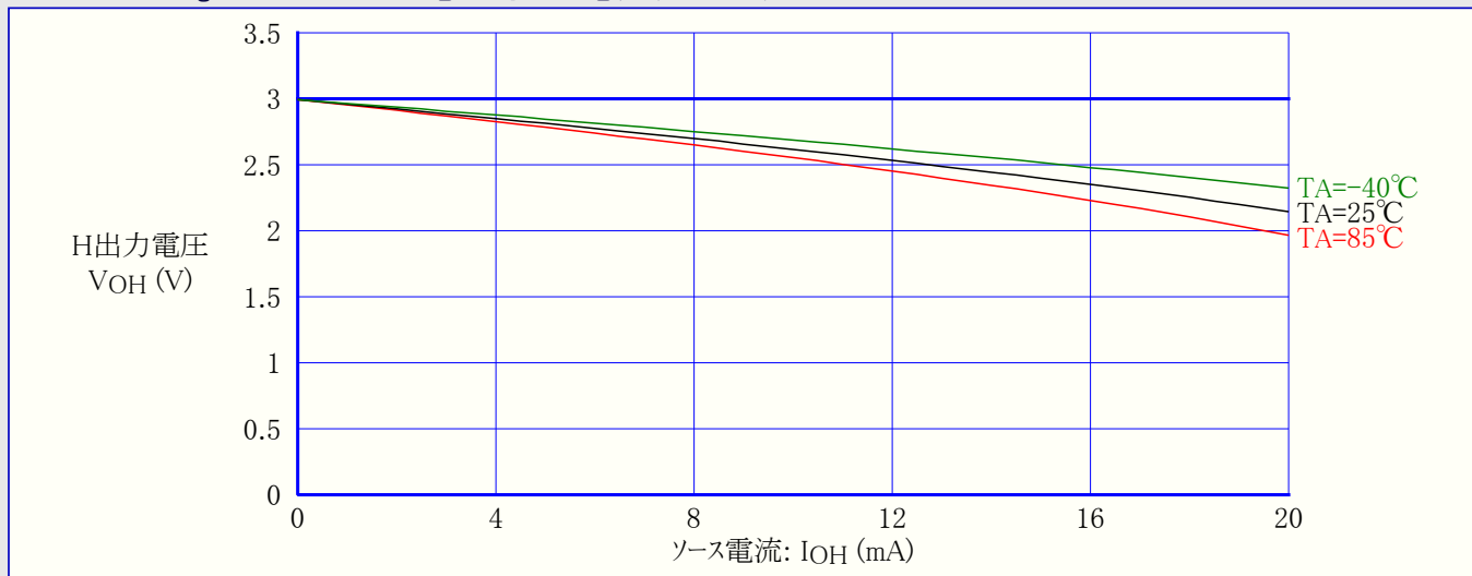
図31-23. ATmega48A:I/Oピン出力電圧 対 ソース電流 (VCC=3V)
