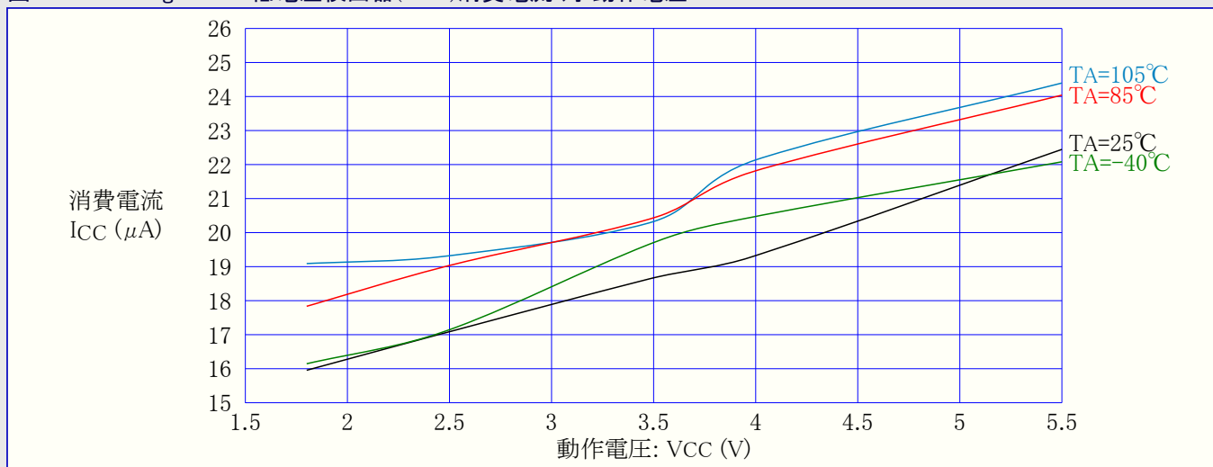
図31-90. ATmega48PA: 低電圧検出器(BOD)消費電流 対 動作電圧
