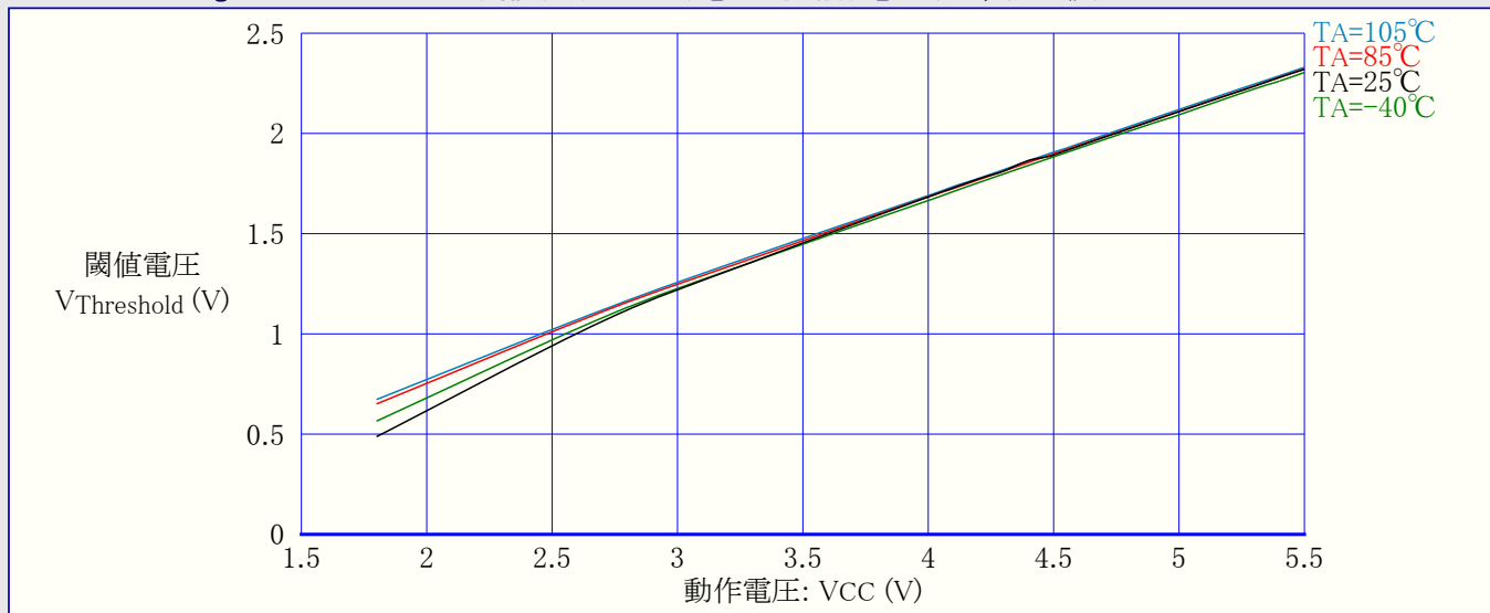
図31-262. ATmega168PA:I/Oピン入力閾値(スレッショルド)電圧 対 動作電圧 (VIL,0読み値)
