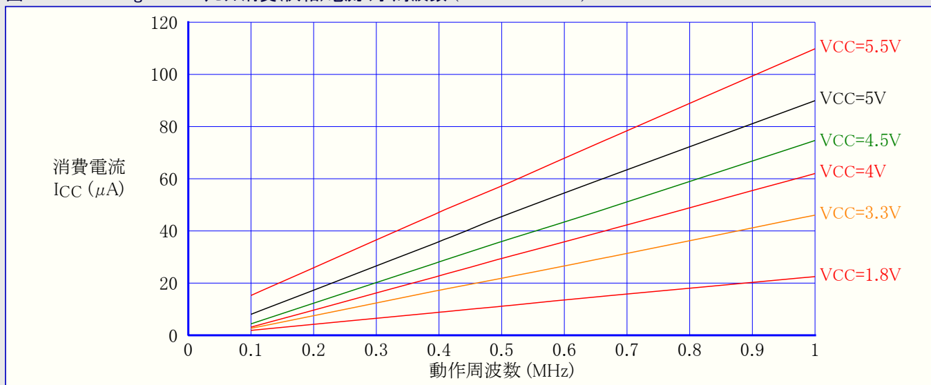
図31-187. ATmega88PA: リセット消費(供給)電流 対 周波数 (100kHz~1MHz)
