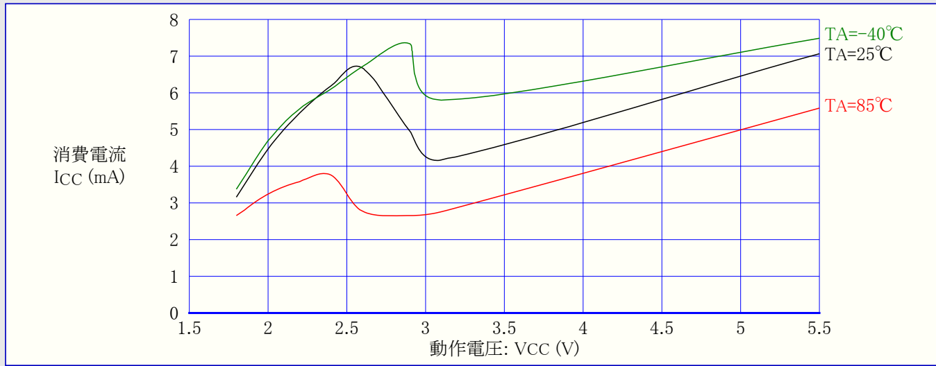
図31-138. ATmega88A:プログラミング電流 対 動作電圧
