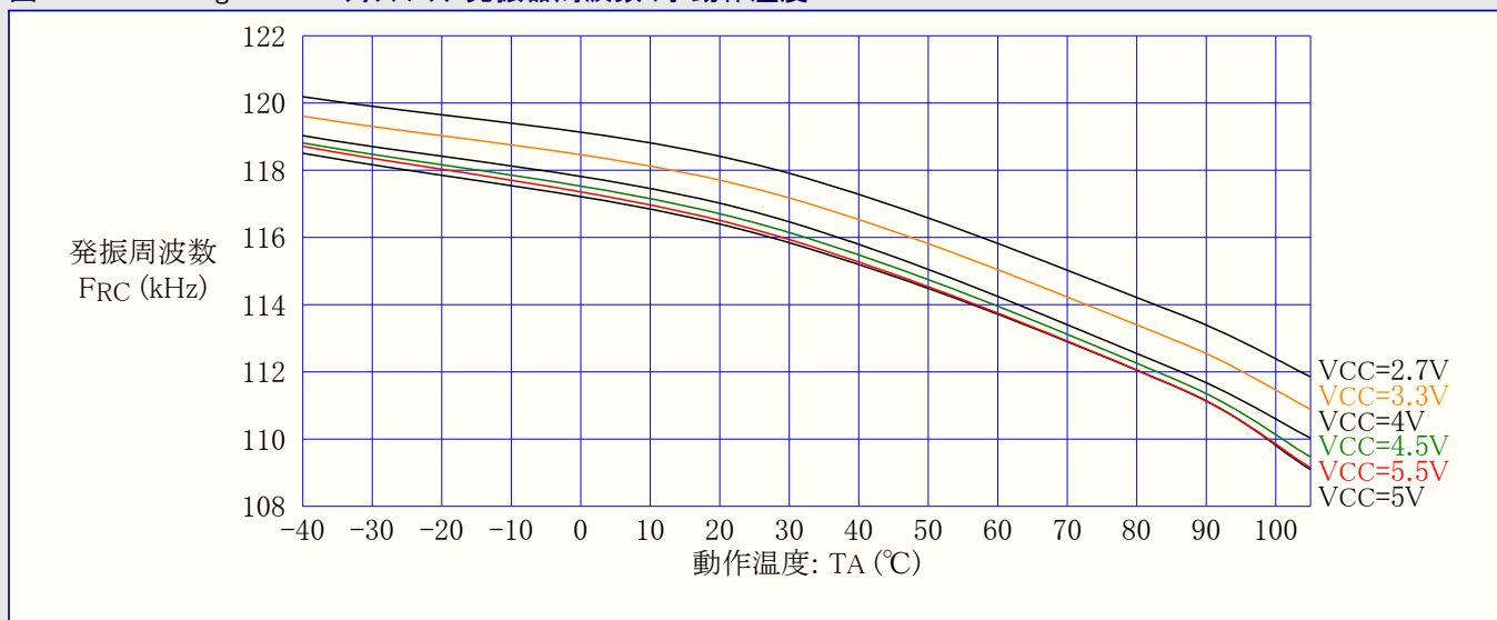
図32-127. ATmega168PA: ウォッチドッグ発振器周波数 対 動作温度
