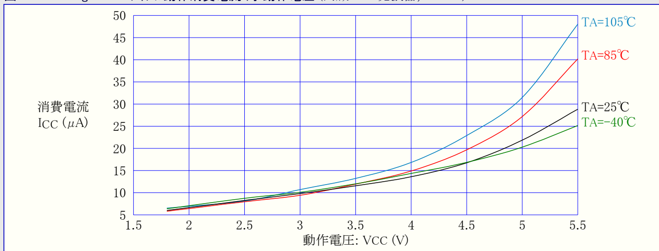
図32-8. ATmega48PA: アイドル動作消費電流 対 動作電圧 (内蔵WDT発振器, 128kHz)
