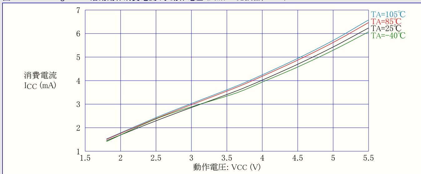
図31-336. ATmega328P: 活動動作消費電流 対 動作電圧 (内蔵RC発振器, 8MHz)
