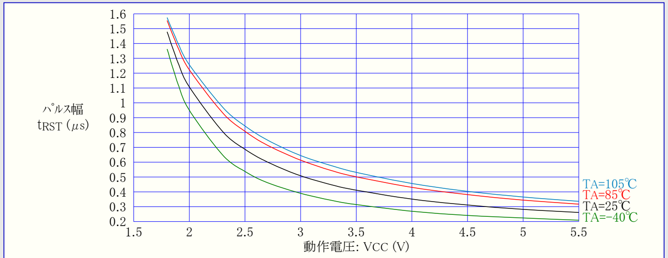
図32-46. ATmega48PA:最小リセットパルス幅 対 動作電圧
