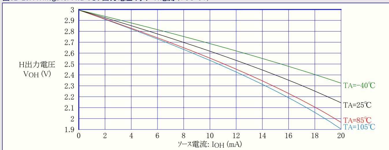
図32-23. ATmega48PA: I/Oピン出力電圧 対 ソース電流 (VCC=3V)
